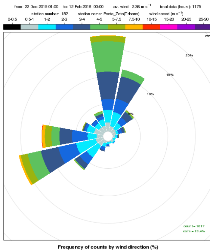
Figura 2: rosa dei venti registrati presso la stazione meteorologica di Tribano nel periodo 22 dicembre 2015 - 11 febbraio 2016
