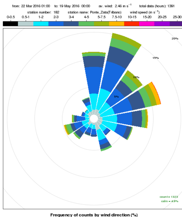
Figura 4: rosa dei venti registrati presso la stazione meteorologica di Tribano nel periodo 22 marzo - 18 maggio 2016
