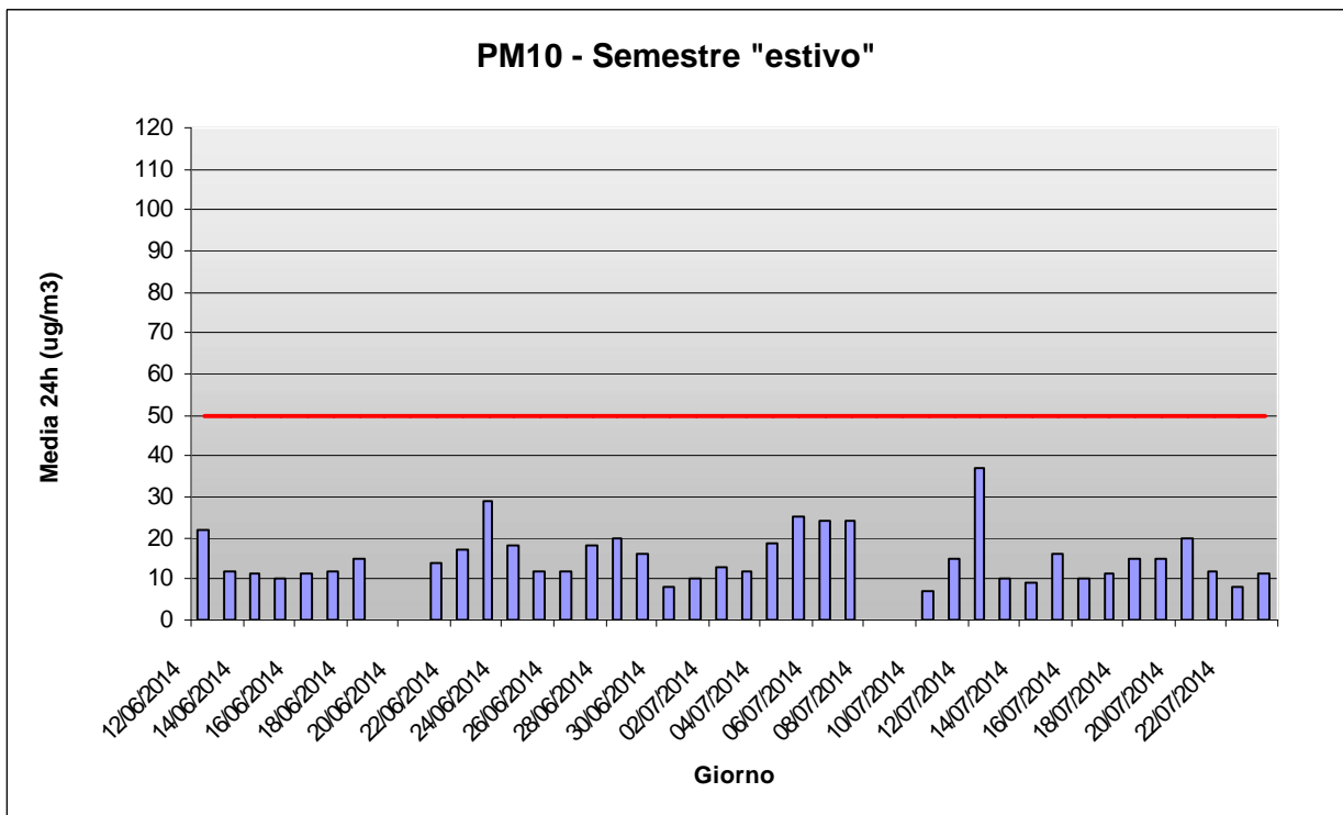
Polveri: andamento della media giornaliera, nel periodo dal 16/06/2014 al 27/07/2014
