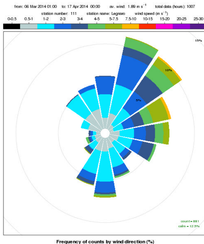
Figura 3. Rosa dei venti registrati presso la stazione meteorologica di Legnaro nel periodo 6 marzo – 16 aprile 2014
