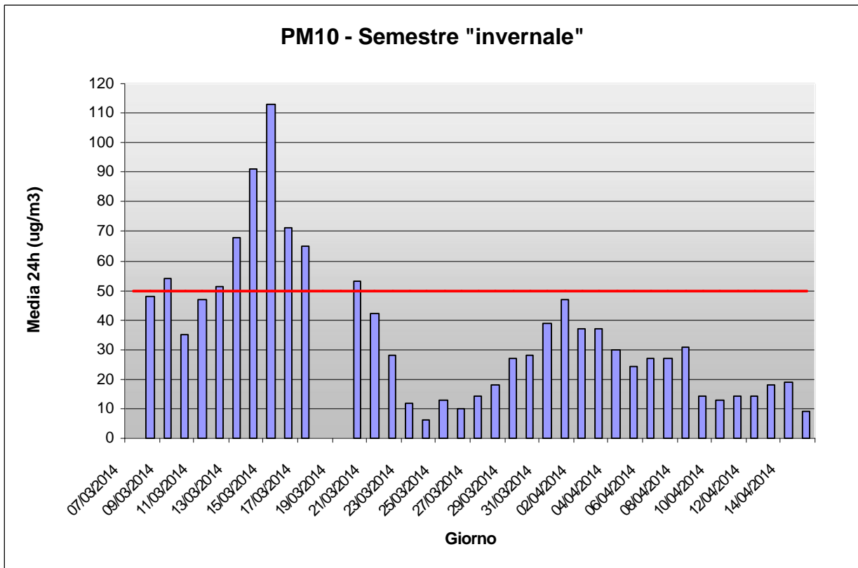
Polveri: andamento della media giornaliera, nel periodo dal 06/03/2014 al 16/04/2014
