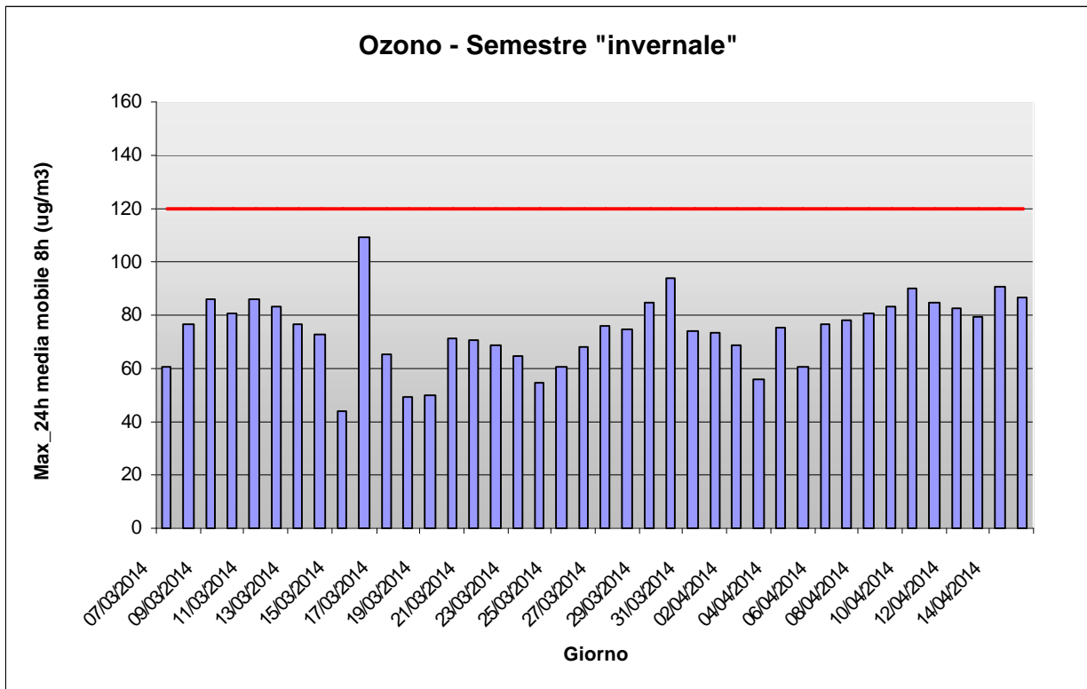
Ozono: andamento della massima media mobile giornaliera su 8h, nel periodo dal 06/03/2014 al 16/04/2014
