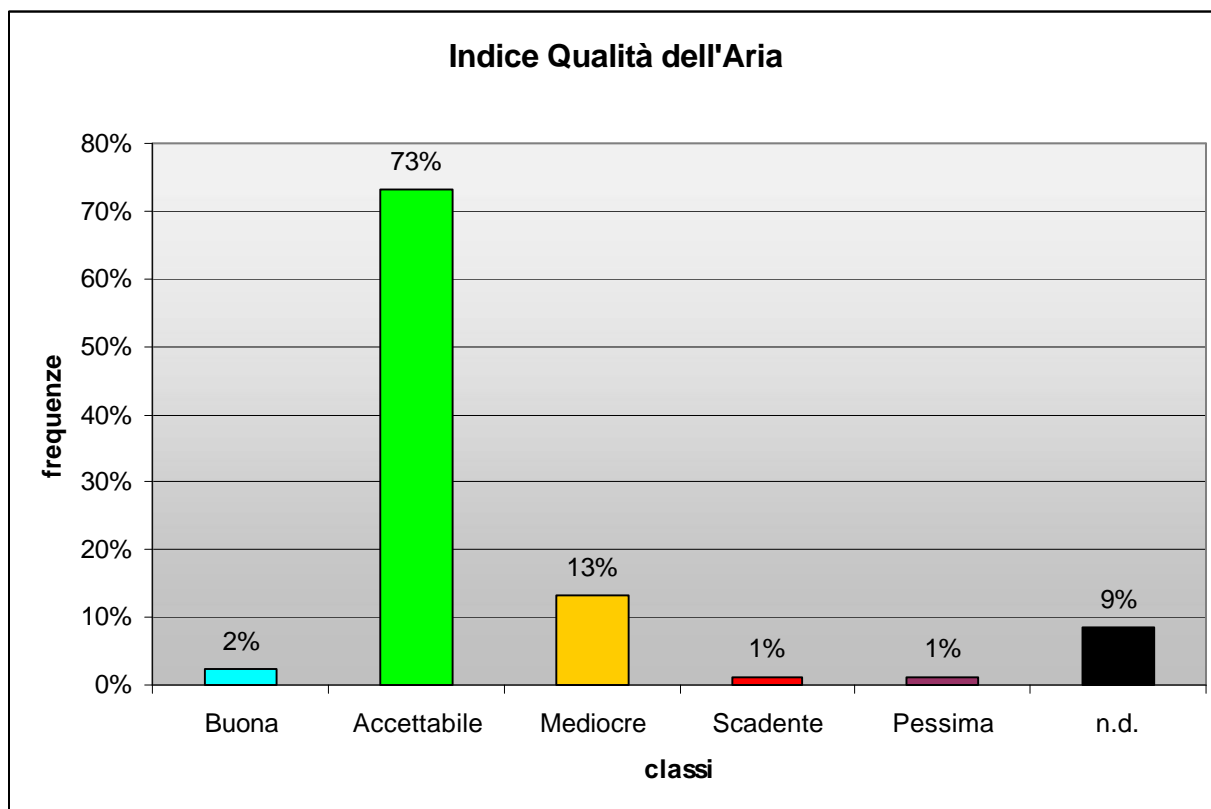
Figura 6. Andamento dell'Indice di Qualità dell'Aria per la campagna di Noventa Padovana (n.d. indica "dato non disponibile")
