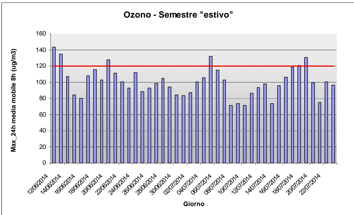
Ozono: andamento della massima media mobile giornaliera su 8h, nel periodo dal 16/06/2014 al 27/07/2014
