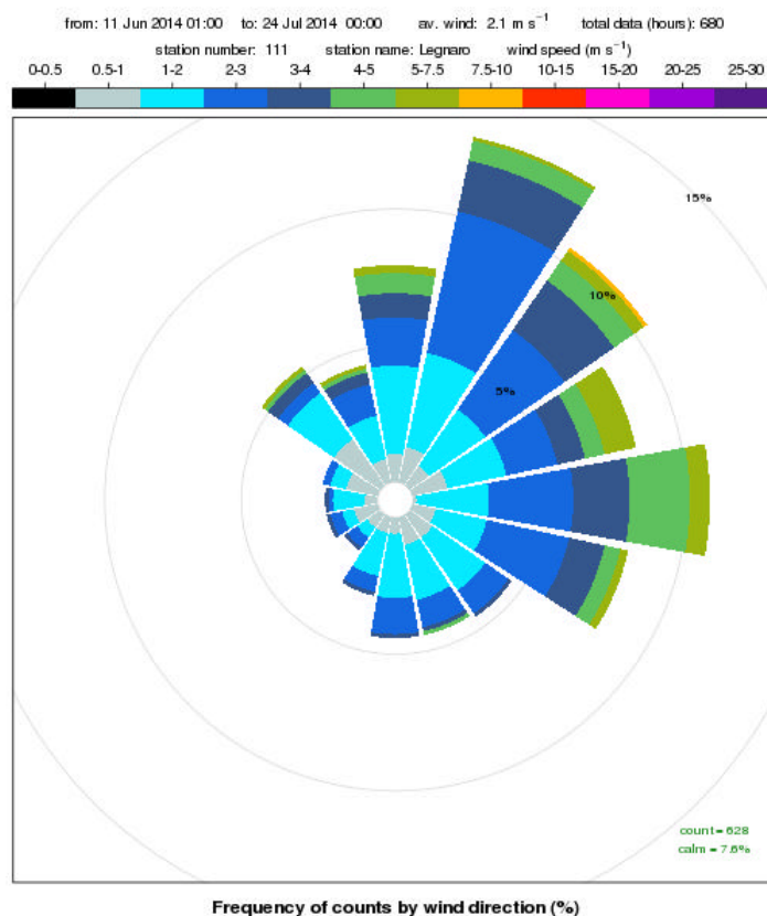
Figura 5. Rosa dei venti registrati presso la stazione meteorologica di Legnaro nel periodo 11 giugno -24 luglio 2014
