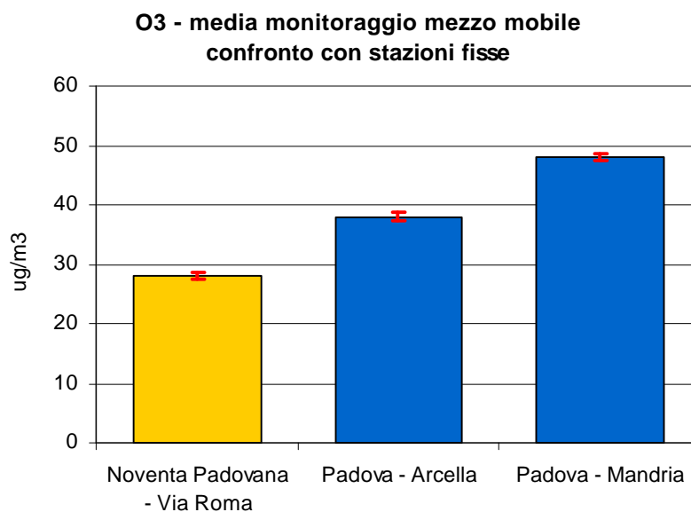
Figura 2.3 Ozono (O 3 ): concentrazione media rilevata durante il monitoraggio in Via Roma nel Comune di Noventa Padovana; le barre indicano l'errore standard della media.
