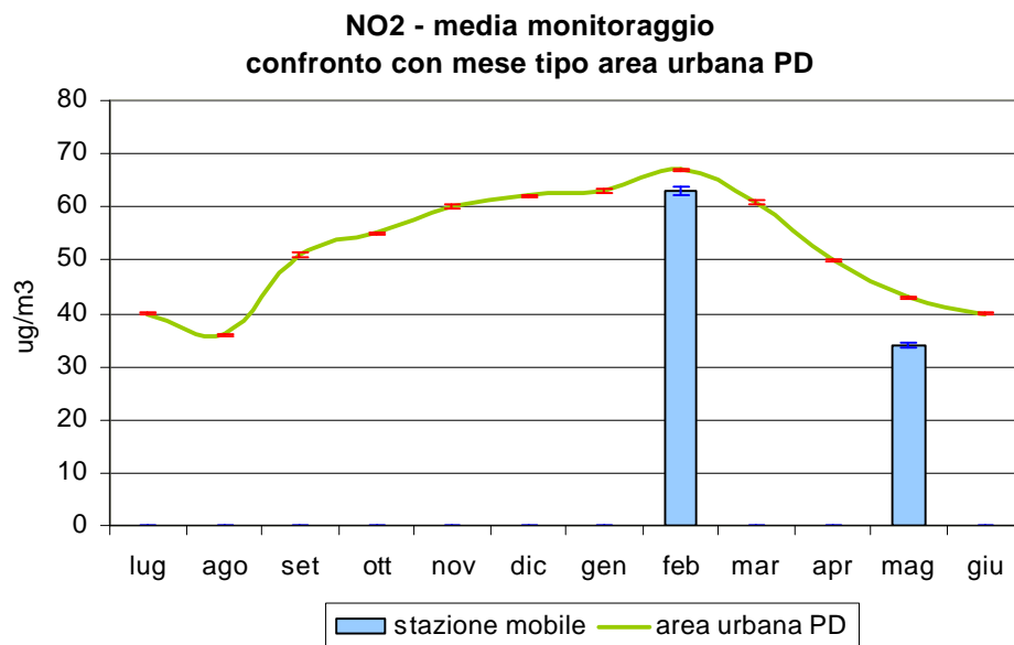
Figura 3.3 Biossido di azoto (NO 2 ): confronto delle concentrazioni medie rilevate durante il monitoraggio in Via Roma nel Comune di Noventa Padovana, con l'andamento caratteristico del 'mese tipo' ricavato dalla serie storica nell'area urbana di Padova; le barre indicano l'errore standard della media.
