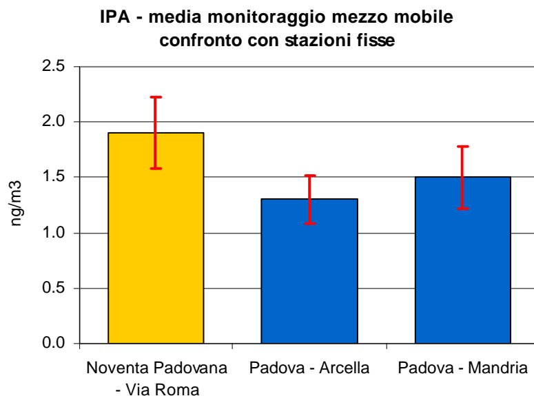
Figura 2.6 Benzo(a)pirene (IPA): concentrazione media rilevata durante il monitoraggio dal 14/01/10 al 23/02/10 e dal 29/04/10 al 24/05/10 in Via Roma nel Comune di Noventa Padovana; le barre indicano l'errore standard della media.
