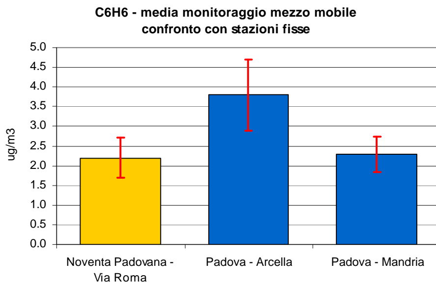
Figura 2.7 Benzene (C 6 H 6 ): concentrazione media rilevata durante il monitoraggio in Via Roma nel Comune di Noventa Padovana; le barre indicano l'errore standard della media.
