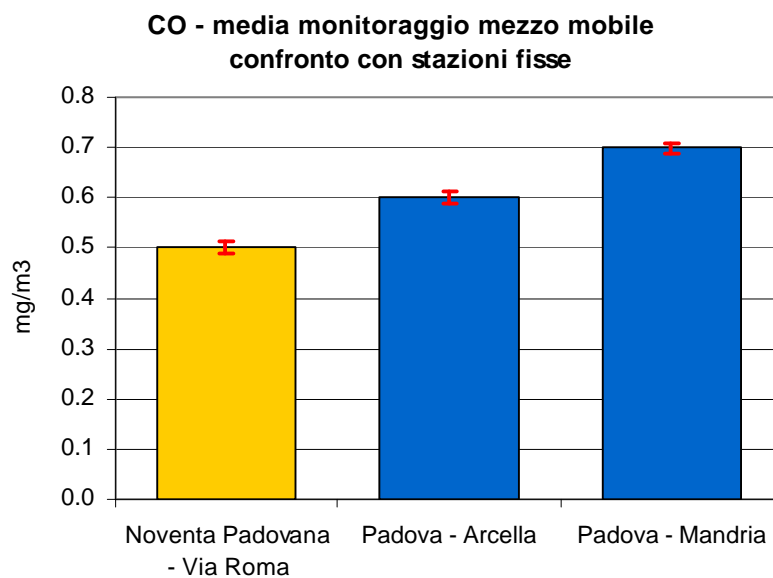
Figura 2.2 Monossido di carbonio (CO): concentrazione media rilevata durante il monitoraggio in Via Roma nel Comune di Noventa Padovana; le barre indicano l'errore standard della media.
