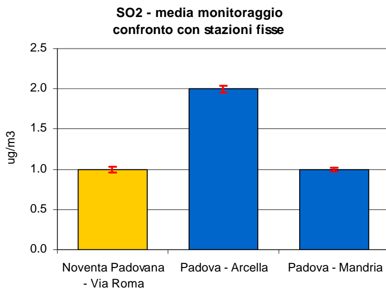
Figura 2.1 Biossido di zolfo (SO 2 ): concentrazione media rilevata durante il monitoraggio dal 14/01/10 al 23/02/10 e dal 29/04/10 al 24/05/10 in Via Roma nel Comune di Noventa Padovana; le barre indicano l'errore standard della media.
