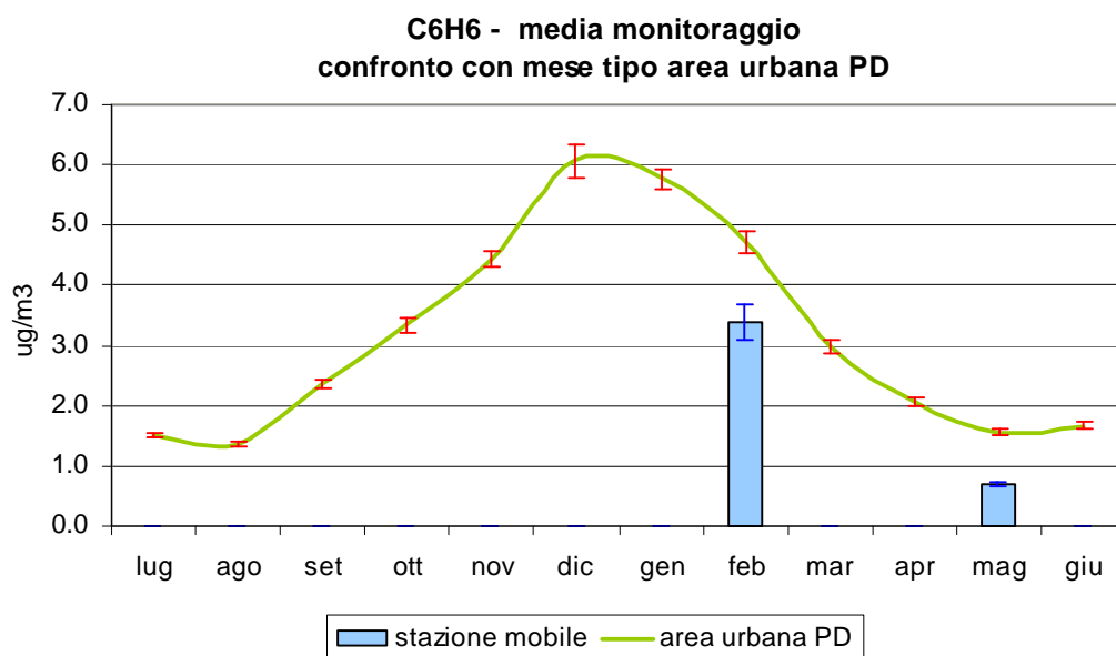
Figura 3.7 Benzene ( C_6H_6 ): confronto delle concentrazioni medie rilevate durante il monitoraggio in Via Roma nel Comune di Noventa Padovana, con l'andamento caratteristico del 'mese tipo' ricavato dalla serie storica nell'area urbana di Padova; le barre indicano l'errore standard della media.
