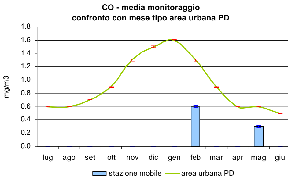
Figura 3.2 Monossido di carbonio (CO): confronto delle concentrazioni medie rilevate durante il monitoraggio in Via Roma nel Comune di Noventa Padovana, con l'andamento caratteristico del 'mese tipo' ricavato dalla serie storica nell'area urbana di Padova; le barre indicano l'errore standard della media.
