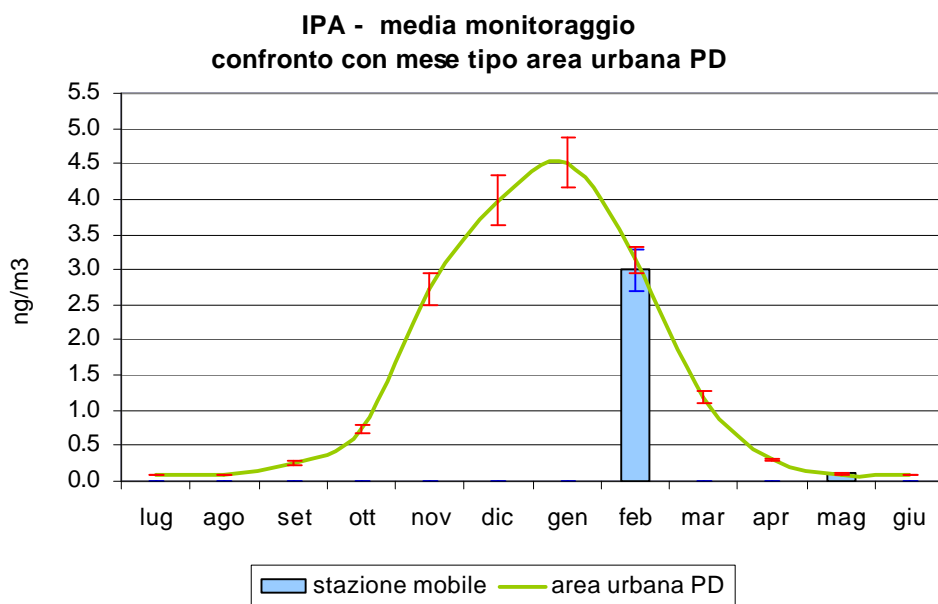
Figura 3.6 Benzo(a)pirene (IPA): confronto delle concentrazioni medie rilevate durante il monitoraggio in Via Roma nel Comune di Noventa Padovana, con l'andamento caratteristico del 'mese tipo' ricavato dalla serie storica nell'area urbana di Padova; le barre indicano l'errore standard della media.
