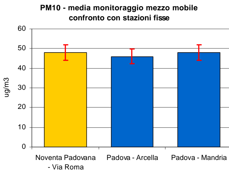
Figura 2.5 Polveri fini (PM 10 ): concentrazione media durante il monitoraggio dal 14/01/10 al 23/02/10 e dal 29/04/10 al 24/05/10 nel Comune di Noventa Padovana; le barre indicano l'errore standard della media.
