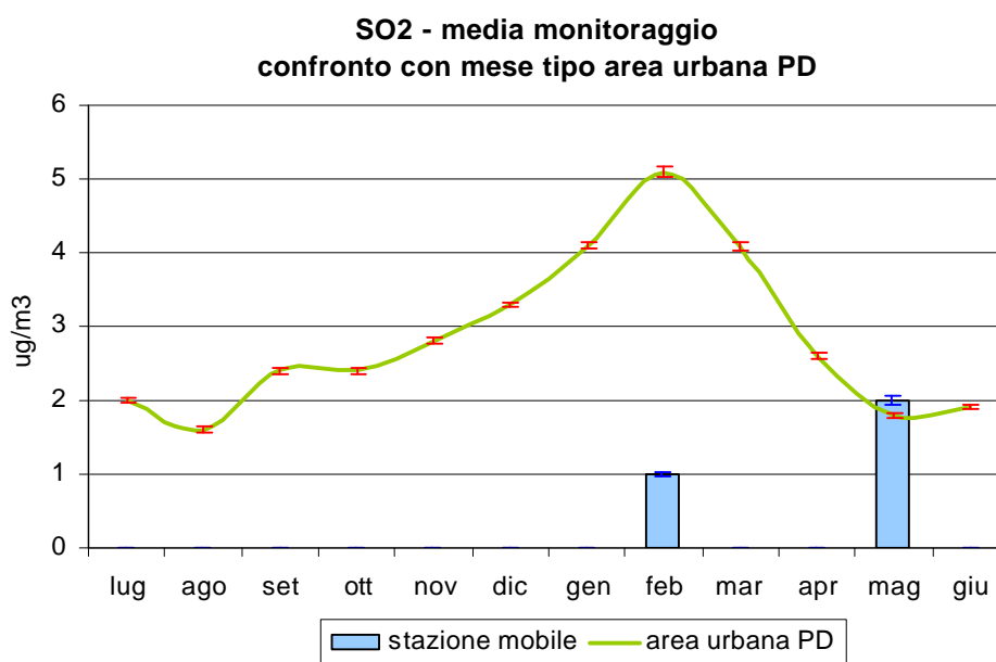
Figura 3.1 Biossido di zolfo (SO 2 ): confronto delle concentrazioni medie rilevate durante il monitoraggio in Via Roma nel Comune di Noventa Padovana, con l’andamento caratteristico del ‘mese tipo’ ricavato dalla serie storica nell’area urbana di Padova; le barre indicano l’errore standard della media.
