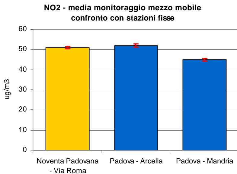
Figura 2.4 Biossido di azoto (NO 2 ): concentrazione media rilevata durante il monitoraggio in Via Roma nel Comune di Noventa Padovana; le barre indicano l'errore standard della media.
