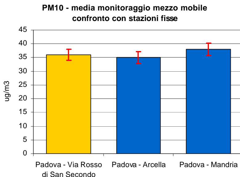
Figura 2.4 Polveri fini (PM 10 ): concentrazione media rilevata durante il monitoraggio dal 13/01/09 al 09/02/09 e dal 24/04/09 al 11/06/09 in Via Rosso San Secondo nel Comune di Padova e confronto con i periodi corrispondenti presso le stazioni fisse di Arcella e Mandria; le barre indicano l'errore standard della media.
