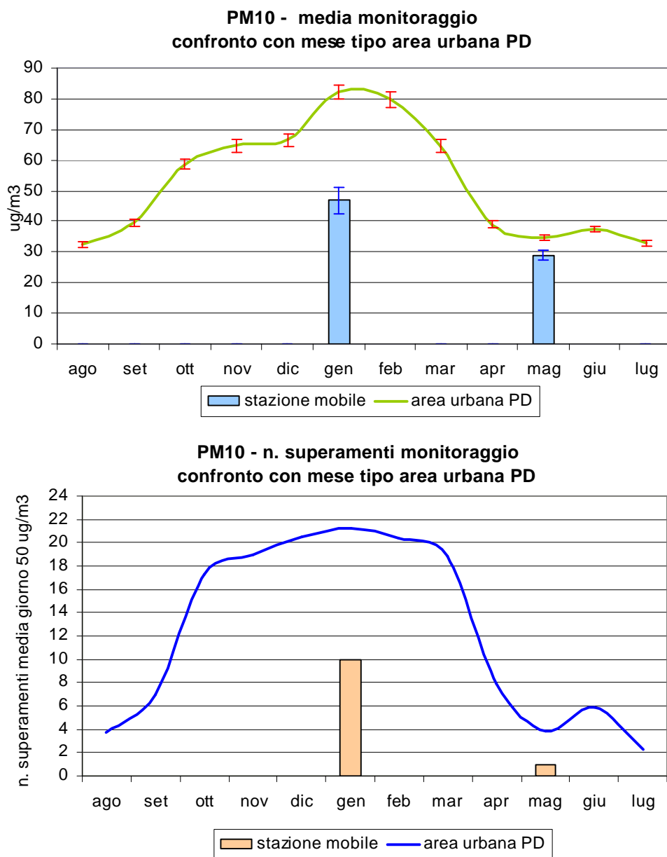
Figura 3.3 Polveri fini ( PM_{10} ): confronto delle concentrazioni medie e del numero di superamenti del valore del limite di protezione della salute ( 50 \mu\text{g}/\text{m}^3 ) rilevate durante il monitoraggio in Via Rosso San Secondo con l'andamento caratteristico del 'mese tipo' ricavato dalla serie storica nell'area urbana di Padova; per i valori di concentrazione mensile le barre indicano l'errore standard della media.
