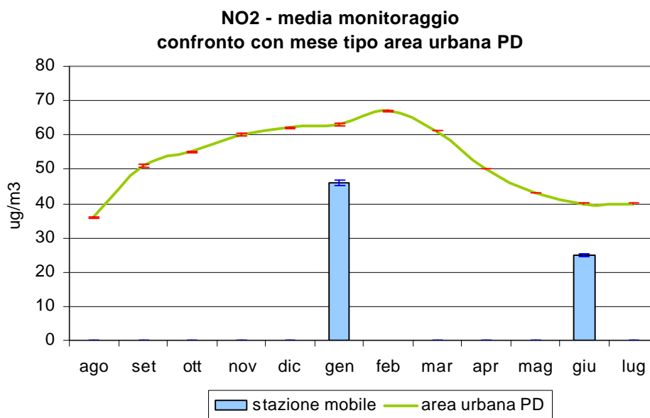
Figura 3.4 Biossido di azoto (NO 2 ): confronto delle concentrazioni medie rilevate durante il monitoraggio in Via Rosso San Secondo con l'andamento caratteristico del 'mese tipo' ricavato dalla serie storica nell'area urbana di Padova; le barre indicano l'errore standard della media.
