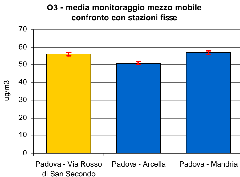
Figura 2.2 Ozono ( O_3 ): concentrazione media rilevata durante in Via Rosso San Secondo nel Comune di Padova e confronto con i periodi corrispondenti presso le stazioni fisse di Arcella e Mandria; le barre indicano l'errore standard della media.
