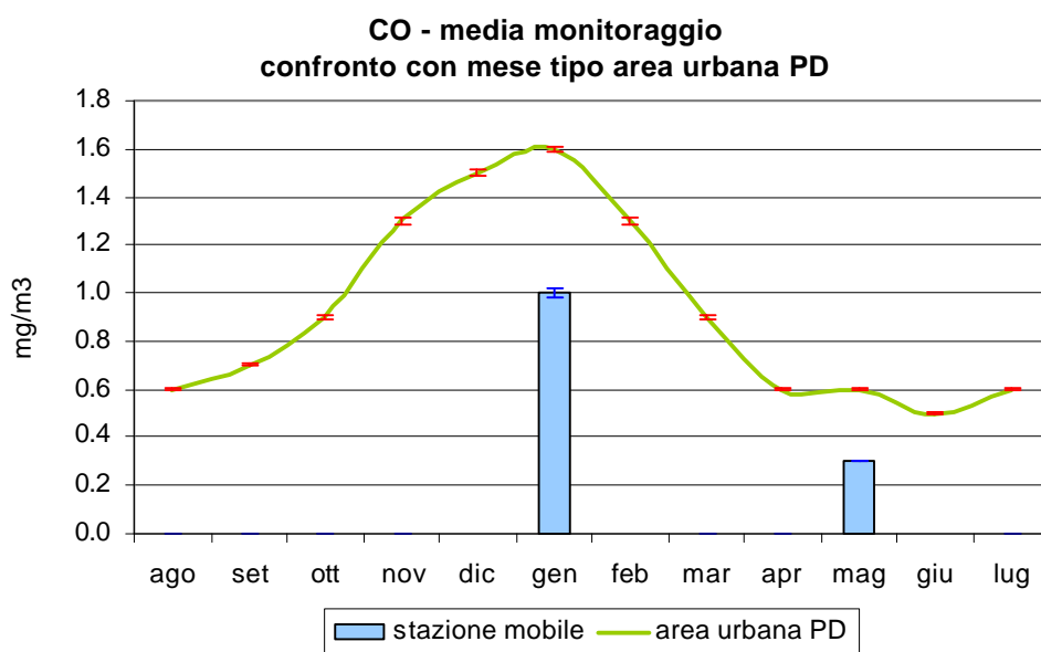
Figura 3.1 Monossido di carbonio (CO): confronto delle concentrazioni medie rilevate durante il monitoraggio in Via Rosso San Secondo con l'andamento caratteristico del 'mese tipo' ricavato dalla serie storica nell'area urbana di Padova; le barre indicano l'errore standard della media.
