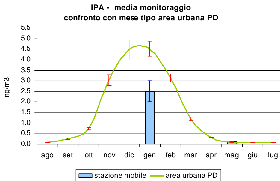
Figura 3.5 Benzo(a)pirene (IPA): confronto delle concentrazioni medie rilevate durante il monitoraggio in Via Rosso San Secondo con l'andamento caratteristico del 'mese tipo' ricavato dalla serie storica nell'area urbana di Padova; le barre indicano l'errore standard della media.
