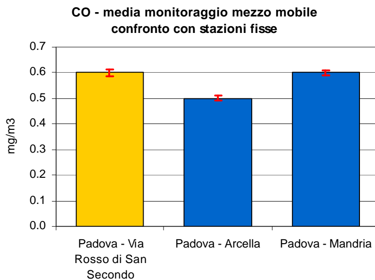
Figura 2.1 Monossido di carbonio (CO): concentrazione media rilevata durante il monitoraggio dal 13/01/09 al 09/02/09 e dal 24/04/09 al 11/06/09 in Via Rosso San Secondo nel Comune di Padova e confronto con i periodi corrispondenti presso le stazioni fisse di Arcella e Mandria; le barre indicano l'errore standard della media.
