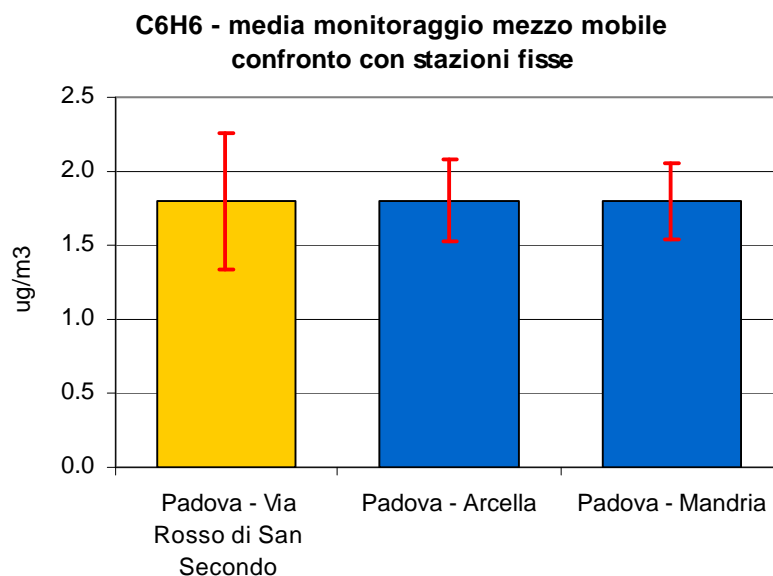
Figura 2.6 Benzene (C 6 H 6 ): concentrazione media rilevata durante il monitoraggio dal 13/01/09 al 09/02/09 e dal 24/04/09 al 11/06/09 in Via Rosso San Secondo nel Comune di Padova e confronto con i periodi corrispondenti presso le stazioni fisse di Arcella e Mandria; le barre indicano l'errore standard della media.
