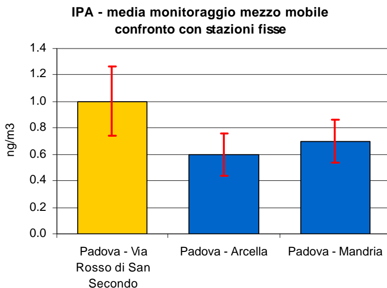
Figura 2.5 Benzo(a)pirene (IPA): concentrazione media rilevata durante il monitoraggio dal 13/01/09 al 09/02/09 e dal 24/04/09 al 11/06/09 in Via Rosso San Secondo nel Comune di Padova e confronto con i periodi corrispondenti presso le stazioni fisse di Arcella e Mandria; le barre indicano l'errore standard della media.
