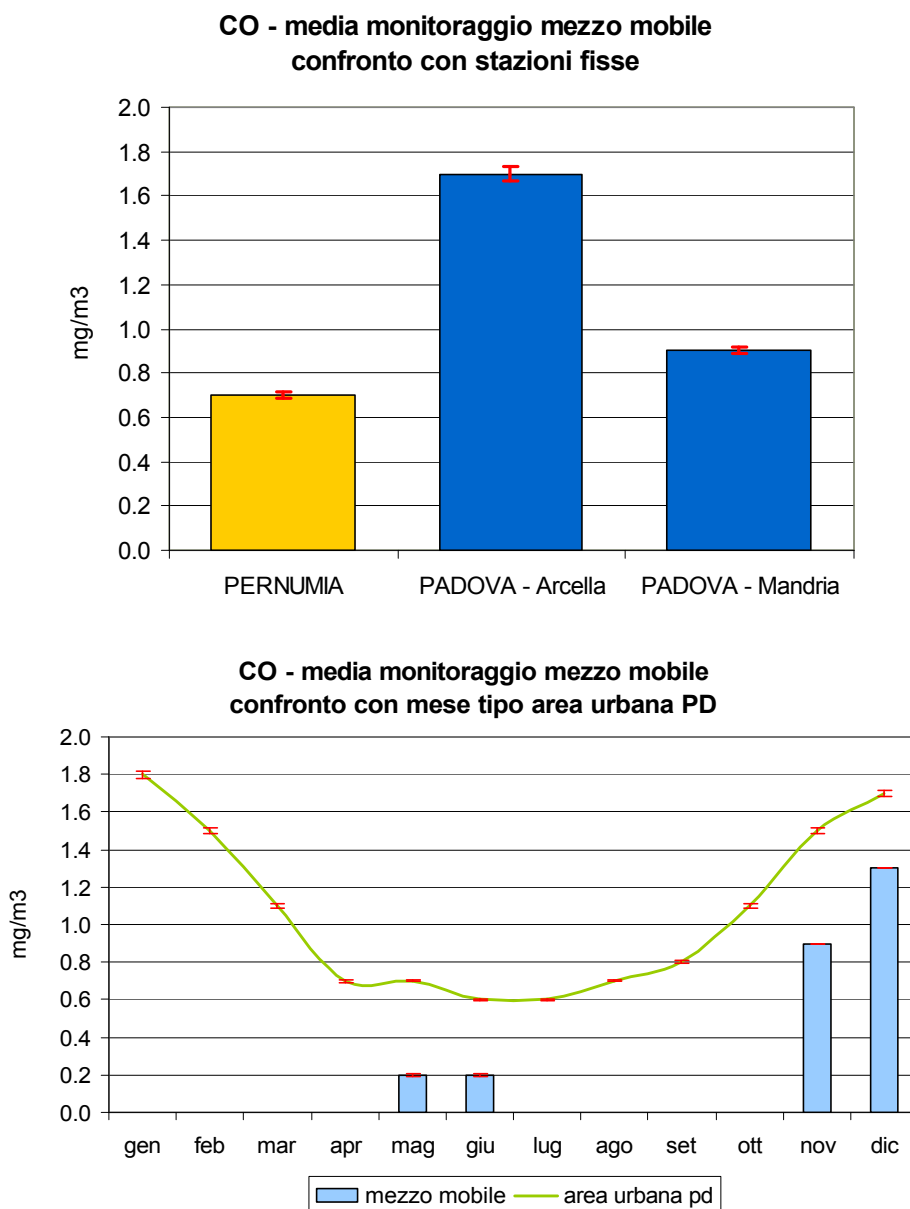
Figura 2.2 Monossido di carbonio (CO): concentrazione media rilevata durante il monitoraggio nel Comune di Pernumia; confronto con i periodi corrispondenti presso le stazioni fisse di Arcella e di Mandria nel Comune di Padova e con l'andamento caratteristico del 'mese tipo' ricavato dalla serie storica nell'area urbana di Padova; le barre indicano l'errore standard della media.
