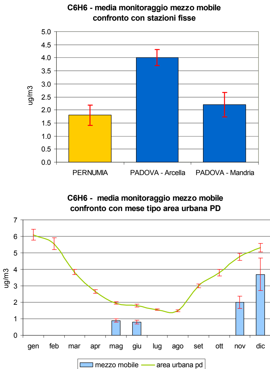
Figura 2.7 Benzene ( C_6H_6 ): concentrazione media rilevata durante il monitoraggio nel Comune di Pernumia; confronto con i periodi corrispondenti presso le stazioni fisse di Arcella e Mandria nel Comune di Padova e con l'andamento caratteristico del 'mese tipo' ricavato dalla serie storica nell'area urbana di Padova; le barre indicano l'errore standard della media.
