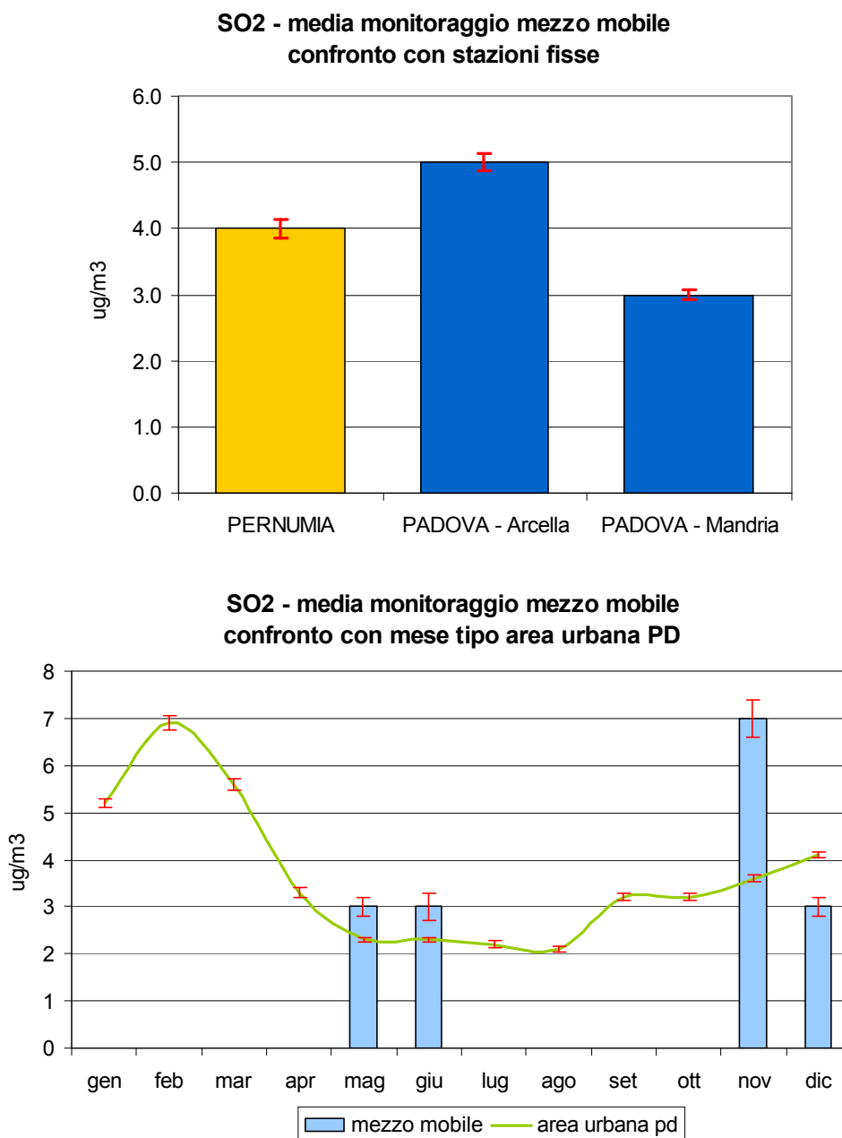
Figura 2.1 Biossido di zolfo (SO 2 ): concentrazione media rilevata durante il monitoraggio nel Comune di Pernumia; confronto con i periodi corrispondenti presso la stazioni fisse di Arcella e Mandria nel Comune di Padova e con l'andamento caratteristico del 'mese tipo' ricavato dalla serie storica nell'area urbana di Padova; le barre indicano l'errore standard della media.
