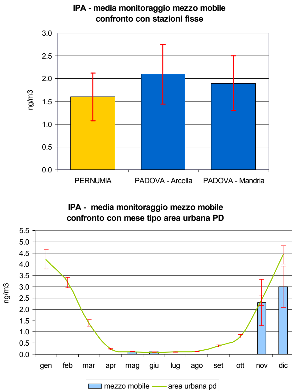
Figura 2.6 Benzo(a)pirene (IPA): concentrazione media rilevata durante il monitoraggio nel Comune di Pernumia; confronto con i periodi corrispondenti presso le stazioni fisse di Arcella e Mandria nel Comune di Padova e con l'andamento caratteristico del 'mese tipo' ricavato dalla serie storica nell'area urbana di Padova; le barre indicano l'errore standard della media.
