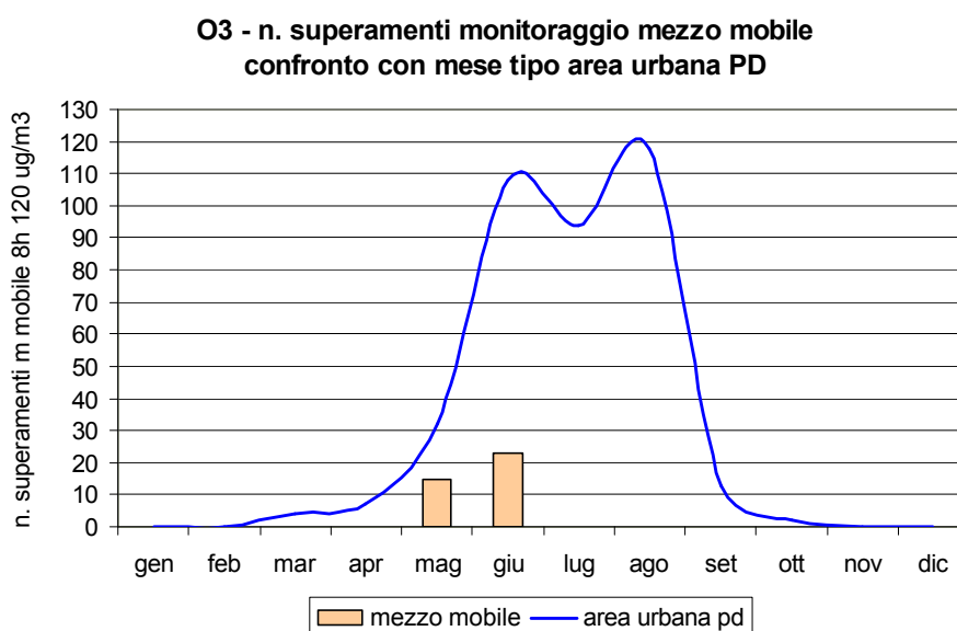
Figura 2.3 Ozono (O 3 ): concentrazione media e numero di superamenti rilevati durante il monitoraggio nel Comune di Pernumia; confronto con i periodi corrispondenti presso le stazioni fisse di Arcella e di Mandria nel Comune di Padova e con l'andamento caratteristico del 'mese tipo' ricavato dalla serie storica nell'area urbana di Padova; per i valori di concentrazione mensile le barre indicano l'errore standard della media.
