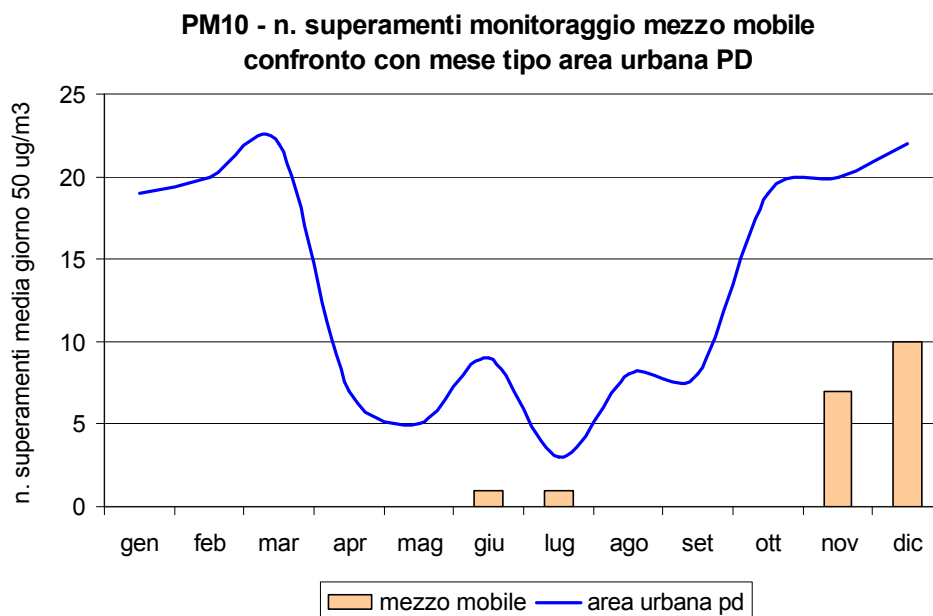
Figura 2.5 Polveri fini (PM 10 ): concentrazione media e numero di superamenti rilevati durante il monitoraggio nel Comune di Pernumia; confronto con i periodi corrispondenti presso le stazioni fisse di Arcella e Mandria nel Comune di Padova e con l'andamento caratteristico del 'mese tipo' ricavato dalla serie storica nell'area urbana di Padova; per i valori di concentrazione mensile le barre indicano l'errore standard della media.
