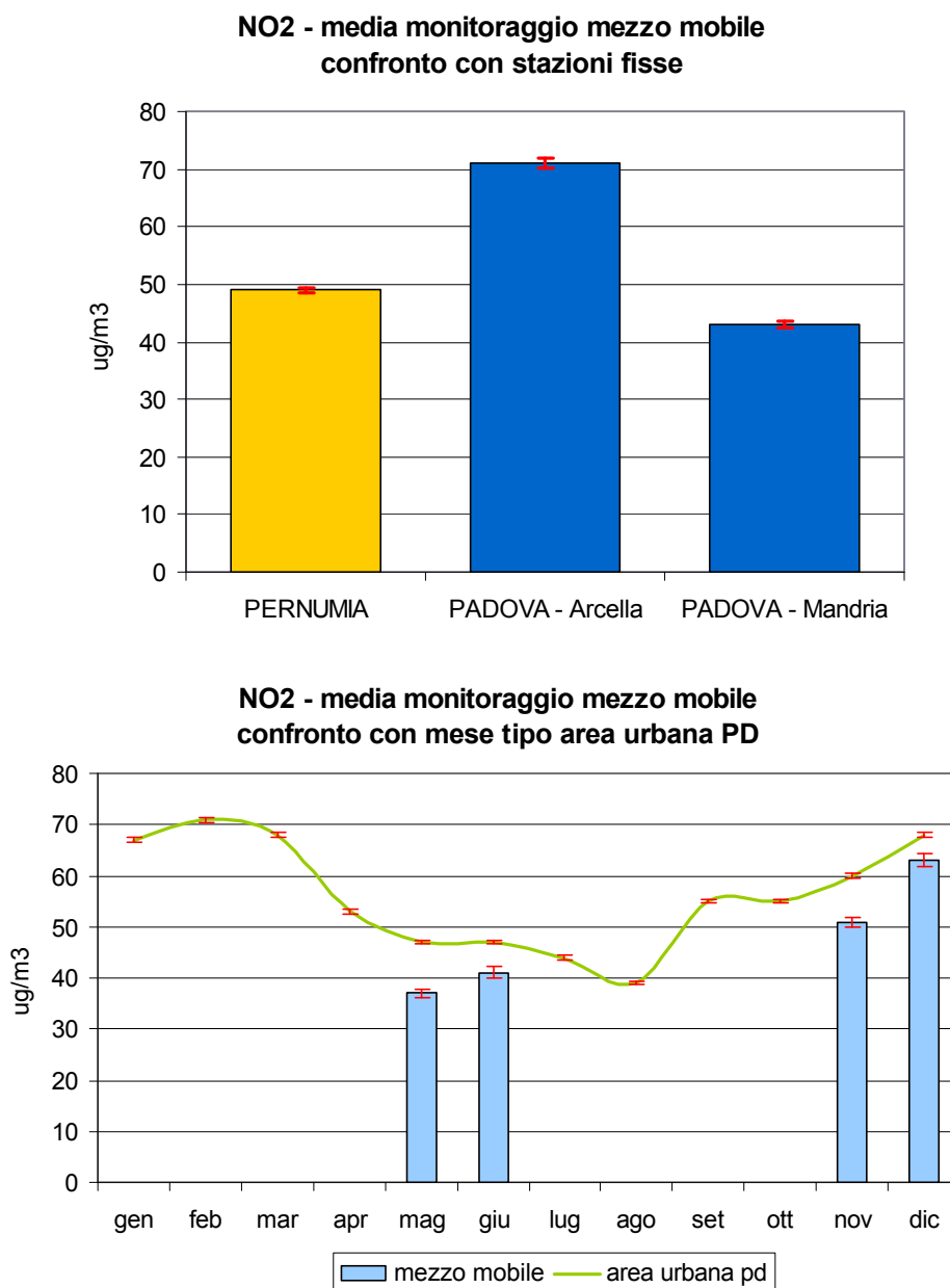
Figura 2.4 Biossido di azoto (NO 2 ): concentrazione media rilevata durante il monitoraggio nel Comune di Pernumia; confronto con i periodi corrispondenti presso le stazioni fisse di Arcella e Mandria nel Comune di Padova e con l'andamento caratteristico del 'mese tipo' ricavato dalla serie storica nell'area urbana di Padova; le barre indicano l'errore standard della media.
