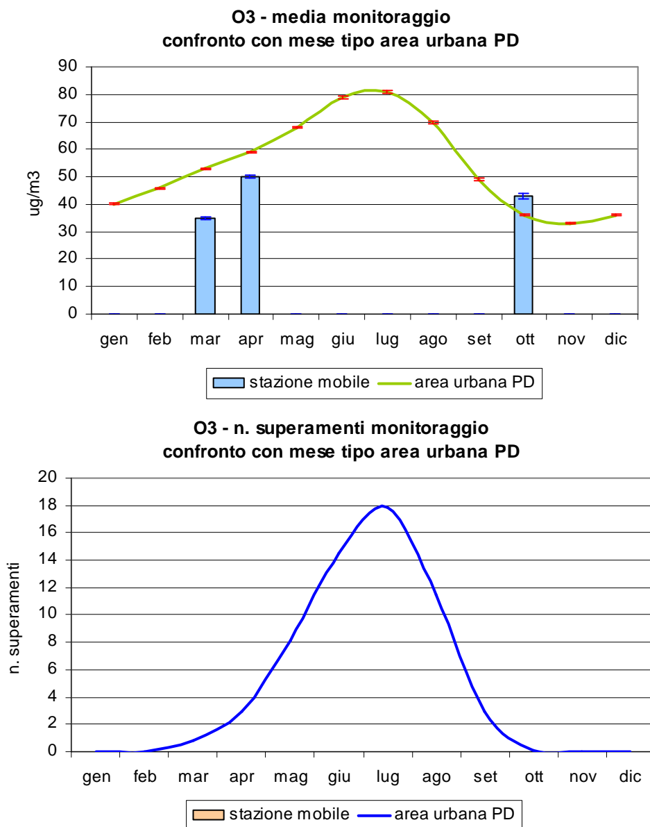
Figura 3.3 Ozono (O 3 ): confronto delle concentrazioni medie e del numero di superamenti del valore del limite di protezione della salute (120 µg/m 3 ) rilevati durante il monitoraggio in Piazzale Chiesa (Frazione Levada) nel Comune di Piombino Dese, con l'andamento caratteristico del 'mese tipo' ricavato dalla serie storica nell'area urbana di Padova (dai dati della serie storica della sola stazione fissa di Mandria); per i valori di concentrazione mensile le barre indicano l'errore standard della media.
