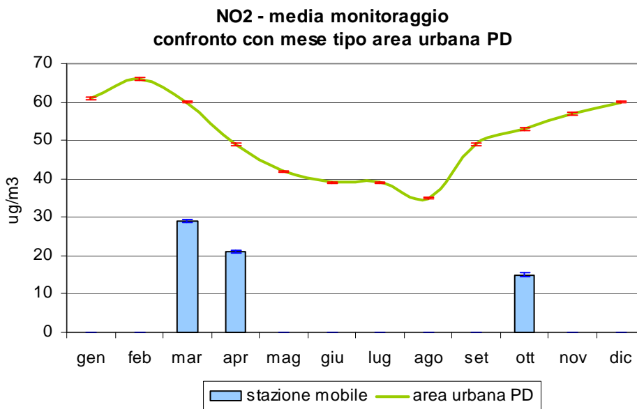
Figura 3.4 Biossido di azoto (NO 2 ): confronto delle concentrazioni medie rilevate durante il monitoraggio in Piazzale Chiesa (Frazione Levada) nel Comune di Piombino Dese, con l'andamento caratteristico del 'mese tipo' ricavato dalla serie storica nell'area urbana di Padova; le barre indicano l'errore standard della media.
