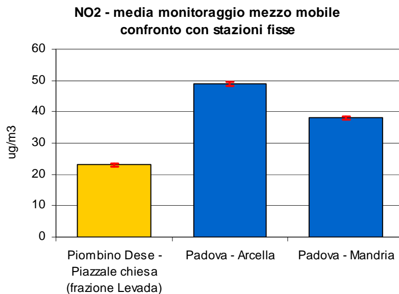
Figura 2.4 Biossido di azoto (NO 2 ): concentrazione media rilevata durante il monitoraggio in Piazzale Chiesa (Frazione Levada) nel Comune di Piombino Dese; le barre indicano l'errore standard della media.
