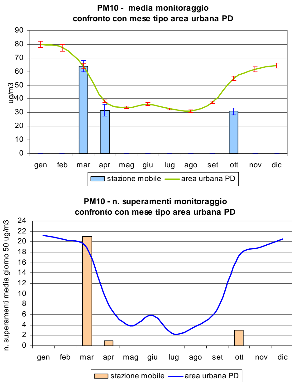
Figura 3.5 Polveri fini (PM 10 ): confronto delle concentrazioni medie e del numero di superamenti del valore limite di protezione della salute (50 µg/m 3 ) rilevati durante il monitoraggio in Piazzale Chiesa (Frazione Levada) nel Comune di Piombino Dese, con l'andamento caratteristico del 'mese tipo' ricavato dalla serie storica nell'area urbana di Padova; per i valori di concentrazione mensile le barre indicano l'errore standard della media.
