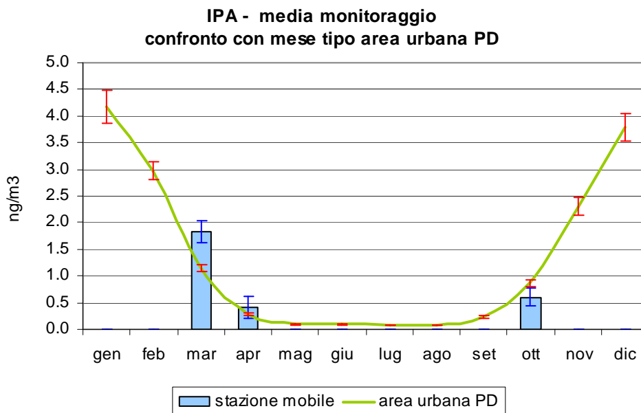
Figura 3.6 Benzo(a)pirene (IPA): confronto delle concentrazioni medie rilevate durante il monitoraggio in Piazzale Chiesa (Frazione Levada) nel Comune di Piombino Dese, con l'andamento caratteristico del 'mese tipo' ricavato dalla serie storica nell'area urbana di Padova; le barre indicano l'errore standard della media.
