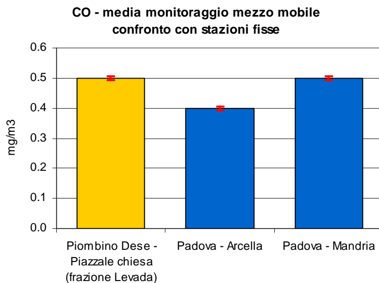
Figura 2.2 Monossido di carbonio (CO): concentrazione media rilevata durante il monitoraggio in Piazzale Chiesa (Frazione Levada) nel Comune di Piombino Dese; le barre indicano l'errore standard della media.
