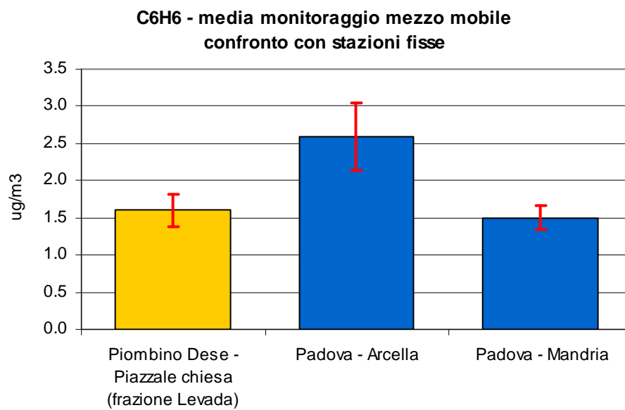
Figura 2.7 Benzene (C 6 H 6 ): concentrazione media rilevata durante il monitoraggio in Piazzale Chiesa (Frazione Levada) nel Comune di Piombino Dese; le barre indicano l'errore standard della media.
