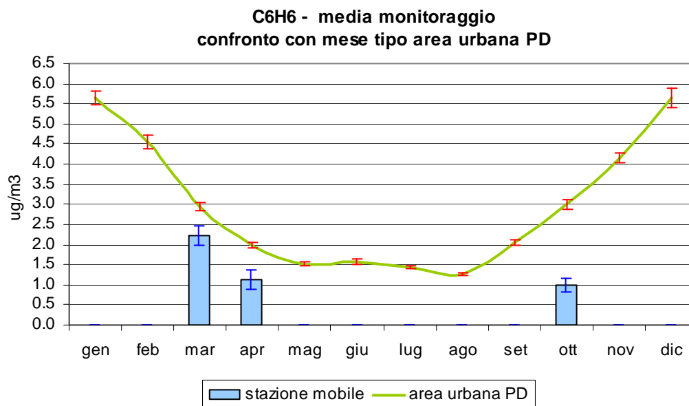
Figura 3.7 Benzene (C 6 H 6 ): confronto delle concentrazioni medie rilevate durante il monitoraggio in Piazzale Chiesa (Frazione Levada) nel Comune di Piombino Dese, con l'andamento caratteristico del 'mese tipo' ricavato dalla serie storica nell'area urbana di Padova; le barre indicano l'errore standard della media.
