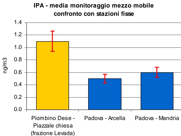
Figura 2.6 Benzo(a)pirene (IPA): concentrazione media rilevata durante il monitoraggio dal 24/02/10 al 20/04/10 e dal 24/09/10 al 19/10/10 in Piazzale Chiesa (Frazione Levada) nel Comune di Piombino Dese; le barre indicano l'errore standard della media.
