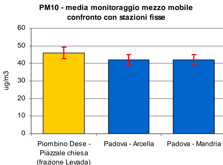
Figura 2.5 Polveri fini ( \text{PM}_{10} ): concentrazione media durante il monitoraggio dal 24/02/10 al 20/04/10 e dal 24/09/10 al 19/10/10 nel Comune di Piombino Dese; le barre indicano l'errore standard della media.
