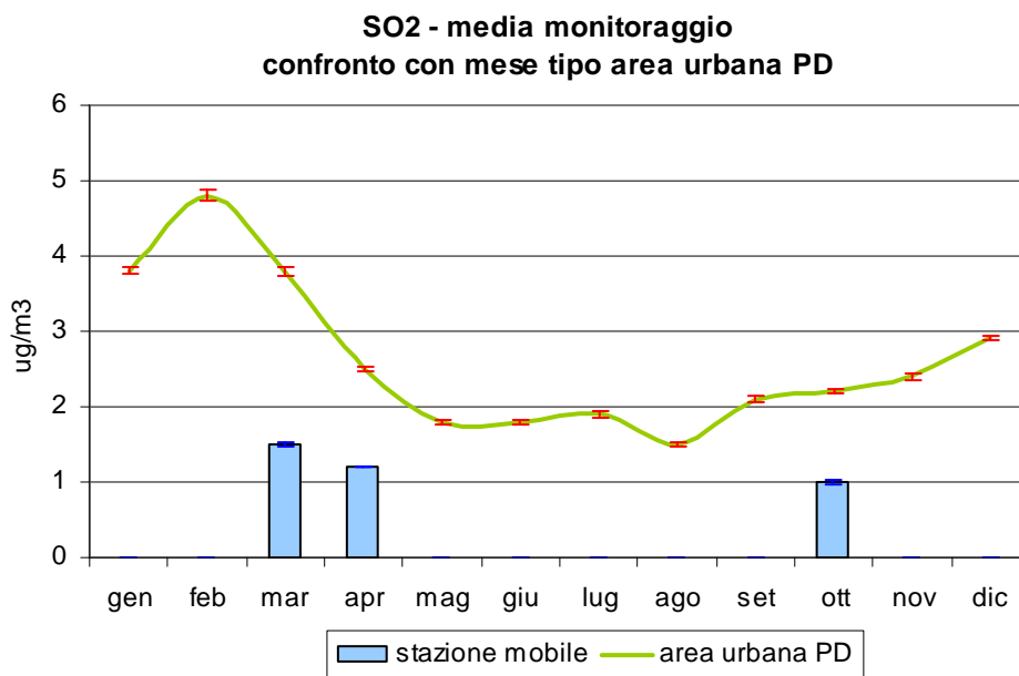
Figura 3.1 Biossido di zolfo (SO 2 ): confronto delle concentrazioni medie rilevate durante il monitoraggio in Piazzale Chiesa (Frazione Levada) nel Comune di Piombino Dese, con l'andamento caratteristico del 'mese tipo' ricavato dalla serie storica nell'area urbana di Padova; le barre indicano l'errore standard della media.
