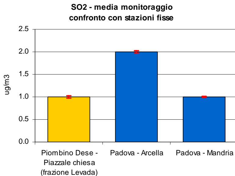
Figura 2.1 Biossido di zolfo (SO 2 ): concentrazione media rilevata durante il monitoraggio dal 24/02/10 al 20/04/10 e dal 24/09/10 al 19/10/10 in Piazzale Chiesa (Frazione Levada) nel Comune di Piombino Dese; le barre indicano l'errore standard della media.
