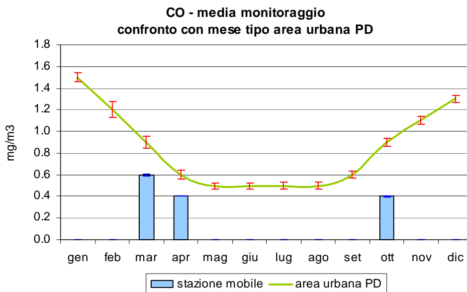
Figura 3.2 Monossido di carbonio (CO): confronto delle concentrazioni medie rilevate durante il monitoraggio in Piazzale Chiesa (Frazione Levada) nel Comune di Piombino Dese, con l'andamento caratteristico del 'mese tipo' ricavato dalla serie storica nell'area urbana di Padova; le barre indicano l'errore standard della media.
