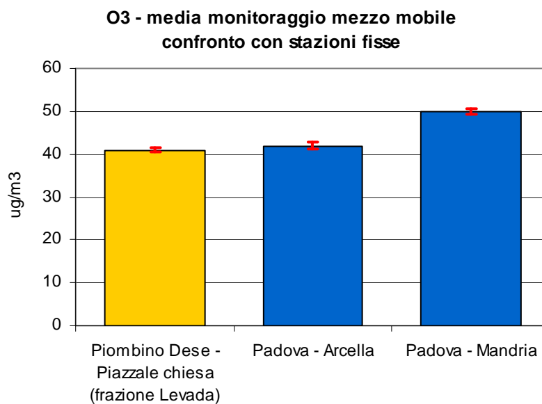
Figura 2.3 Ozono ( O_3 ): concentrazione media rilevata durante il monitoraggio in Piazzale Chiesa (Frazione Levada) nel Comune di Piombino Dese; le barre indicano l'errore standard della media.
