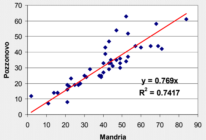
Correlazione Mandria - Pozzonovo
