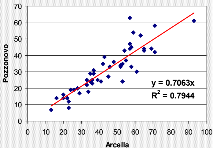
Correlazione Arcella - Pozzonovo
