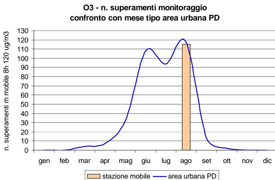
Figura 2.3 Ozono (O 3 ): concentrazione media e numero di superamenti rilevati durante il monitoraggio dal 30/06/05 al 03/08/05 e dal 23/11/05 al 14/12/05 in Via Favaro nel Comune di Pozzonovo; confronto con i periodi corrispondenti presso le stazioni fisse di Arcella e Mandria nel Comune di Padova e con l'andamento caratteristico del 'mese tipo' ricavato dalla serie storica nell'area urbana di Padova; per i valori di concentrazione mensile le barre indicano l'errore standard della media.
