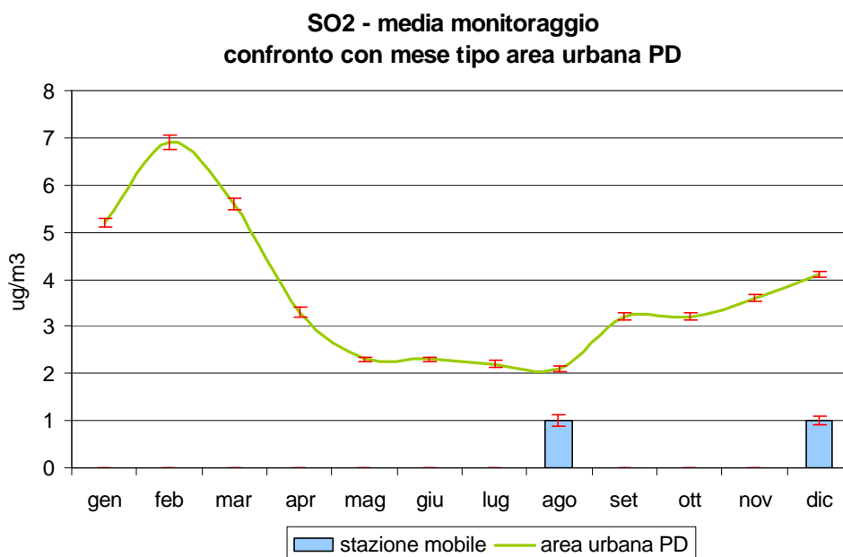
Figura 2.1 Biossido di zolfo (SO 2 ): concentrazione media rilevata durante il monitoraggio dal 30/06/05 al 03/08/05 e dal 23/11/05 al 14/12/05 in Via Favaro nel Comune di Pozzonovo; confronto con i periodi corrispondenti presso la stazioni fissa di Arcella e di Mandria nel Comune di Padova e con l'andamento caratteristico del 'mese tipo' ricavato dalla serie storica nell'area urbana di Padova; le barre indicano l'errore standard della media.
