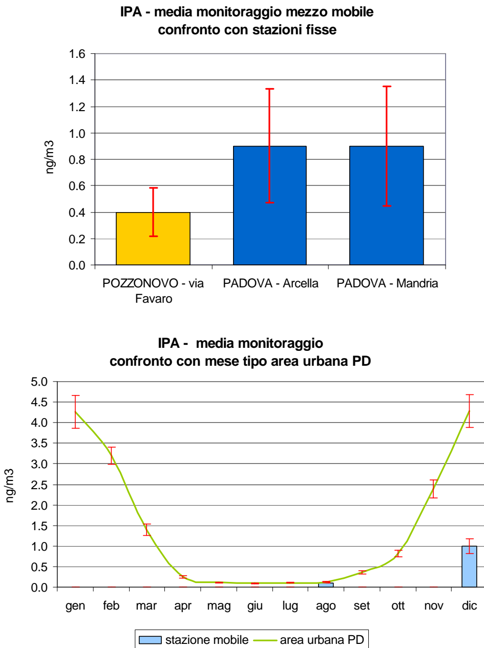
Figura 2.6 Benzo(a)pirene (IPA): concentrazione media rilevata durante il monitoraggio dal 30/06/05 al 03/08/05 e dal 23/11/05 al 14/12/05 in Via Favaro nel Comune di Pozzonovo; confronto con i periodi corrispondenti presso le stazioni fisse di Arcella e Mandria nel Comune di Padova e con l'andamento caratteristico del 'mese tipo' ricavato dalla serie storica nell'area urbana di Padova; le barre indicano l'errore standard della media.
