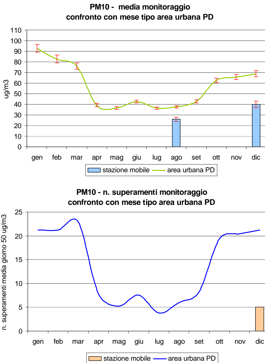
Figura 2.5 Polveri fini ( PM_{10} ): concentrazione media e numero di superamenti rilevati durante il monitoraggio dal 30/06/05 al 03/08/05 e dal 23/11/05 al 14/12/05 in Via Favaro nel Comune di Pozzonovo; confronto con i periodi corrispondenti presso le stazioni fisse di Arcella e Mandria nel Comune di Padova e con l'andamento caratteristico del 'mese tipo' ricavato dalla serie storica nell'area urbana di Padova; per i valori di concentrazione mensile le barre indicano l'errore standard della media.
