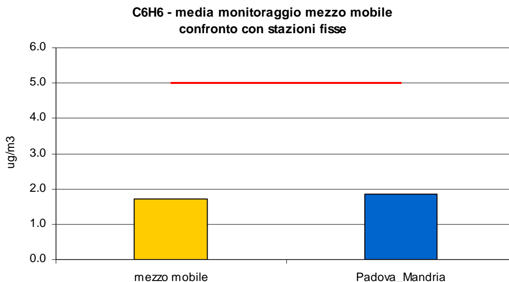
Figura 2.4 Benzene ( \text{C}_6\text{H}_6 ): concentrazione media rilevata durante il monitoraggio in via Rossi nel Comune di Rubano.
