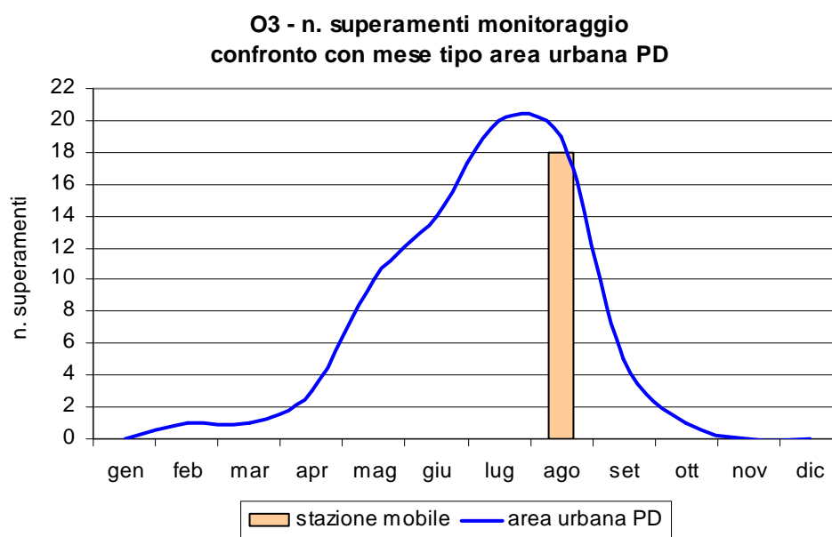
Figura 3.1 Ozono (O 3 ): confronto del numero di superamenti del valore del limite di protezione della salute (120 \mu\text{g}/\text{m}^3 ) rilevati durante il monitoraggio in via Rossi nel Comune di Rubano, con l'andamento caratteristico del 'mese tipo' ricavato dai dati della serie storica della stazione fissa di Mandria.
