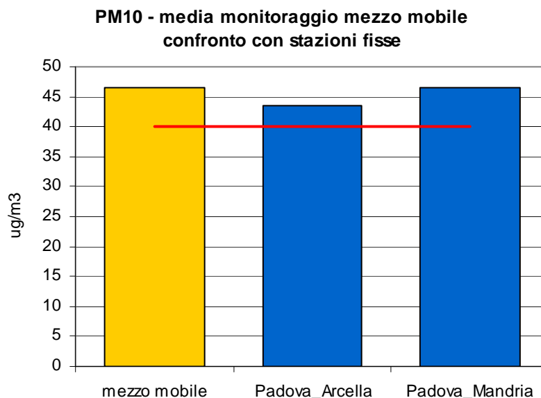
Figura 2.2 Polveri fini (PM 10 ): concentrazione media durante il monitoraggio dal 08/08/12 al 13/09/12 e dal 12/12/12 al 16/01/13 nel Comune di Rubano.
