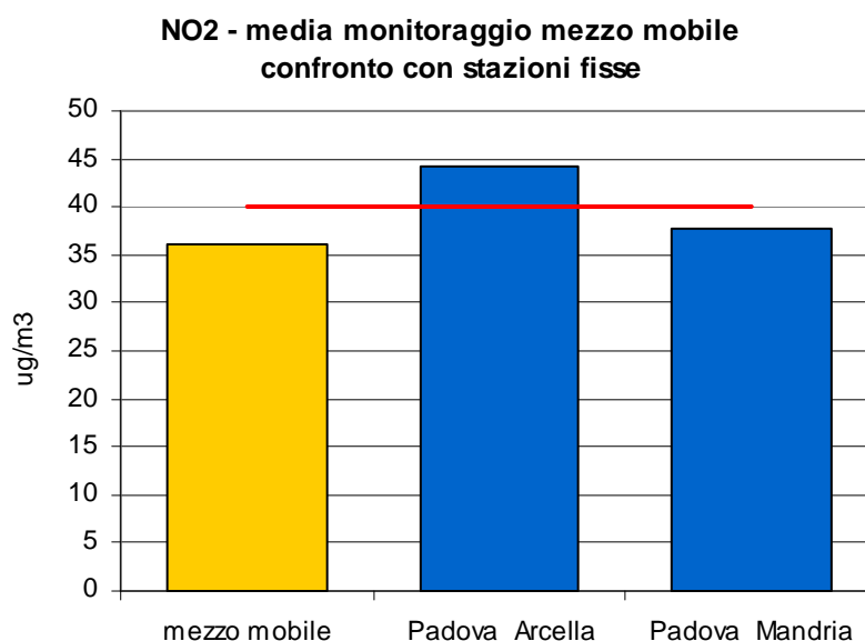
Figura 2.1 Biossido di azoto (NO 2 ): concentrazione media rilevata durante il monitoraggio in via Rossi nel Comune di Rubano.
