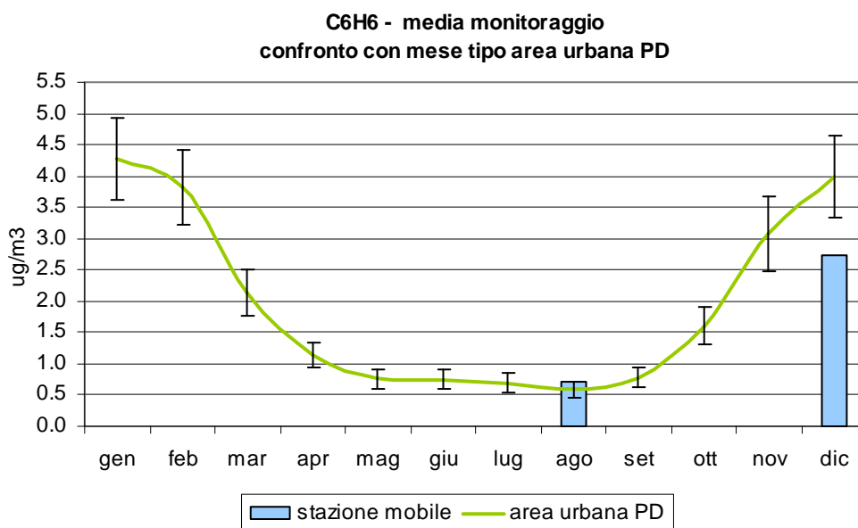
Figura 3.5 Benzene (C 6 H 6 ): confronto delle concentrazioni medie rilevate durante il monitoraggio in via Rossi nel Comune di Rubano, con l'andamento caratteristico del 'mese tipo' ricavato dalla serie storica nell'area urbana di Padova.
