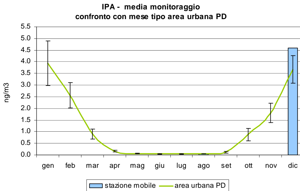
Figura 3.4 Benzo(a)pirene (IPA): confronto delle concentrazioni medie rilevate durante il monitoraggio in via Rossi nel Comune di Rubano, con l'andamento caratteristico del 'mese tipo' ricavato dalla serie storica nell'area urbana di Padova.
