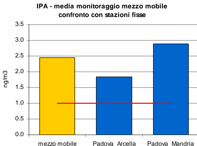
Figura 2.3 Benzo(a)pirene (IPA): concentrazione media rilevata durante il monitoraggio dal 08/08/12 al 13/09/12 e dal 12/12/12 al 16/01/13 in via Rossi nel Comune di Rubano.
