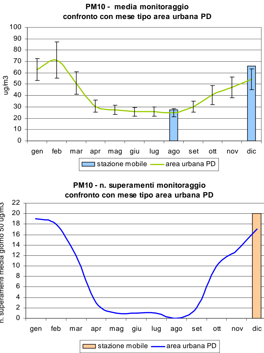
Figura 3.3 Polveri fini (PM 10 ): confronto delle concentrazioni medie e del numero di superamenti del valore limite di protezione della salute (50 µg/m 3 ) rilevati durante il monitoraggio in via Rossi nel Comune di Rubano, con l'andamento caratteristico del 'mese tipo' ricavato dalla serie storica nell'area urbana di Padova.
