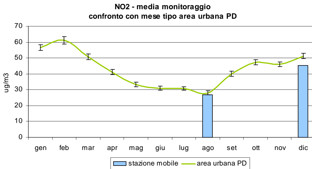
Figura 3.2 Biossido di azoto (NO 2 ): confronto delle concentrazioni medie rilevate durante il monitoraggio in via Rossi nel Comune di Rubano, con l'andamento caratteristico del 'mese tipo' ricavato dalla serie storica nell'area urbana di Padova.
