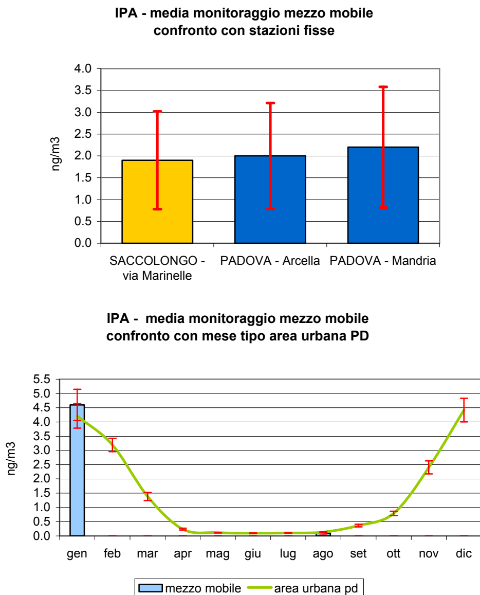
Figura 2.6 Benzo(a)pirene (IPA): concentrazione media rilevata durante il monitoraggio dal 22/07/04 al 11/08/04 e dal 05/01/05 al 27/01/05 in via Marinelle nel Comune di Saccolongo; confronto con i periodi corrispondenti presso le stazioni fisse di Arcella e Mandria nel Comune di Padova e con l'andamento caratteristico del 'mese tipo' ricavato dalla serie storica nell'area urbana di Padova; le barre indicano l'errore standard della media.
