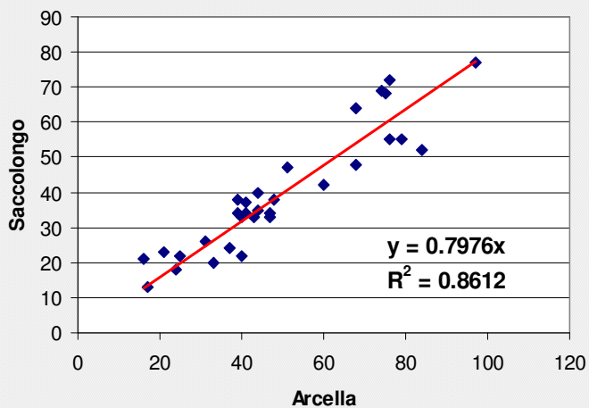
Correlazione Arcella - Saccolongo
