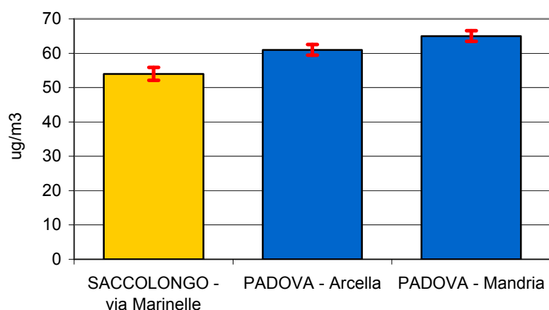
O3 - media monitoraggio mezzo mobile confronto con mese tipo area urbana PD
