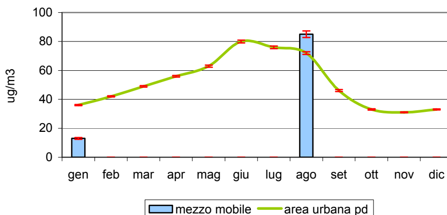
O3 - media monitoraggio mezzo mobile confronto con mese tipo area urbana PD
