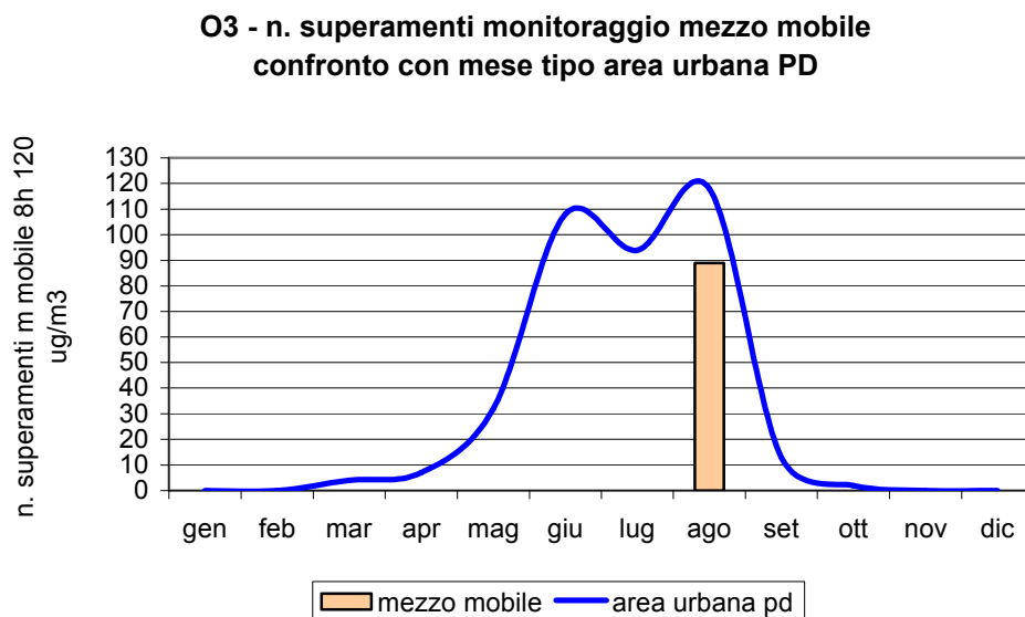
Figura 2.3 Ozono (O 3 ): concentrazione media e numero di superamenti rilevati durante il monitoraggio dal 22/07/04 al 11/08/04 e dal 05/01/05 al 27/01/05 in via Marinelle nel Comune di Saccolongo; confronto con i periodi corrispondenti presso le stazioni fisse di Arcella e Mandria nel Comune di Padova e con l'andamento caratteristico del 'mese tipo' ricavato dalla serie storica nell'area urbana di Padova; per i valori di concentrazione mensile le barre indicano l'errore standard della media.
