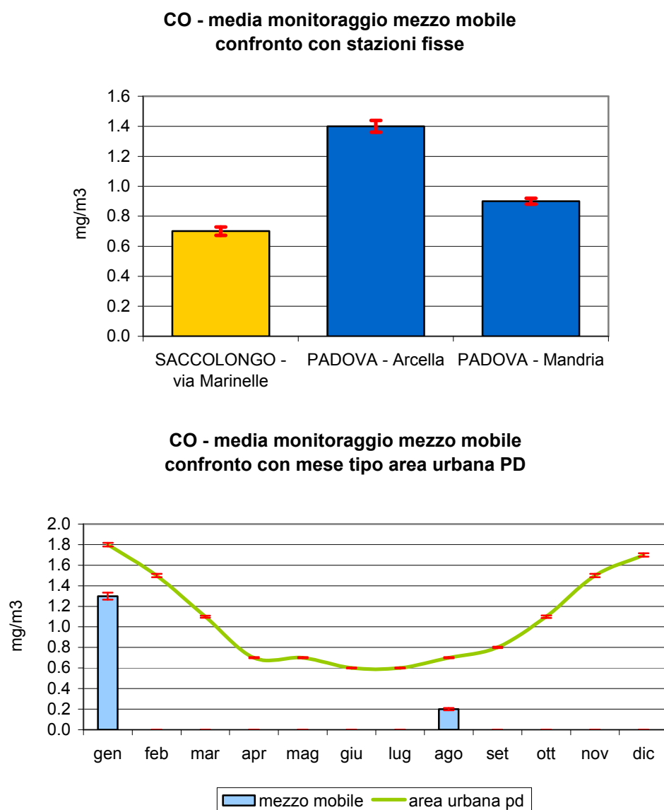
Figura 2.2 Monossido di carbonio (CO): concentrazione media rilevata durante il monitoraggio dal 22/07/04 al 11/08/04 e dal 05/01/05 al 27/01/05 in via Marinelle nel Comune di Saccolongo; confronto con i periodi corrispondenti presso le stazioni fisse di Arcella e Mandria nel Comune di Padova e con l'andamento caratteristico del 'mese tipo' ricavato dalla serie storica nell'area urbana di Padova; le barre indicano l'errore standard della media.
