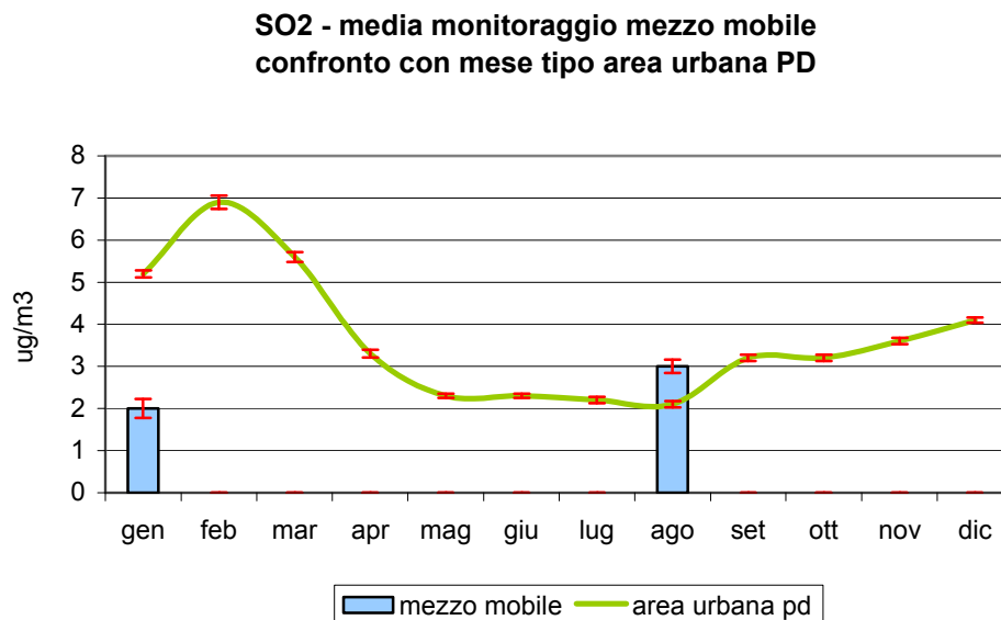
Figura 2.1 Biossido di zolfo (SO 2 ): concentrazione media rilevata durante il monitoraggio dal 22/07/04 al 11/08/04 e dal 05/01/05 al 27/01/05 in via Marinelle nel Comune di Saccolongo; confronto con i periodi corrispondenti presso la stazioni fissa di Arcella e di Mandria nel Comune di Padova e con l'andamento caratteristico del 'mese tipo' ricavato dalla serie storica nell'area urbana di Padova; le barre indicano l'errore standard della media.
