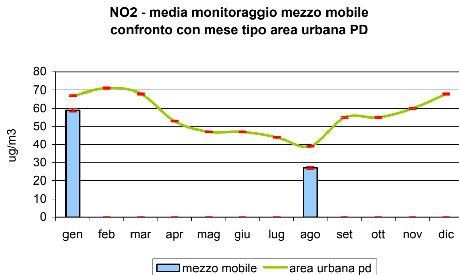
Figura 2.4 Biossido di azoto (NO 2 ): concentrazione media rilevata durante il monitoraggio dal 22/07/04 al 11/08/04 e dal 05/01/05 al 27/01/05 in via Marinelle nel Comune di Saccolongo; confronto con i periodi corrispondenti presso le stazioni fisse di Arcella e Mandria nel Comune di Padova e con l'andamento caratteristico del 'mese tipo' ricavato dalla serie storica nell'area urbana di Padova; le barre indicano l'errore standard della media.
