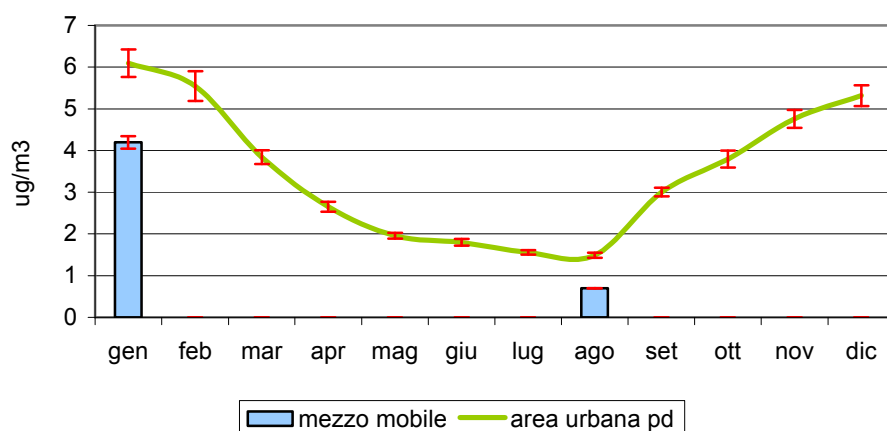
Figura 2.7 Benzene (C 6 H 6 ): concentrazione media rilevata durante il monitoraggio dal 22/07/04 al 11/08/04 e dal 05/01/05 al 27/01/05 in via Marinelle nel Comune di Saccolongo; confronto con i periodi corrispondenti presso le stazioni fisse di Arcella e Mandria nel Comune di Padova e con l'andamento caratteristico del 'mese tipo' ricavato dalla serie storica nell'area urbana di Padova; le barre indicano l'errore standard della media.
