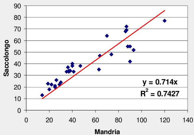
Correlazione Mandria - Saccolongo
