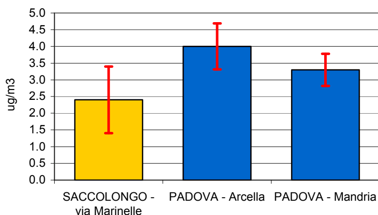
C6H6 - media monitoraggio mezzo mobile confronto con stazioni fisse
