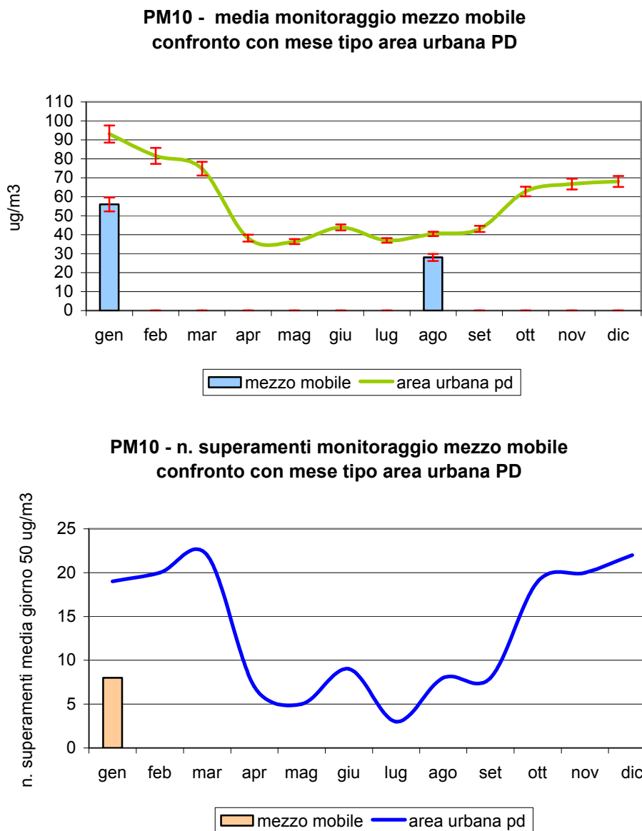
Figura 2.5 Polveri fini (PM 10 ): concentrazione media e numero di superamenti rilevati durante il monitoraggio dal 22/07/04 al 11/08/04 e dal 05/01/05 al 27/01/05 in via Marinelle nel Comune di Saccolongo; confronto con i periodi corrispondenti presso le stazioni fisse di Arcella e Mandria nel Comune di Padova e con l'andamento caratteristico del 'mese tipo' ricavato dalla serie storica nell'area urbana di Padova; per i valori di concentrazione mensile le barre indicano l'errore standard della media.
