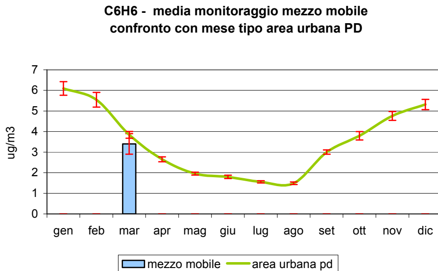
Figura 2.7 Benzene (C 6 H 6 ): concentrazione media rilevata durante il monitoraggio dal 23/02/05 al 16/03/05 in viale della Repubblica nel Comune di Selvazzano; confronto con il periodo corrispondente presso le stazioni fisse di Arcella e Mandria nel Comune di Padova e con l'andamento caratteristico del 'mese tipo' ricavato dalla serie storica; le barre indicano l'errore standard della media.
