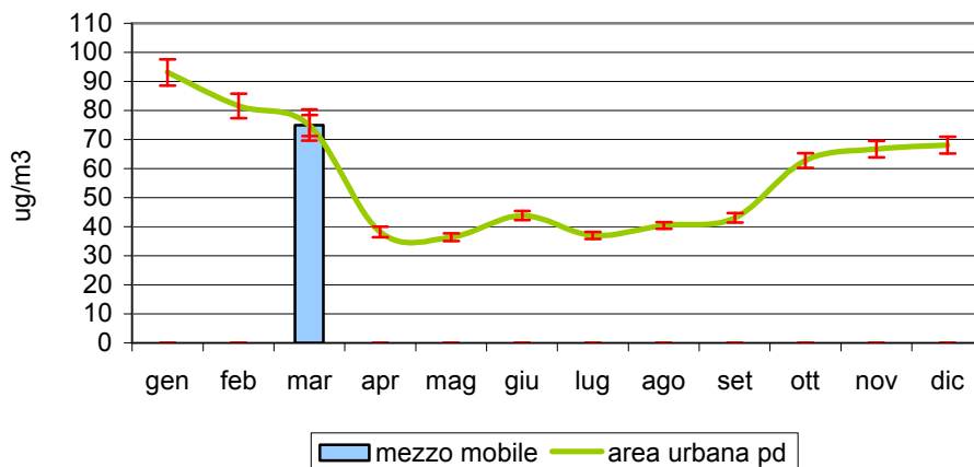
PM10 - media monitoraggio mezzo mobile confronto con mese tipo area urbana PD
