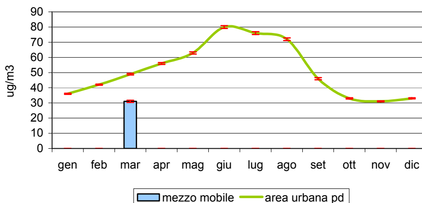
Figura 2.3 Ozono (O 3 ): concentrazione durante il monitoraggio dal 23/02/05 al 16/03/05 in viale della Repubblica nel Comune di Selvazzano; confronto con il periodo corrispondente presso le stazioni fisse di Arcella e Mandria nel Comune di Padova e con l'andamento caratteristico del 'mese tipo' ricavato dalla serie storica nell'area urbana di Padova; per i valori di concentrazione mensile le barre indicano l'errore standard della media.
