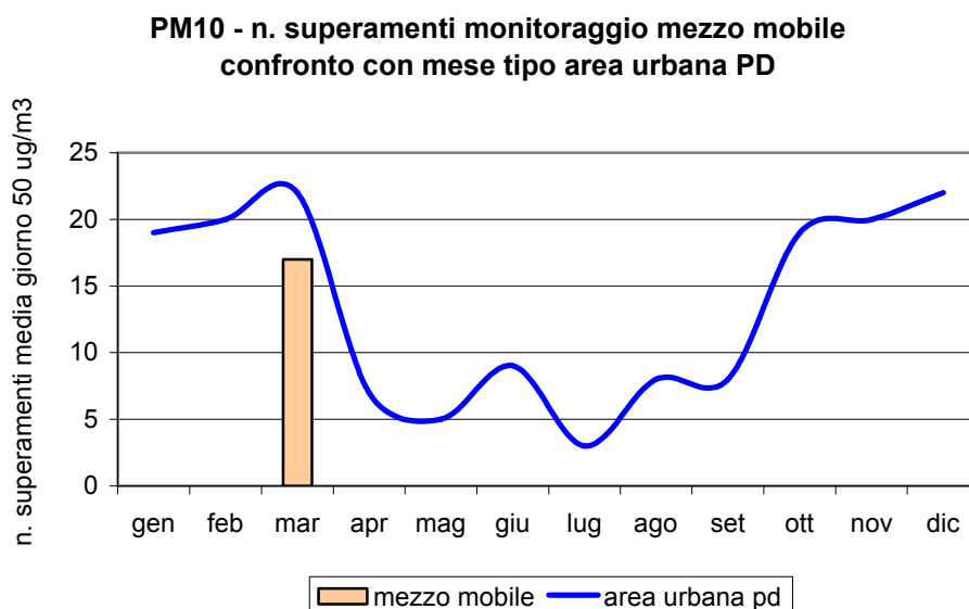
Figura 2.5 Polveri fini ( PM_{10} ): concentrazione media e numero di superamenti rilevati durante il monitoraggio dal 23/02/05 al 16/03/05 in viale della Repubblica nel Comune di Selvazzano; confronto con il periodo corrispondente presso le stazioni fisse di Arcella e Mandria nel Comune di Padova e con l'andamento caratteristico del 'mese tipo' ricavato dalla serie storica; per i valori di concentrazione mensile le barre indicano l'errore standard della media.
