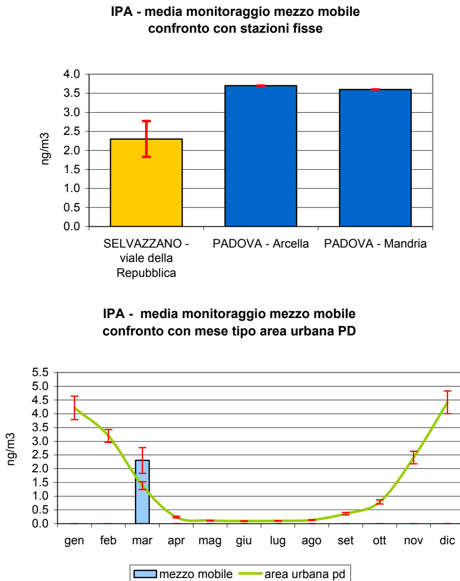
Figura 2.6 Benzo(a)pirene (IPA): concentrazione media rilevata durante il monitoraggio dal 23/02/05 al 16/03/05 in viale della Repubblica nel Comune di Selvazzano; confronto con il periodo corrispondente presso le stazioni fisse di Arcella e Mandria nel Comune di Padova e con l'andamento caratteristico del 'mese tipo' ricavato dalla serie storica; le barre indicano l'errore standard della media.
