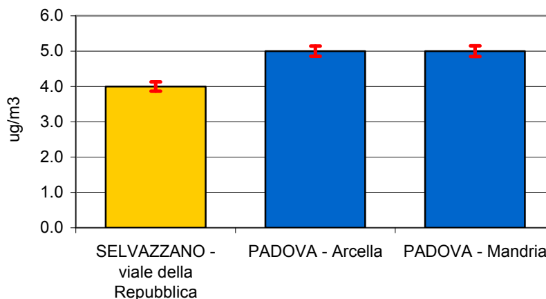
SO 2 - media monitoraggio mezzo mobile confronto con stazioni fisse
