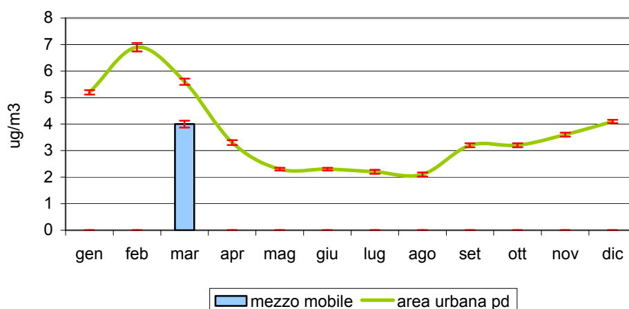
Figura 2.1 Biossido di zolfo (SO 2 ): concentrazione media rilevata durante il monitoraggio dal 23/02/05 al 16/03/05 in viale della Repubblica nel Comune di Selvazzano; confronto con il periodo corrispondente presso le stazioni fisse di Arcella e Mandria nel Comune di Padova e con l'andamento caratteristico del 'mese tipo' ricavato dalla serie storica nell'area urbana di Padova; le barre indicano l'errore standard della media.
