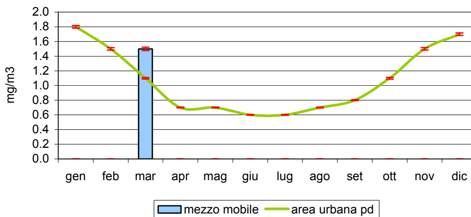
Figura 2.2 Monossido di carbonio (CO): concentrazione media rilevata durante il monitoraggio dal 23/02/05 al 16/03/05 in viale della Repubblica nel Comune di Selvazzano; confronto con il periodo corrispondente presso le stazioni fisse di Arcella e Mandria nel Comune di Padova e con l'andamento caratteristico del 'mese tipo' ricavato dalla serie storica nell'area urbana di Padova; le barre indicano l'errore standard della media.
