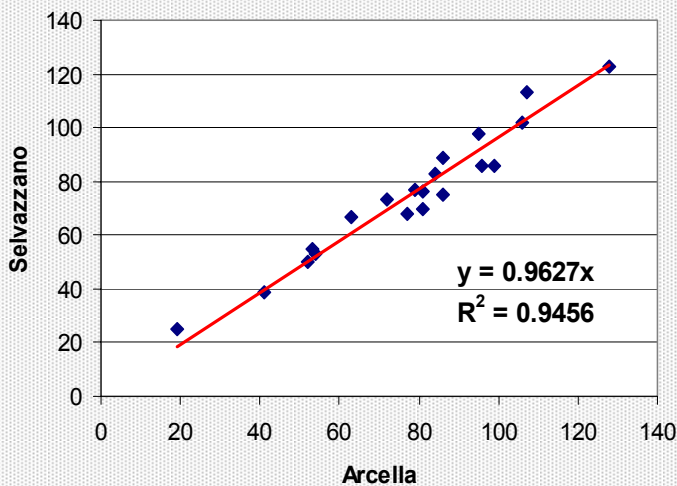
Correlazione Arcella - Selvazzano
