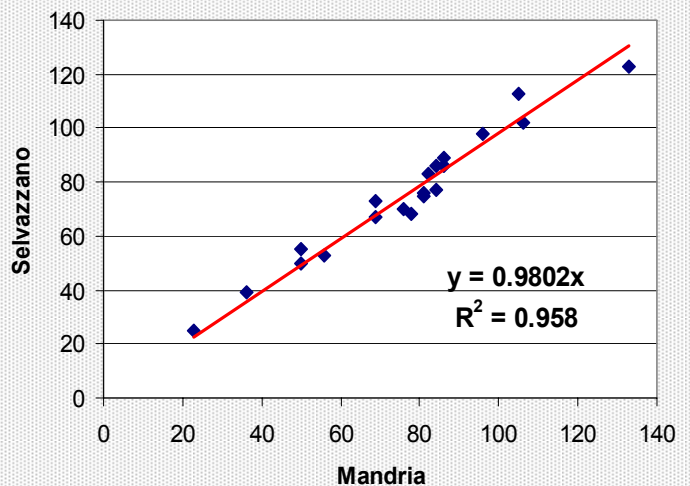
Correlazione Mandria - Selvazzano
