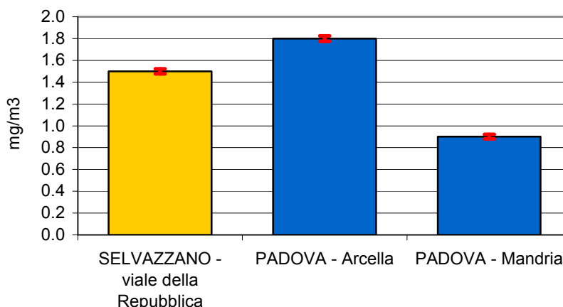
CO - media monitoraggio mezzo mobile confronto con mese tipo area urbana PD
