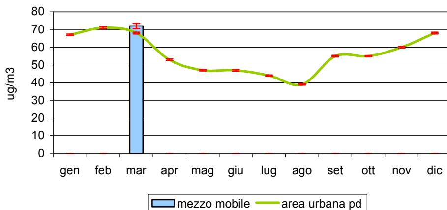
Figura 2.4 Biossido di azoto ( \text{NO}_2 ): concentrazione media rilevata durante il monitoraggio dal 23/02/05 al 16/03/05 in viale della Repubblica nel Comune di Selvazzano; confronto con il periodo corrispondente presso le stazioni fisse di Arcella e Mandria nel Comune di Padova e con l'andamento caratteristico del 'mese tipo' ricavato dalla serie storica nell'area urbana di Padova; le barre indicano l'errore standard della media.
