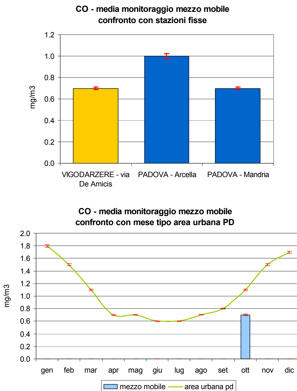
Figura 2.2 Monossido di carbonio (CO): concentrazione media rilevata durante il monitoraggio dal 28/09/04 al 20/10/04 in Via De Amicis nel Comune di Vigodarzere; confronto con il periodo corrispondente presso le stazioni fisse di Arcella e Mandria nel Comune di Padova e con l'andamento caratteristico del 'mese tipo' ricavato dalla serie storica nell'area urbana di Padova; le barre indicano l'errore standard della media.
