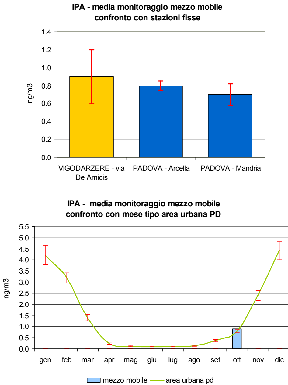
Figura 2.6 Benzo(a)pirene (IPA): concentrazione media rilevata durante il monitoraggio dal 28/09/04 al 20/10/04 in Via De Amicis nel Comune di Vigodarzere; confronto con il periodo corrispondente presso le stazioni fisse di Arcella e Mandria nel Comune di Padova e con l'andamento caratteristico del 'mese tipo' ricavato dalla serie storica; le barre indicano l'errore standard della media.
