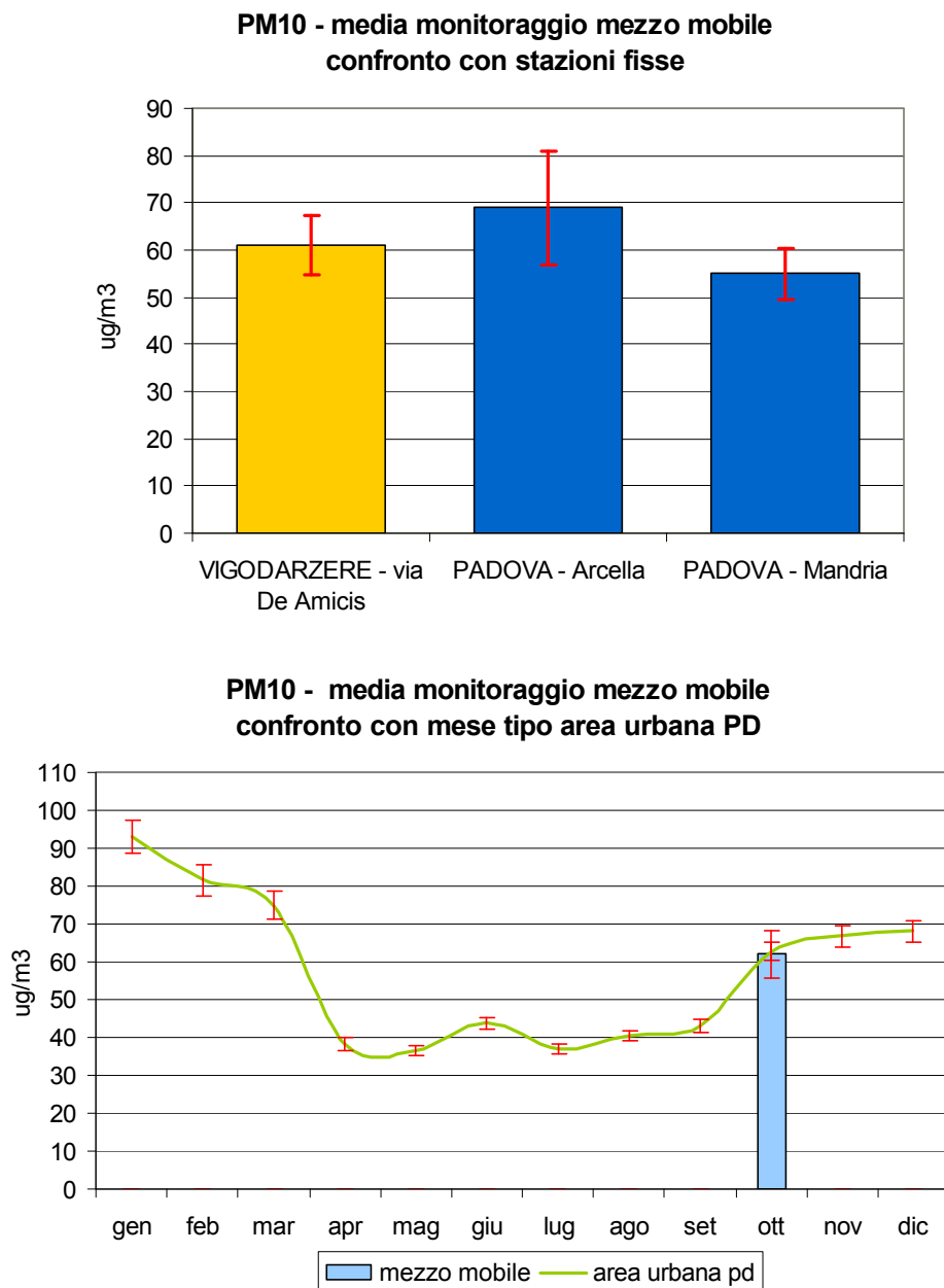
Figura 2.5 Polveri fini (PM 10 ): concentrazione media rilevata durante il monitoraggio dal 28/09/04 al 20/10/04 in Via De Amicis nel Comune di Vigodarzere; confronto con il periodo corrispondente presso le stazioni fisse di Arcella e Mandria nel Comune di Padova e con l'andamento caratteristico del 'mese tipo' ricavato dalla serie storica; le barre indicano l'errore standard della media.
