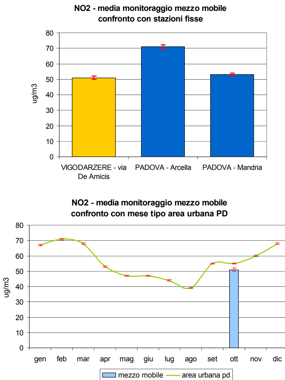
Figura 2.4 Biossido di azoto ( \text{NO}_2 ): concentrazione media rilevata durante il monitoraggio dal 28/09/04 al 20/10/04 in Via De Amicis nel Comune di Vigodarzere; confronto con il periodo corrispondente presso le stazioni fisse di Arcella e Mandria nel Comune di Padova e con l'andamento caratteristico del 'mese tipo' ricavato dalla serie storica nell'area urbana di Padova; le barre indicano l'errore standard della media.
