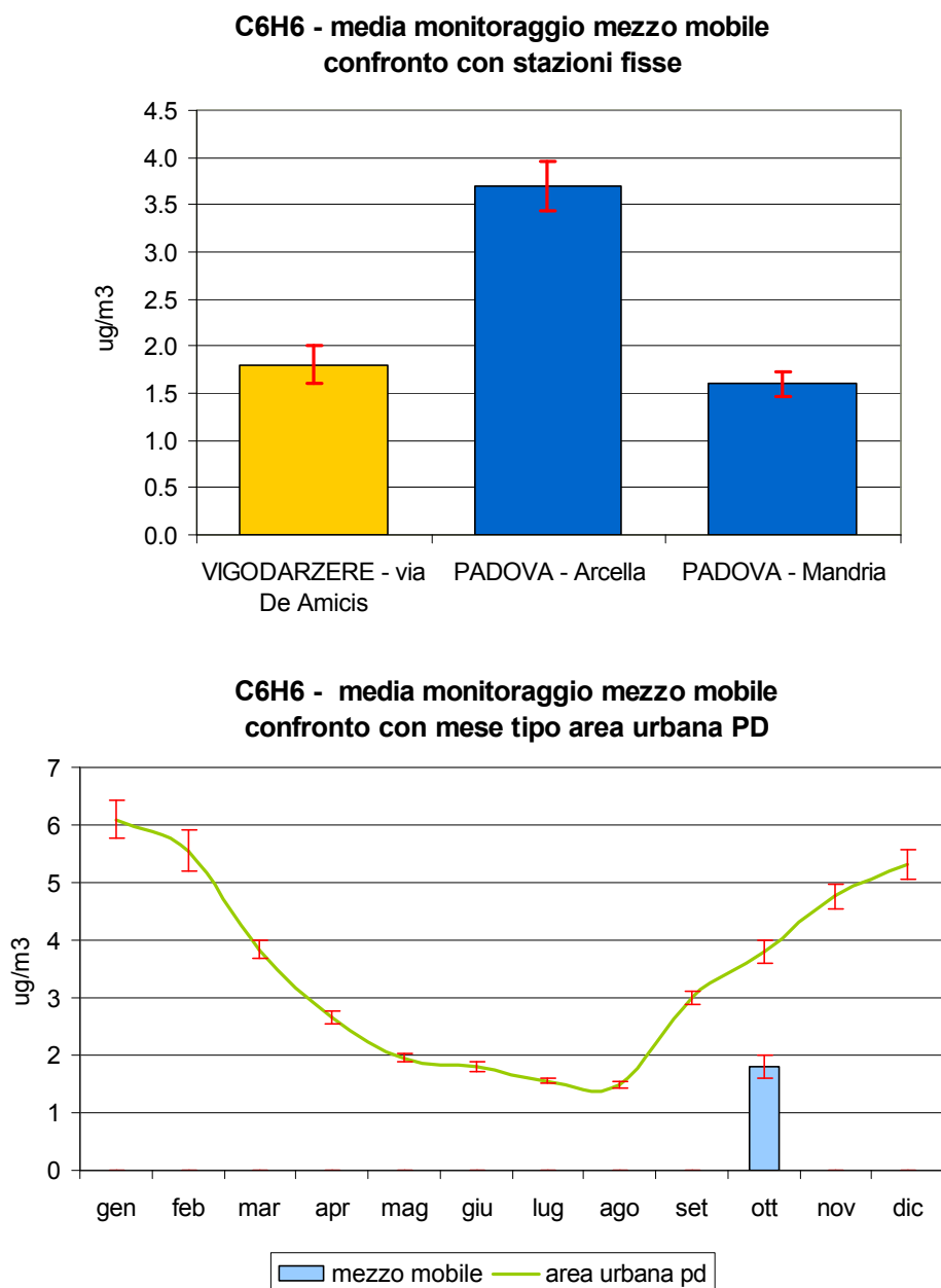
Figura 2.7 Benzene ( C_6H_6 ): concentrazione media rilevata durante il monitoraggio dal 28/09/04 al 20/10/04 in Via De Amicis nel Comune di Vigodarzere; confronto con il periodo corrispondente presso le stazioni fisse di Arcella e Mandria nel Comune di Padova e con l'andamento caratteristico del 'mese tipo' ricavato dalla serie storica; le barre indicano l'errore standard della media.
