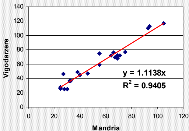
Correlazione Mandria - Vigodarzere
