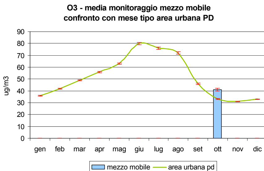
Figura 2.3 Ozono (O 3 ): concentrazione media rilevata durante il monitoraggio dal 28/09/04 al 20/10/04 in Via De Amicis nel Comune di Vigodarzere; confronto con il periodo corrispondente presso le stazioni fisse di Arcella e Mandria nel Comune di Padova e con l'andamento caratteristico del 'mese tipo' ricavato dalla serie storica nell'area urbana di Padova; le barre indicano l'errore standard della media.
