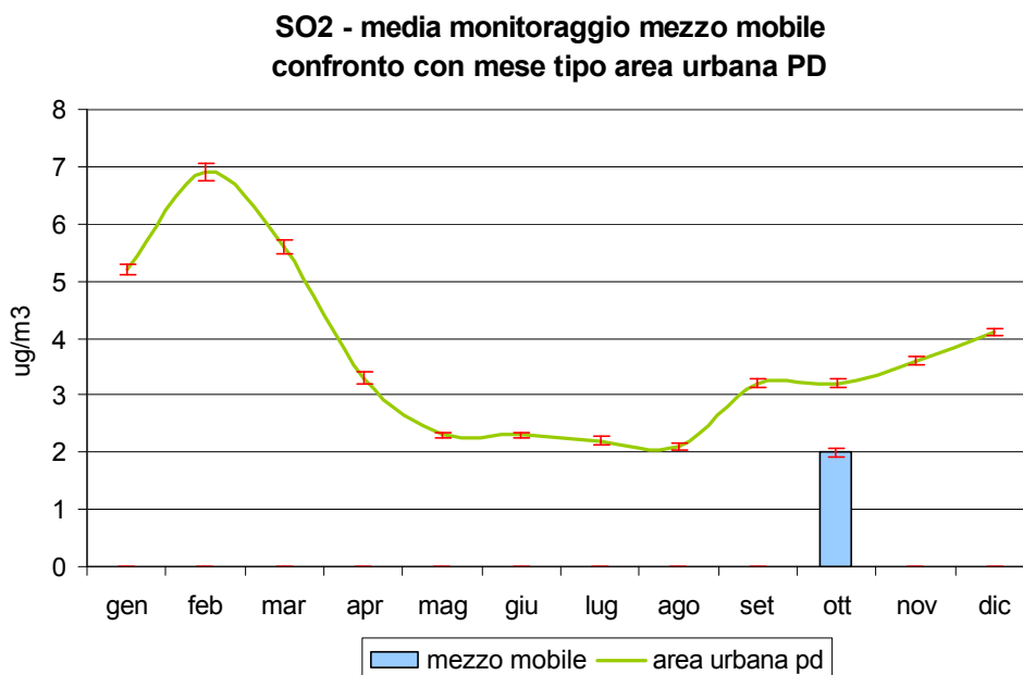
Figura 2.1 Biossido di zolfo (SO 2 ): concentrazione media rilevata durante il monitoraggio dal 28/09/04 al 20/10/04 in Via De Amicis nel Comune di Vigodarzere; confronto con il periodo corrispondente presso la stazione fissa di Mandria nel Comune di Padova e con l'andamento caratteristico del 'mese tipo' ricavato dalla serie storica nell'area urbana di Padova; le barre indicano l'errore standard della media.
