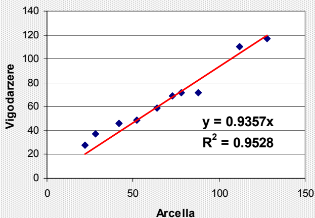
Correlazione Arcella - Vigodarzere
