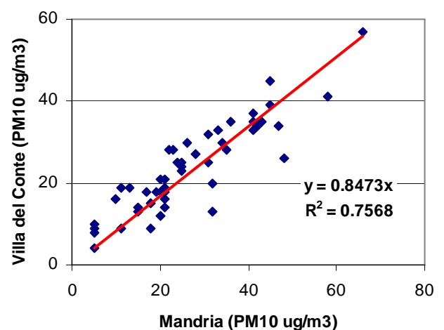
Correlazione Mandria - Villa del Conte
