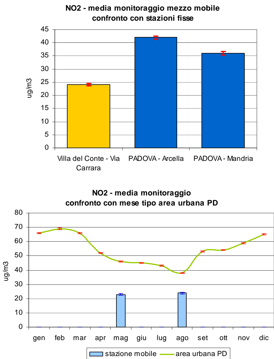
Figura 2.4 Biossido di azoto (NO 2 ): concentrazione media rilevata durante il monitoraggio dal 03/08/06 al 30/08/06 e dal 25/04/07 al 22/05/07 in Via Don Carrari nel Comune di Villa del Conte; confronto con i periodi corrispondenti presso le stazioni fisse di Arcella e Mandria nel Comune di Padova e con l'andamento caratteristico del 'mese tipo' ricavato dalla serie storica nell'area urbana di Padova; le barre indicano l'errore standard della media.
