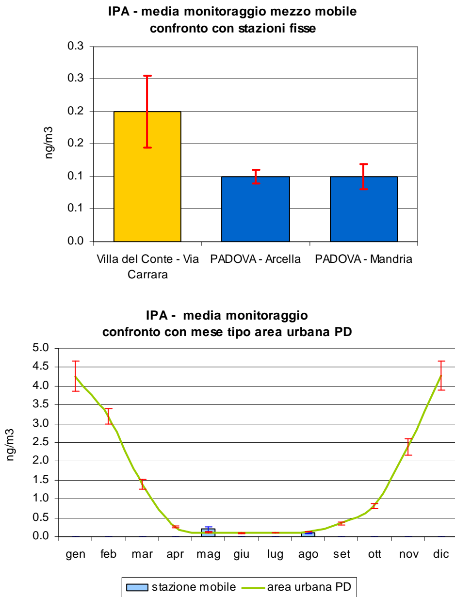
Figura 2.6 Benzo(a)pirene (IPA): concentrazione media rilevata durante il monitoraggio dal 03/08/06 al 30/08/06 e dal 25/04/07 al 22/05/07 in Via Don Carrari nel Comune di Villa del Conte; confronto con i periodi corrispondenti presso le stazioni fisse di Arcella e Mandria nel Comune di Padova e con l'andamento caratteristico del 'mese tipo' ricavato dalla serie storica nell'area urbana di Padova; le barre indicano l'errore standard della media.
