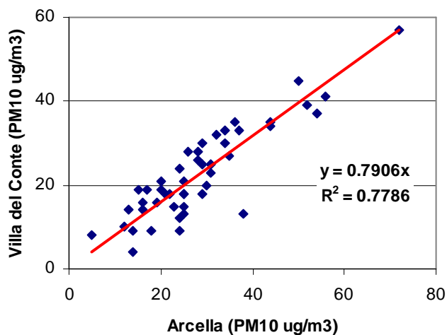
Correlazione Arcella - Villa del Conte
