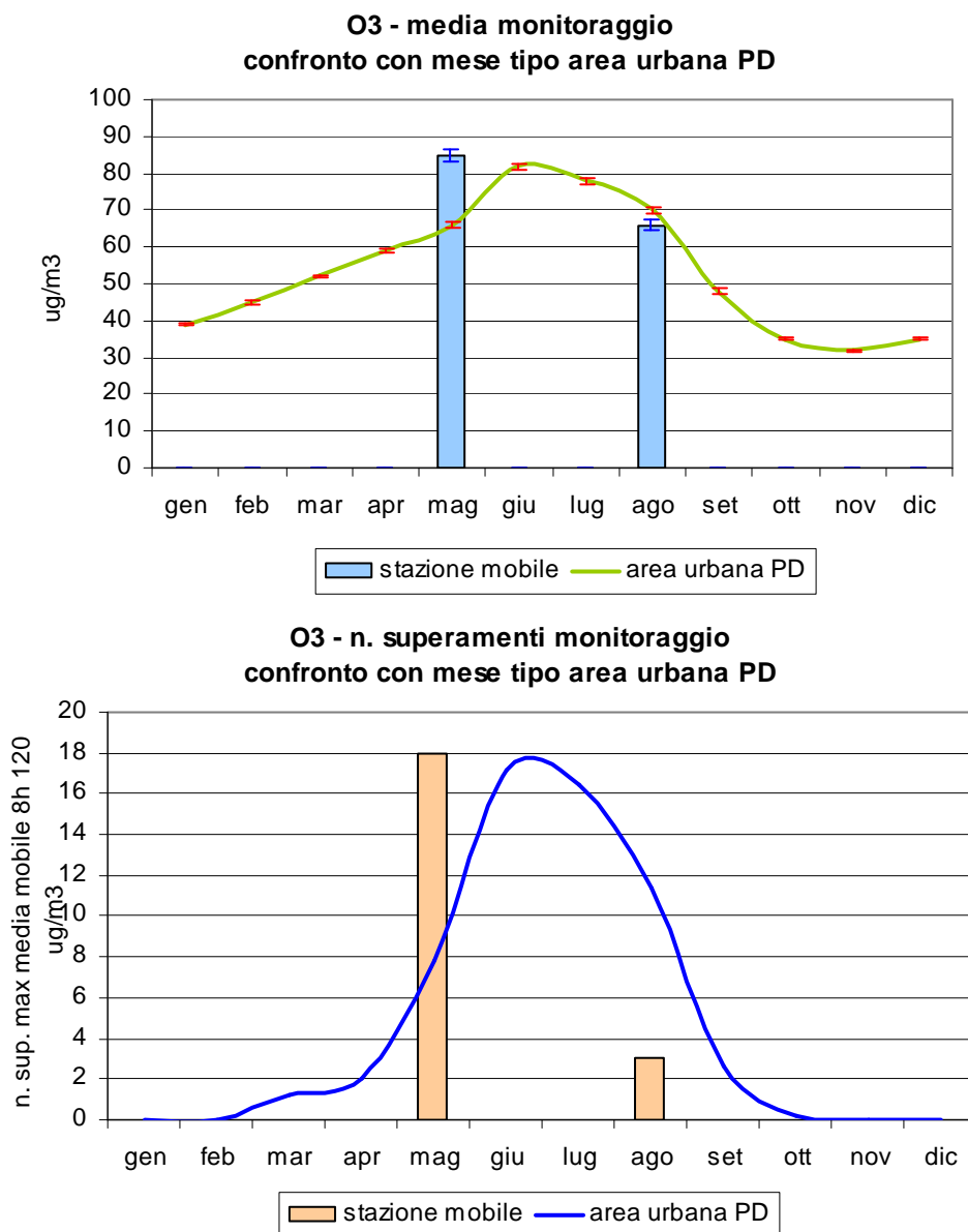
Figura 2.3 Ozono (O 3 ): concentrazione media e numero di superamenti rilevati durante il monitoraggio dal 03/08/06 al 30/08/06 e dal 25/04/07 al 22/05/07 in Via Don Carrari nel Comune di Villa del Conte; confronto con i periodi corrispondenti presso le stazioni fisse di Arcella e Mandria nel Comune di Padova e con l'andamento caratteristico del 'mese tipo' ricavato dalla serie storica nell'area urbana di Padova; per i valori di concentrazione mensile le barre indicano l'errore standard della media.
