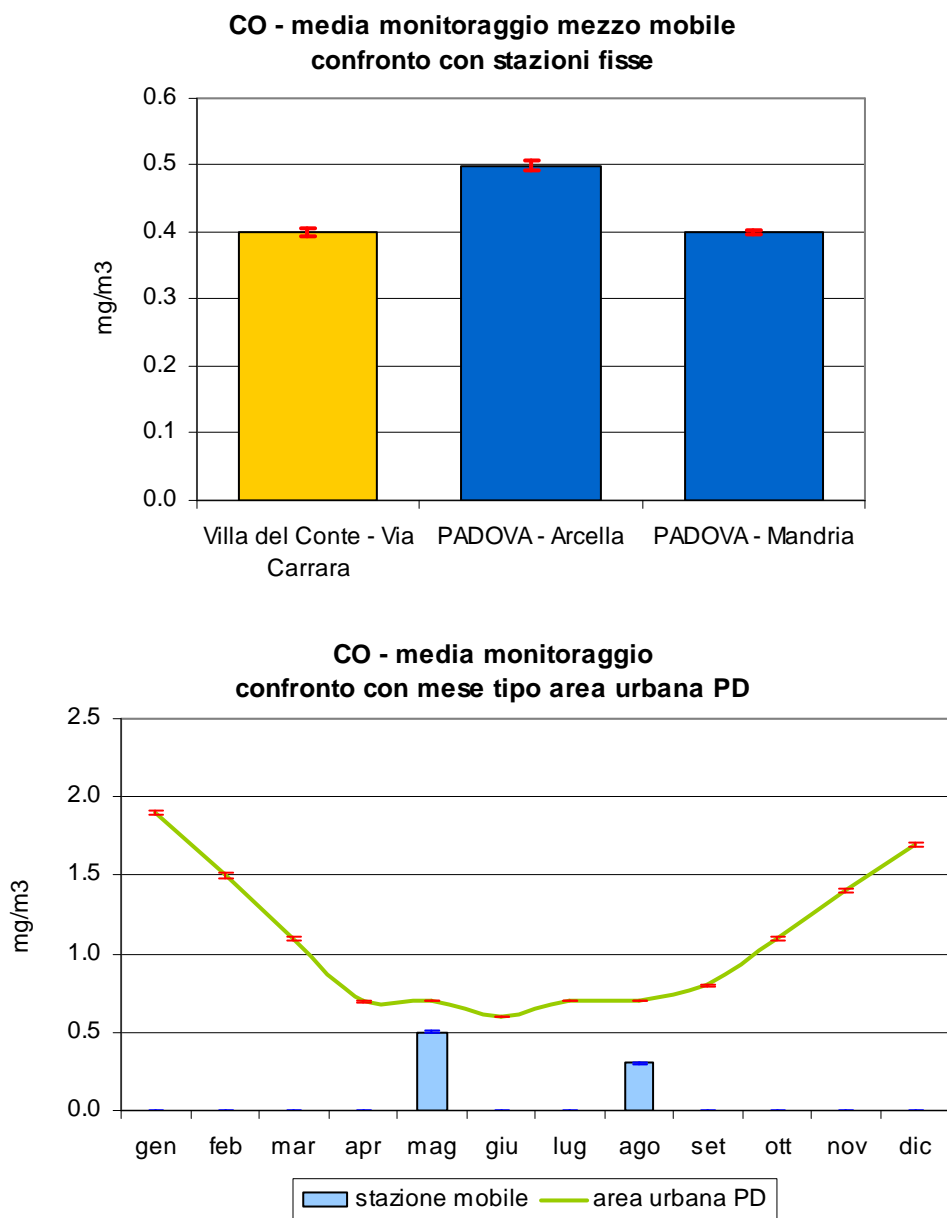
Figura 2.2 Monossido di carbonio (CO): concentrazione media rilevata durante il monitoraggio dal 03/08/06 al 30/08/06 e dal 25/04/07 al 22/05/07 in Via Don Carrari nel Comune di Villa del Conte; confronto con i periodi corrispondenti presso le stazioni fisse di Arcella e Mandria nel Comune di Padova e con l'andamento caratteristico del 'mese tipo' ricavato dalla serie storica nell'area urbana di Padova; le barre indicano l'errore standard della media.
