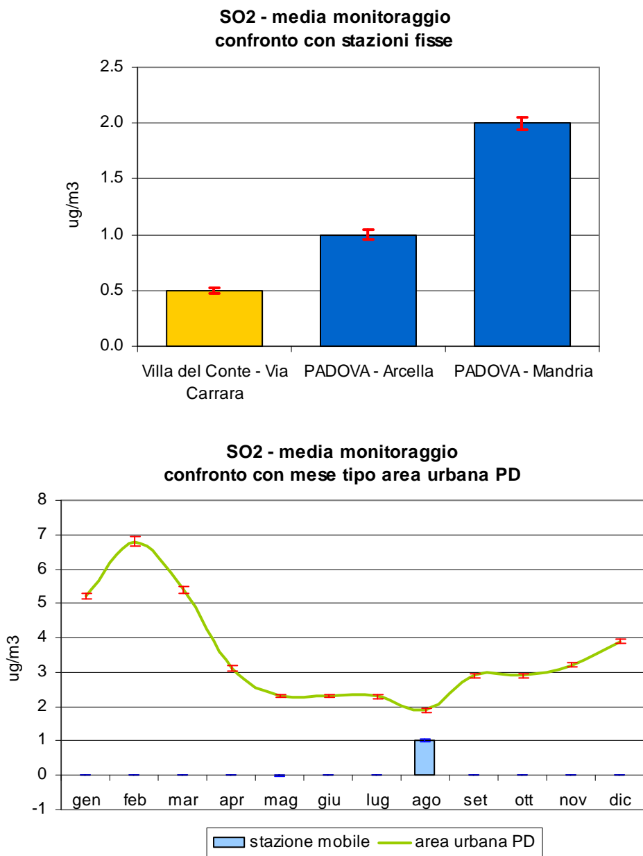
Figura 2.1 Biossido di zolfo (SO 2 ): concentrazione media rilevata durante il monitoraggio dal 03/08/06 al 30/08/06 e dal 25/04/07 al 22/05/07 in Via Don Carrari nel Comune di Villa del Conte; confronto con i periodi corrispondenti presso la stazioni fissa di Arcella e di Mandria nel Comune di Padova e con l'andamento caratteristico del 'mese tipo' ricavato dalla serie storica nell'area urbana di Padova; le barre indicano l'errore standard della media.
