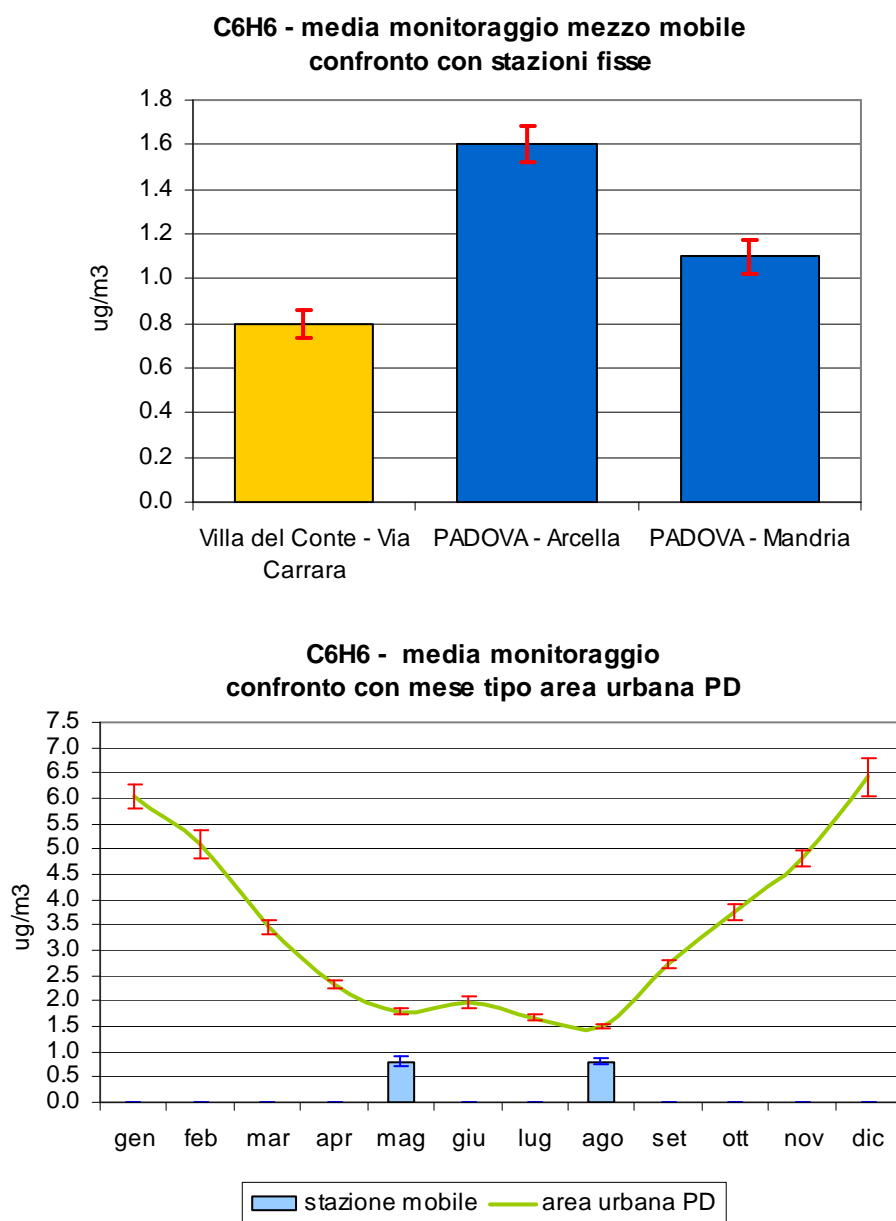
Figura 2.7 Benzene (C 6 H 6 ): concentrazione media rilevata durante il monitoraggio dal 03/08/06 al 30/08/06 e dal 25/04/07 al 22/05/07 in Via Don Carrari nel Comune di Villa del Conte; confronto con i periodi corrispondenti presso le stazioni fisse di Arcella e Mandria nel Comune di Padova e con l'andamento caratteristico del 'mese tipo' ricavato dalla serie storica nell'area urbana di Padova; le barre indicano l'errore standard della media.
