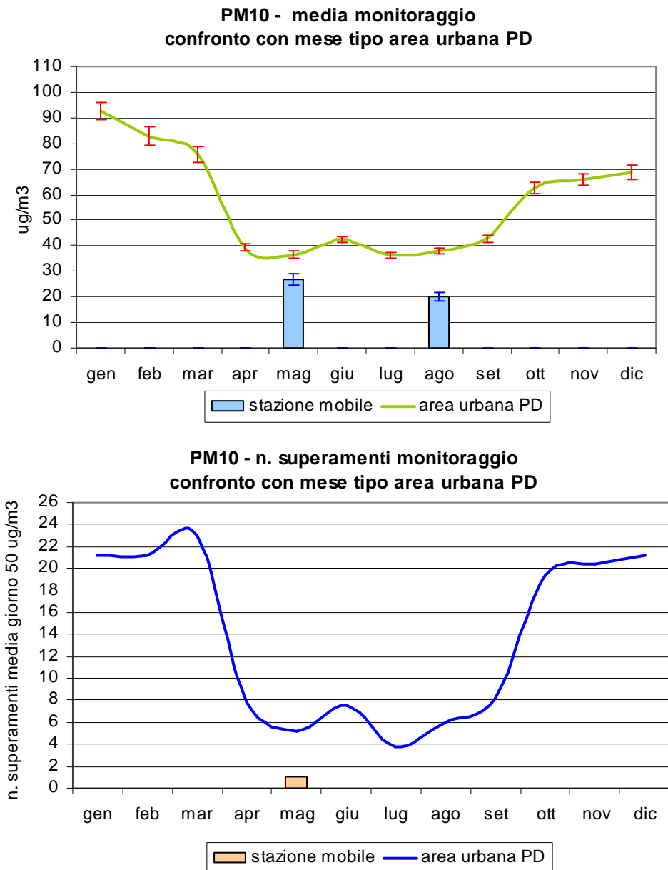
Figura 2.5 Polveri fini ( PM_{10} ): concentrazione media e numero di superamenti rilevati durante il monitoraggio dal 03/08/06 al 30/08/06 e dal 25/04/07 al 22/05/07 in Via Don Carrari nel Comune di Villa del Conte; confronto con i periodi corrispondenti presso le stazioni fisse di Arcella e Mandria nel Comune di Padova e con l'andamento caratteristico del 'mese tipo' ricavato dalla serie storica nell'area urbana di Padova; per i valori di concentrazione mensile le barre indicano l'errore standard della media.
