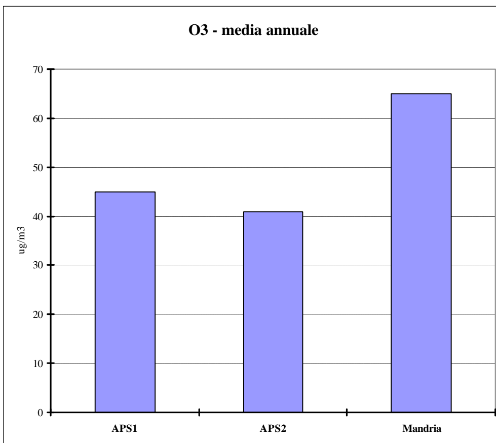
Figura 3.2 Ozono (O 3 ). Concentrazione media rilevata nel 2012.
