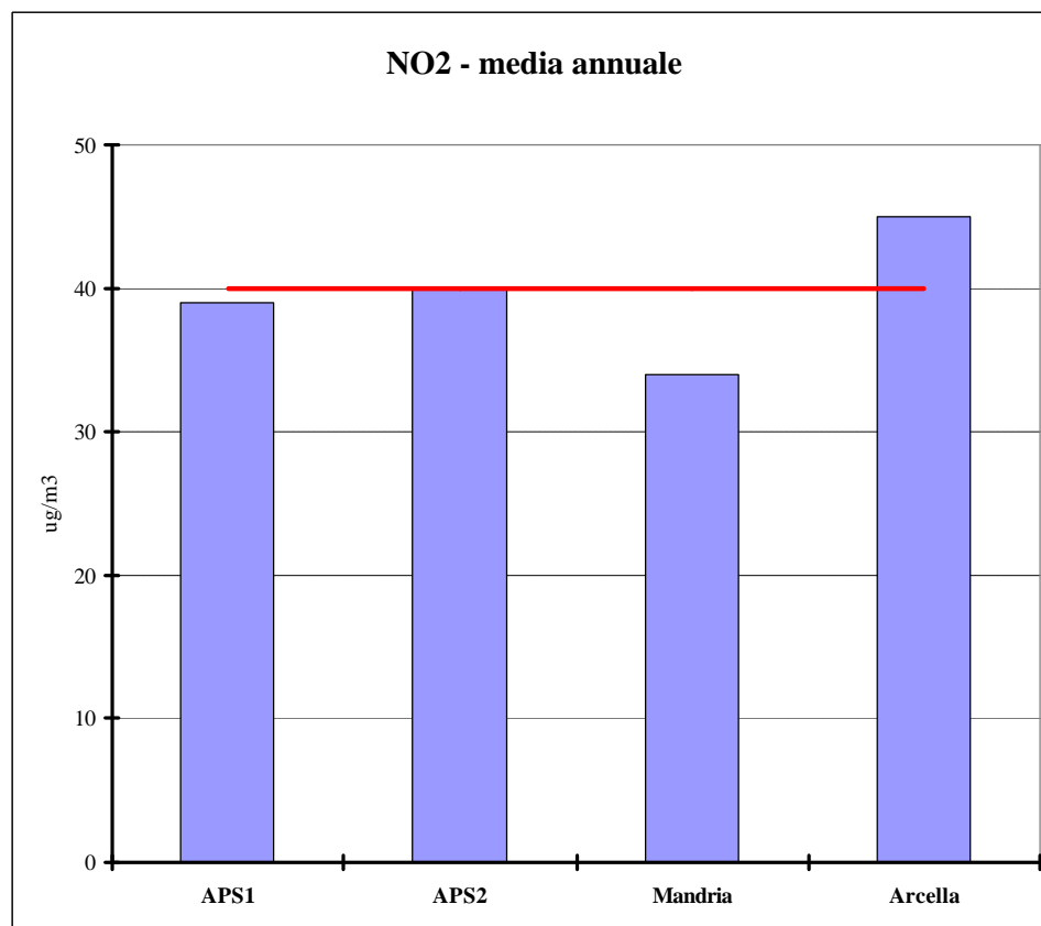
Figura 3.1 Biossido di azoto (NO 2 ). Confronto tra la concentrazione media rilevata nel 2012 e il limite annuale per la protezione della salute umana (40 µg/m 3 ).
