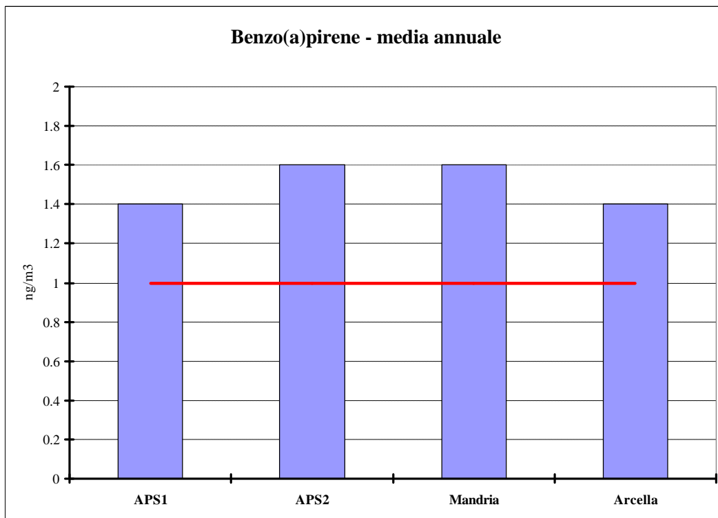
Figura 3.7 Benzo(a)pirene. Confronto tra la concentrazione media rilevata nel 2012 e il valore obiettivo (1 \text{ng}/\text{m}^3 ).
