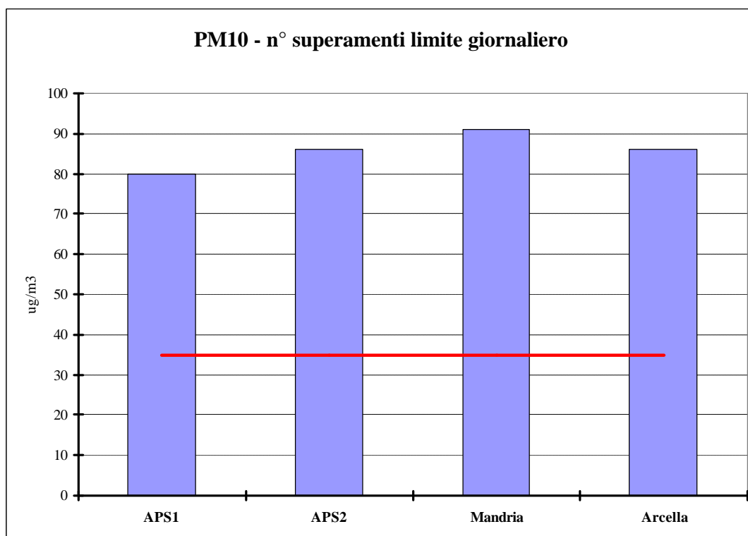
Figura 3.5 Polveri fini ( PM_{10} ). Confronto tra il numero di superamenti del valore limite di protezione della salute ( 50 \text{ } \mu\text{g}/\text{m}^3 ) rilevato nel 2012, da non superare più di 35 volte per anno civile.
