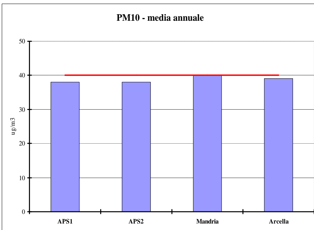
Figura 3.4 Polveri fini ( PM_{10} ). Confronto tra la concentrazione media rilevata nel 2012 e il limite annuale per la protezione della salute umana ( 40 \text{ } \mu\text{g}/\text{m}^3 ).
