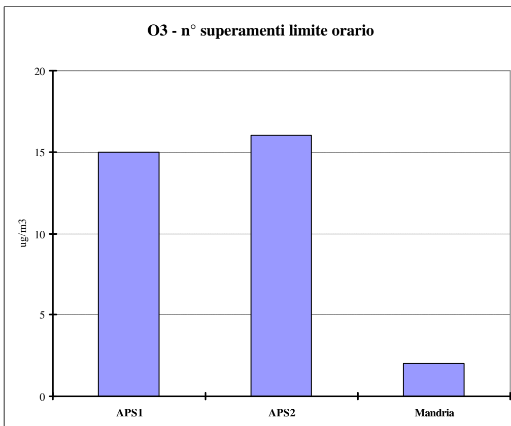
Figura 3.3 Ozono (O 3 ). Numero di superamenti della soglia di informazione (180 \mu\text{g}/\text{m}^3 , media 1h).
