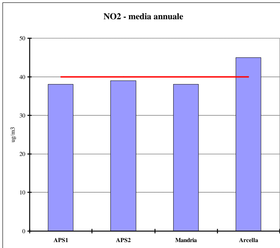
Figura 3.1 Biossido di azoto (NO 2 ). Confronto tra la concentrazione media rilevata nel 2013 e il limite annuale per la protezione della salute umana (40 µg/m 3 ).
