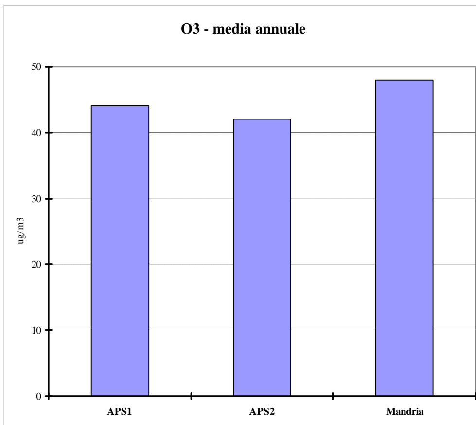
Figura 3.2 Ozono (O 3 ). Concentrazione media rilevata nel 2013.
