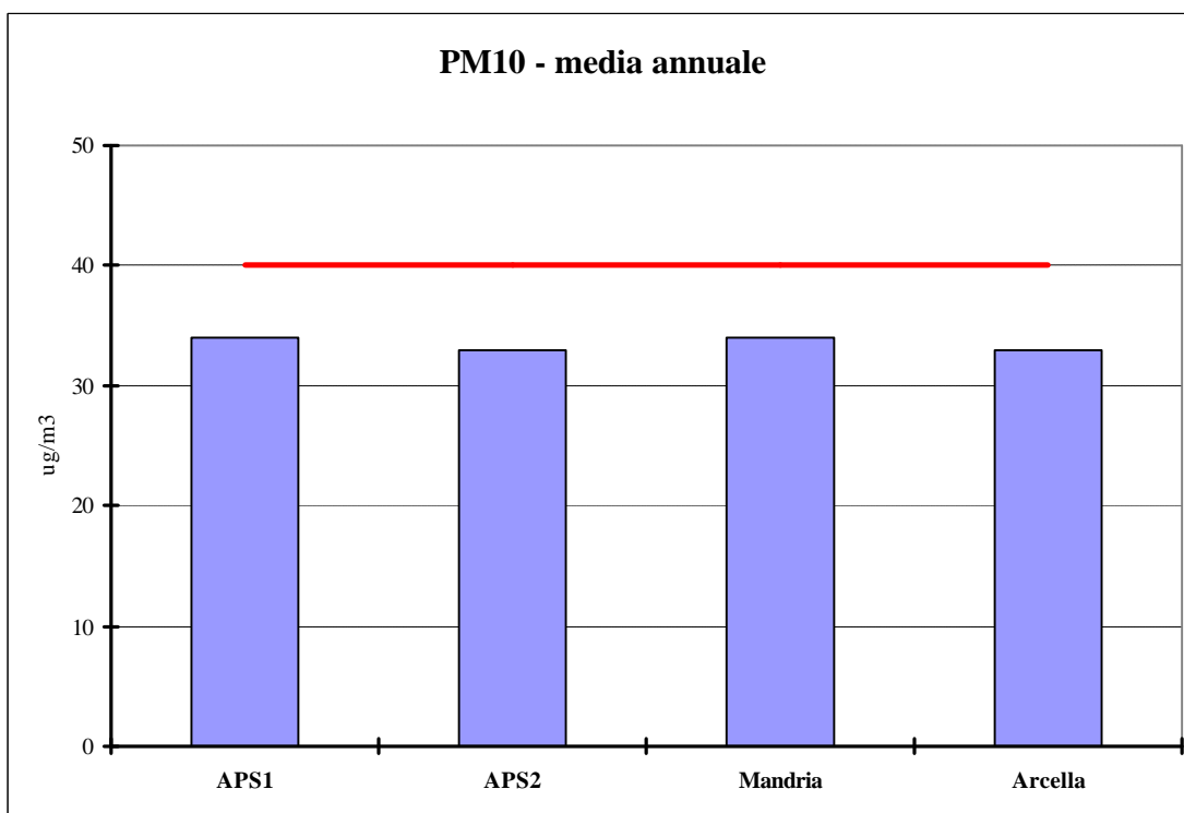
Figura 3.4 Polveri fini ( PM_{10} ). Confronto tra la concentrazione media rilevata nel 2013 e il limite annuale per la protezione della salute umana ( 40 \text{ } \mu\text{g}/\text{m}^3 ).
