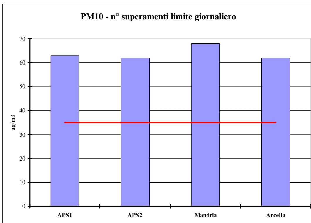
Figura 3.5 Polveri fini ( PM_{10} ). Confronto tra il numero di superamenti del valore limite di protezione della salute ( 50 \text{ } \mu\text{g}/\text{m}^3 ) rilevato nel 2013, da non superare più di 35 volte per anno civile.
