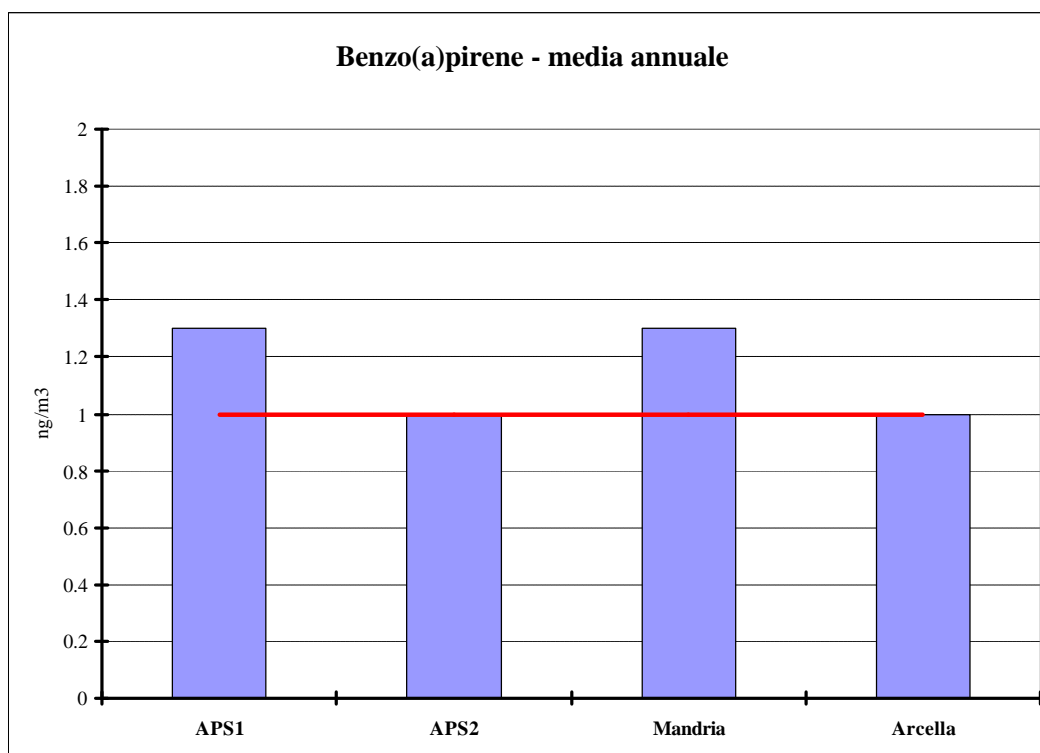
Figura 3.7 Benzo(a)pirene. Confronto tra la concentrazione media rilevata nel 2013 e il valore obiettivo (1 \text{ng}/\text{m}^3 ).
