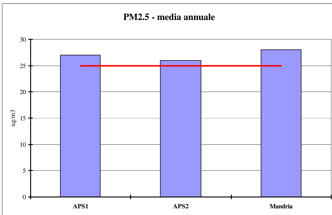
Figura 3.6 Polveri fini (PM 2.5 ). Confronto tra la concentrazione media rilevata nel 2013 e il valore obiettivo per la protezione della salute umana (25 \mu\text{g}/\text{m}^3 ).
