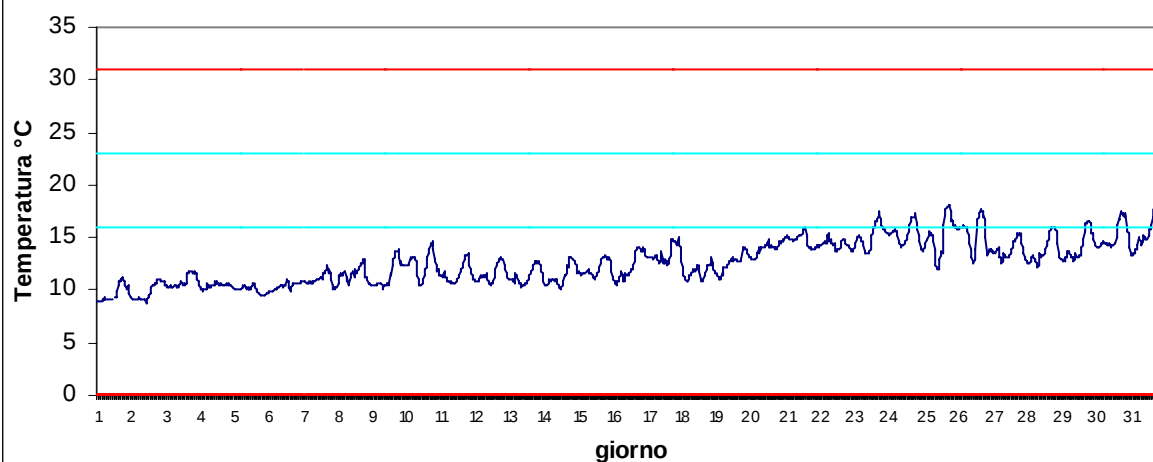
Stazione Canarin Marzo 2017 - Temperatura
