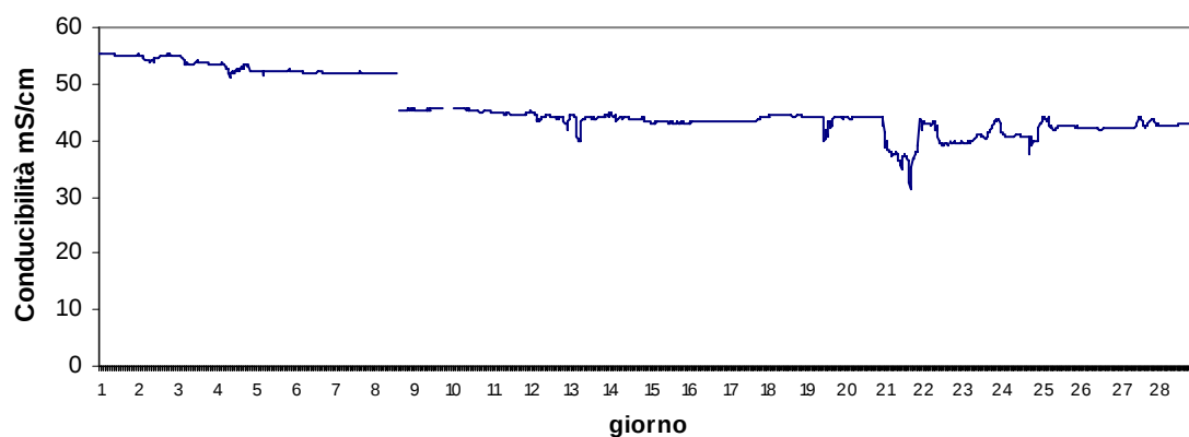
Stazione Scardovari interno Marzo 2017 - Conducibilità mS/cm
