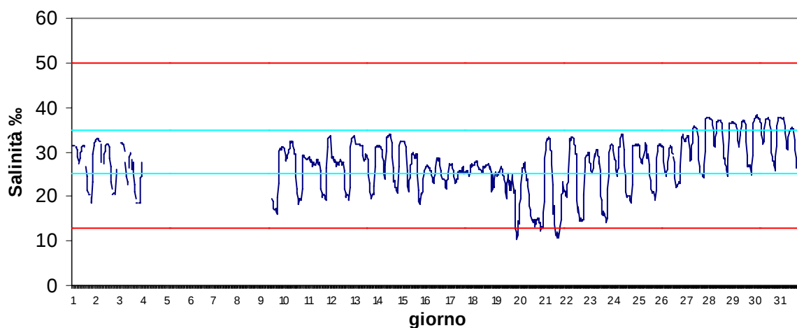
Stazione Marinetta Gennaio 2017 - Salinità ‰
