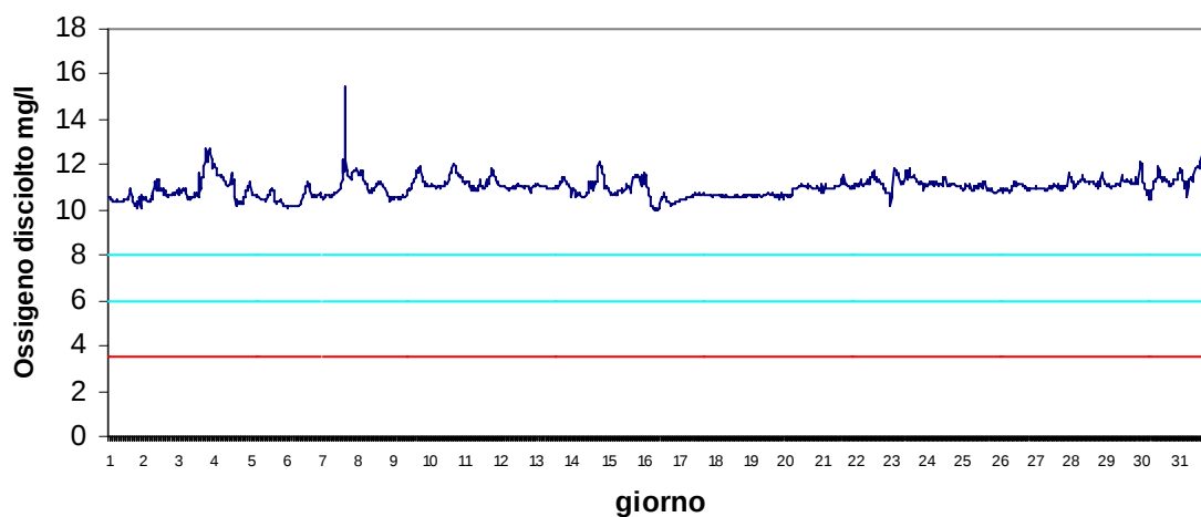
Stazione Scardovari interno Gennaio 2017 - Ossigeno disciolto mg/l
