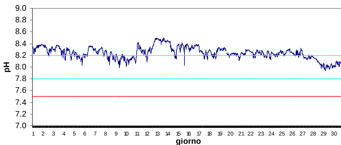
Stazione Scardovari interno Aprile 2017 - pH
