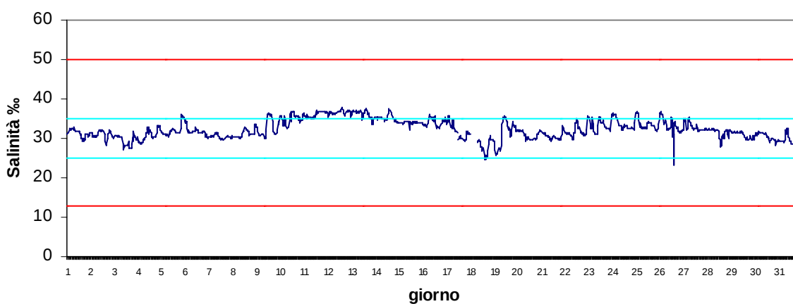
Stazione Barbamarco Settembre 2017 - Salinità ‰
