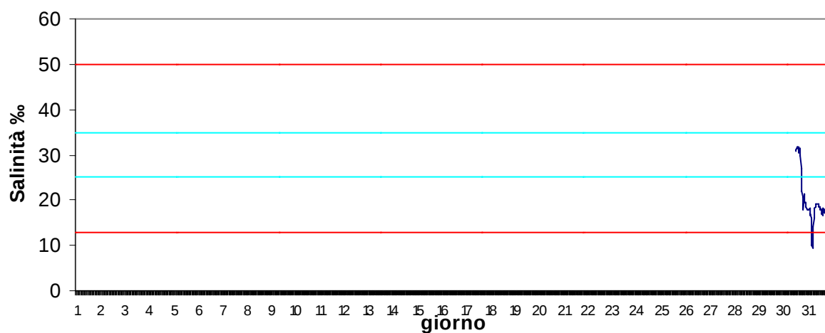
Stazione Basson Agosto 2017 - Salinità ‰
