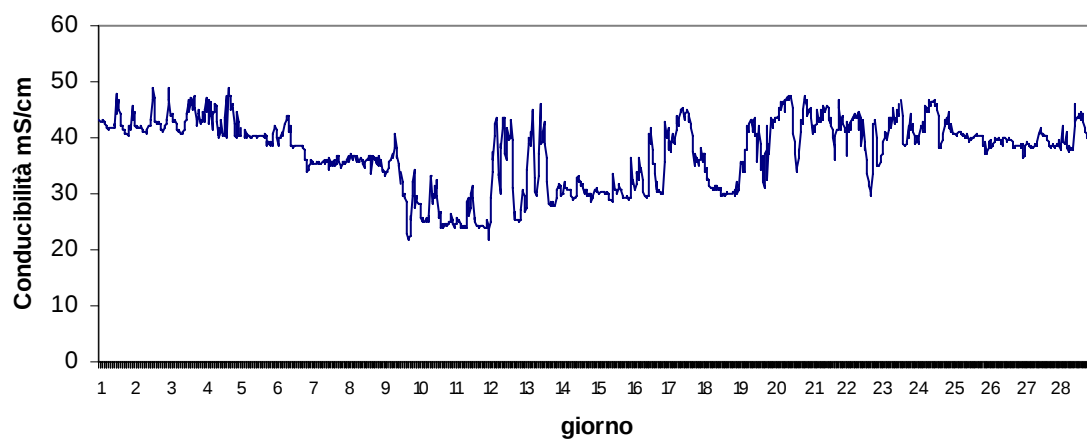
Stazione Vallona Febbraio 2017 - Conducibilità mS/cm
