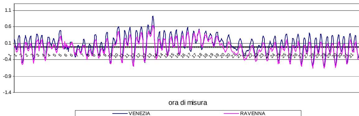
CONFRONTI CICLO di MAREA VENEZIA-RAVENNA GENNAIO 2017
