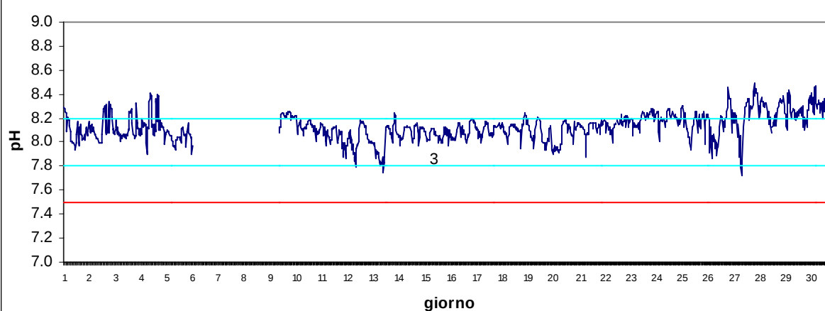
Stazione Canarin Settembre 2017 - pH
