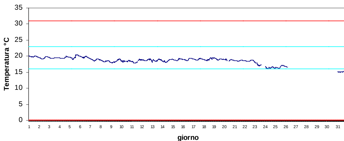
Stazione Scardovari interno Ottobre 2017 - Temperatura
