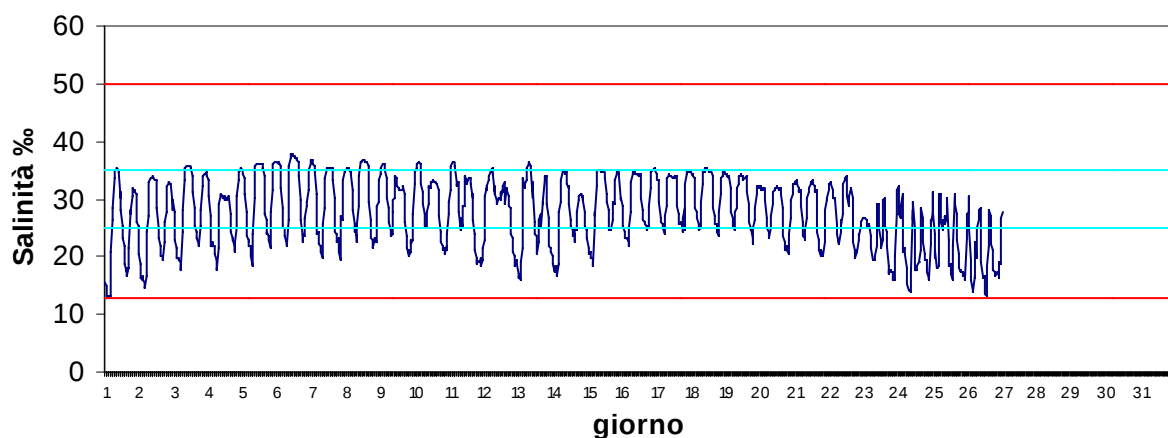
Stazione Marinetta Novembre 2017 - Salinità ‰
