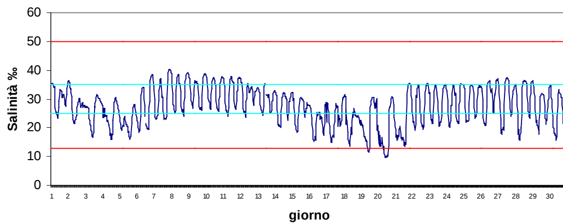
Stazione Marinetta Aprile 2017 - Salinità ‰
