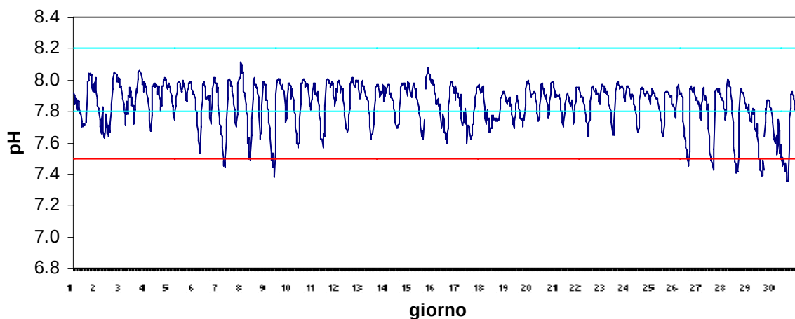
Stazione Marinetta Giugno 2017 - pH
