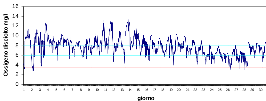
Stazione Canarin Giugno 2017 - Ossigeno disciolto mg/l
