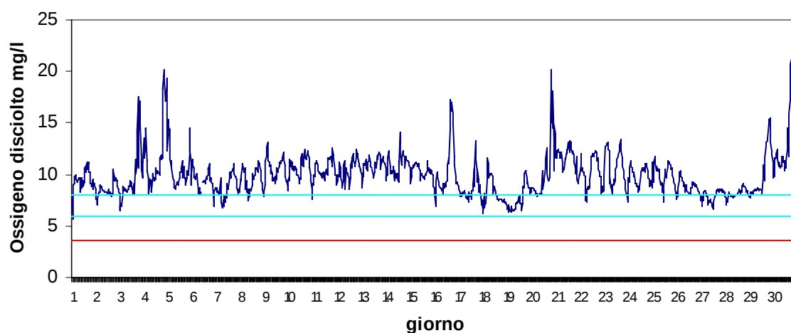
Stazione Vallona Aprile 2017 - Ossigeno disciolto mg/l
