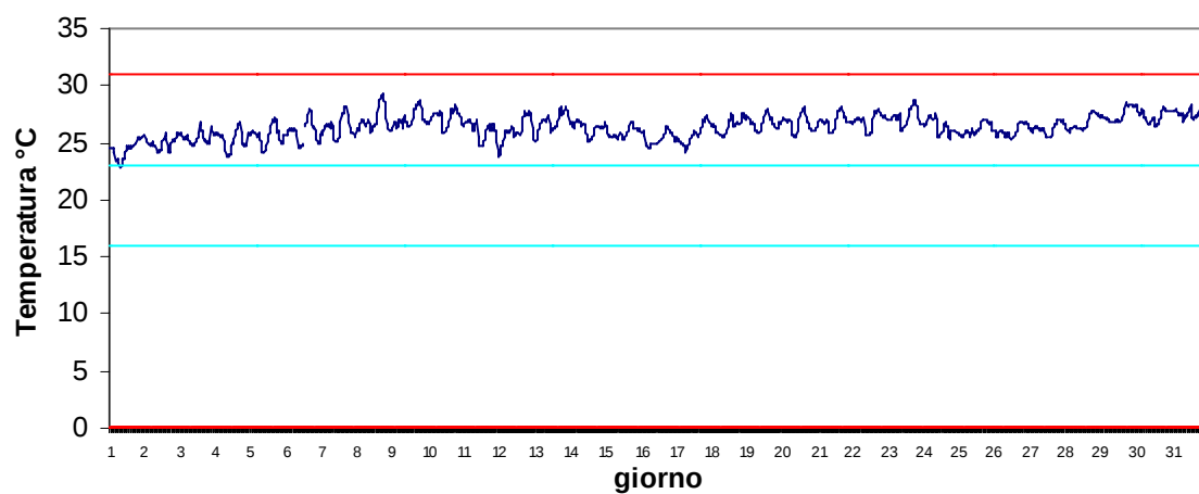
Stazione Marinetta Agosto 2017 - Temperatura
