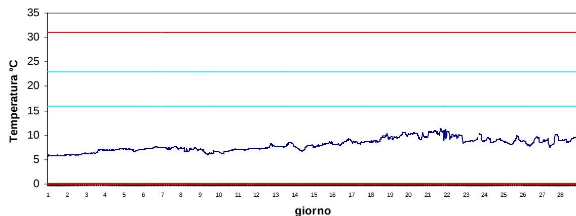
Stazione Barbamarco Febbraio 2017 - Temperatura
