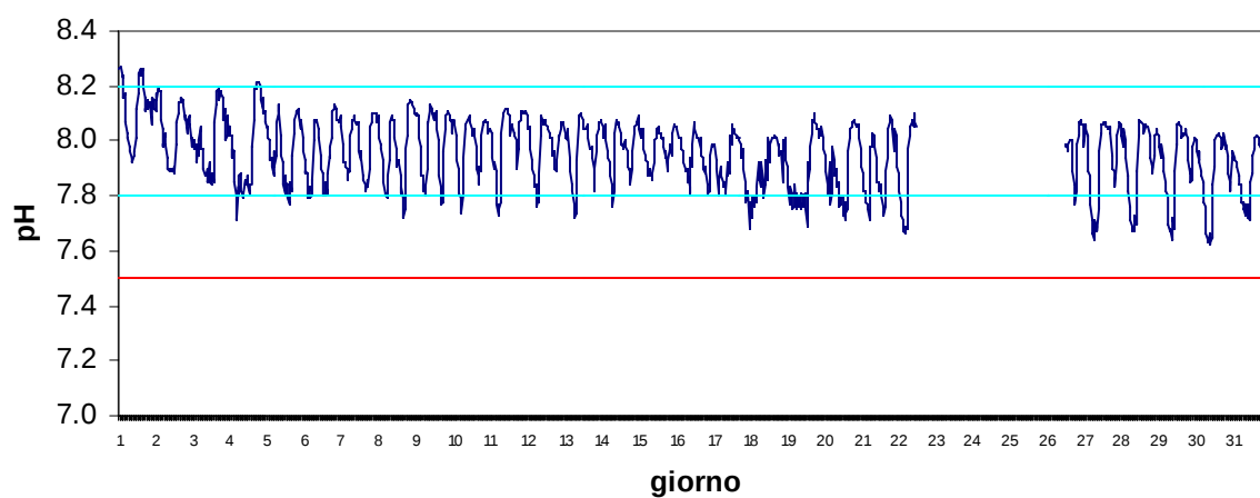
Stazione Marinetta Maggio 2017 - pH
