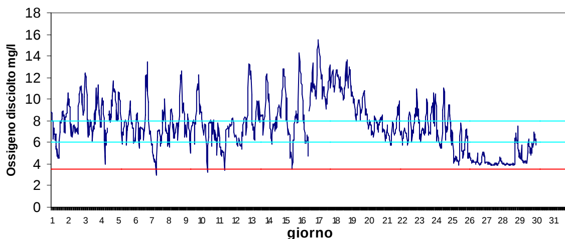
Stazione Basson Agosto 2017 - Ossigeno disciolto mg/l
