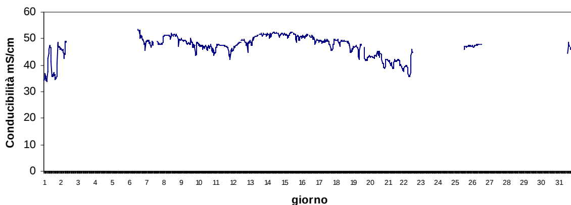
Stazione Barbamarco Novembre 2017 - Conducibilità mS/cm
