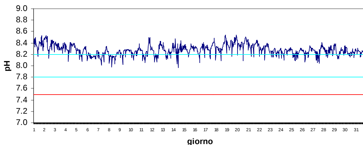
Stazione Canarin Ottobre 2017 - pH
