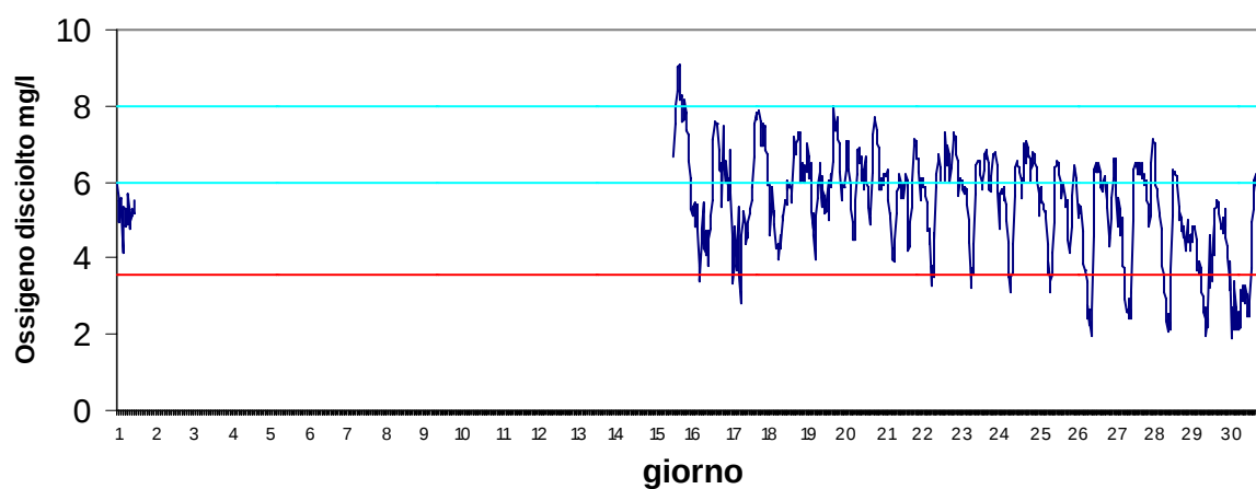
Stazione Marinetta Giugno 2017 - Ossigeno disciolto mg/l
