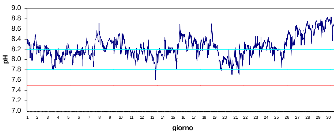
Stazione Barbamarco Settembre 2017 - pH
