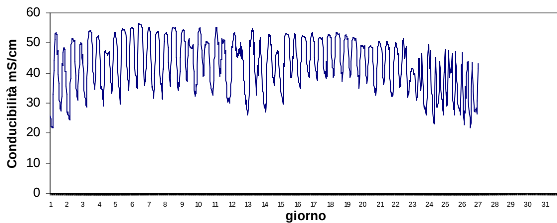
Stazione Marinetta Novembre 2017 - Conducibilità mS/cm
