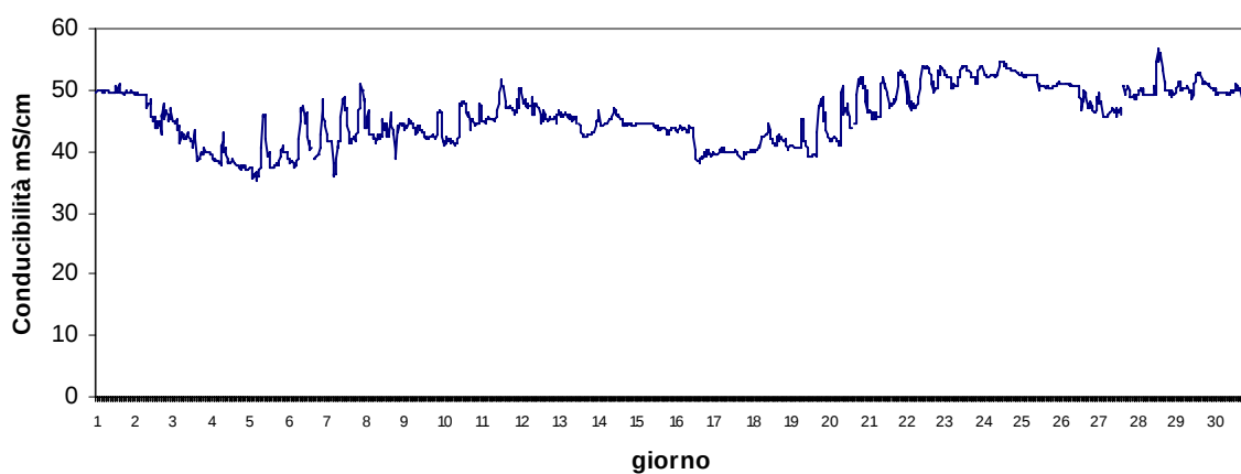
Stazione Barbamarco Agosto 2017 - Conducibilità mS/cm
