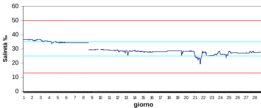
Stazione Scardovari interno Marzo 2017 - Salinità ‰
