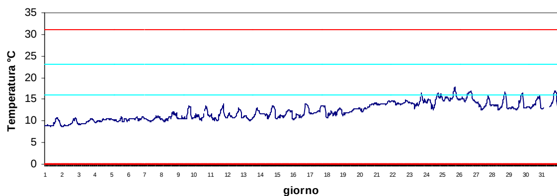
Stazione Barbamarco Marzo 2017 - Temperatura
