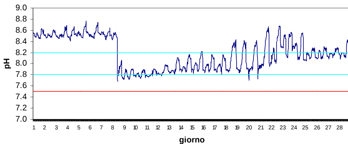
Stazione Basson Febbraio 2017 - pH
