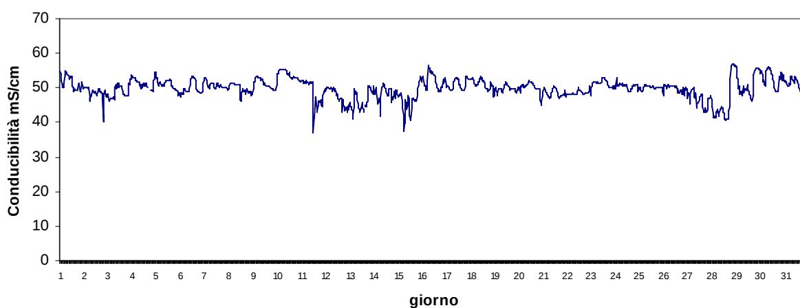
Stazione Scardovari mare Dicembre 2017 - Conducibilità mS/cm
