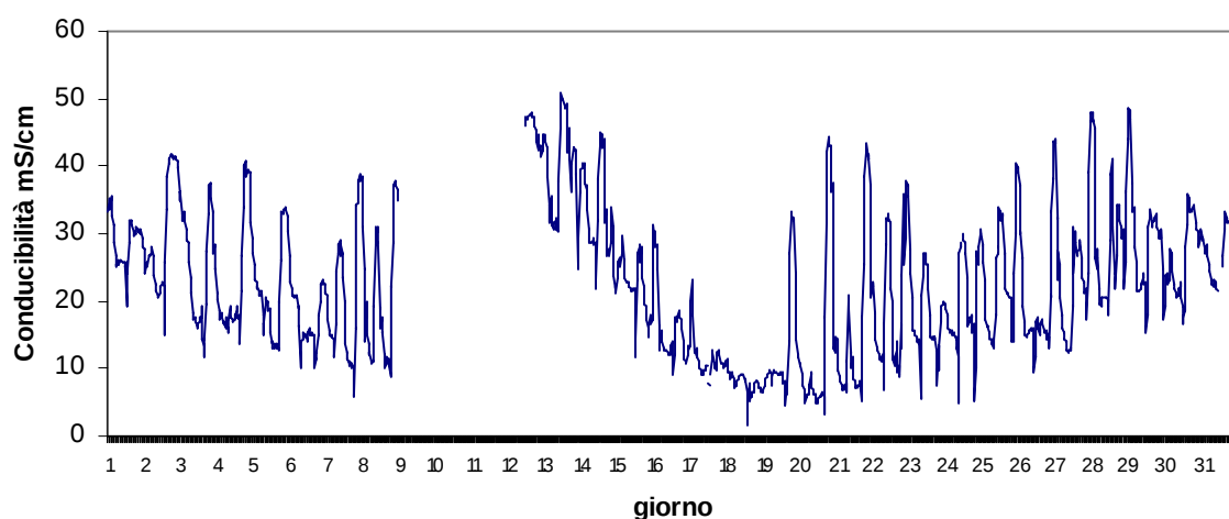
Stazione Basson Maggio 2017 - Conducibilità mS/cm
