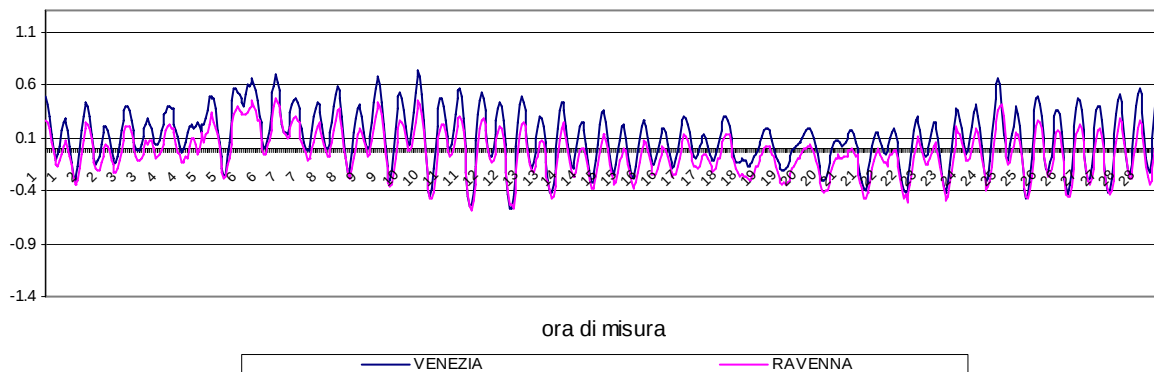
CONFRONTI CICLO di MAREA VENEZIA-RAVENNA FEBBRAIO 2017
