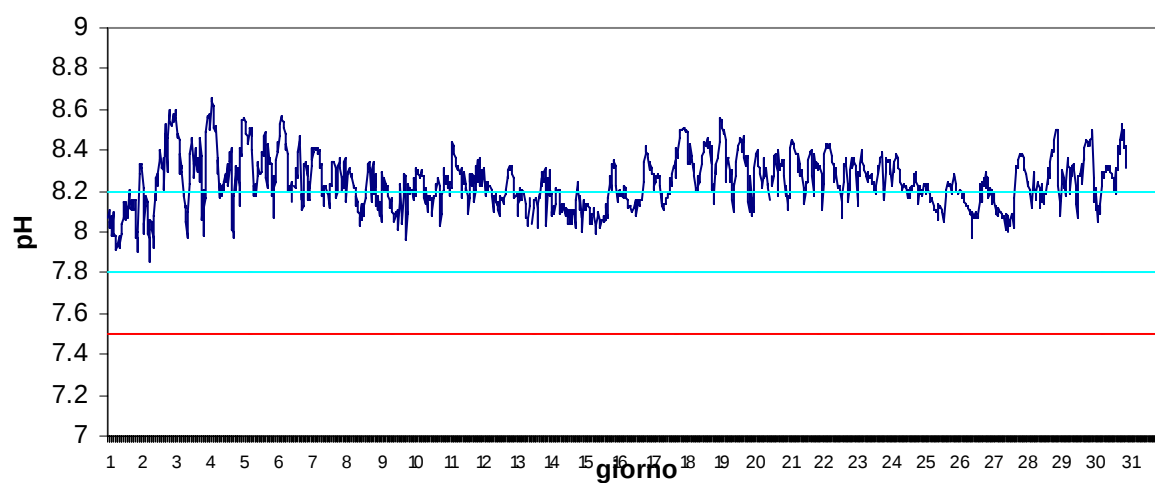
Stazione Vallona Luglio 2017 - pH
