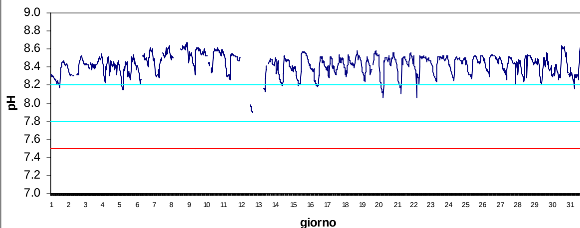
Stazione Scardovari mare Agosto 2017 - pH
