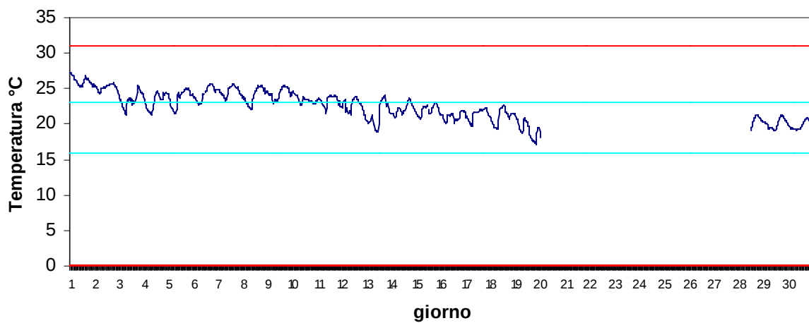
Stazione Basson Settembre 2017 - Temperatura
