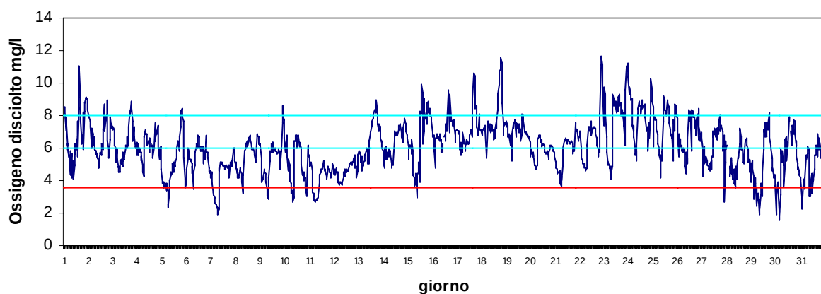
Stazione Scardovari mare Agosto 2017 - Ossigeno disciolto mg/l
