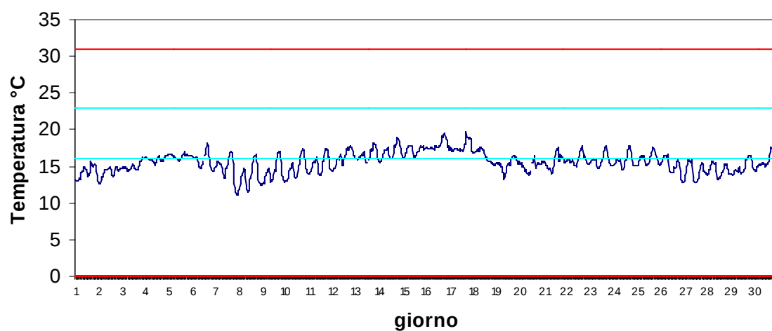
Stazione Marinetta Aprile 2017 - Temperatura
