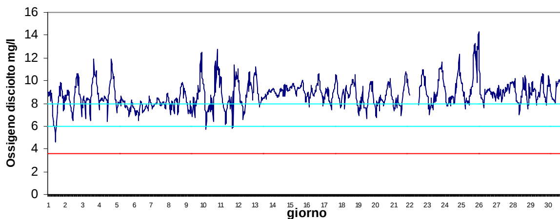
Stazione Canarin Dicembre 2017 - Ossigeno disciolto mg/l
