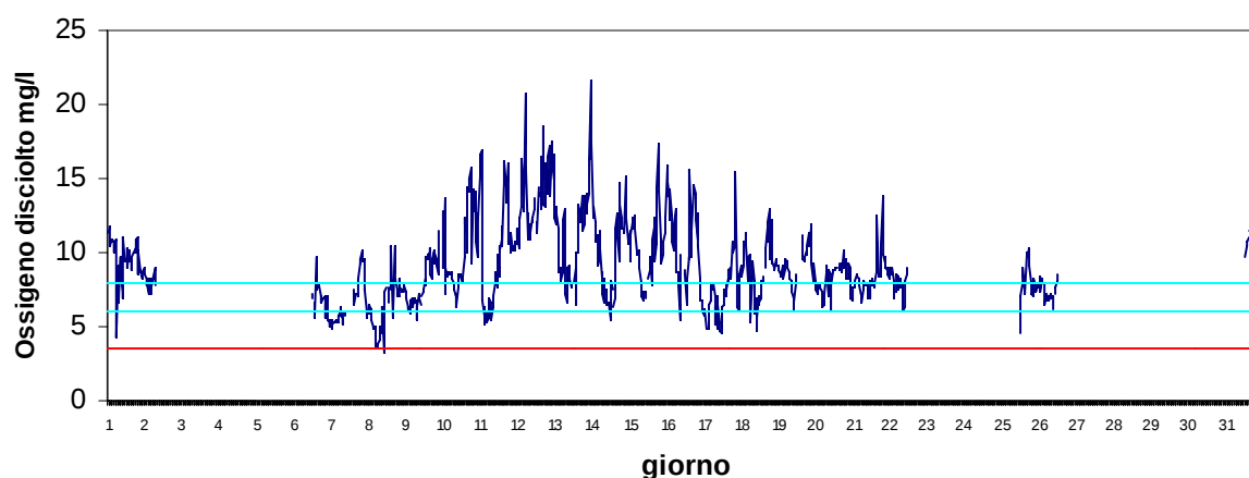
Stazione Barbamarco Ottobre 2017 - Ossigeno disciolto mg/l
