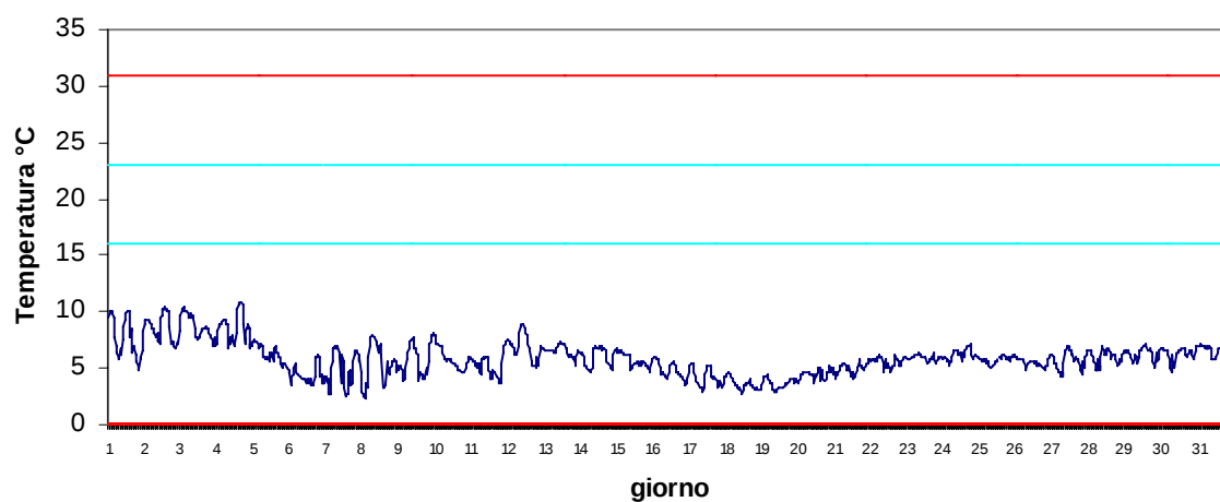
Stazione Canarin Febbraio 2017 - Temperatura
