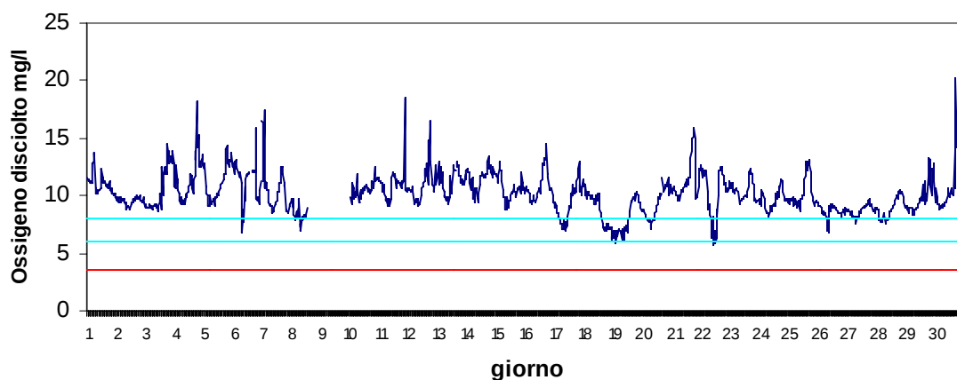
Stazione Barbamarco Aprile 2017 - Ossigeno disciolto mg/l
