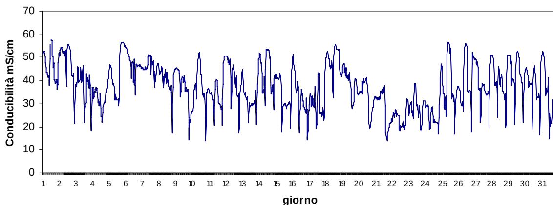
Stazione Canarin Marzo 2017 - Conducibilità mS/cm
