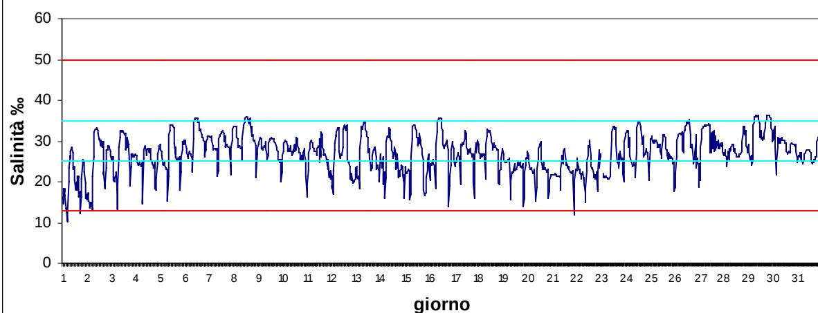
Stazione Canarin Ottobre 2017 - Salinità ‰
