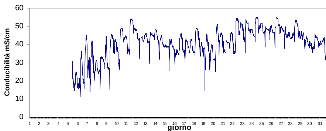
Stazione Canarin Agosto 2017 - Conducibilità mS/cm
