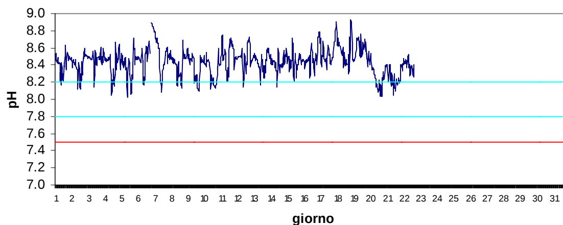
Stazione Barbamarco Giugno 2017 - pH
