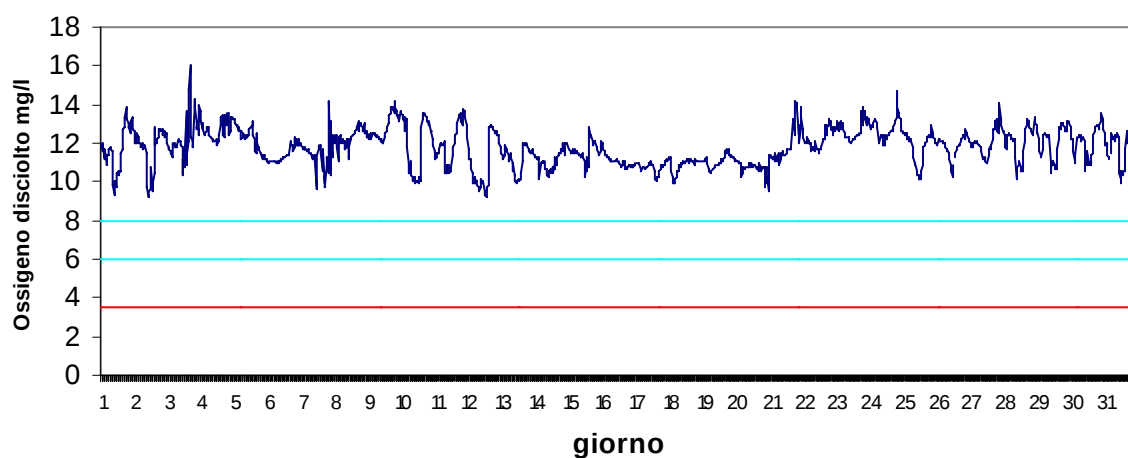
Stazione Vallona Febbraio 2017 - Ossigeno disciolto mg/l
