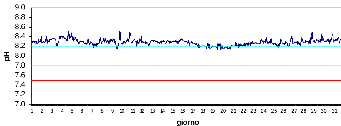
Stazione Barbamarco Gennaio 2017 - pH
