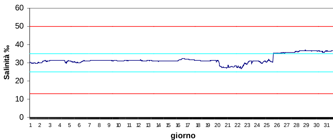
Stazione Scardovari interno Febbraio 2017 - Salinità ‰
