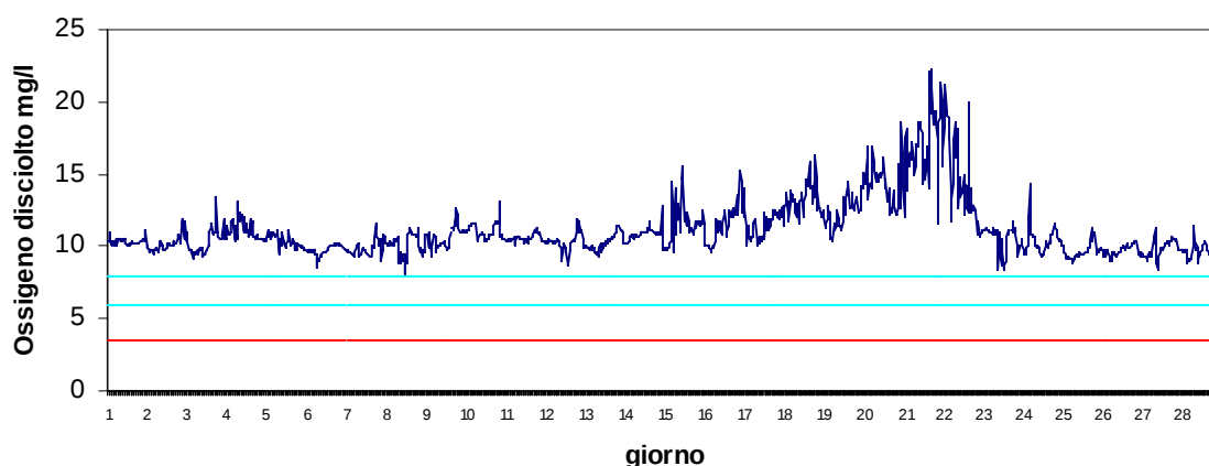
Stazione Barbamarco Marzo 2017 - Ossigeno disciolto mg/l
