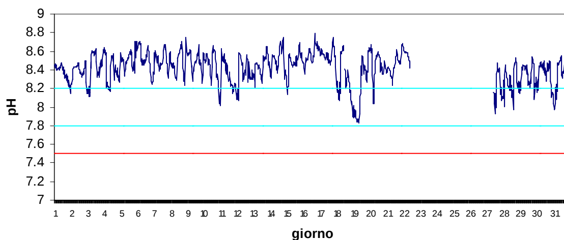
Stazione Vallona Maggio 2017 - pH
