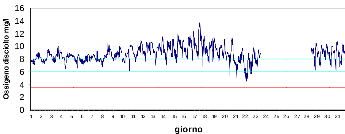
Stazione Marinetta Marzo 2017 - Ossigeno disciolto mg/l
