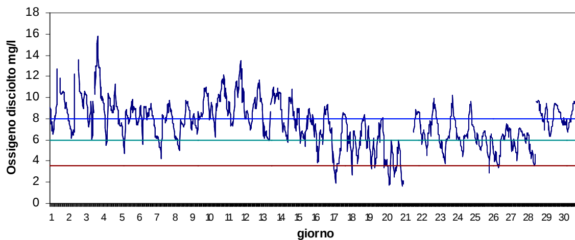
Stazione Basson Giugno 2017 - Ossigeno disciolto mg/l
