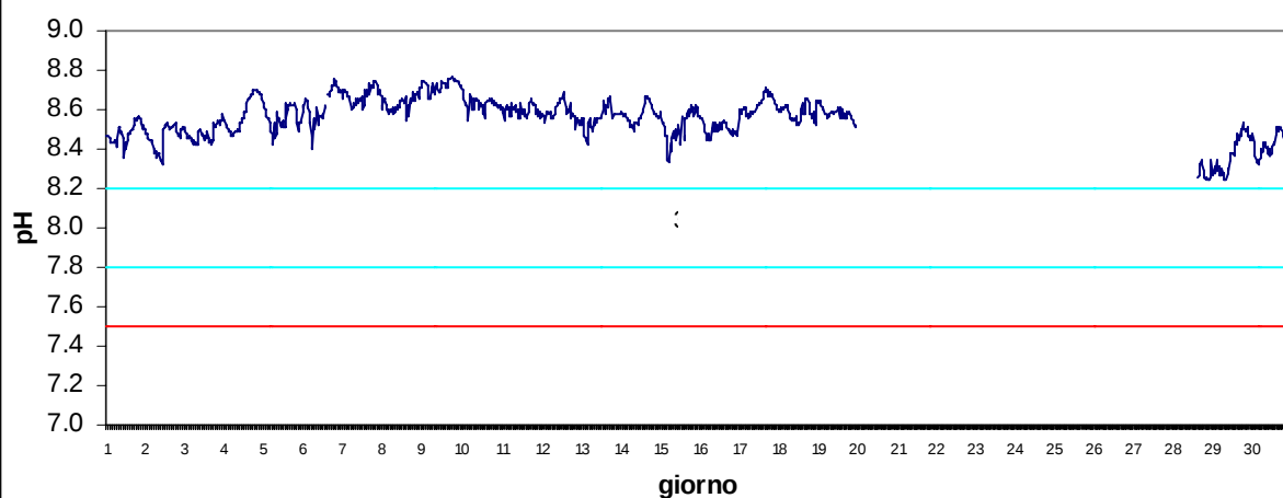
Stazione Scardovari interno Settembre 2017 - pH
