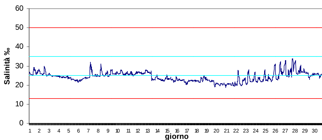
Stazione Vallona Aprile 2017 - Salinità ‰
