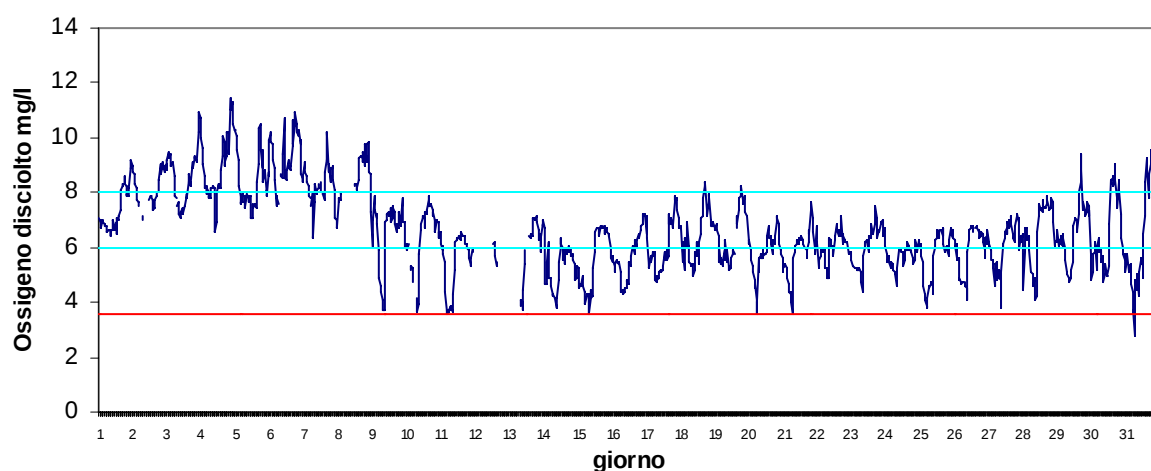
Stazione Scardovari mare Luglio 2017 - Ossigeno disciolto mg/l
