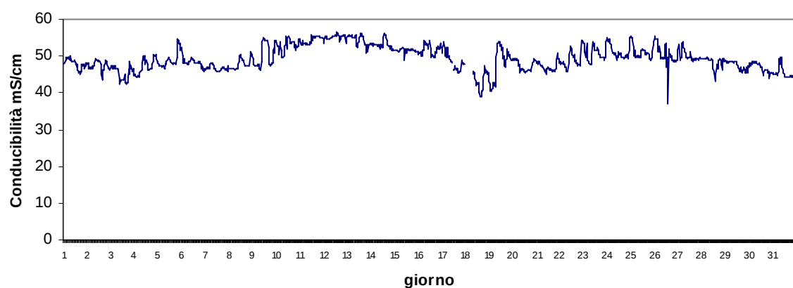
Stazione Barbamarco Settembre 2017 - Conducibilità mS/cm
