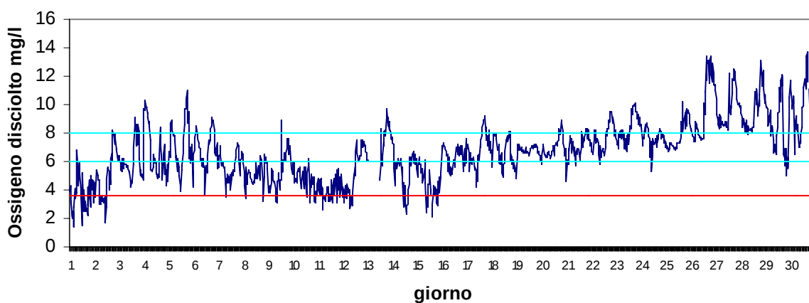
Stazione Vallona Settembre 2017 - Ossigeno disciolto mg/l
