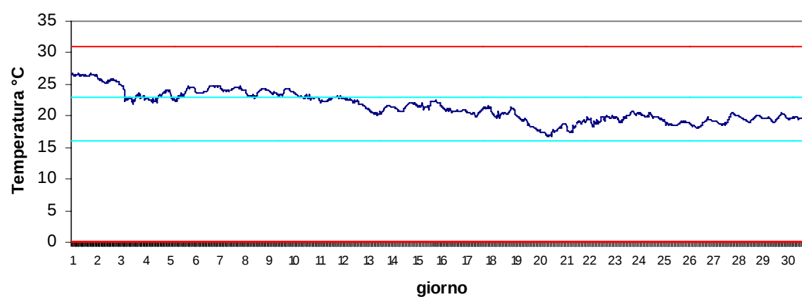
Stazione Vallona Settembre 2017 - Temperatura
