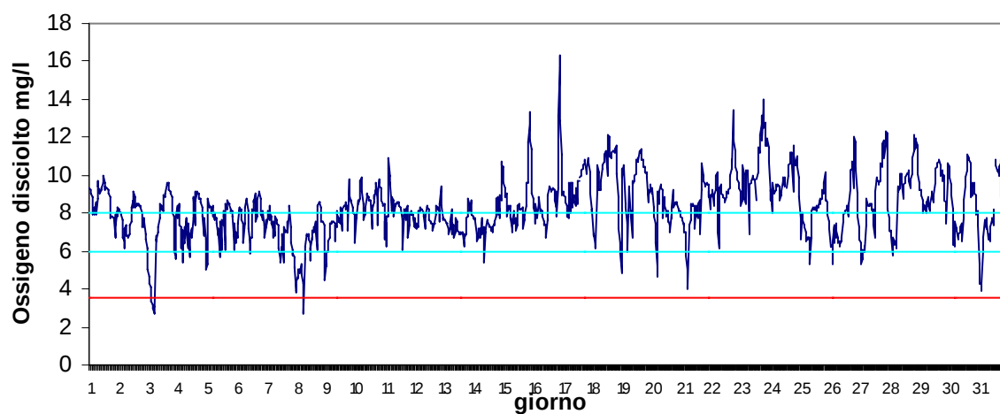
Stazione Canarin Maggio 2017 - Ossigeno disciolto mg/l
