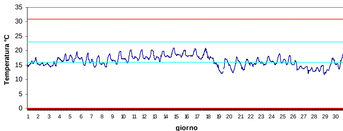
Stazione Basson Maggio 2017 - Temperatura
