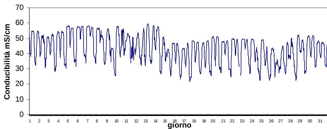
Stazione Marinetta Dicembre 2017 - Conducibilità mS/cm
