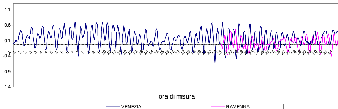
CONFRONTI CICLO di MAREA VENEZIA-RAVENNA AGOSTO 2017
