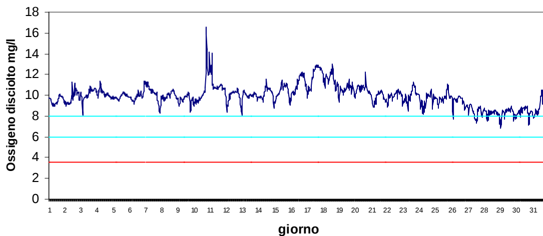
Stazione Scardovari interno Marzo 2017 - Ossigeno disciolto mg/l
