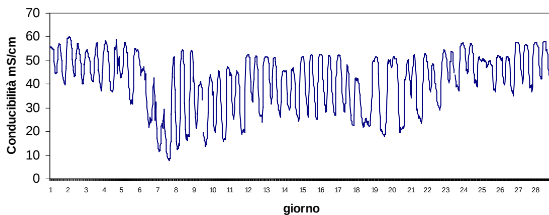
Stazione Marinetta Febbraio 2017 - Conducibilità mS/cm
