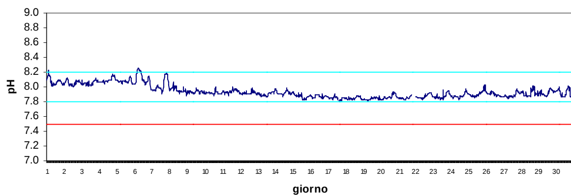
Stazione Scardovari mare Novembre 2017 - pH
