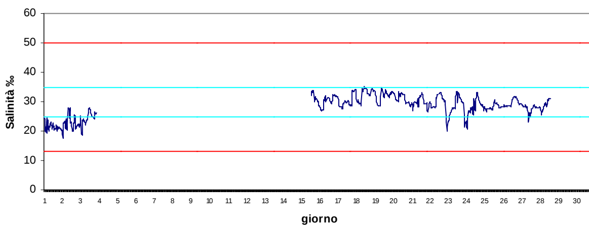
Stazione Scardovari mare Settembre 2017 - Salinità ‰
