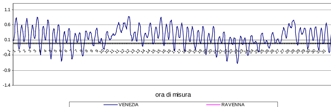
CONFRONTI CICLO di MAREA VENEZIA-RAVENNA DICEMBRE 2017
