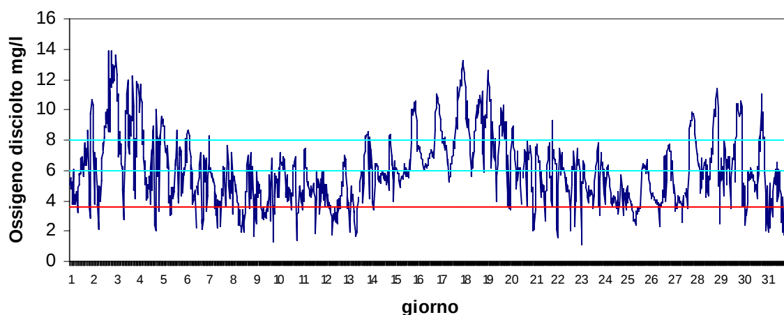
Stazione Vallona Luglio 2017 - Ossigeno disciolto mg/l
