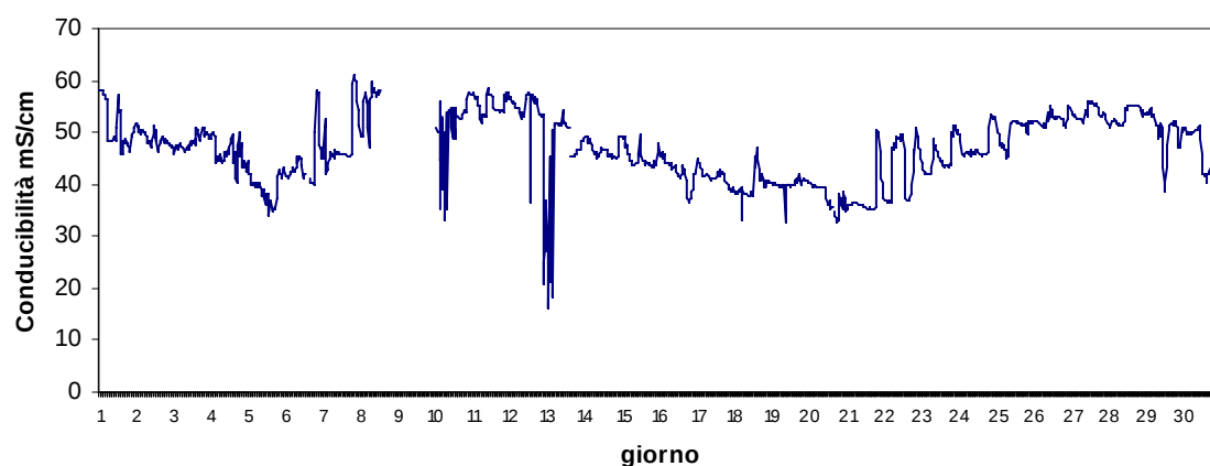
Stazione Barbamarco Maggio 2017 - Conducibilità mS/cm
