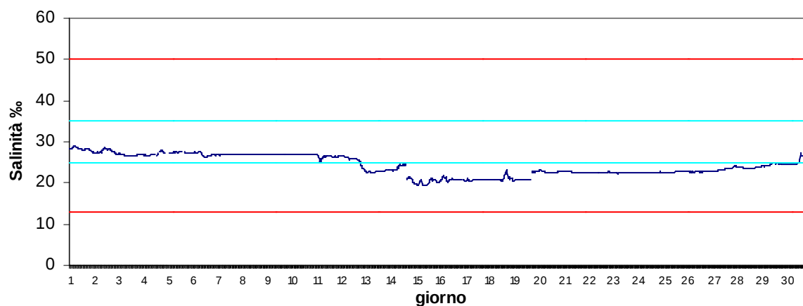
Stazione Scardovari interno Maggio 2017 - Salinità ‰
