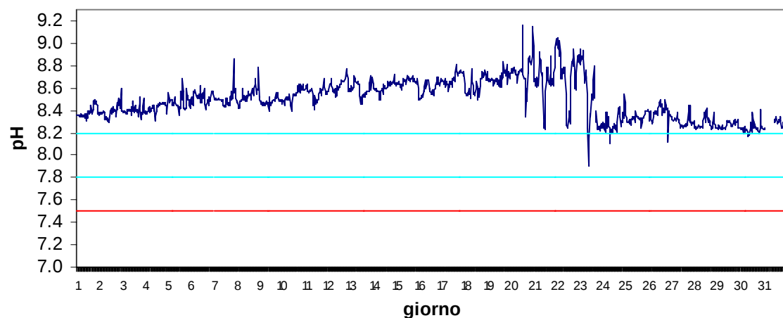
Stazione Barbamarco Marzo 2017 - pH
