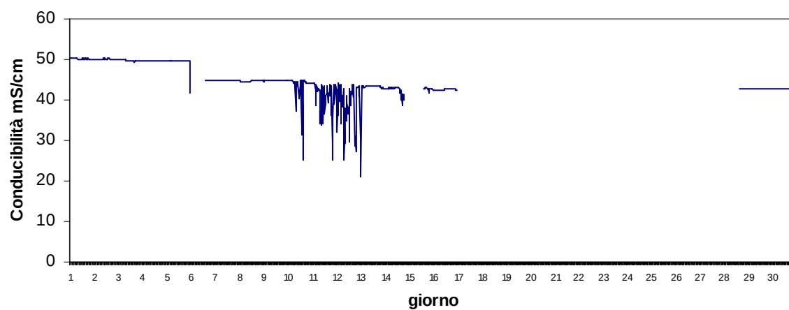
Stazione Scardovari interno Settembre 2017 - Conducibilità mS/cm
