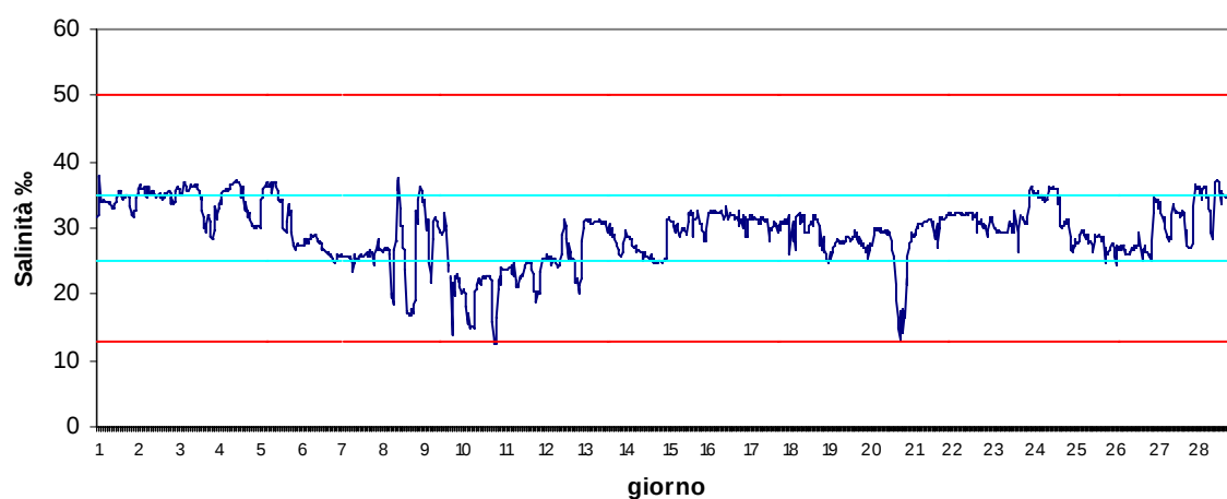
Stazione Barbamarco Marzo 2017 - Salinità ‰
