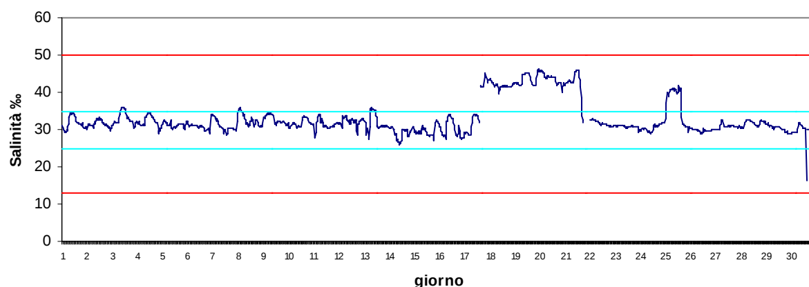
Stazione Scardovari mare Novembre 2017 - Salinità ‰
