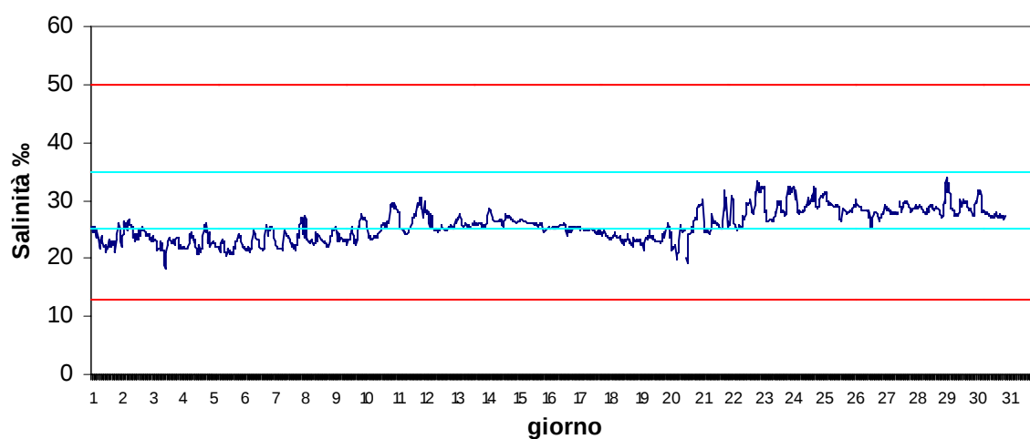
Stazione Vallona Luglio 2017 - Salinità ‰
