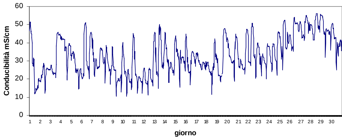
Stazione Canarin Aprile 2017 - Conducibilità mS/cm
