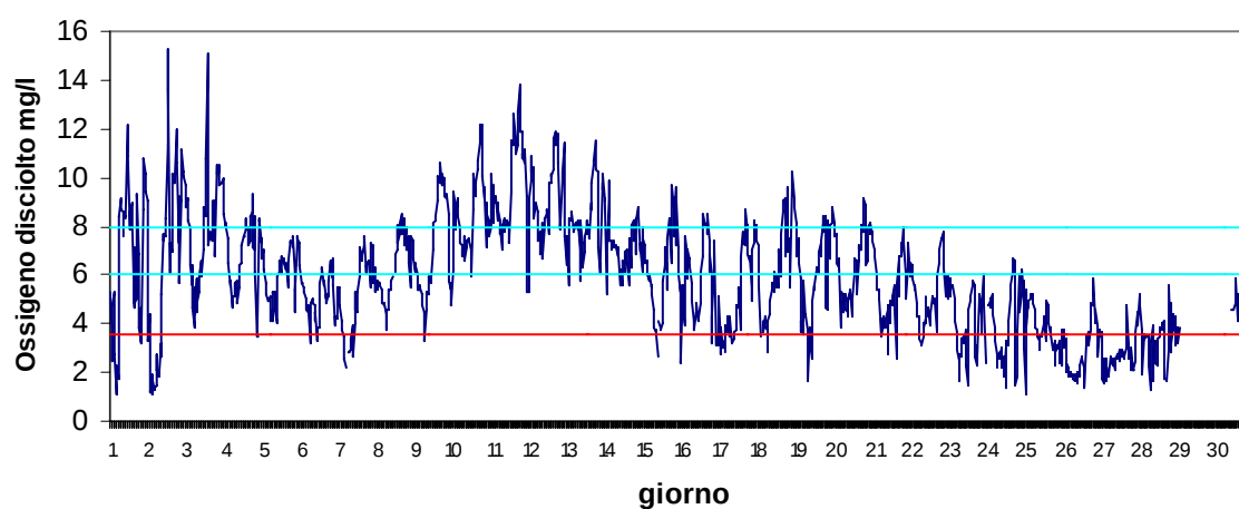
Stazione Vallona Giugno 2017 - Ossigeno disciolto mg/l
