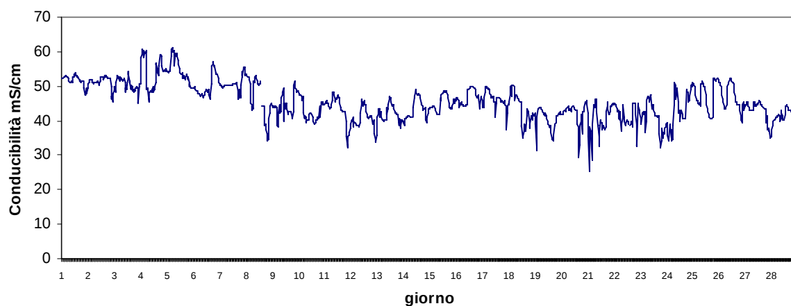
Stazione Scardovari mare Febbraio 2017 - Conducibilità mS/cm
