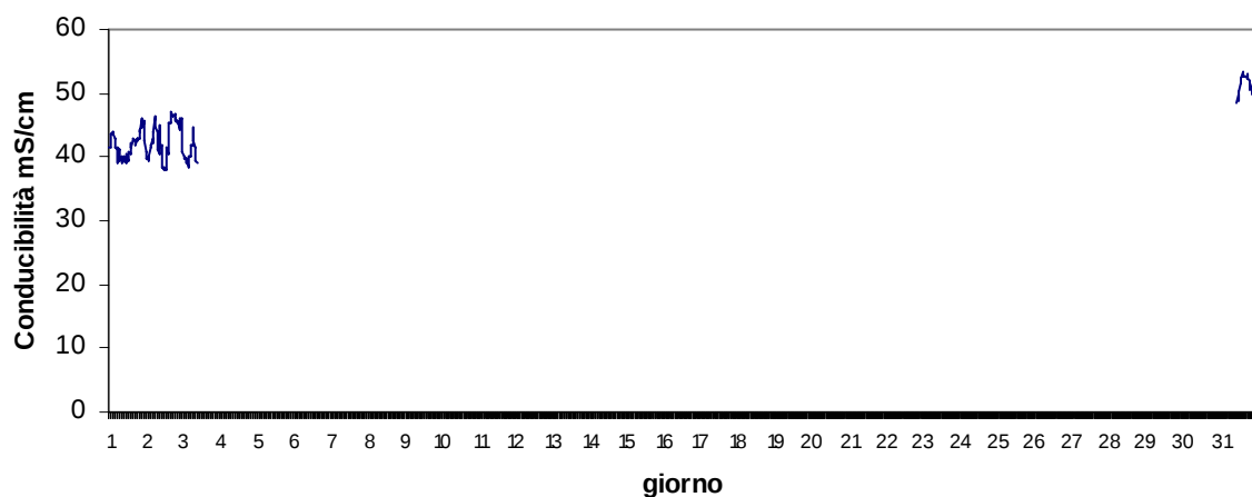
Stazione Vallona Settembre 2017 - Conducibilità mS/cm
