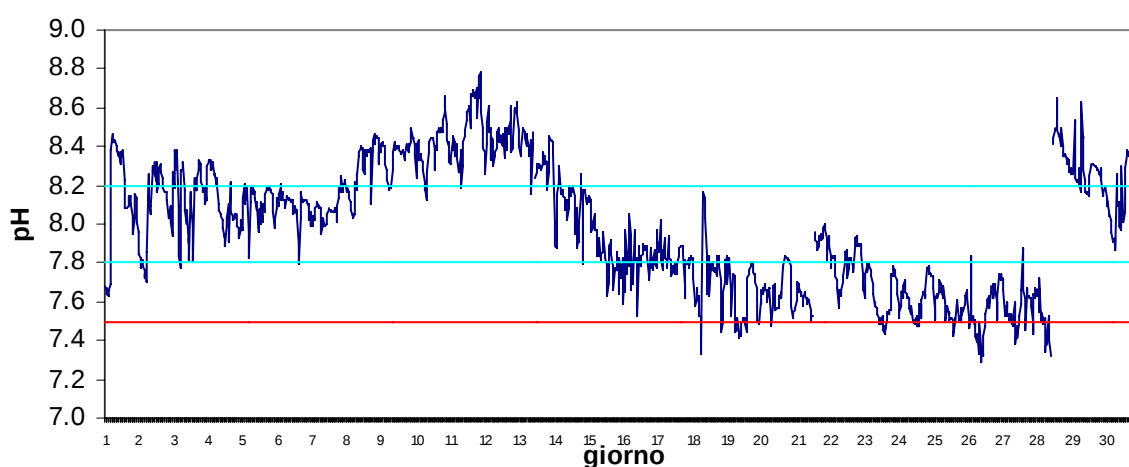
Stazione Canarin Giugno 2017 - pH
