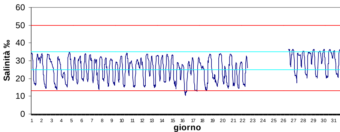
Stazione Marinetta Maggio 2017 - Salinità ‰
