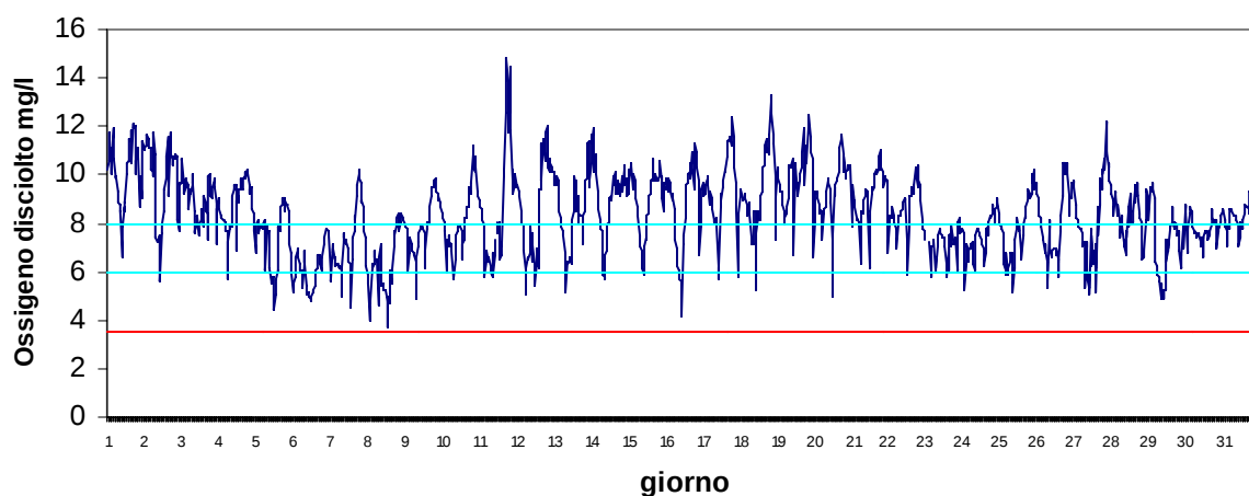
Stazione Canarin Ottobre 2017 - Ossigeno disciolto mg/l
