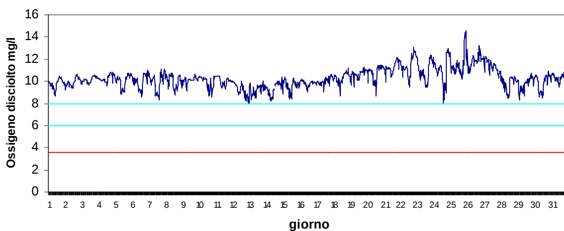
Stazione Vallona Dicembre 2017 - Ossigeno disciolto mg/l
