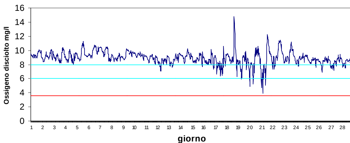
Stazione Marinetta Marzo 2017 - Ossigeno disciolto mg/l
