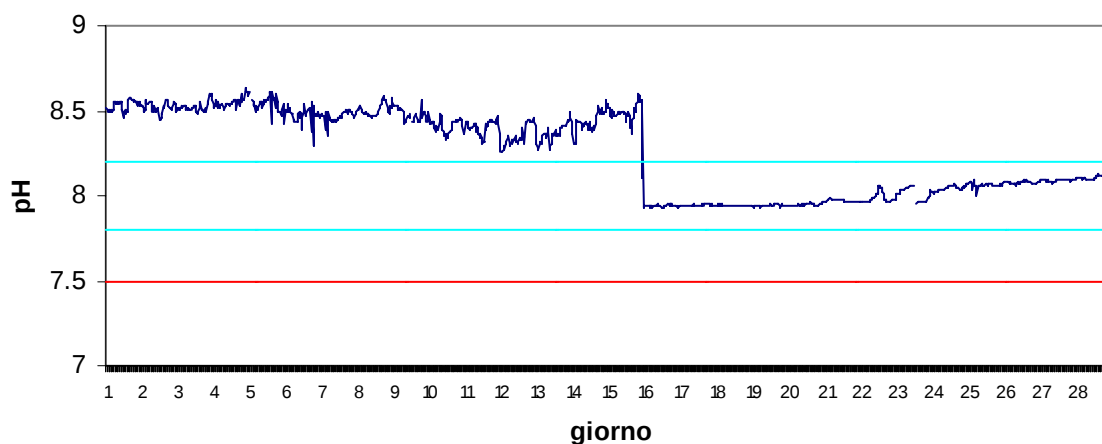
Stazione Vallona Marzo 2017 - pH
