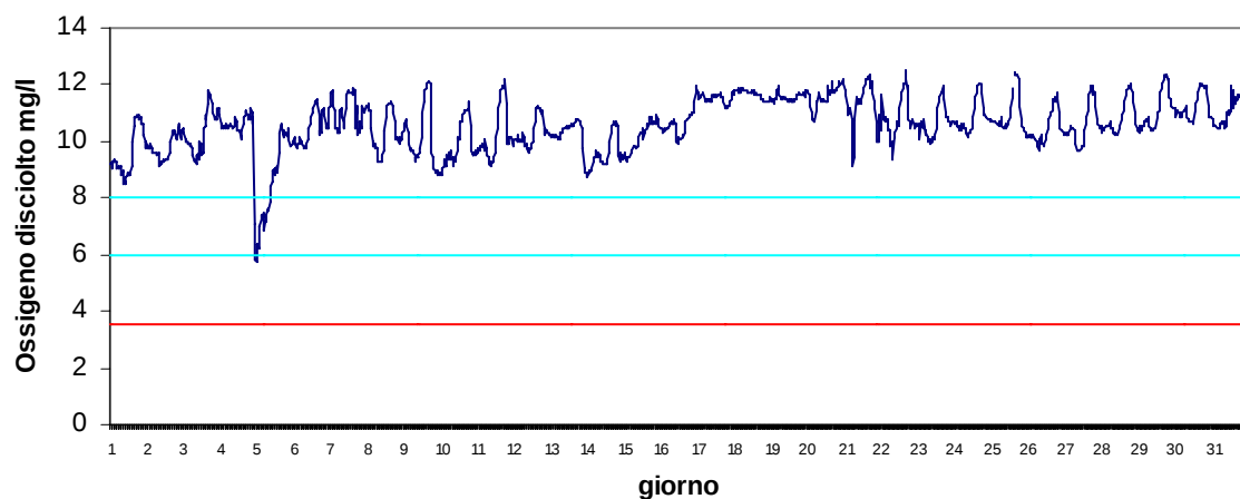
Stazione Scardovari mare Febbraio 2017 - Ossigeno disciolto mg/l
