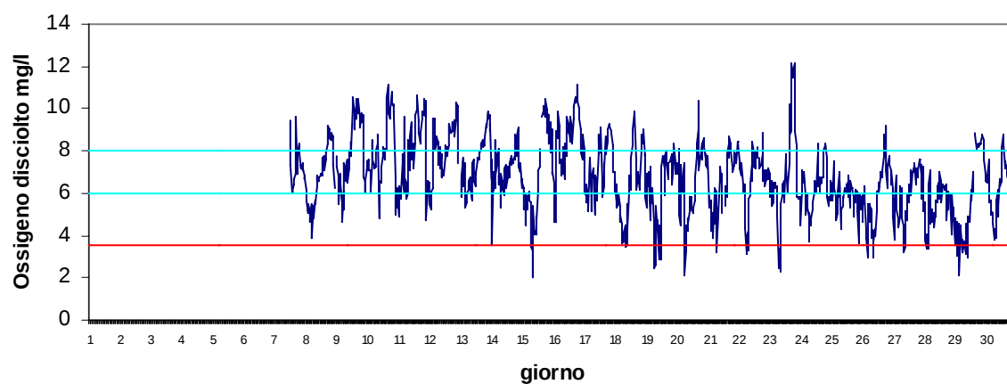
Stazione Barbamarco Giugno 2017 - Ossigeno disciolto mg/l
