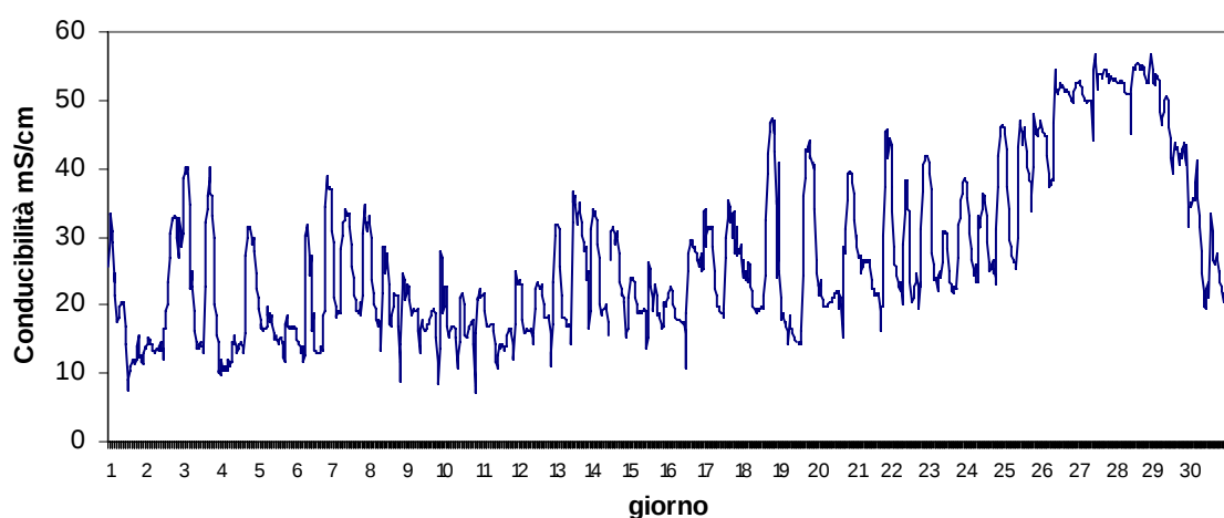
Stazione Basson Aprile 2017 - Conducibilità mS/cm
