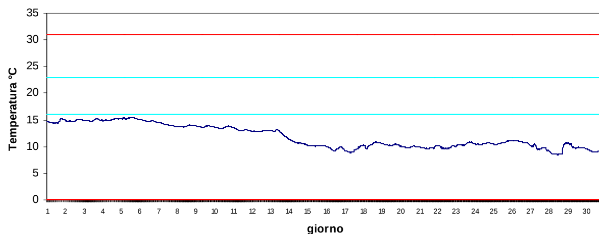
Stazione Scardovari interno Novembre 2017 - Temperatura
