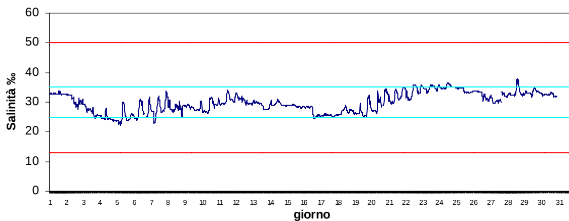
Stazione Barbamarco Agosto 2017 - Salinità ‰
