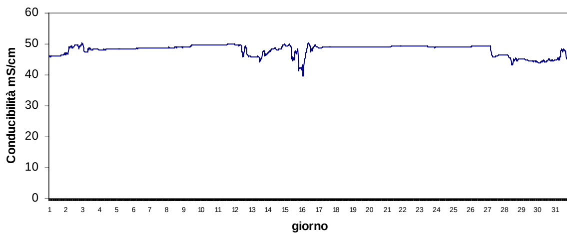
Stazione Scardovari interno Dicembre 2017 - Conducibilità mS/cm
