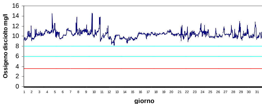
Stazione Barbamarco Febbraio 2017 - Ossigeno disciolto mg/l
