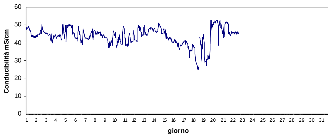
Stazione Barbamarco Giugno 2017 - Conducibilità mS/cm
