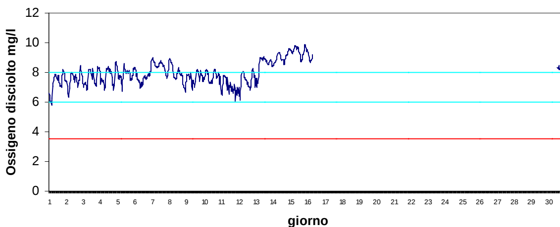
Stazione Marinetta Dicembre 2017 - Ossigeno disciolto mg/l
