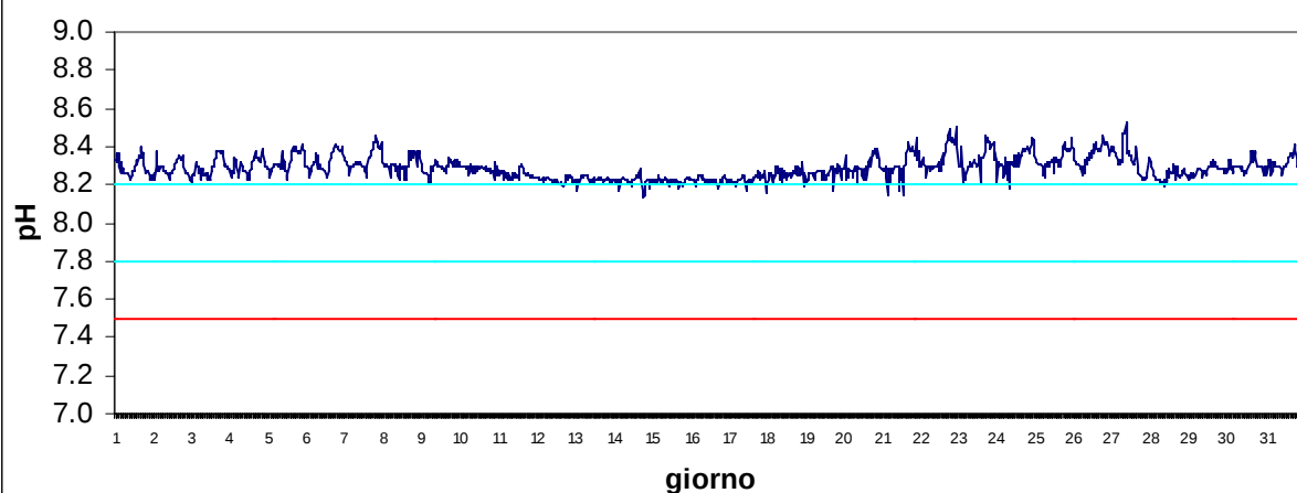
Stazione Canarin Dicembre 2017 - pH
