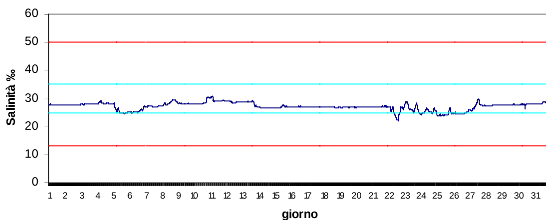
Stazione Scardovari interno Marzo 2017 - Salinità ‰
