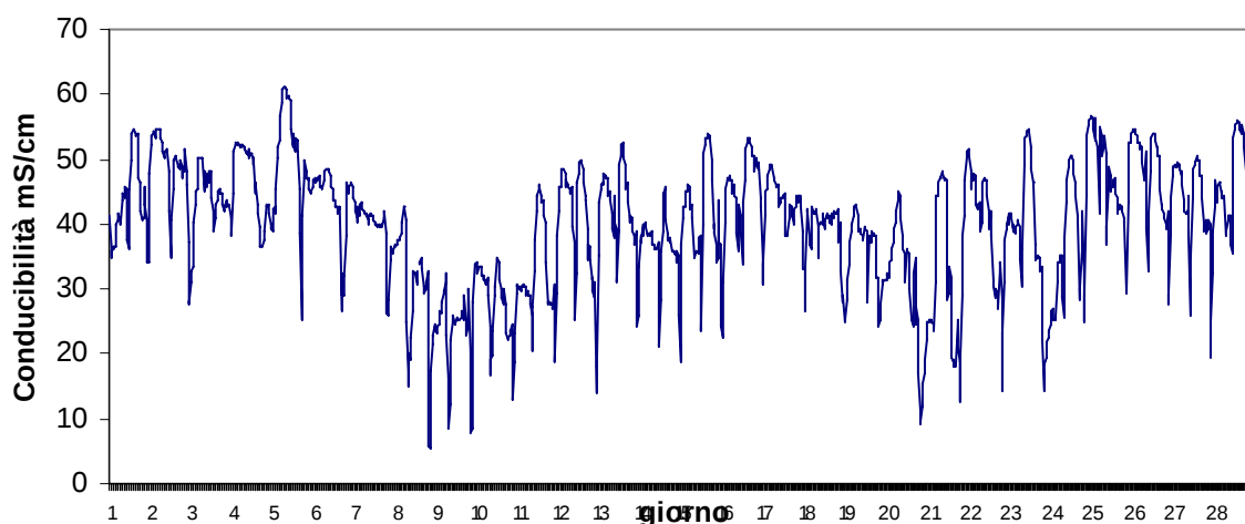
Stazione Canarin Febbraio 2017 - Conducibilità mS/cm
