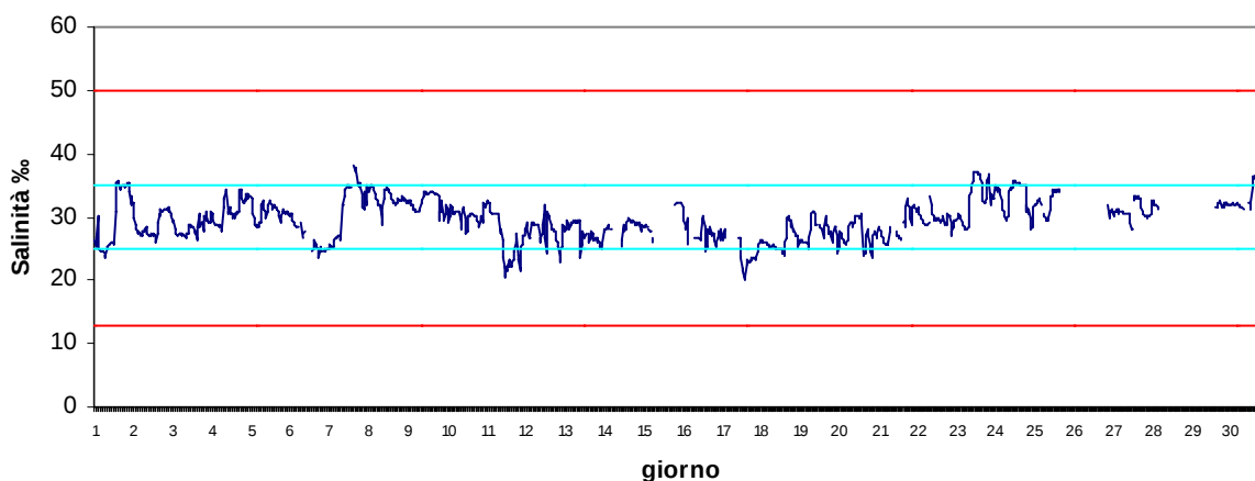
Stazione Scardovari mare Giugno 2017 - Salinità ‰
