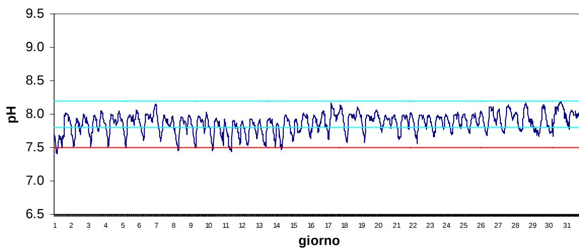
Stazione Marinetta Agosto 2017 - pH
