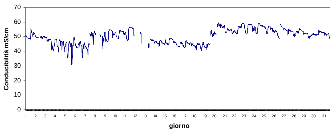
Stazione Scardovari mare Luglio 2017 - Conducibilità mS/cm
