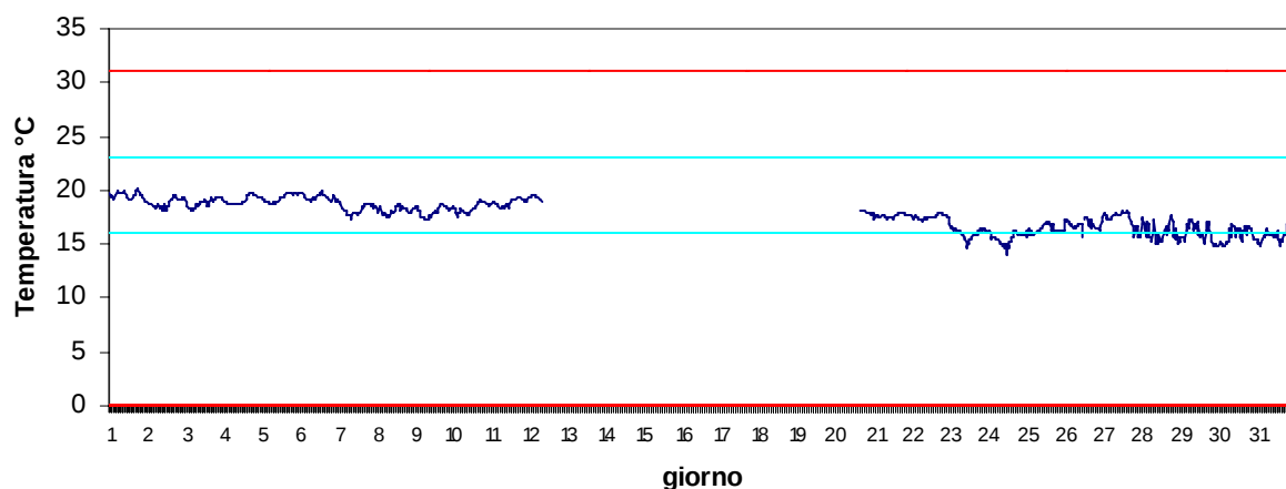
Stazione Vallona Ottobre 2017 - Temperatura
