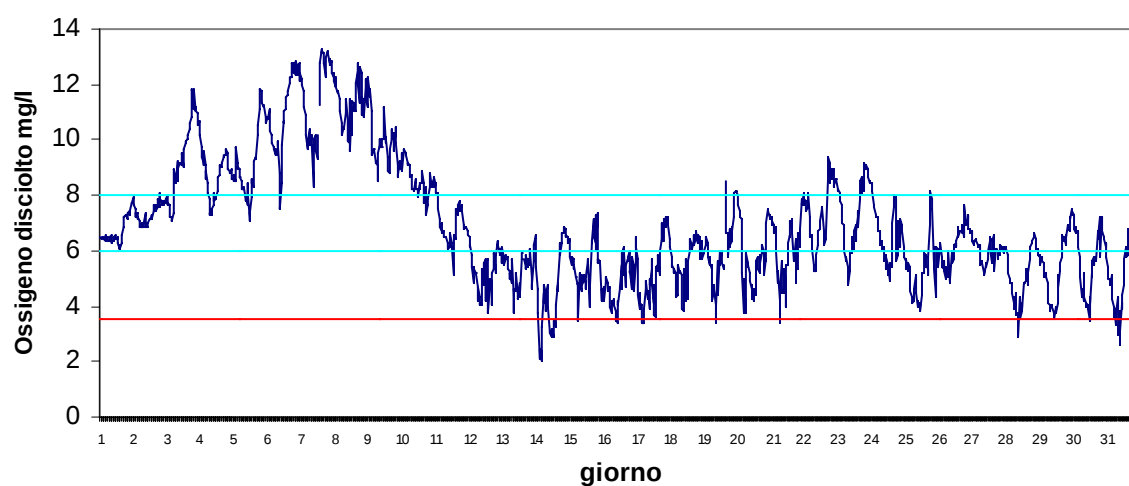
Stazione Scardovari interno Luglio 2017 - Ossigeno disciolto mg/l
