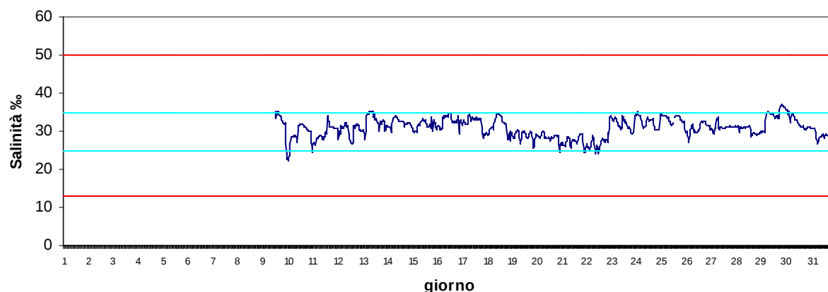
Stazione Scardovari mare Ottobre 2017 - Salinità ‰
