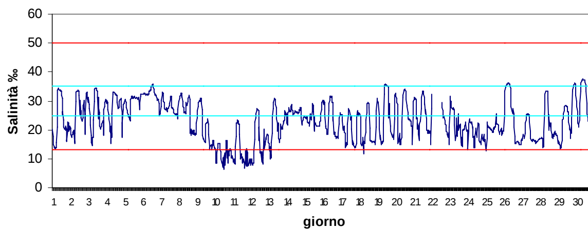
Stazione Basson Novembre 2017 - Salinità ‰
