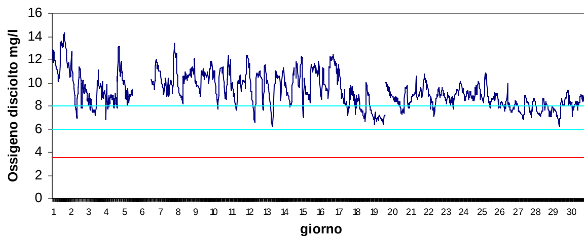
Stazione Scardovari mare Maggio 2017 - Ossigeno disciolto mg/l
