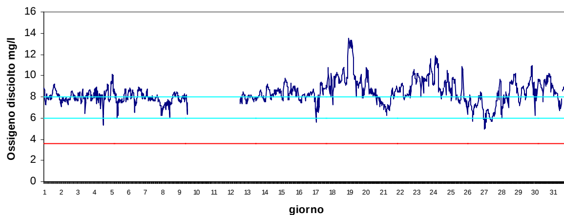
Stazione Scardovari mare Maggio 2017 - Ossigeno disciolto mg/l
