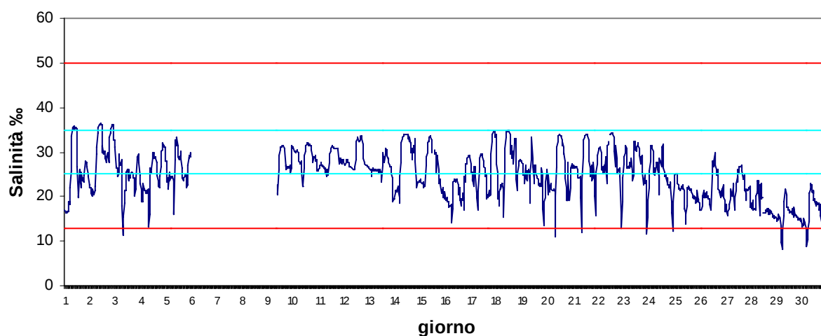
Stazione Canarin Settembre 2017 - Salinità ‰
