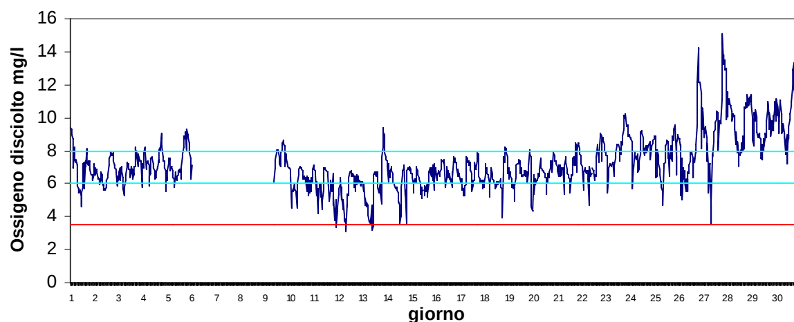
Stazione Canarin Settembre 2017 - Ossigeno disciolto mg/l
