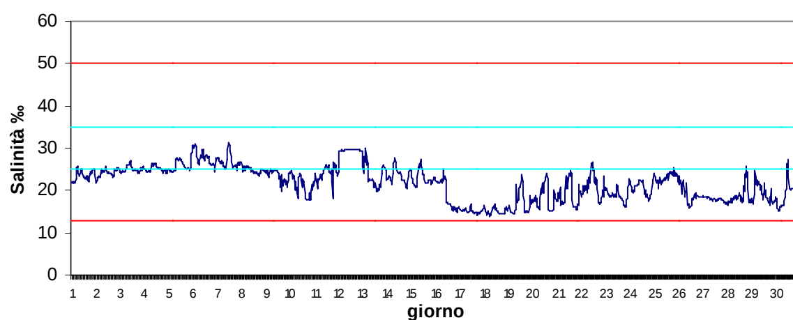
Stazione Vallona Novembre 2017 - Salinità ‰
