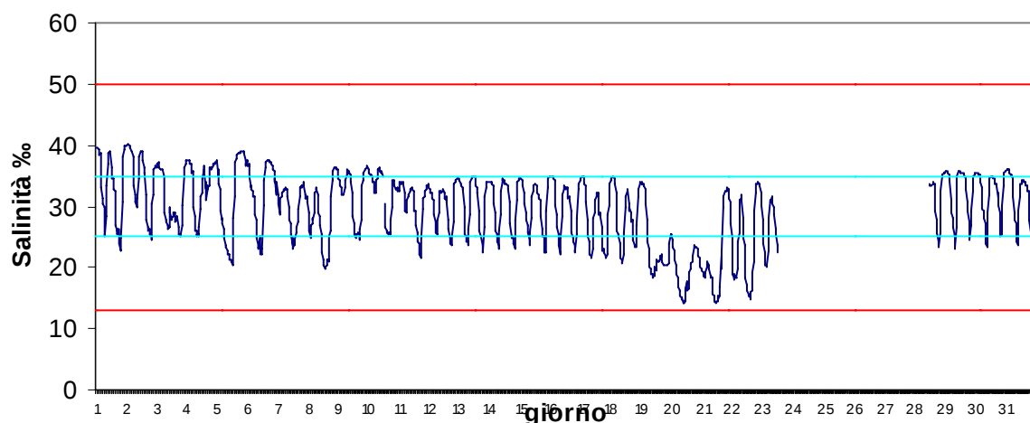
Stazione Marinetta Marzo 2017 - Salinità ‰
