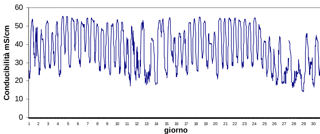
Stazione Marinetta Settembre 2017 - Conducibilità mS/cm
