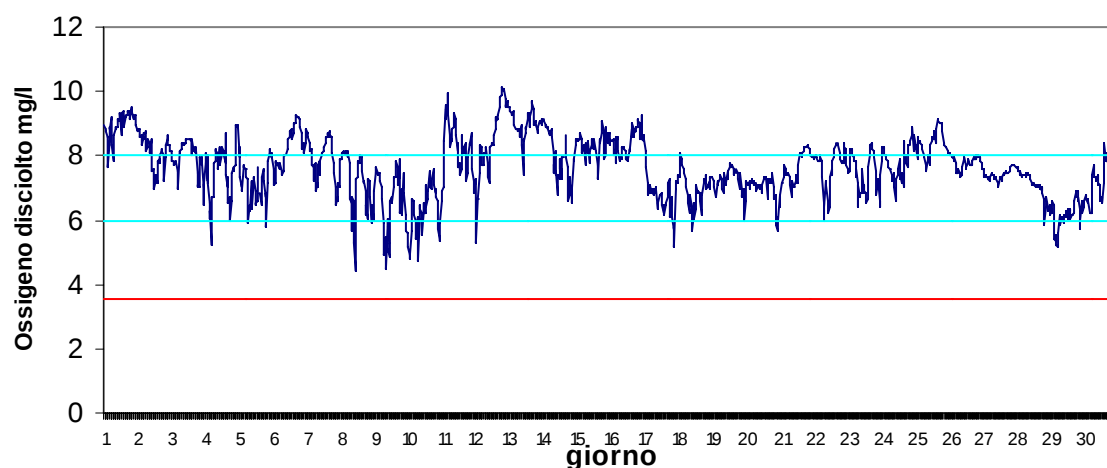
Stazione Scardovari interno Maggio 2017 - Ossigeno disciolto mg/l
