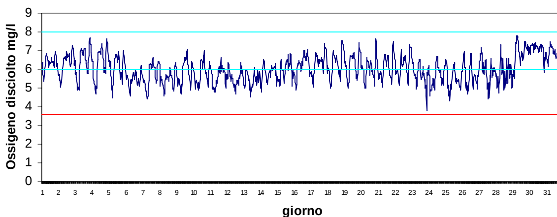
Stazione Marinetta Ottobre 2017 - Ossigeno disciolto mg/l
