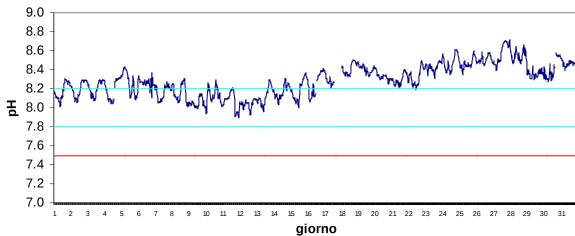
Stazione Scardovari interno Agosto 2017 - pH
