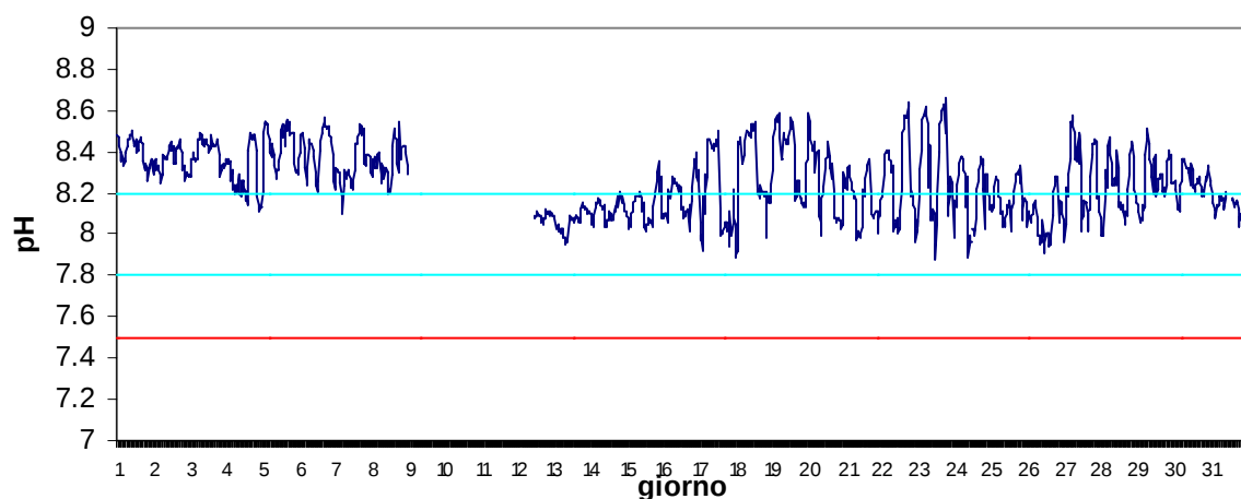
Stazione Basson Giugno 2017 - pH
