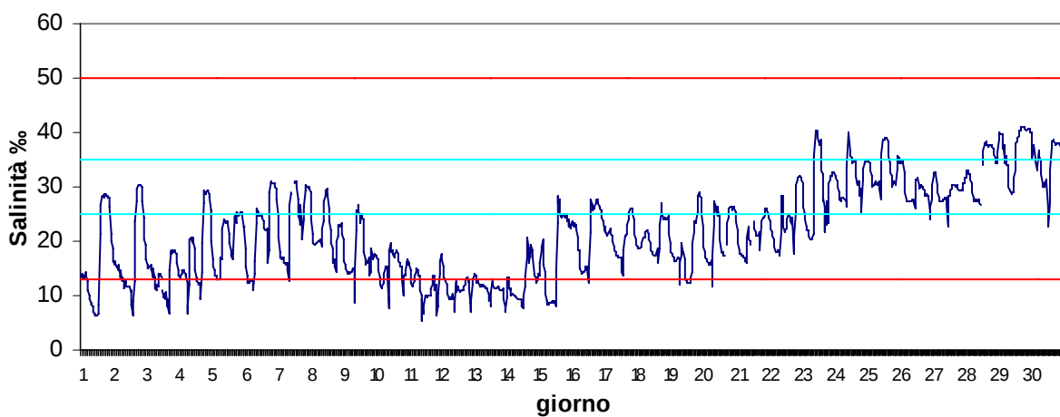
Stazione Basson Giugno 2017 - Salinità ‰
