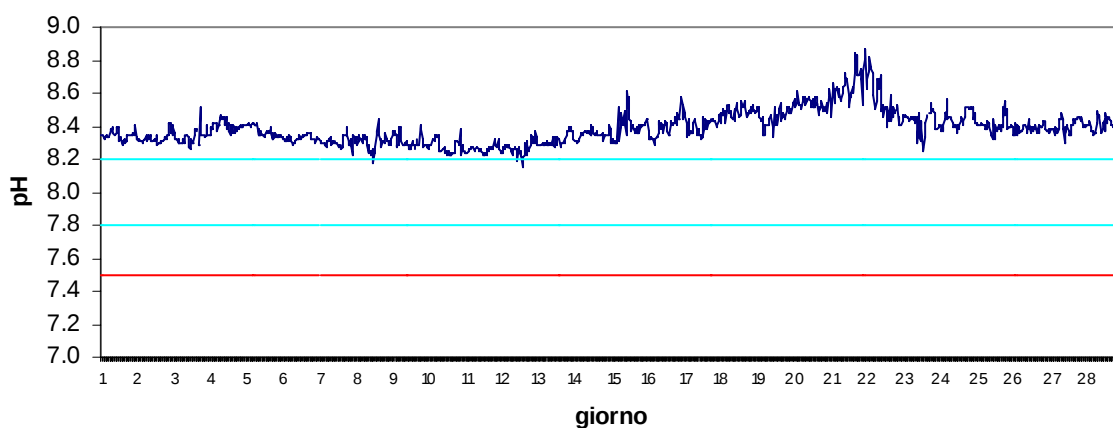
Stazione Barbamarco Marzo 2017 - pH
