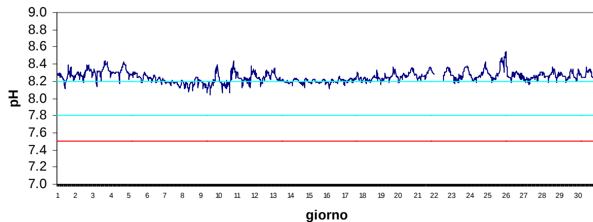
Stazione Canarin Novembre 2017 - pH
