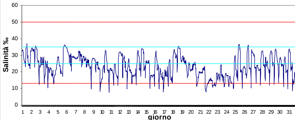
Stazione Canarin Marzo 2017 - Salinità ‰
