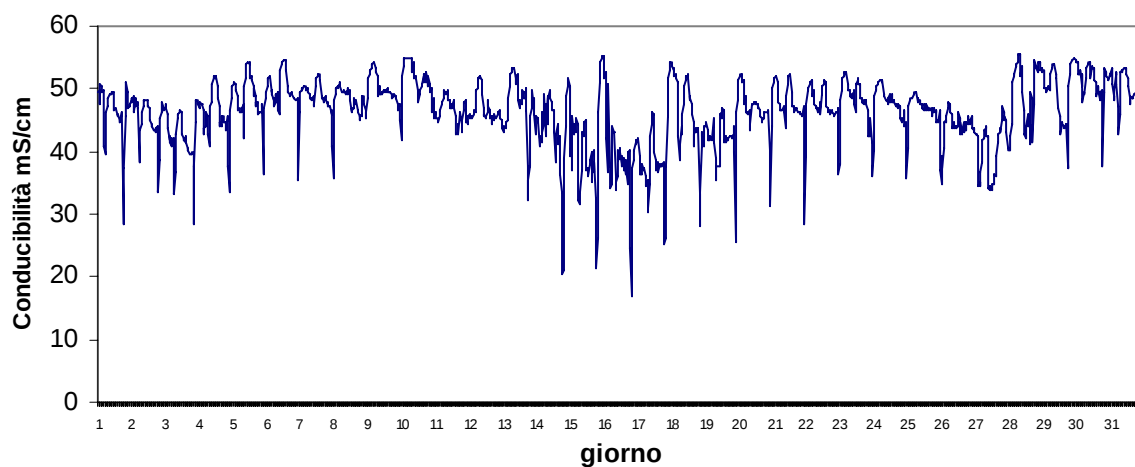
Stazione Canarin Dicembre 2017 - Conducibilità mS/cm
