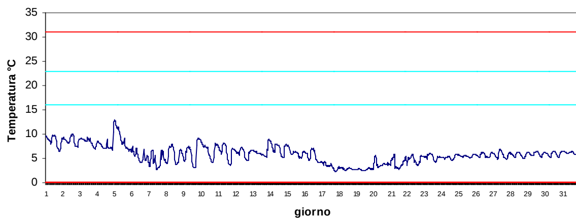
Stazione Scardovari mare Gennaio 2017 - Temperatura
