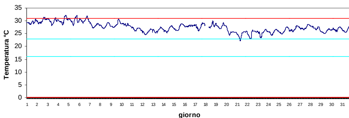
Stazione Barbamarco Agosto 2017 - Temperatura
