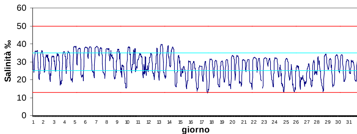
Stazione Marinetta Dicembre 2017 - Salinità ‰
