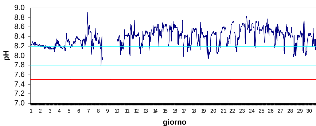
Stazione Barbamarco Aprile 2017 - pH
