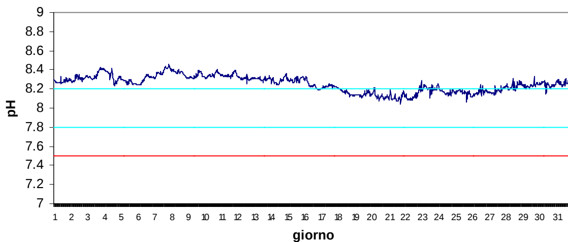
Stazione Scardovari interno Gennaio 2017 - pH
