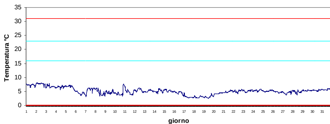
Stazione Barbamarco Gennaio 2017 - Temperatura
