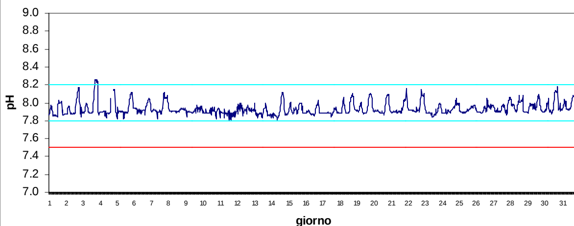
Stazione Scardovari mare Dicembre 2017 - pH
