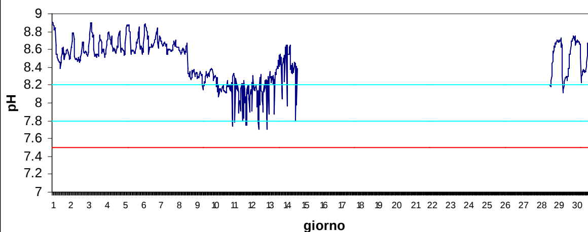
Stazione Basson Settembre 2017 - pH
