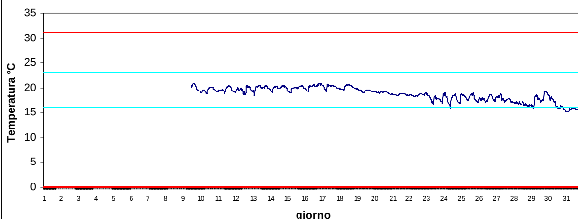
Stazione Scardovari mare Novembre 2017 - Temperatura
