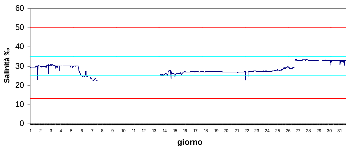
Stazione Scardovari interno Luglio 2017 - Salinità ‰
