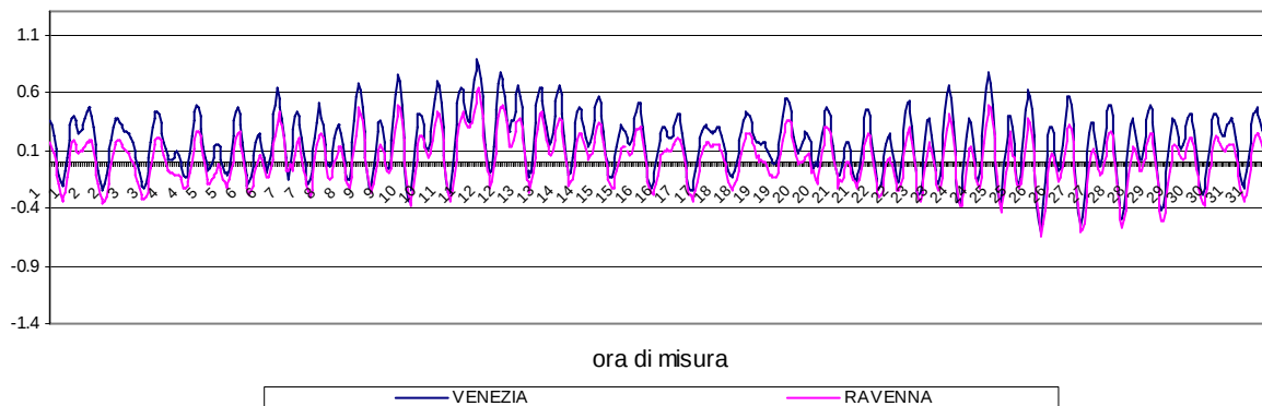
CONFRONTI CICLO di MAREA VENEZIA-RAVENNA MAGGIO 2017
