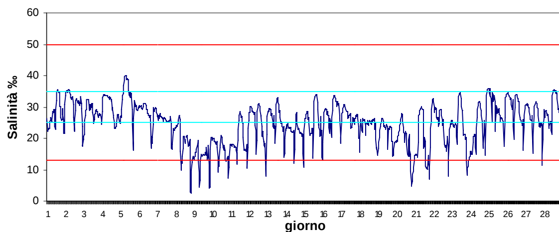
Stazione Canarin Febbraio 2017 - Salinità ‰
