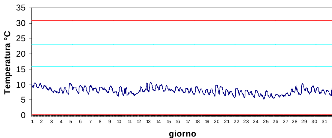
Stazione Marinetta Dicembre 2017 - Temperatura
