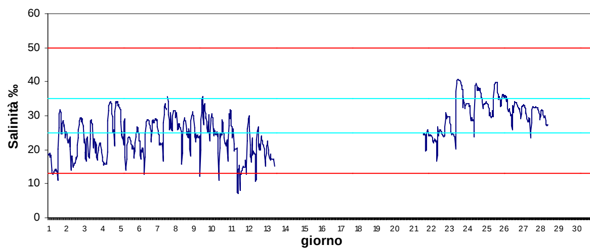
Stazione Canarin Giugno 2017 - Salinità ‰
