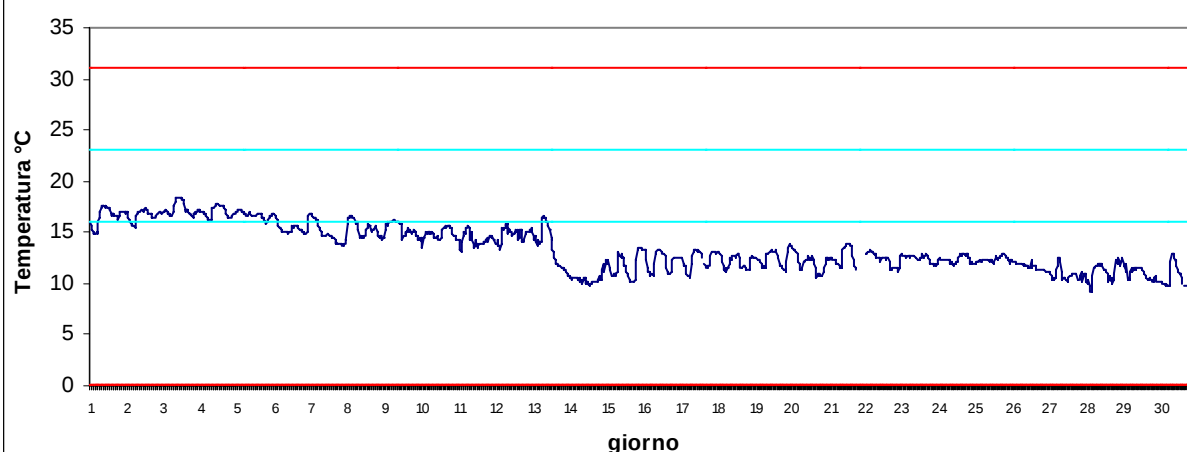
Stazione Scardovari mare Dicembre 2017 - Temperatura
