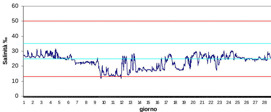
Stazione Vallona Febbraio 2017 - Salinità ‰
