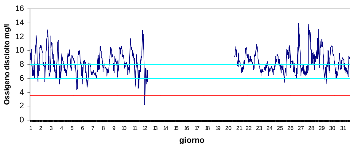
Stazione Vallona Ottobre 2017 - Ossigeno disciolto mg/l
