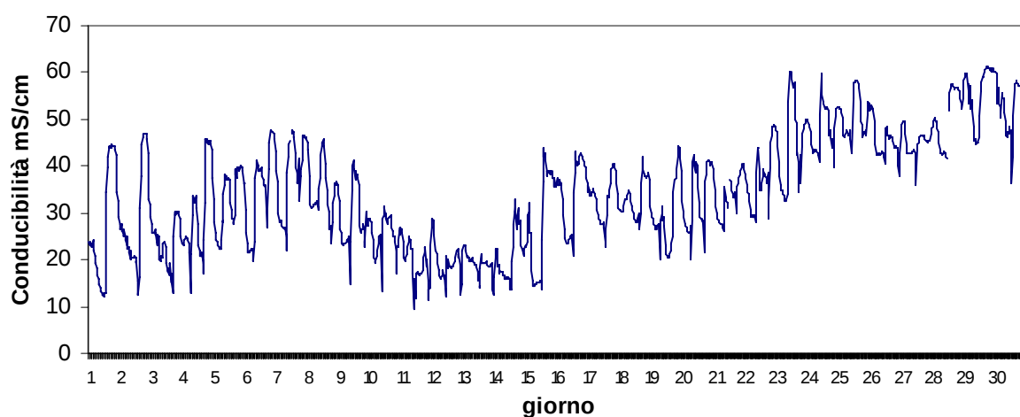
Stazione Basson Giugno 2017 - Conducibilità mS/cm
