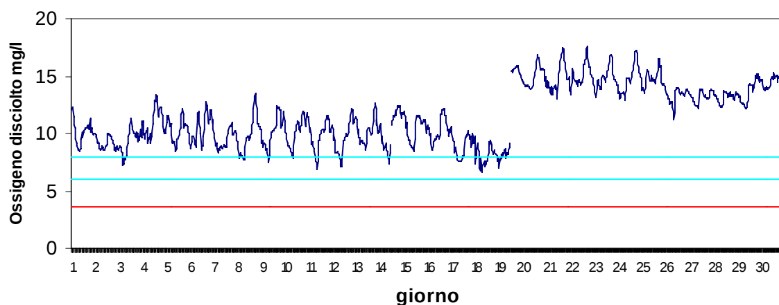
Stazione Basson Aprile 2017 - Ossigeno disciolto mg/l
