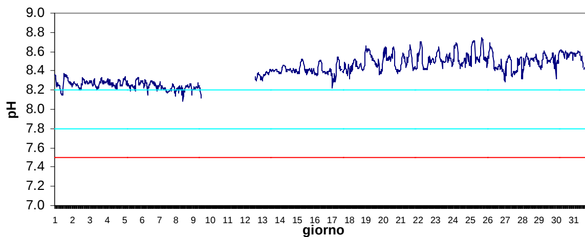
Stazione Scardovari mare Giugno 2017 - pH
