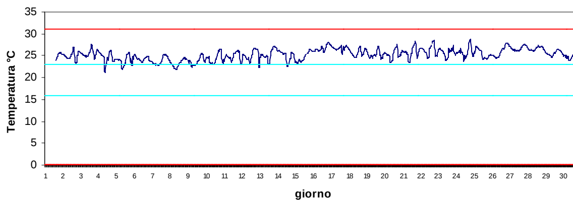
Stazione Barbamarco Giugno 2017 - Temperatura
