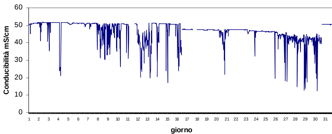
Stazione Scardovari interno Agosto 2017 - Conducibilità mS/cm
