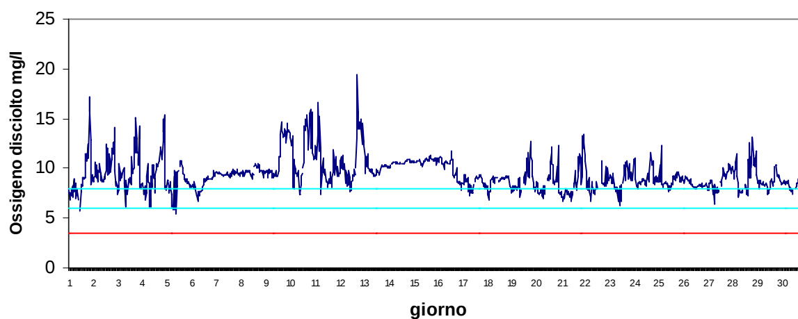
Stazione Barbamarco Novembre 2017 - Ossigeno disciolto mg/l
