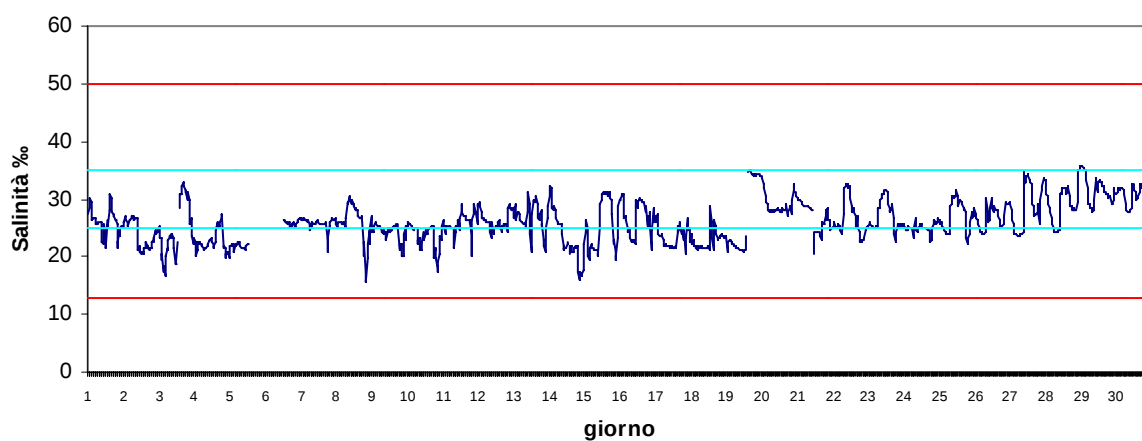
Stazione Scardovari mare Aprile 2017 - Salinità ‰
