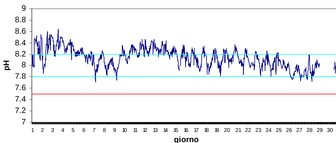
Stazione Vallona Giugno 2017 - pH
