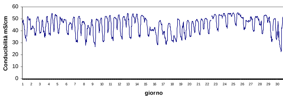
Stazione Marinetta Giugno 2017 - Conducibilità mS/cm
