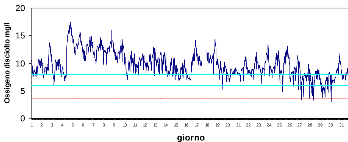
Stazione Canarin Agosto 2017 - Ossigeno disciolto mg/l
