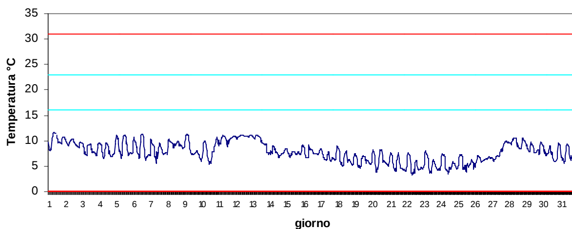
Stazione Basson Dicembre 2017 - Temperatura
