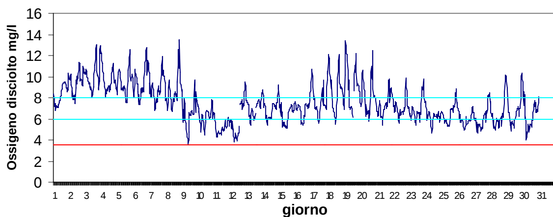
Stazione Basson Agosto 2017 - Ossigeno disciolto mg/l
