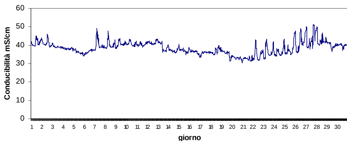
Stazione Vallona Aprile 2017 - Conducibilità mS/cm
