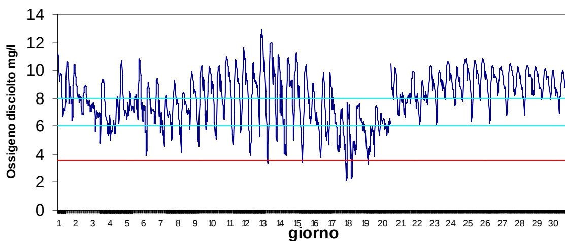
Stazione Marinetta Aprile 2017 - Ossigeno disciolto mg/l
