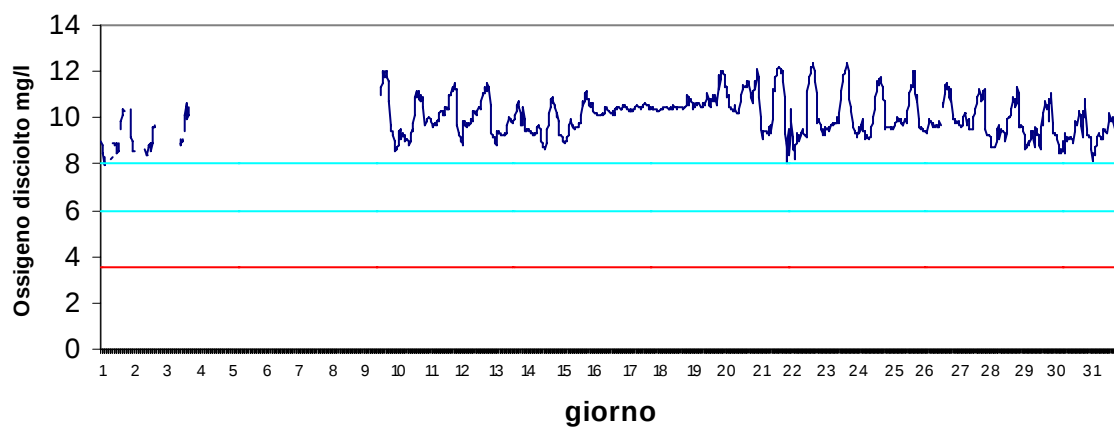
Stazione Marinetta Gennaio 2017 - Ossigeno disciolto mg/l
