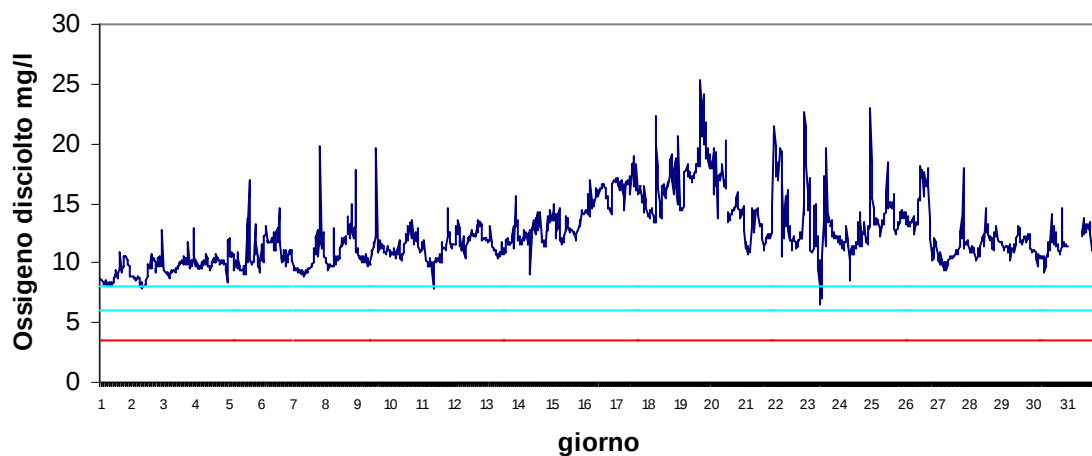
Stazione Barbamarco Marzo 2017 - Ossigeno disciolto mg/l
