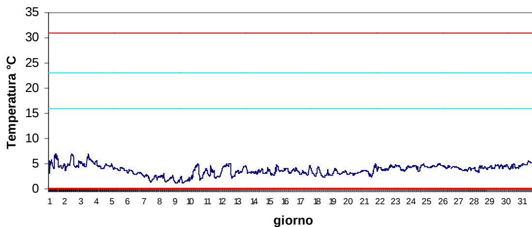
Stazione Vallona Gennaio 2017 - Temperatura
