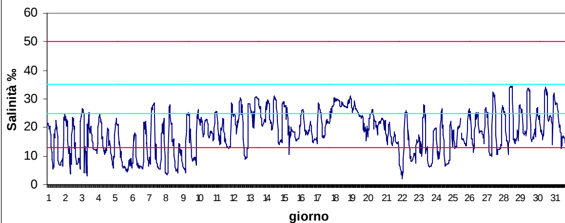
Stazione Basson Gennaio 2017 - Salinità ‰
