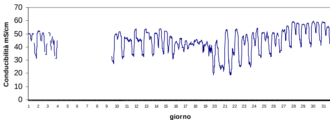
Stazione Marinetta Gennaio 2017 - Conducibilità mS/cm
