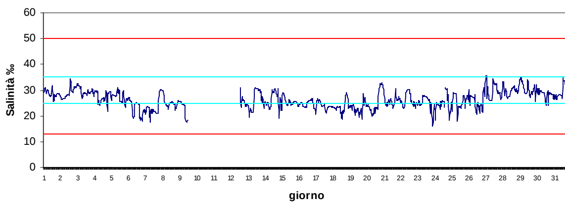
Stazione Scardovari mare Maggio 2017 - Salinità ‰
