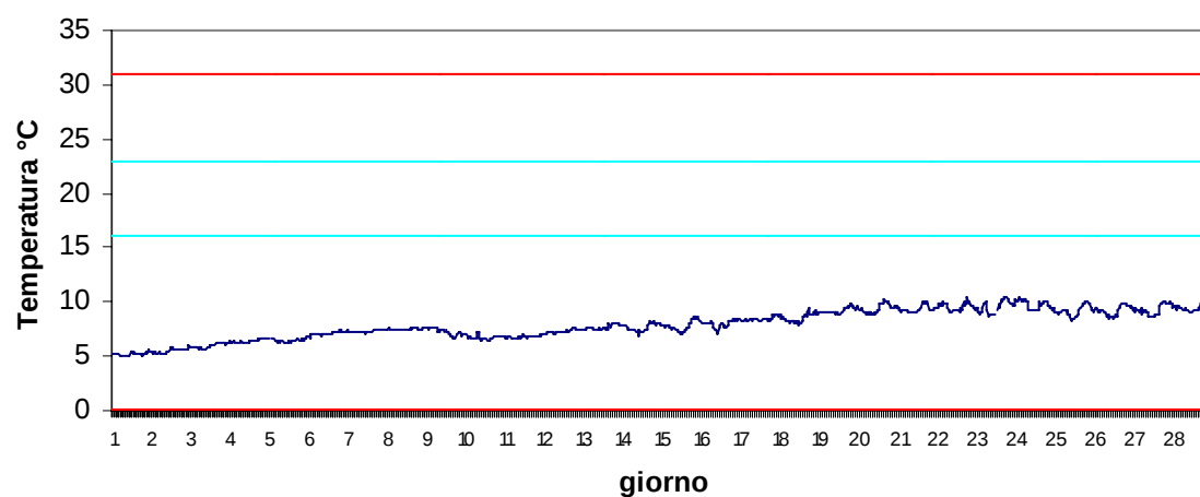
Stazione Vallona Marzo 2017 - Temperatura
