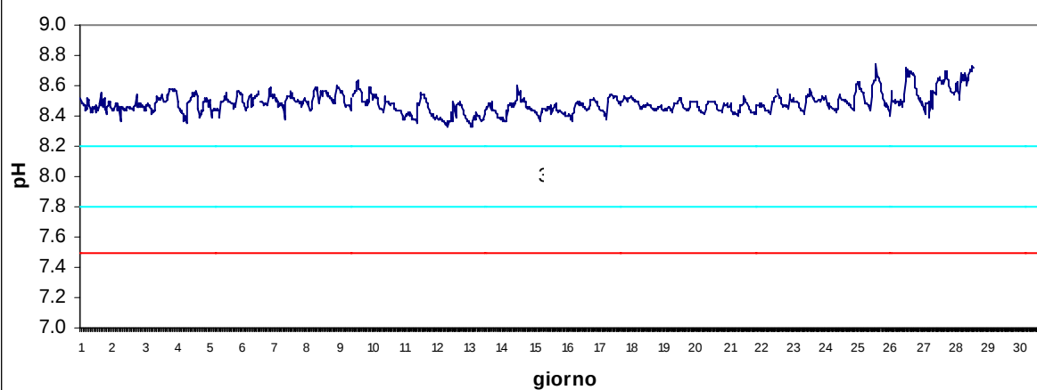
Stazione Scardovari mare Settembre 2017 - pH
