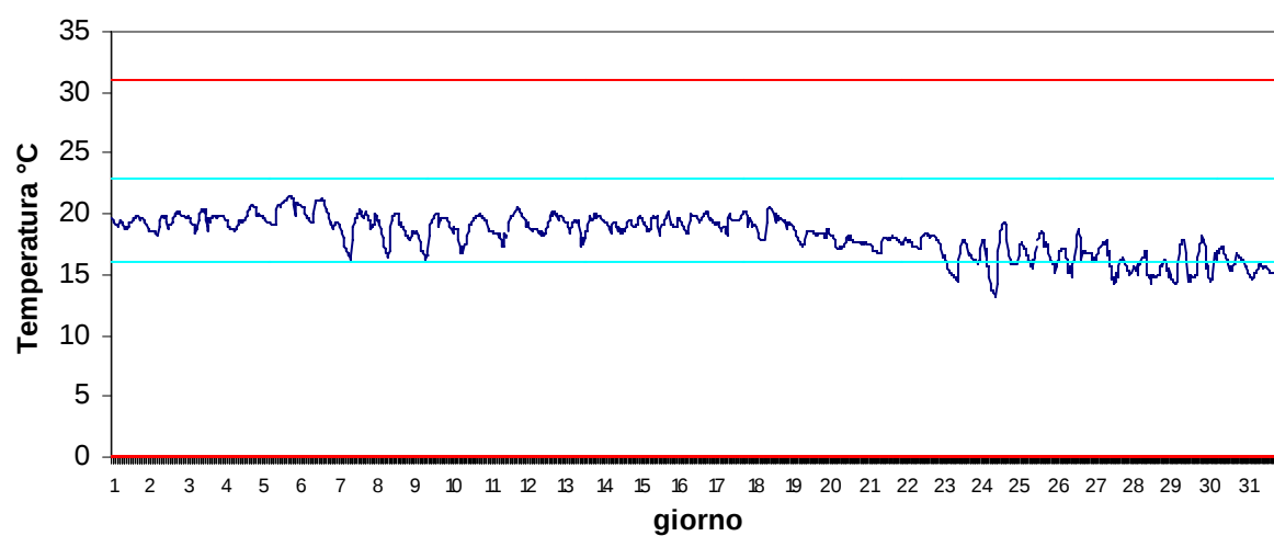
Stazione Basson Ottobre 2017 - Temperatura
