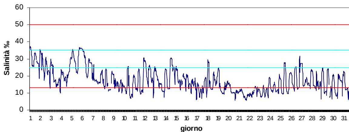
Stazione Basson Marzo 2017 - Salinità ‰
