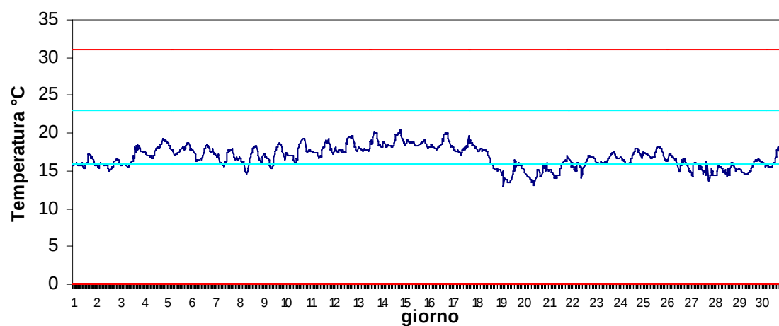
Stazione Vallona Maggio 2017 - Temperatura
