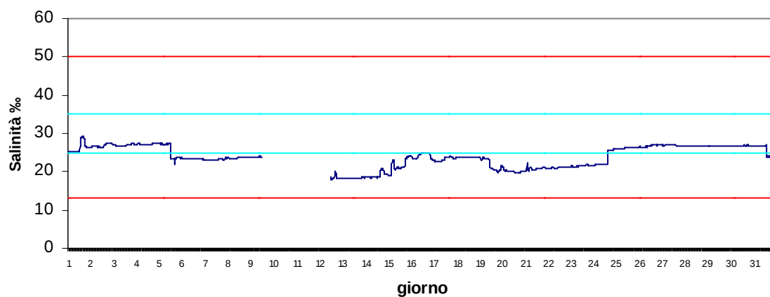
Stazione Scardovari interno Maggio 2017 - Salinità ‰
