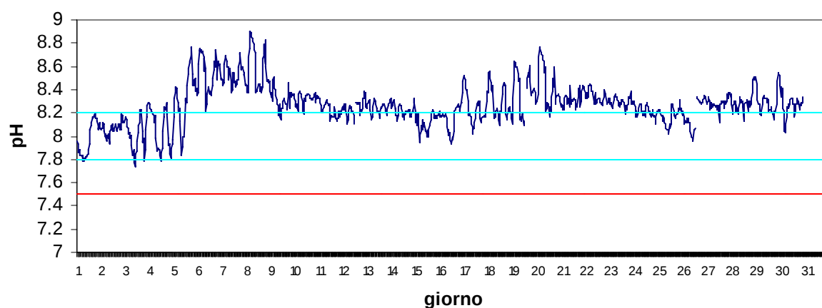
Stazione Basson Luglio 2017 - pH
