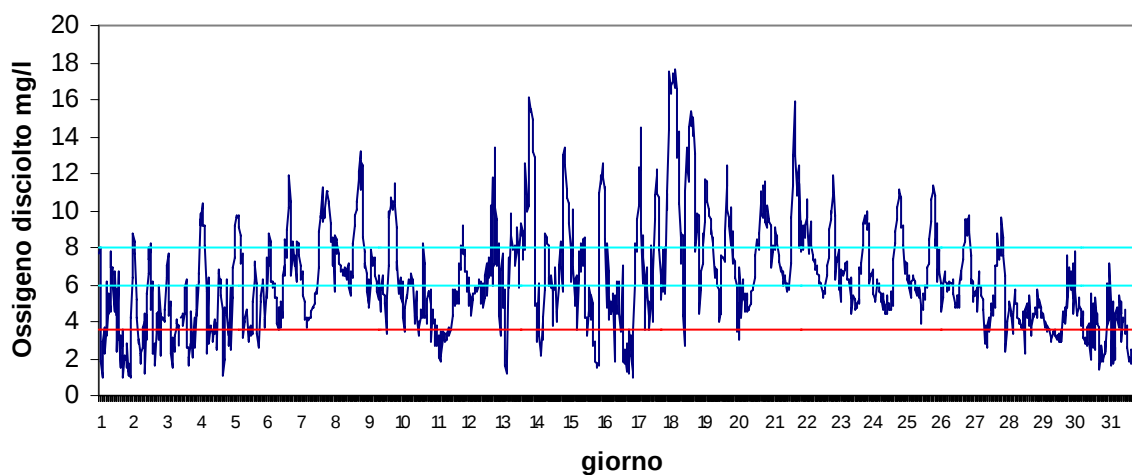
Stazione Vallona Agosto 2017 - Ossigeno disciolto mg/l
