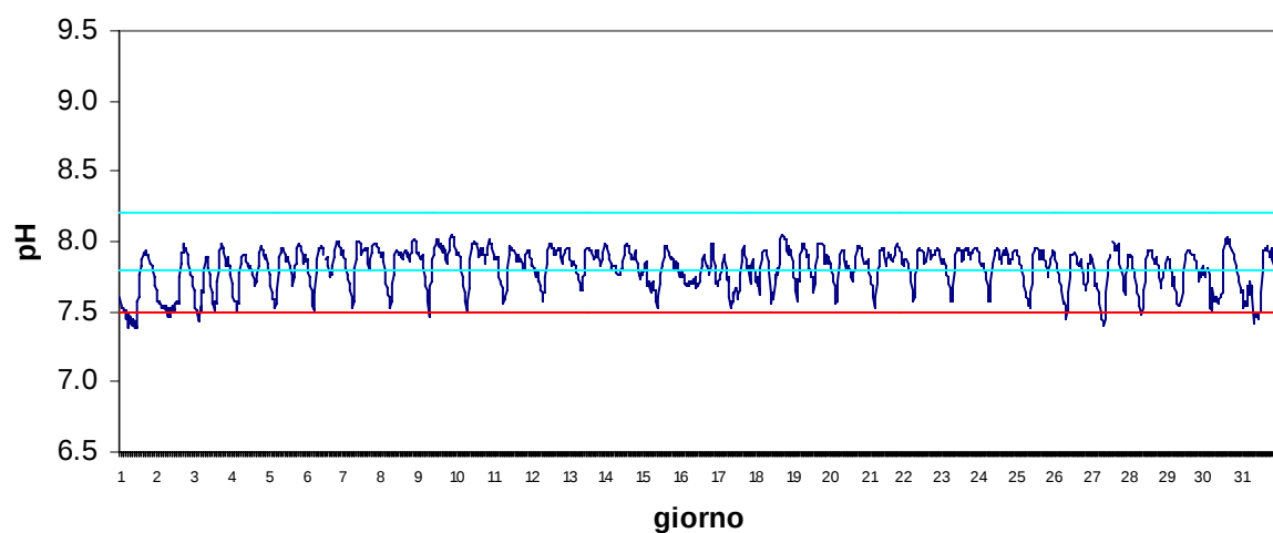
Stazione Marinetta Luglio 2017 - pH
