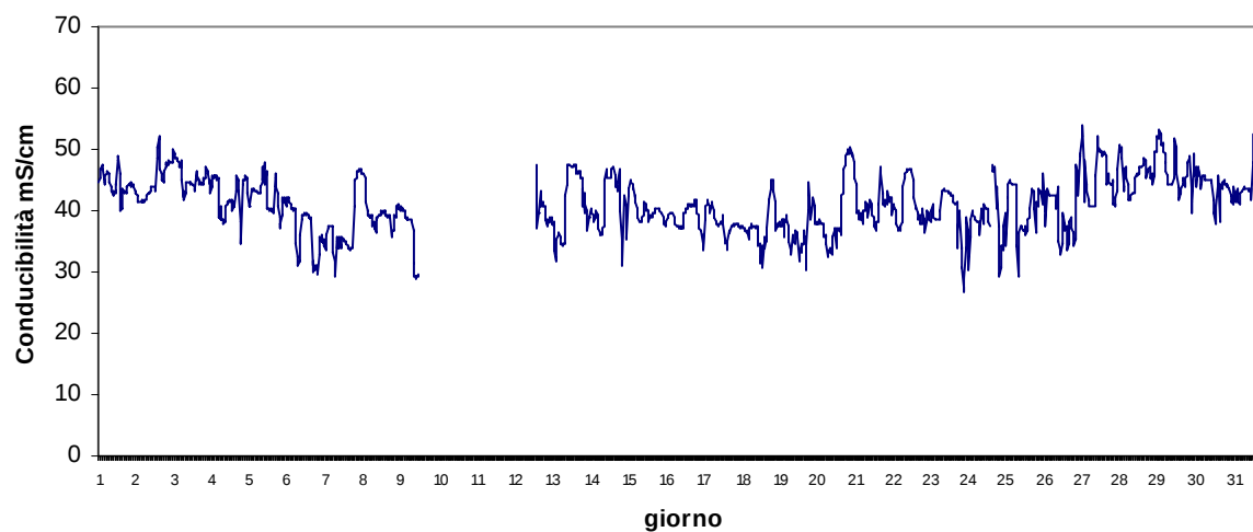
Stazione Scardovari mare Maggio 2017 - Conducibilità mS/cm
