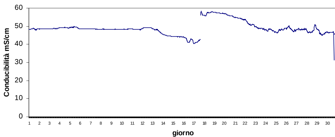
Stazione Scardovari interno Novembre 2017 - Conducibilità mS/cm
