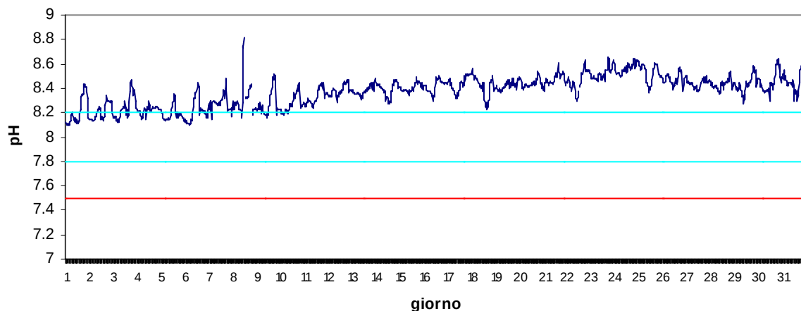
Stazione Basson Marzo 2017 - pH
