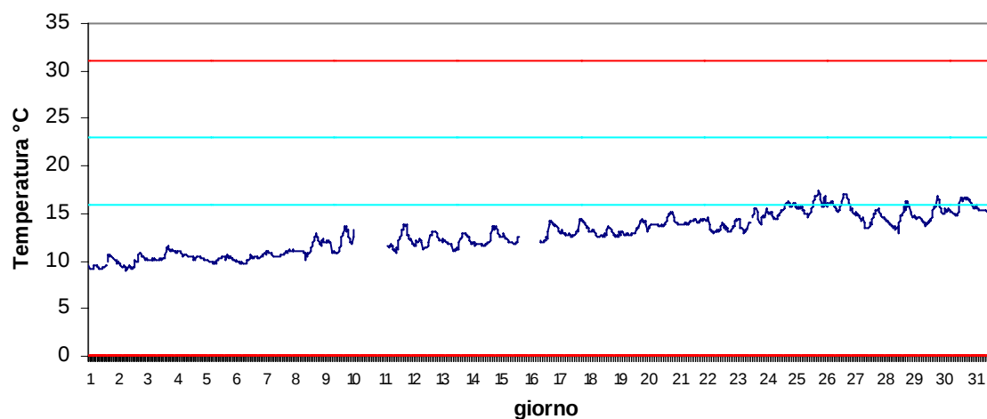
Stazione Vallona Marzo 2017 - Temperatura
