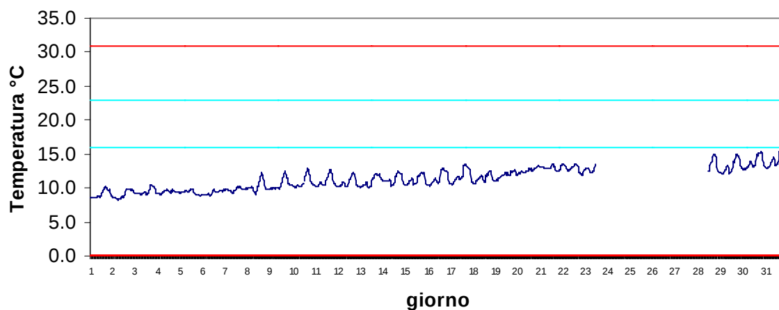
Stazione Marinetta Marzo 2017 - Temperatura
