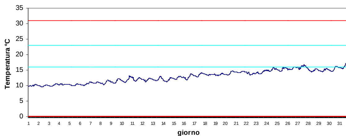
Stazione Scardovari interno Marzo 2017 - Temperatura
