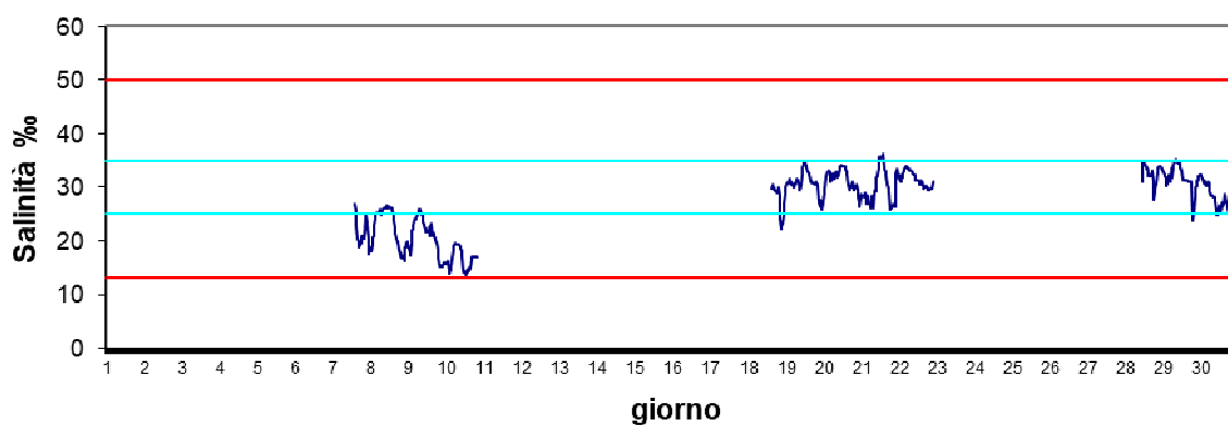
Stazione Canarin Dicembre 2024 - Salinità ‰
