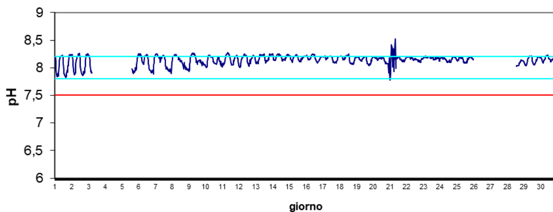
Stazione Marinetta Novembre 2024 - pH
