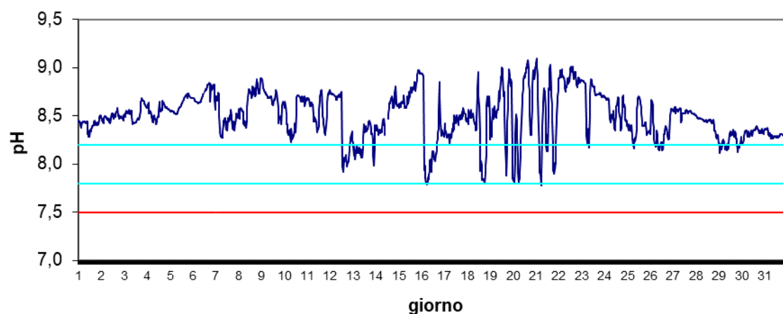
Stazione Scardovari interno Marzo 2024 - pH
