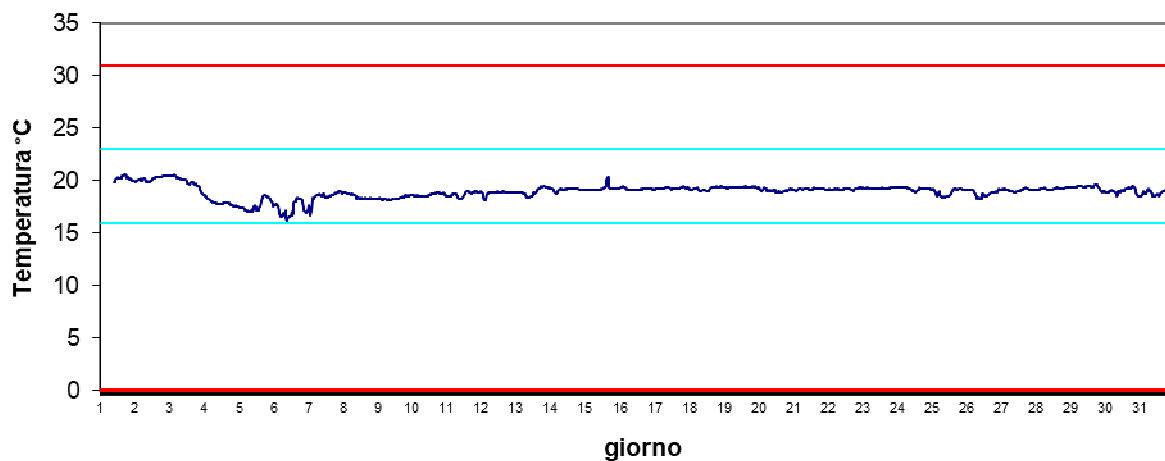
Stazione Scardovari interno Ottobre 2024 - Temperatura
