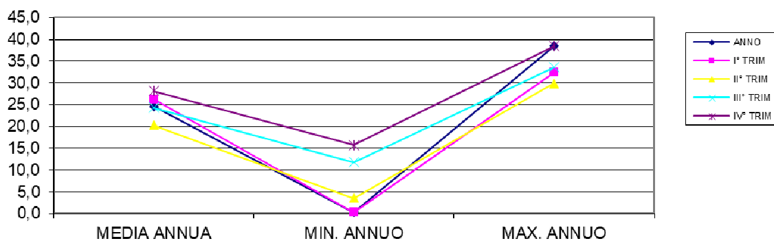
LAGUNA SCARDOVARI INTERNO - SALINITA'
