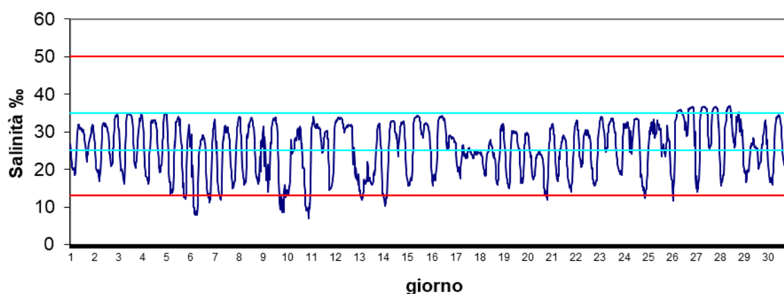
Stazione Marinetta Ottobre 2024 - Salinità ‰
