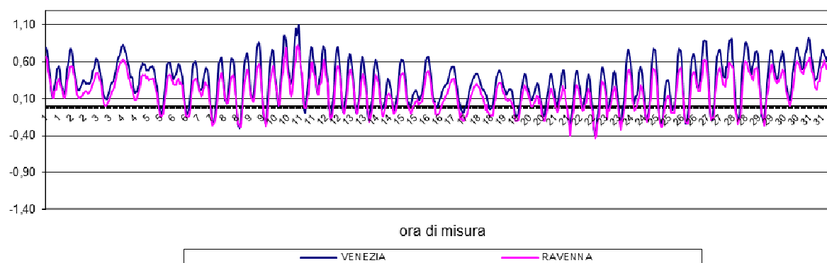
CONFRONTI CICLO di MAREA VENEZIA-RAVENNA MARZO 2024
