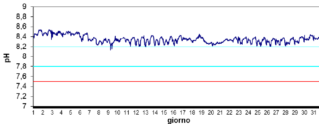
Stazione Vallona Febbraio 2024 - pH
