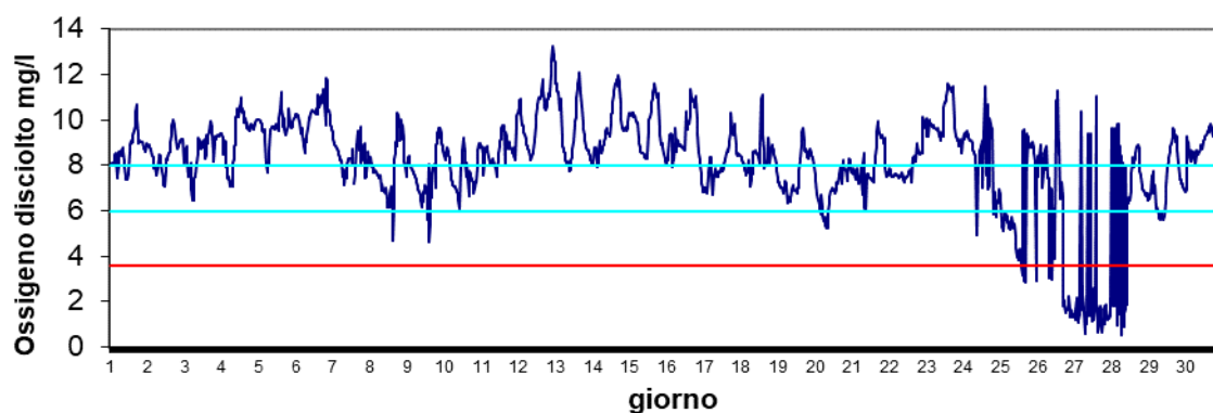
Stazione Canarin Dicembre 2024 - Ossigeno disciolto mg/l
