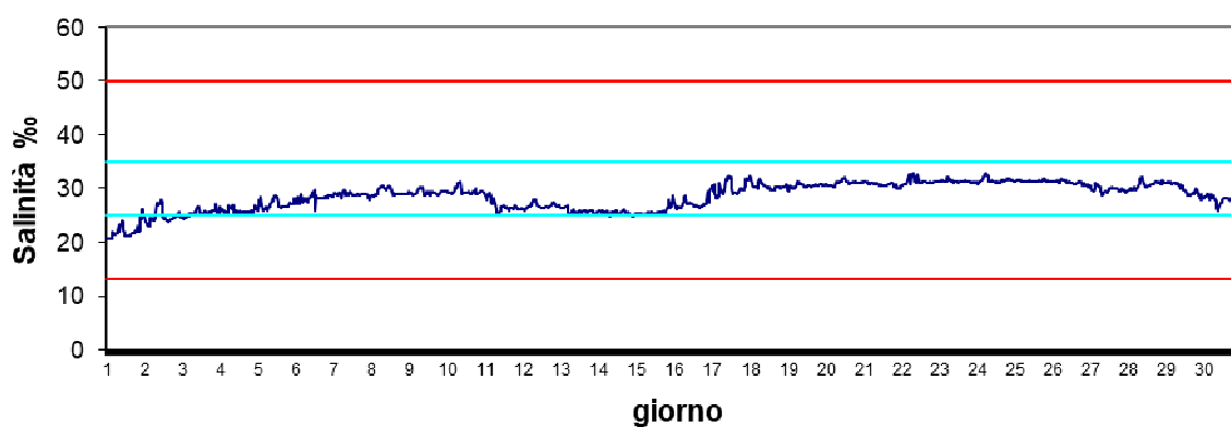
Stazione Caleri Dicembre 2024 - Salinità ‰
