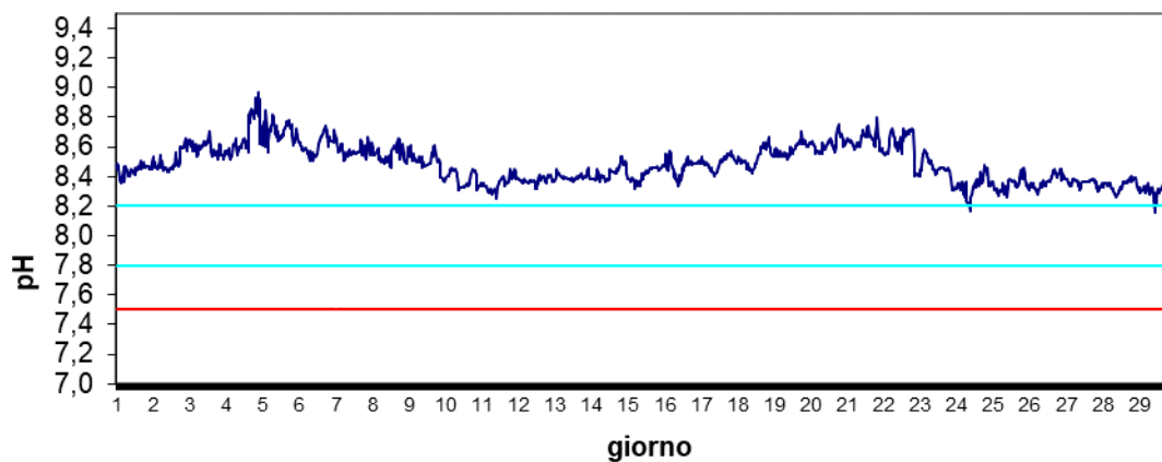
Stazione Barbamarco Febbraio 2024 - pH
