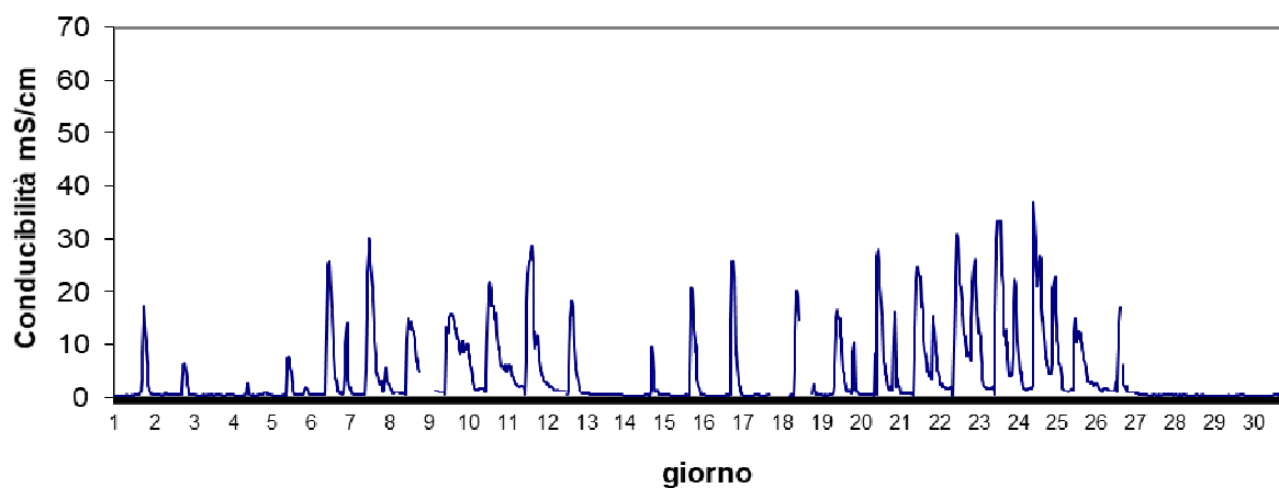
Stazione Basson Giugno 2024 - Conducibilità mS/cm
