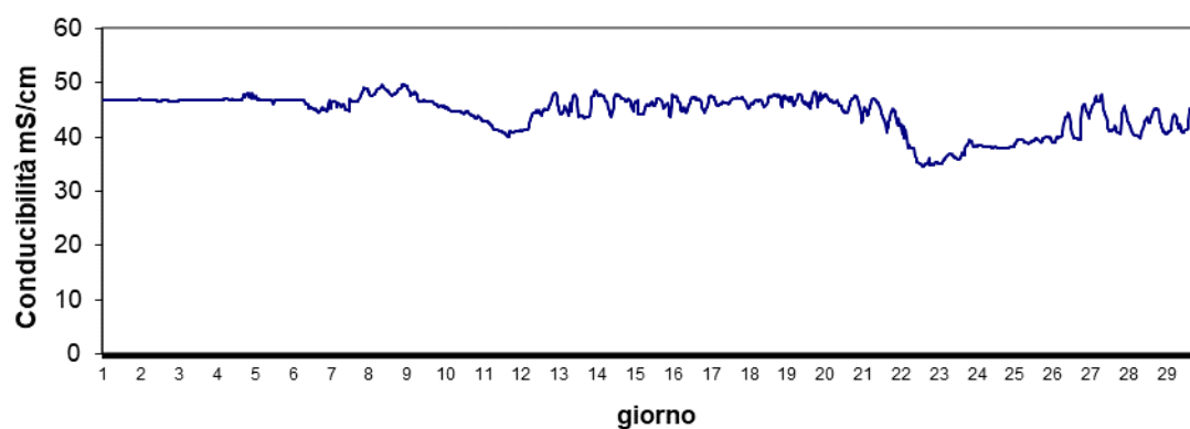
Stazione Scardovari interno Marzo 2024 - Conducibilità mS/cm
