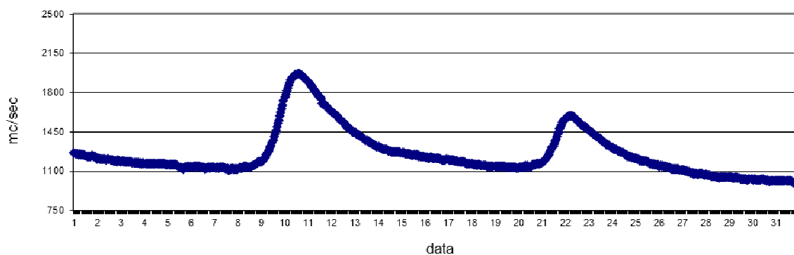
PORTATA PONTELAGOSCURO mc/sec DICEMBRE 2024
