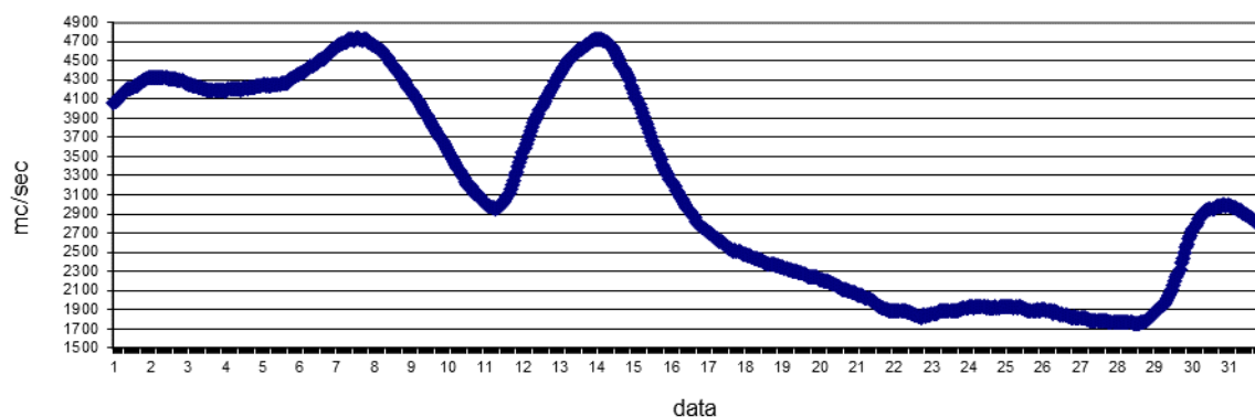
PORTATA PONTELAGOSCURO mc/sec MARZO 2024
