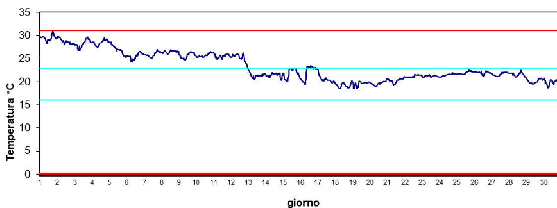
Stazione Barbamarco Settembre 2024 - Temperatura
