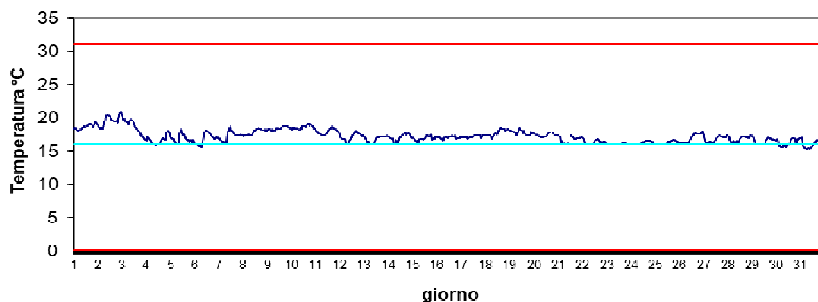
Stazione Basson Novembre 2024 - Temperatura
