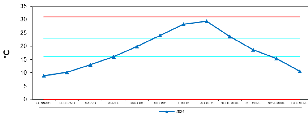
Scardovari S. Giulia - confronto Temperatura MEDIA 2024
