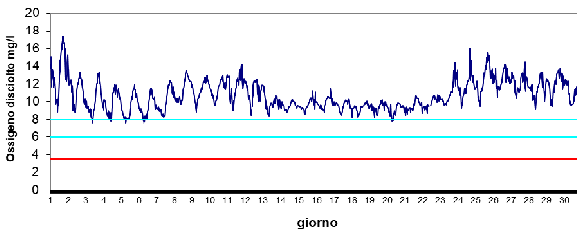
Stazione Vallona Novembre 2024 - Ossigeno disciolto mg/l
