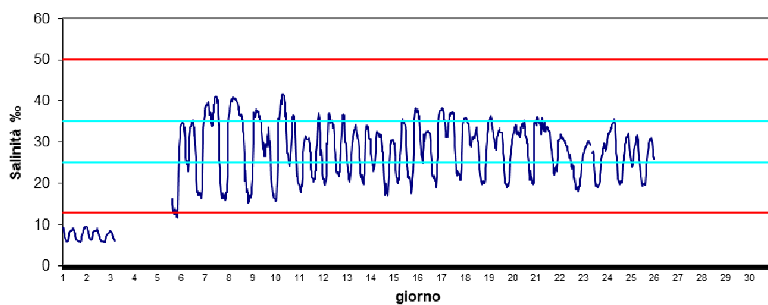
Stazione Marinetta Novembre 2024 - Salinità ‰
