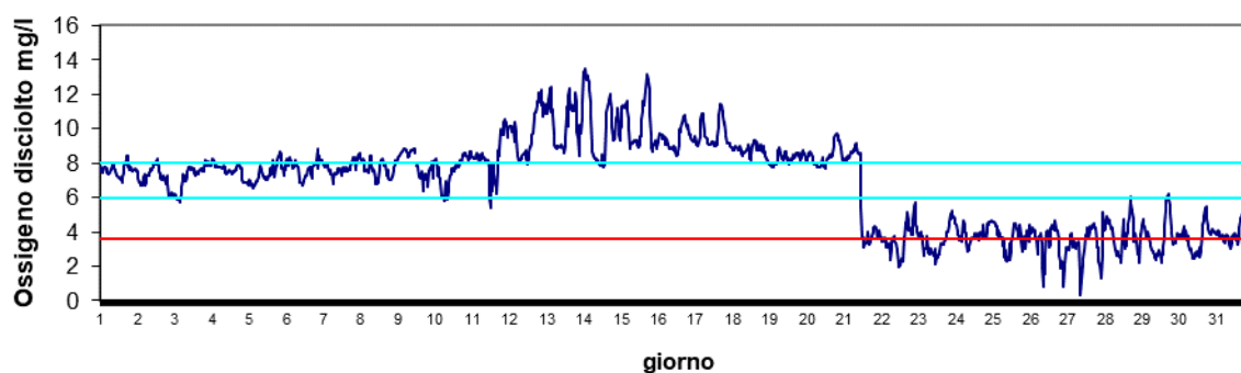
Stazione Scardovari mare Novembre 2024 - Ossigeno disciolto mg/l
