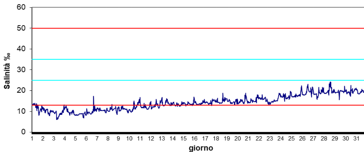
Stazione Vallona Marzo 2024 - Salinità ‰
