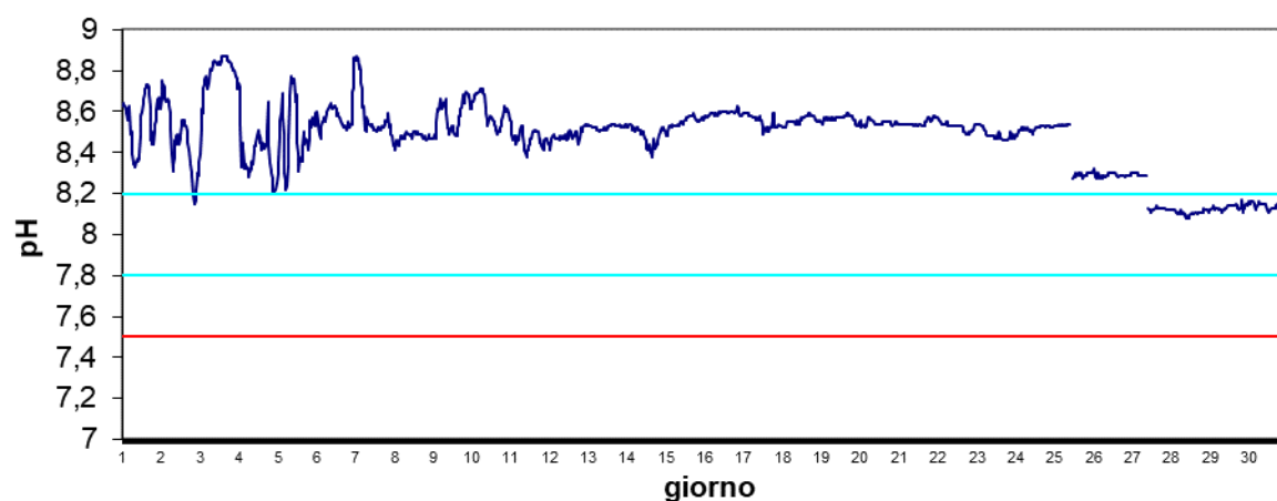
Stazione Scardovari interno Dicembre 2024 - pH
