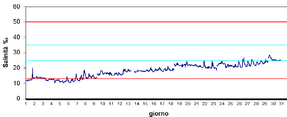
Stazione Vallona Luglio 2024 - Salinità ‰
