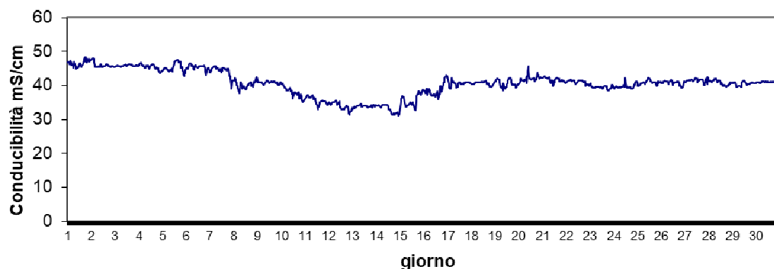
Stazione Caleri Maggio 2024 - Conducibilità mS/cm
