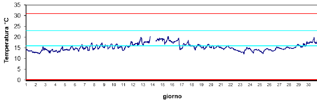
Stazione Scardovari mare Maggio 2024 - Temperatura
