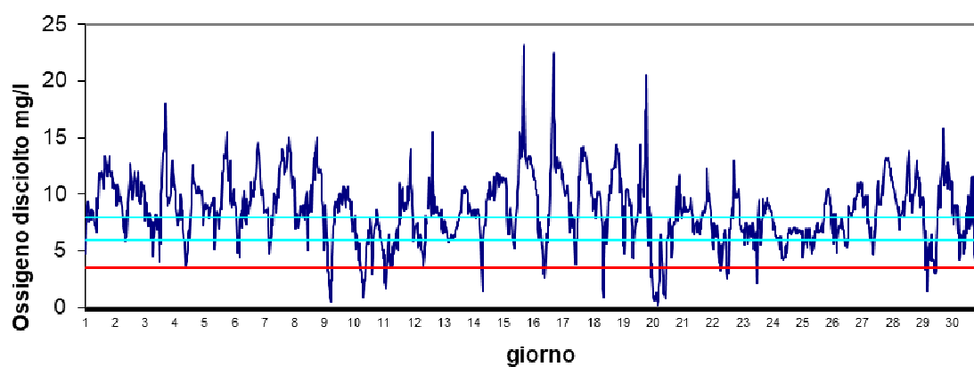
Stazione Barbamarco Giugno 2024 - Ossigeno disciolto mg/l
