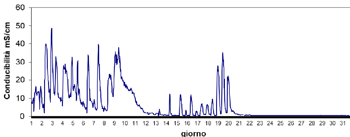
Stazione Basson Novembre 2024 - Conducibilità mS/cm
