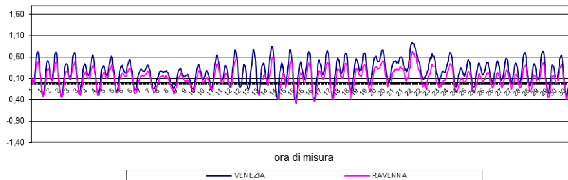
CONFRONTI CICLO di MAREA VENEZIA-RAVENNA NOVEMBRE 2024
