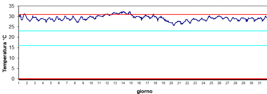
Stazione Barbamarco Agosto 2024 - Temperatura
