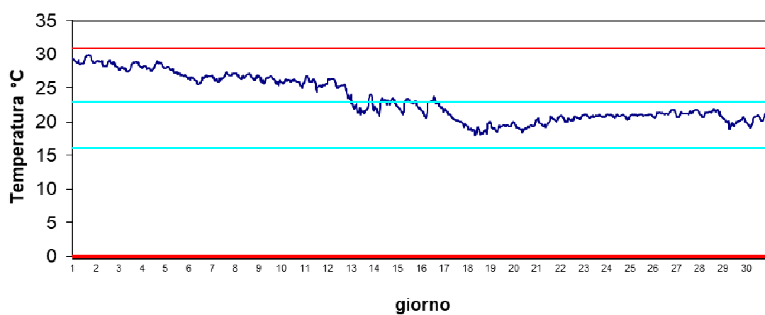
Stazione Marinetta Ottobre 2024 - Temperatura
