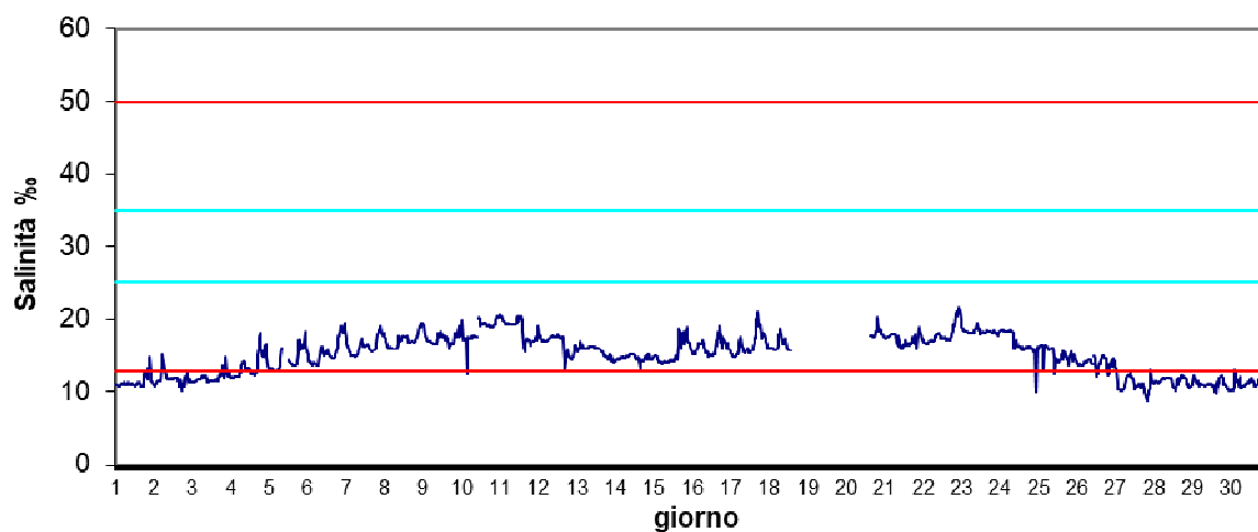
Stazione Vallona Giugno 2024 - Salinità ‰
