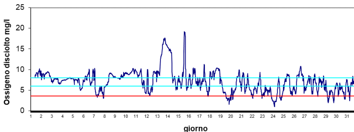
Stazione Scardovari interno Novembre 2024 - Ossigeno disciolto mg/l
