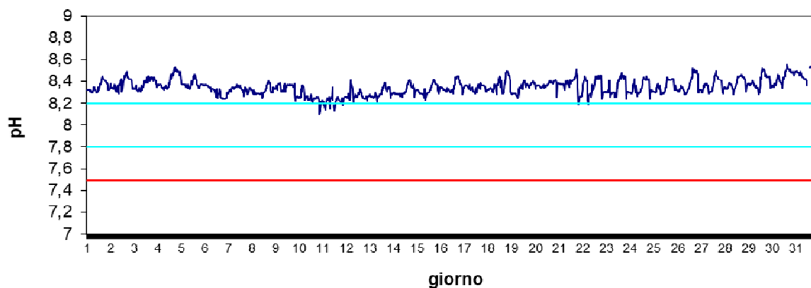
Stazione Basson Febbraio 2024 - pH
