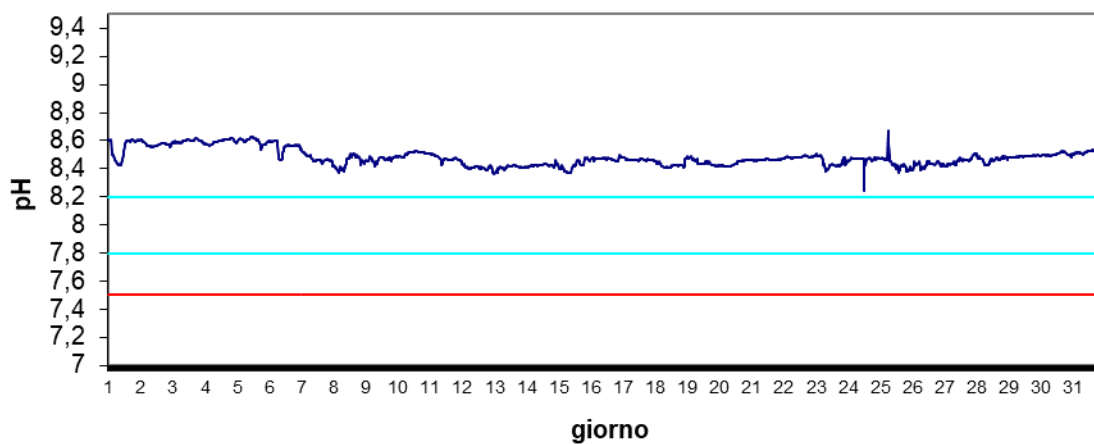
Stazione Scardovari interno Gennaio 2024 - pH
