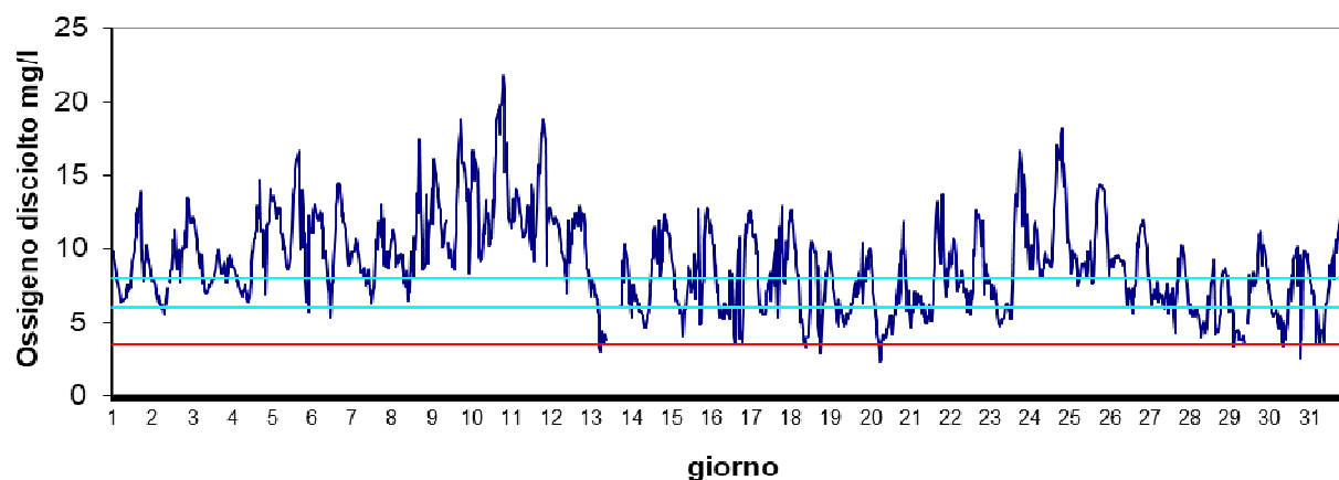
Stazione Vallona Agosto 2024 - Ossigeno disciolto mg/l
