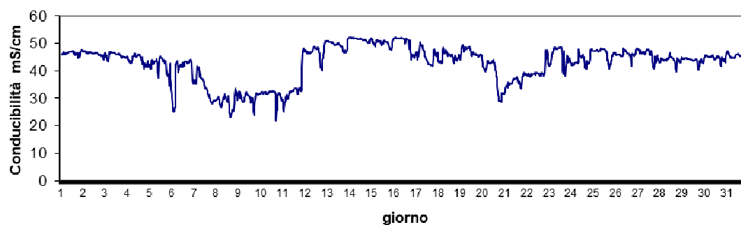
Stazione Barbamarco Febbraio 2024 - Conducibilità mS/cm
