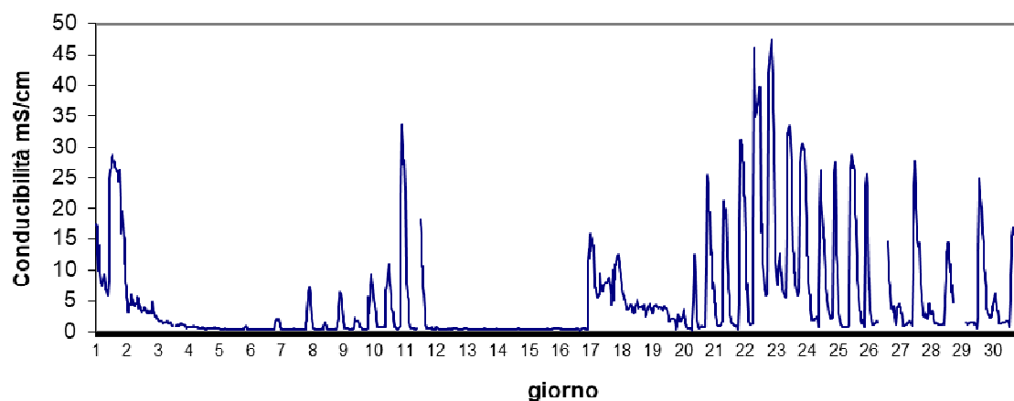
Stazione Basson Maggio 2024 - Conducibilità mS/cm
