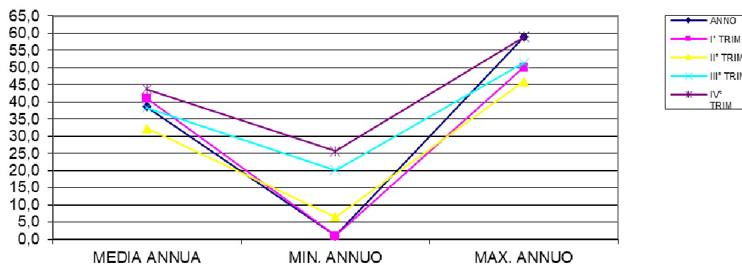
LAGUNA SCARDOVARI INTERNO - CONDUCIBILITA'
