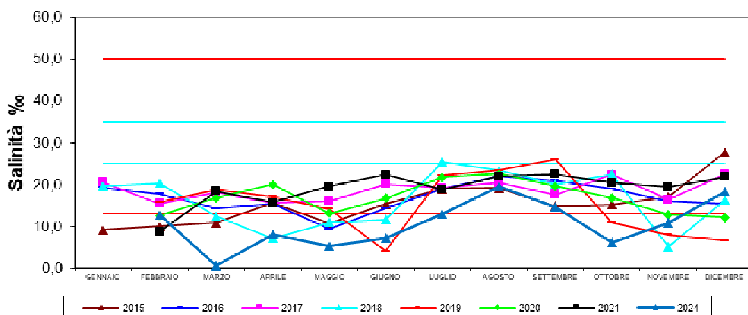
Scardovari mare - confronto Salinità MINIMA 2015 - 2016 - 2017 - 2018 - 2019- 2020 - 2021 - 2024
