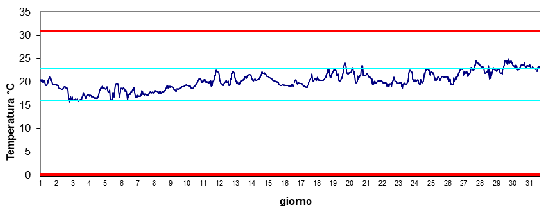
Stazione Barbamarco Maggio 2024 - Temperatura
