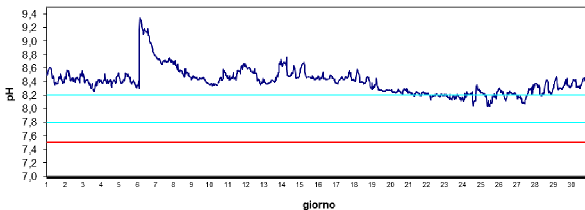
Stazione Scardovari mare Settembre 2024 - pH
