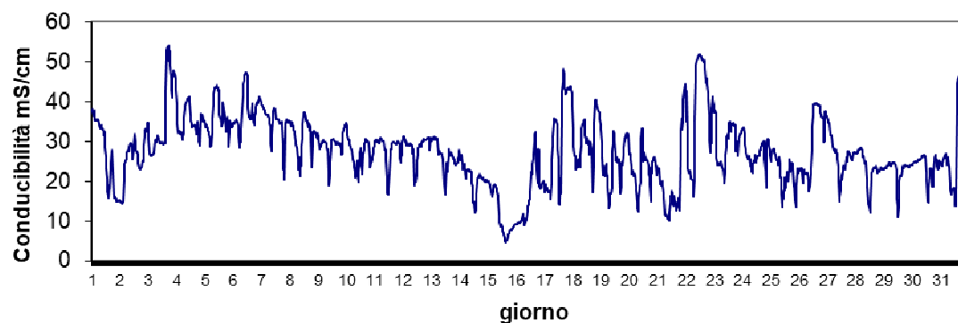
Stazione Scardovari S.Giulia Giugno 2024 - Conducibilità mS/cm
