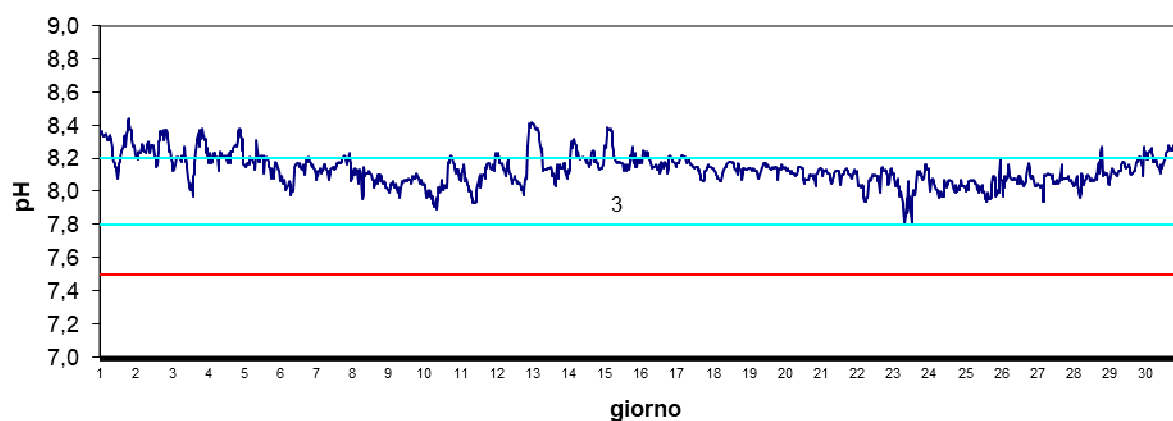
Stazione Scardovari S.Giulia Settembre 2024 - pH
