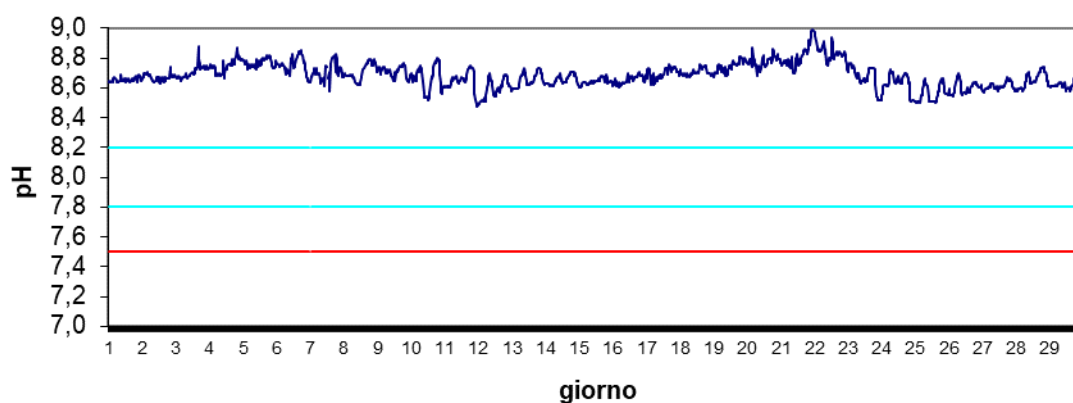
Stazione Scardovari mare Marzo 2024 - pH
