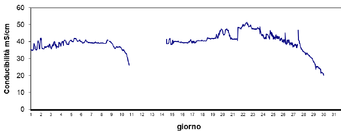
Stazione Scardovari interno Agosto 2024 - Conducibilità mS/cm
