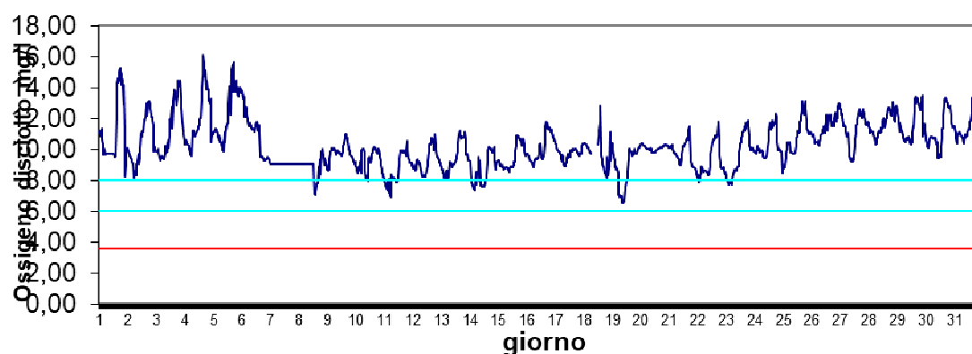
Stazione Scardovari S.Giulia Febbraio 2024 - Ossigeno disciolto mg/l
