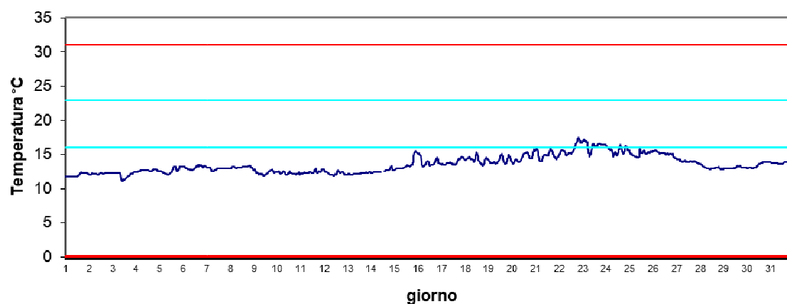
Stazione Scardovari interno Aprile 2024 - Temperatura
