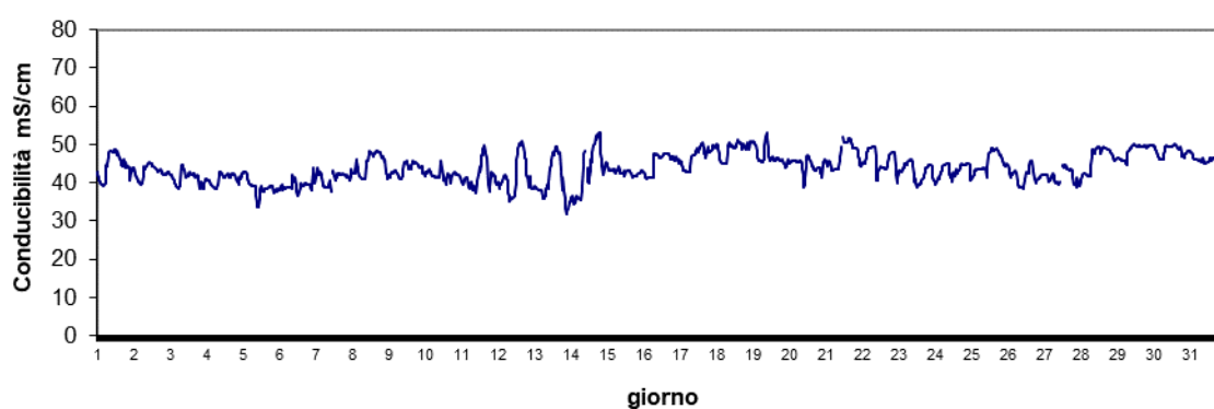
Stazione Scardovari mare Settembre 2024 - Conducibilità mS/cm
