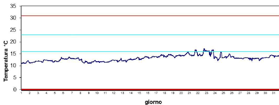
Stazione Barbamarco Marzo 2024 - Temperatura
