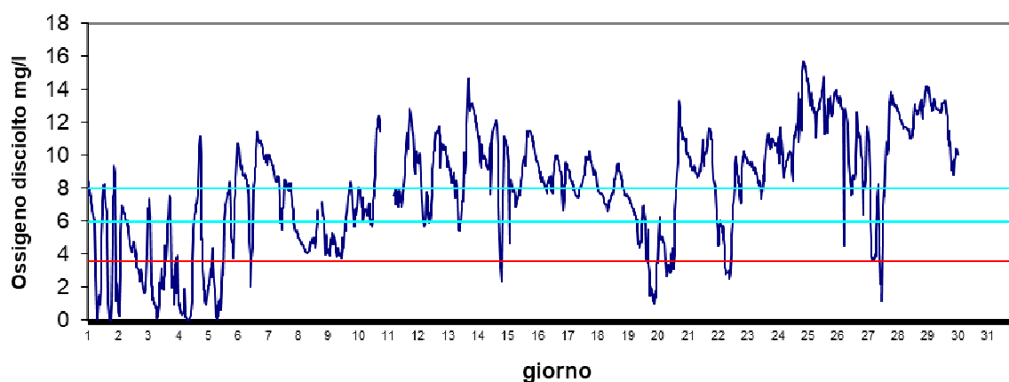
Stazione Scardovari interno Agosto 2024 - Ossigeno disciolto mg/l
