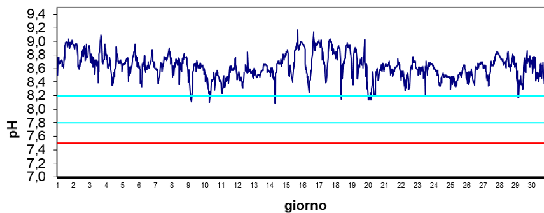
Stazione Barbamarco Giugno 2024 - pH
