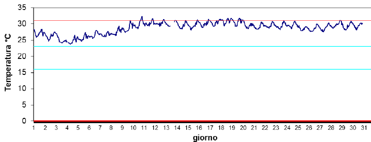
Stazione Vallona Agosto 2024 - Temperatura
