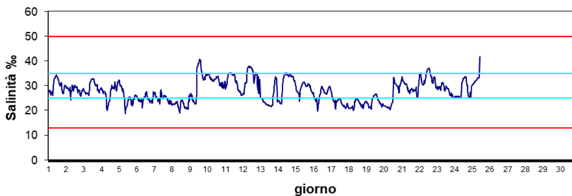
Stazione Canarin Ottobre 2024 - Salinità ‰
