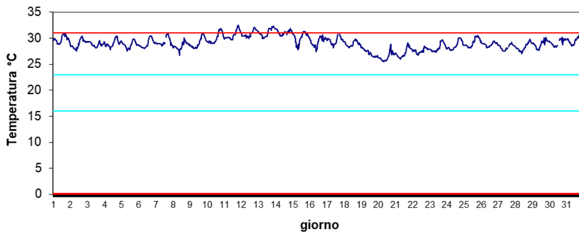
Stazione Vallona Settembre 2024 - Temperatura
