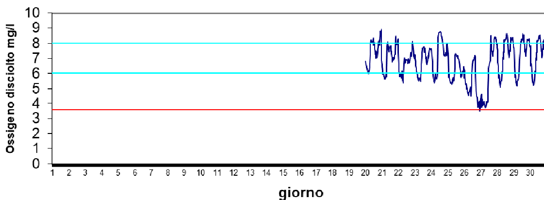
Stazione Marinetta Luglio 2024 - Ossigeno disciolto mg/l
