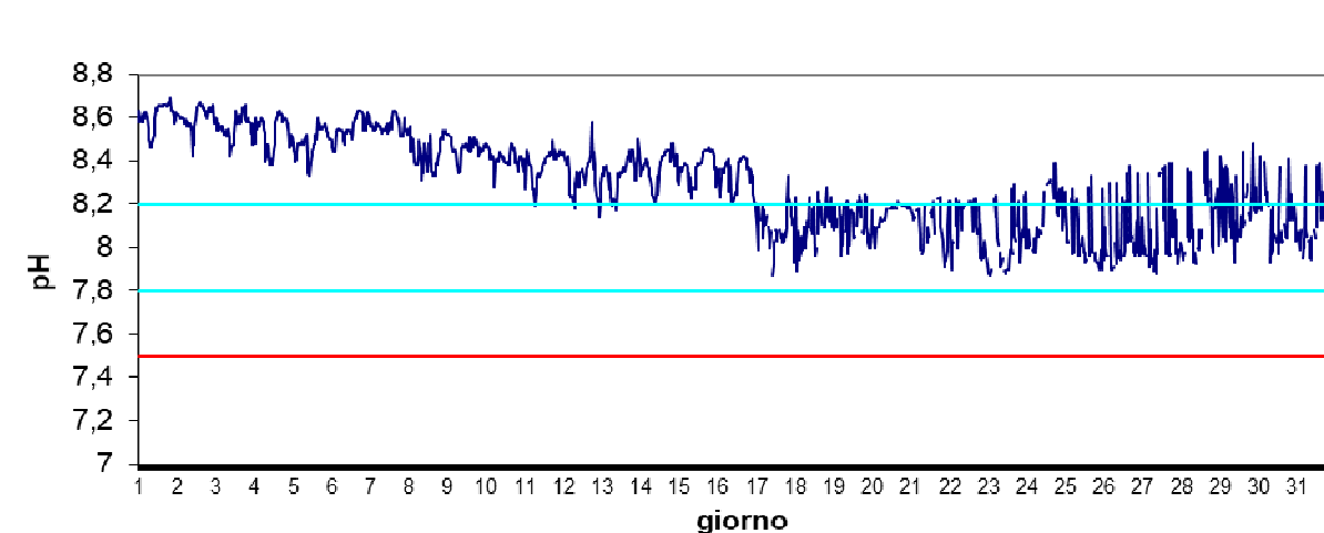
Stazione Vallona Dicembre 2024 - pH
