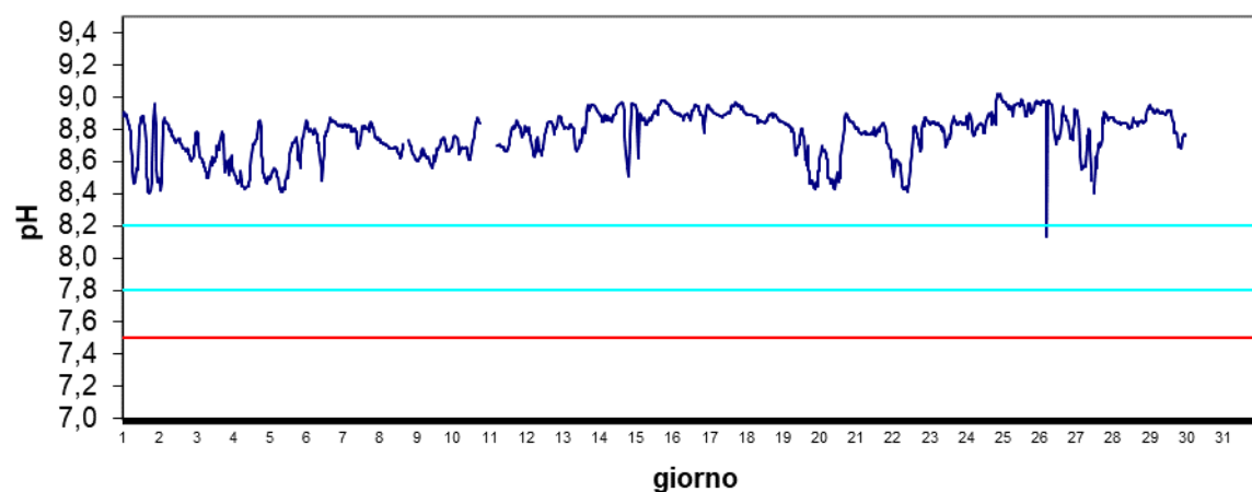
Stazione Scardovari interno Settembre 2024 - pH
