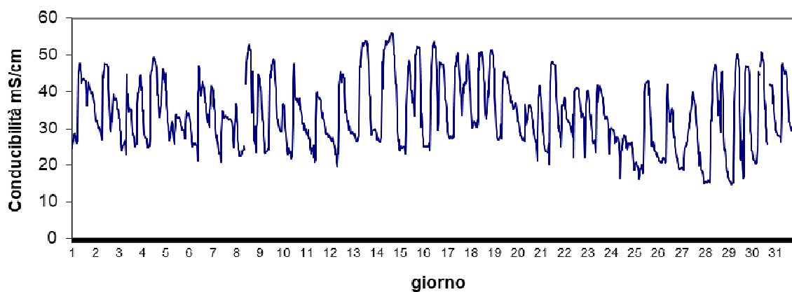
Stazione Basson Settembre 2024 - Conducibilità mS/cm
