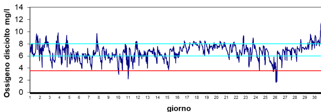
Stazione Canarin Ottobre 2024 - Ossigeno disciolto mg/l
