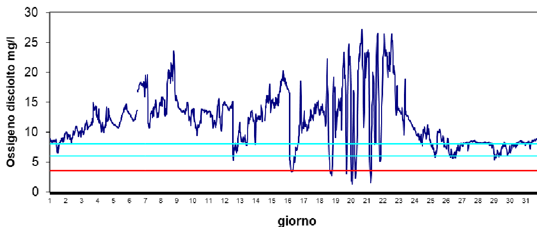
Stazione Scardovari interno Marzo 2024 - Ossigeno disciolto mg/l
