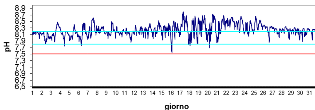
Stazione Scardovari S.Giulia Aprile 2024 - pH
