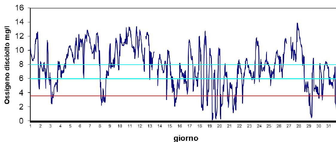
Stazione Scardovari interno Agosto 2024 - Ossigeno disciolto mg/l
