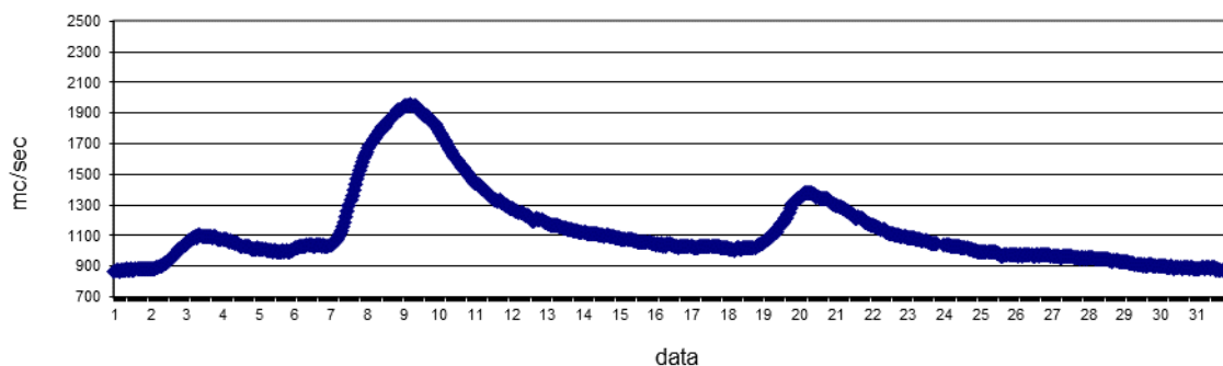
PORTATA PONTELAGOSCURO mc/sec GENNAIO 2024
