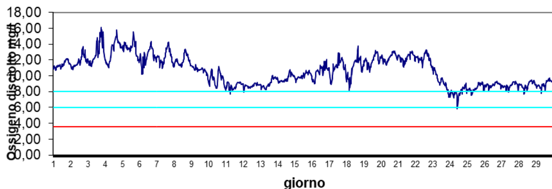
Stazione Caleri Marzo 2024 - Ossigeno disciolto mg/l
