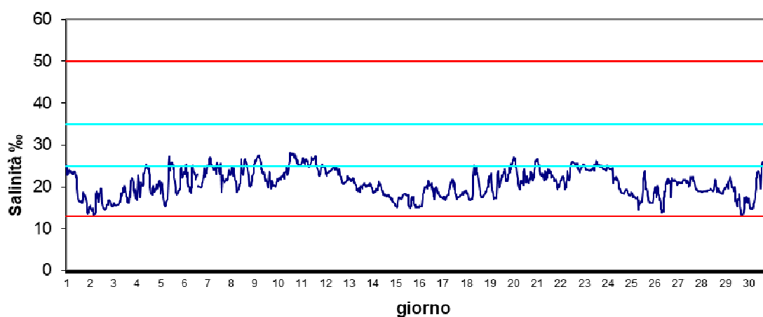
Stazione Barbamarco Giugno 2024 - Salinità ‰
