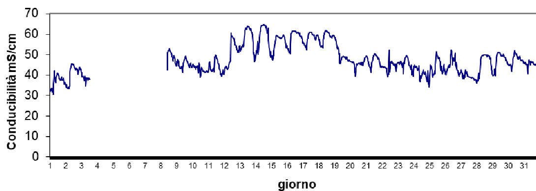
Stazione Canarin Settembre 2024 - Conducibilità mS/cm
