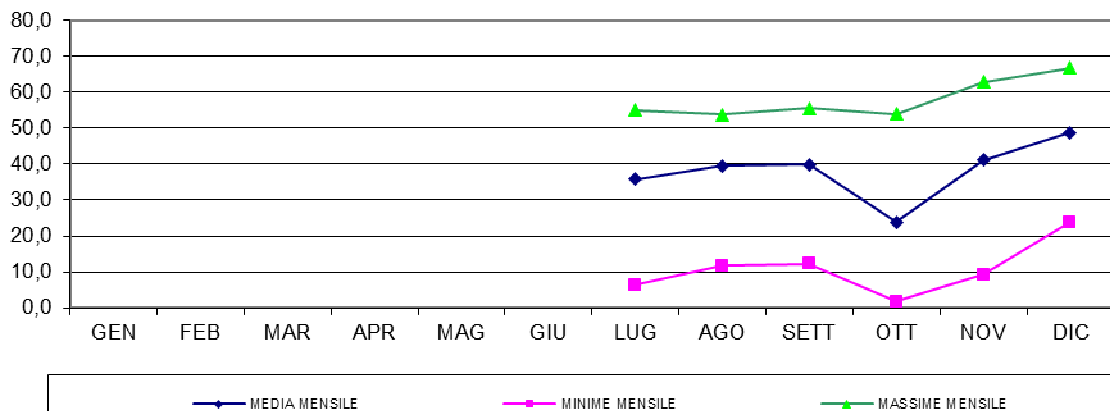
LAGUNA MARINETTA - SALINITA'
