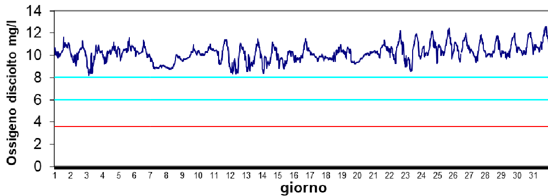
Stazione Caleri Febbraio 2024 - Ossigeno disciolto mg/l
