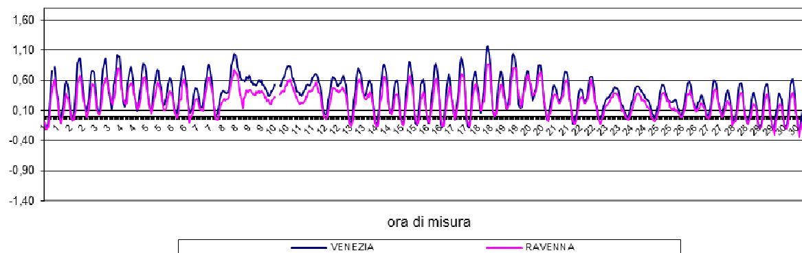
CONFRONTI CICLO di MAREA VENEZIA-RAVENNA OTTOBRE 2024
