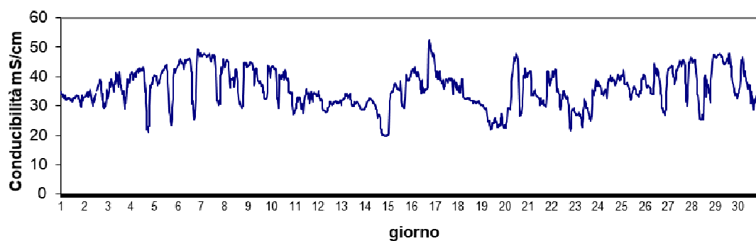
Stazione Barbamarco Maggio 2024 - Conducibilità mS/cm
