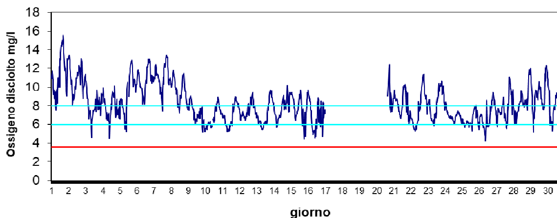
Stazione Vallona Giugno 2024- Ossigeno disciolto mg/l
