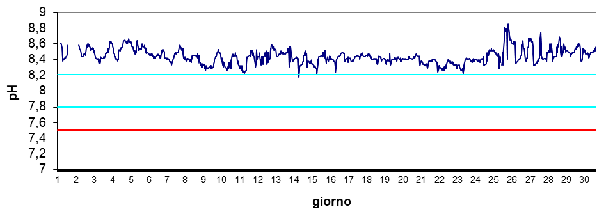
Stazione Basson Settembre 2024 - pH
