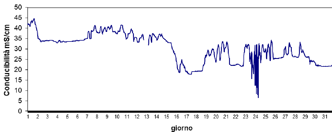
Stazione Scardovari interno Giugno 2024 - Conducibilità mS/cm
