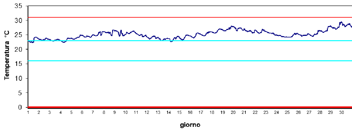
Stazione Scardovari interno Luglio 2024 - Temperatura
