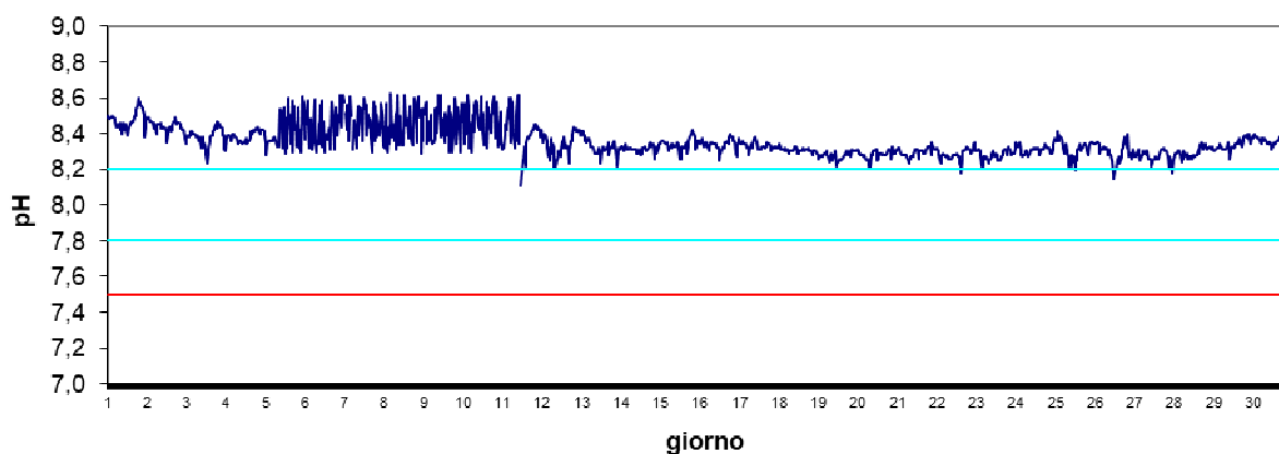
Stazione Caleri Settembre 2024 - pH
