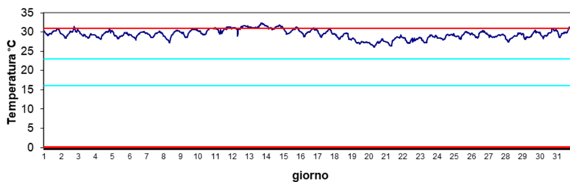
Stazione Scardovari S.Giulia Settembre 2024 - Temperatura
