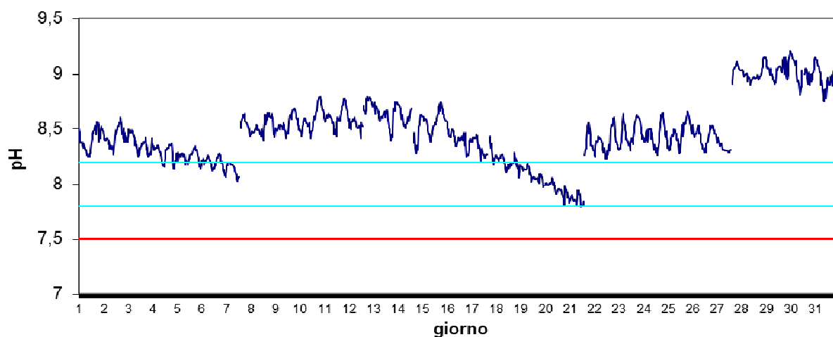
Stazione Vallona Agosto 2024 - pH
