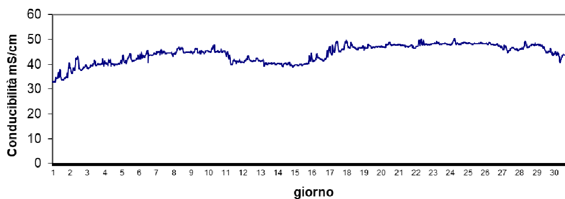
Stazione Caleri Dicembre 2024 - Conducibilità mS/cm
