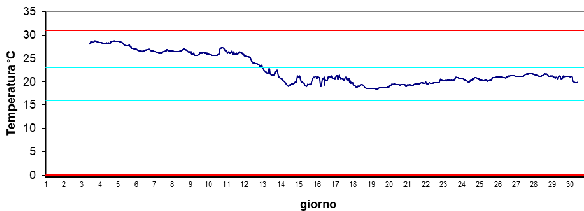
Stazione Scardovari interno Ottobre 2024 - Temperatura
