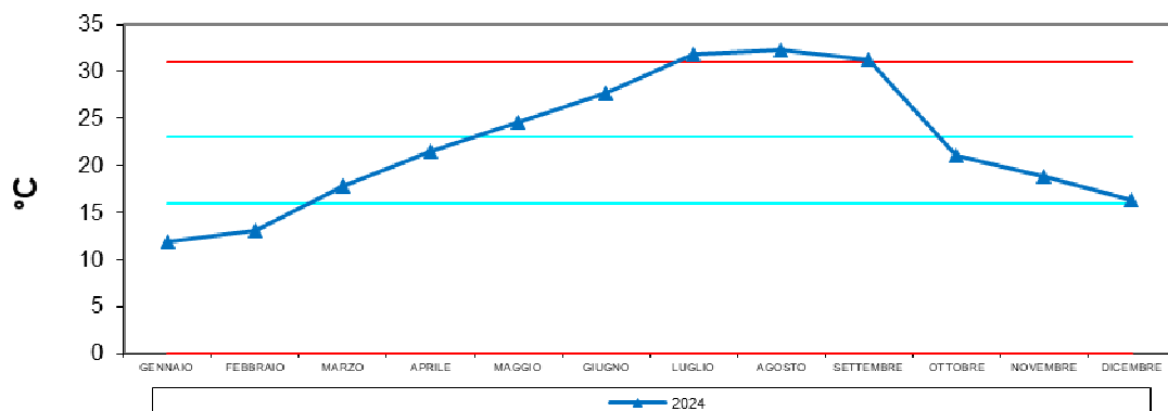
Scardovari S. Giulia - confronto Temperatura MASSIMA 2024
