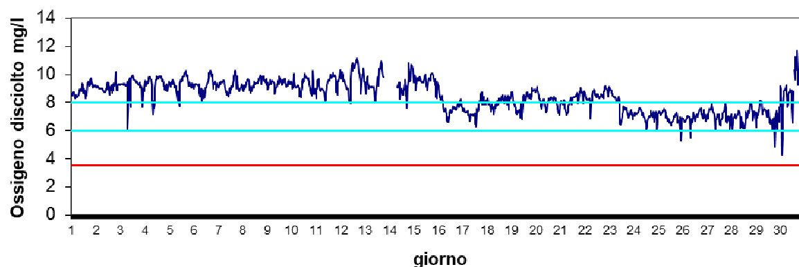
Stazione Scardovari mare Maggio 2024 - Ossigeno disciolto mg/l
