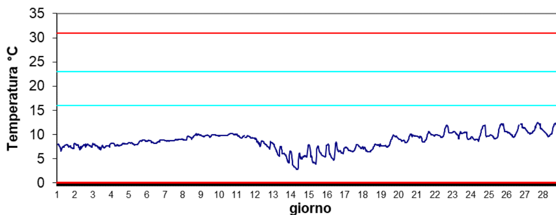
Stazione Basson Marzo 2024 - Temperatura
