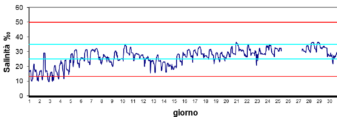
Stazione Scardovari S.Giulia Dicembre 2024 - Salinità ‰
