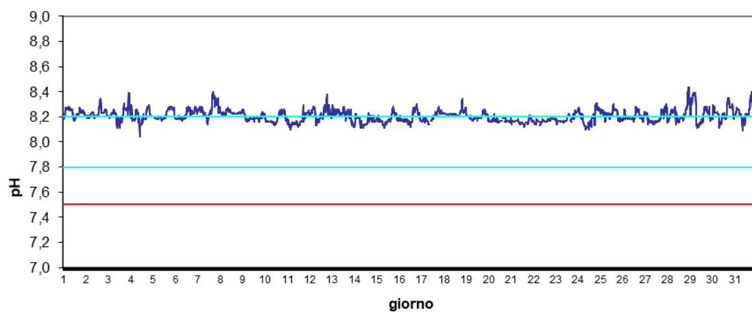
Stazione Barbamarco Dicembre 2024 - pH
