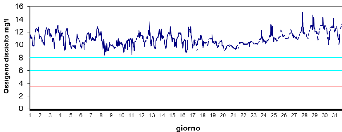
Stazione Vallona Dicembre 2024 - Ossigeno disciolto mg/l
