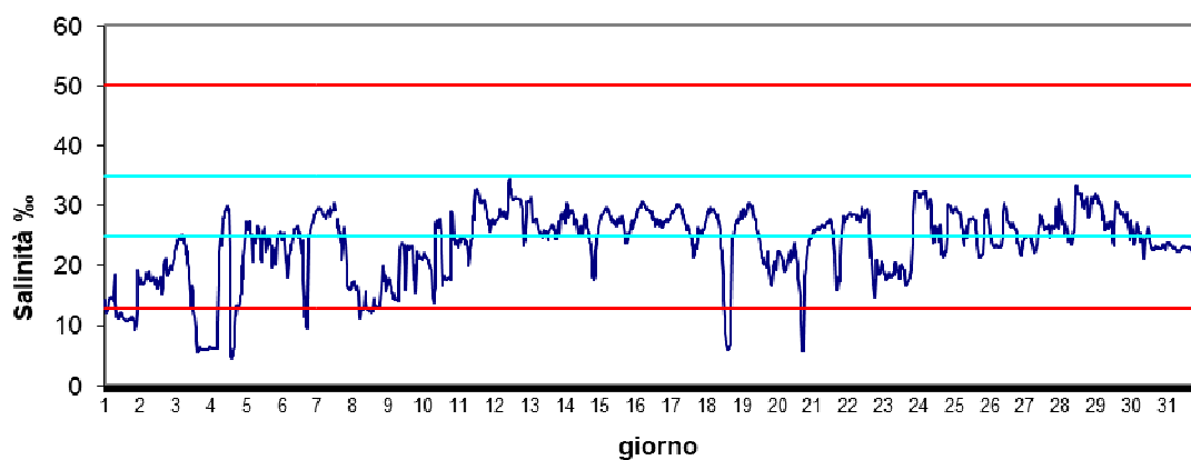
Stazione Barbamarco Marzo 2024 - Salinità ‰
