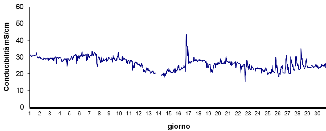
Stazione Vallona Maggio 2024 - Conducibilità mS/cm
