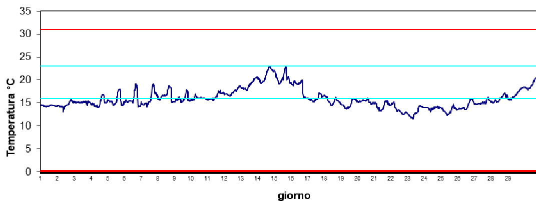
Stazione Barbamarco Aprile 2024 - Temperatura
