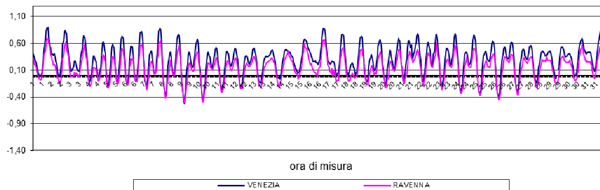
CONFRONTI CICLO di MAREA VENEZIA-RAVENNA MAGGIO 2024
