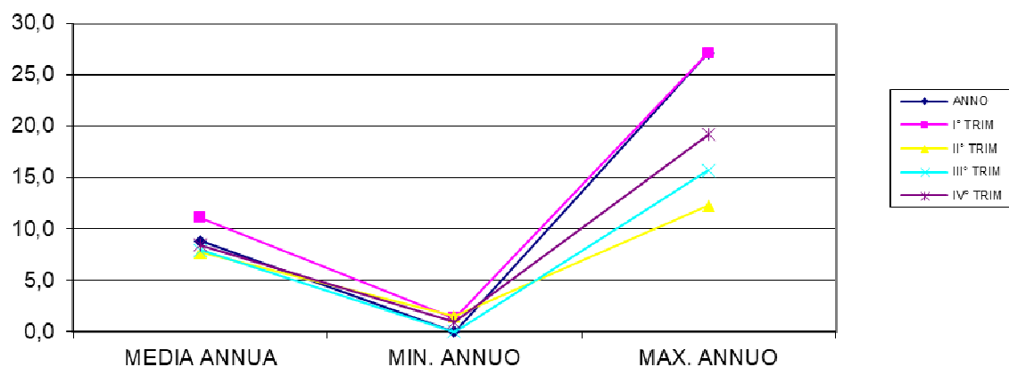
LAGUNA SCARDOVARI S. GIULIA - OSSIGENO DISCIOLTO
