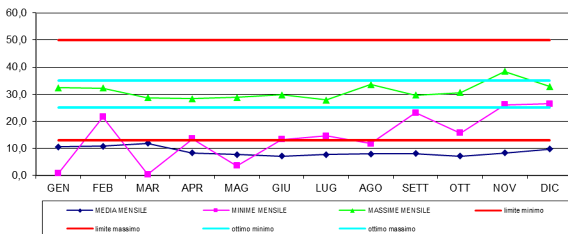
LAGUNA SCARDOVARI INTERNO - OSSIGENO DISCIOLTO
