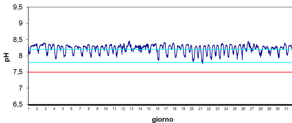
Stazione Marinetta Agosto 2024 - pH
