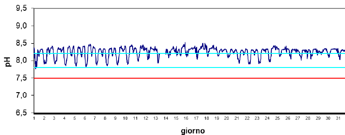
Stazione Marinetta Luglio 2024 - pH
