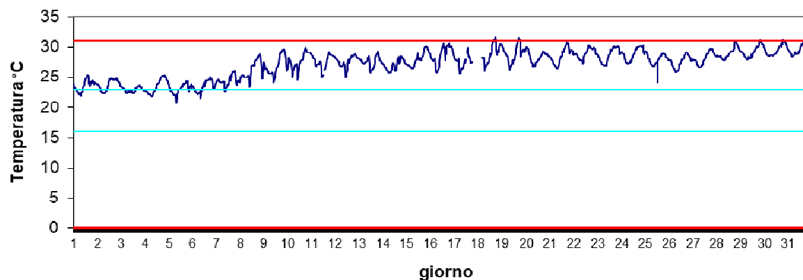
Stazione Basson Agosto 2024 - Temperatura
