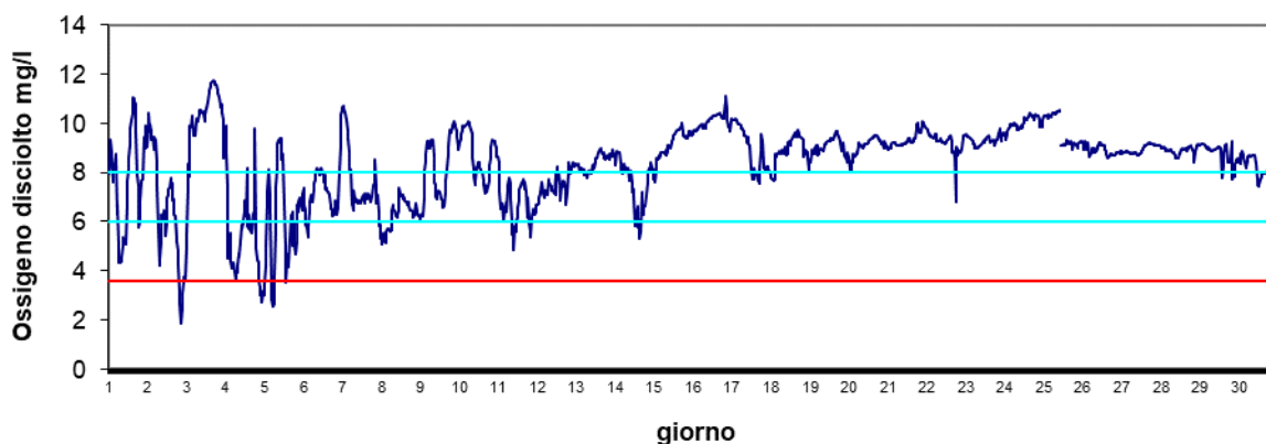
Stazione Scardovari interno Novembre 2024 - Ossigeno disciolto mg/l
