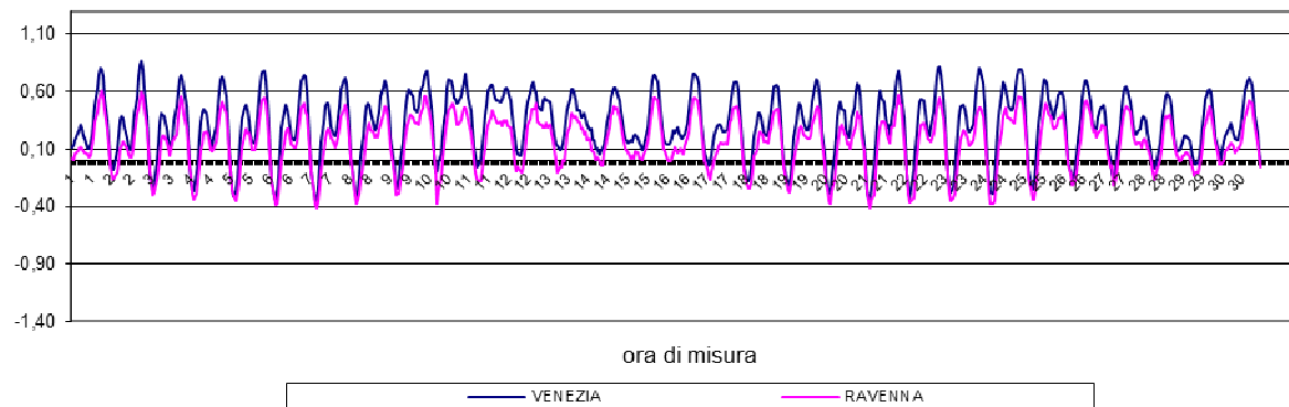
CONFRONTI CICLO di MAREA VENEZIA-RAVENNA GIUGNO 2024
