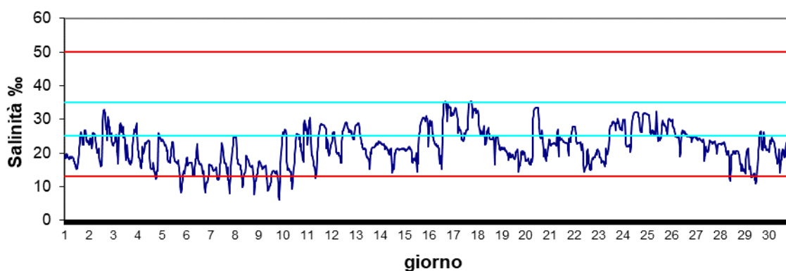
Stazione Scardovari S.Giulia Maggio 2024 - Salinità ‰
