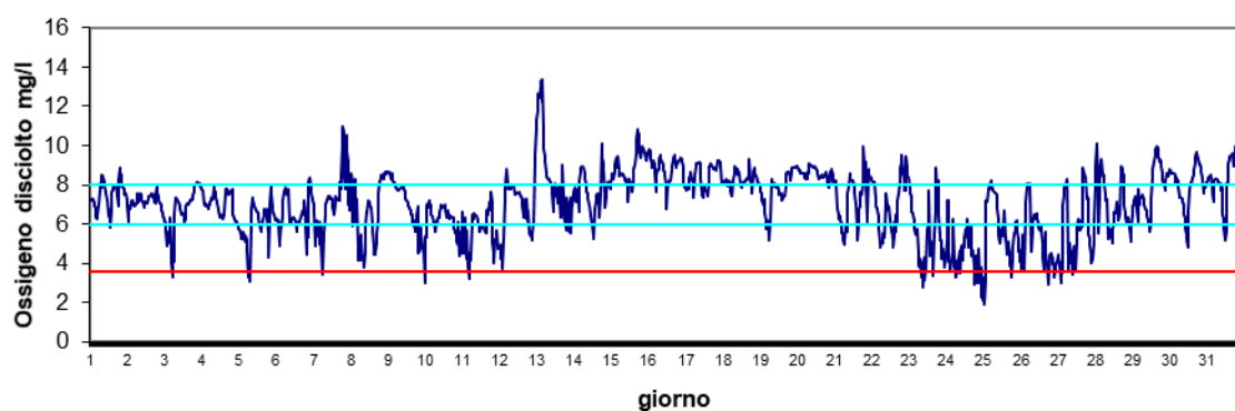
Stazione Scardovari S.Giulia Novembre 2024 - Ossigeno disciolto mg/l
