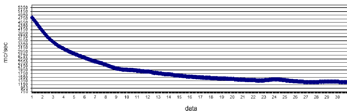
PORTATA PONTELAGOSCURO mc/sec NOVEMBRE 2024
