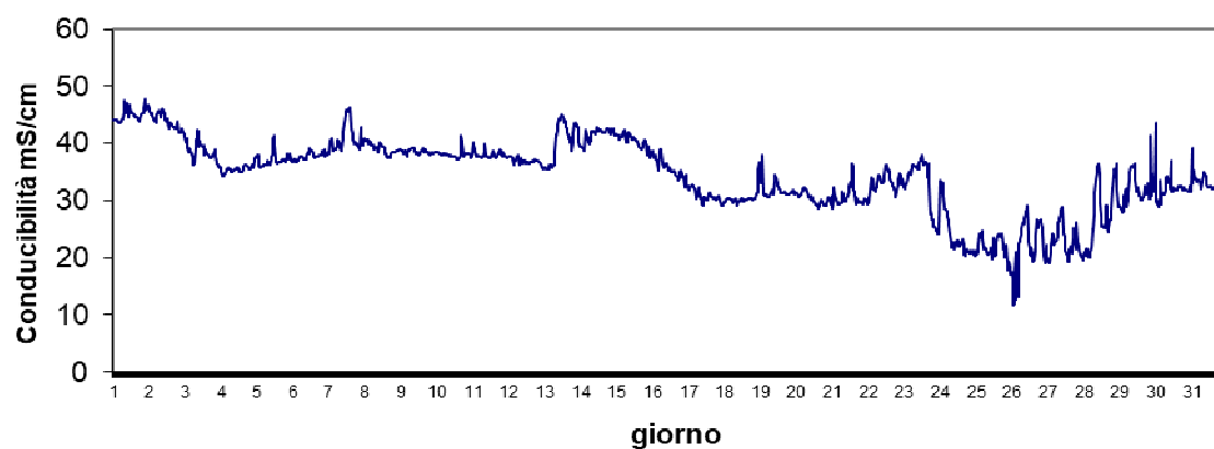
Stazione Caleri Novembre 2024 - Conducibilità mS/cm
