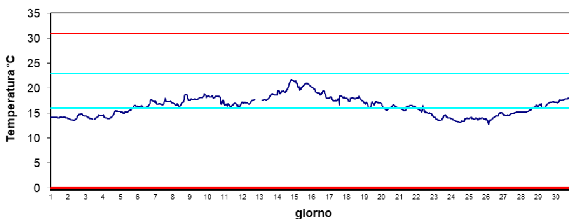
Stazione Scardovari interno Maggio 2024 - Temperatura
