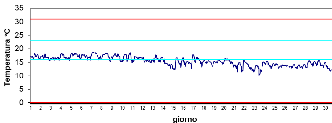
Stazione Canarin Novembre 2024 - Temperatura
