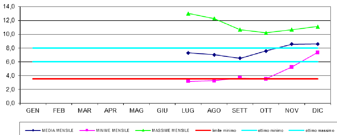
LAGUNA MARINETTA - OSSIGENO DISCIOLTO
