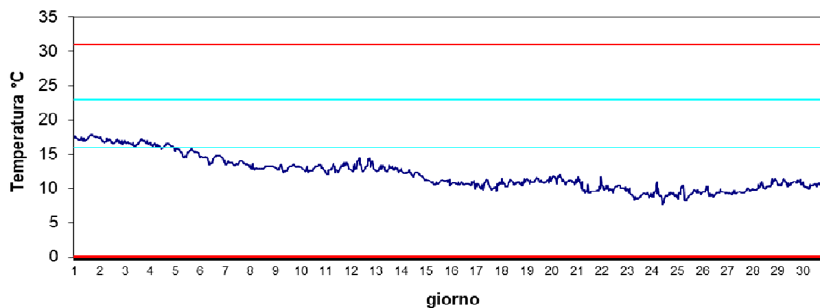
Stazione Vallona Novembre 2024 - Temperatura
