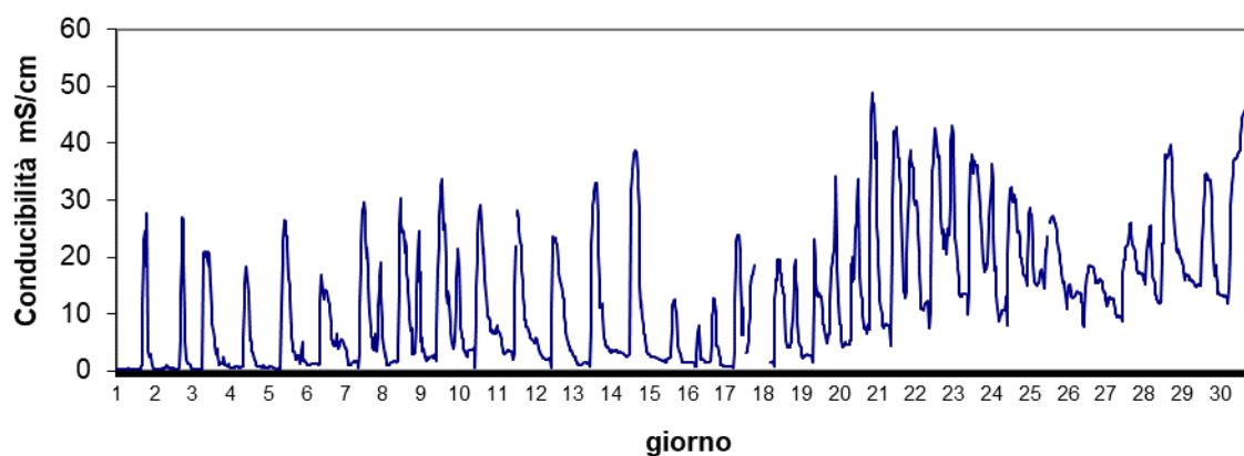
Stazione Basson Agosto 2024 - Conducibilità mS/cm
