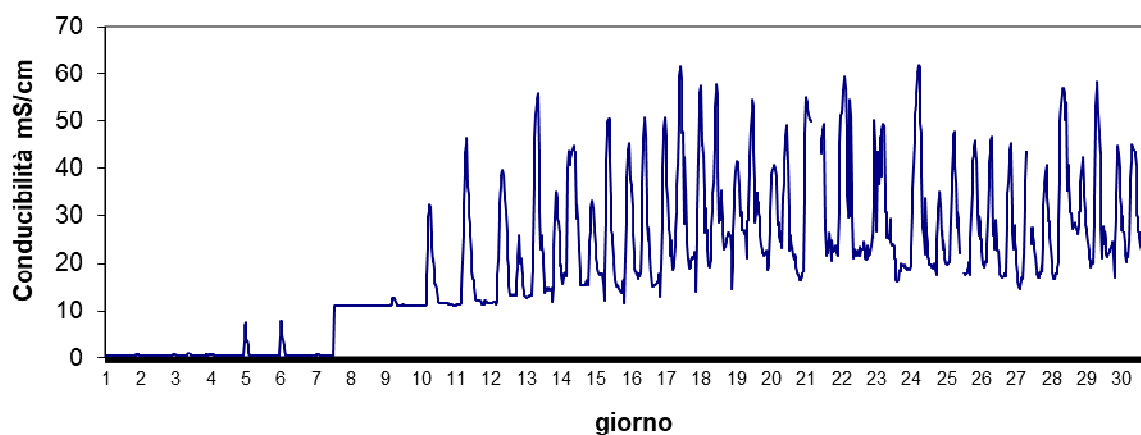
Stazione Basson Dicembre 2024 - Conducibilità mS/cm
