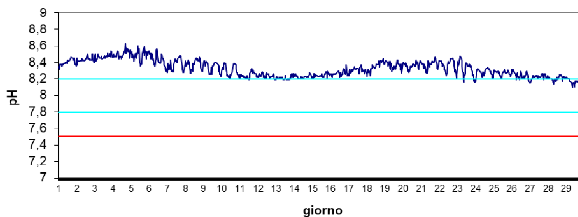
Stazione Vallona Marzo 2024 - pH
