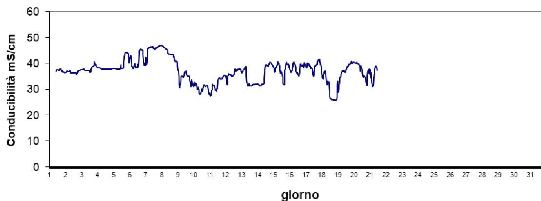
Stazione Scardovari interno Novembre 2024 - Conducibilità mS/cm
