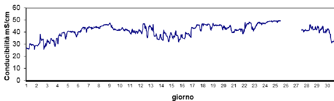
Stazione Barbamarco Dicembre 2024 - Conducibilità mS/cm
