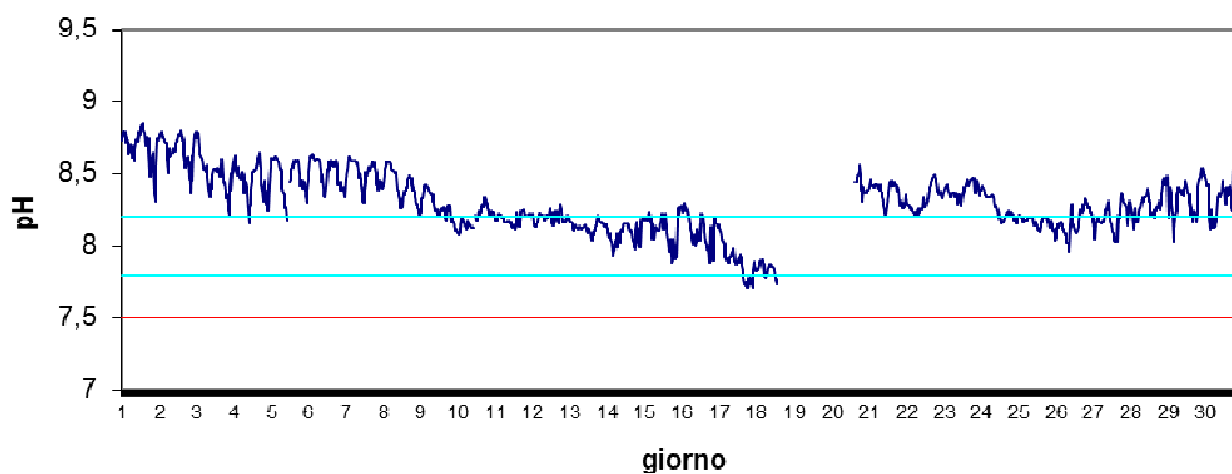
Stazione Vallona Giugno 2024 - pH
