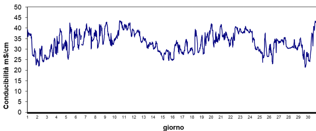
Stazione Barbamarco Giugno 2024 - Conducibilità mS/cm
