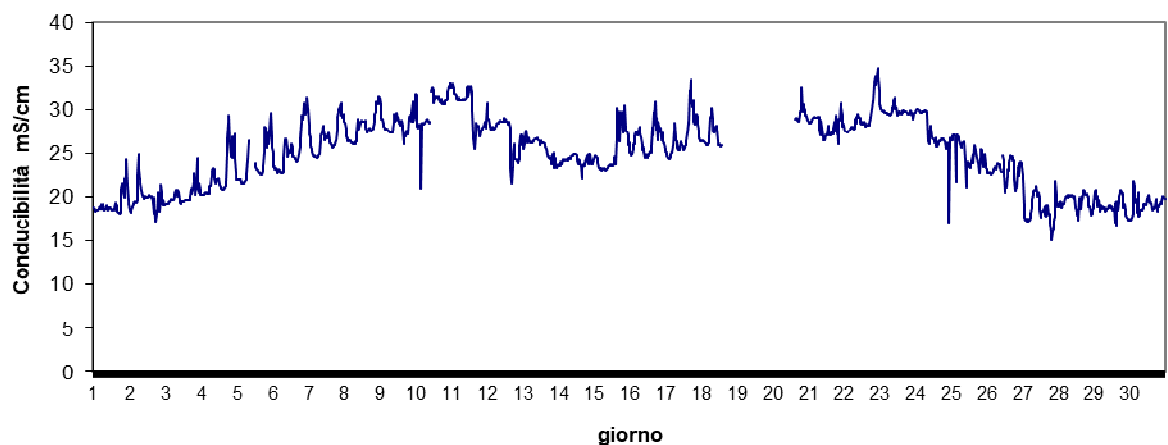
Stazione Vallona Giugno 2024 - Conducibilità mS/cm
