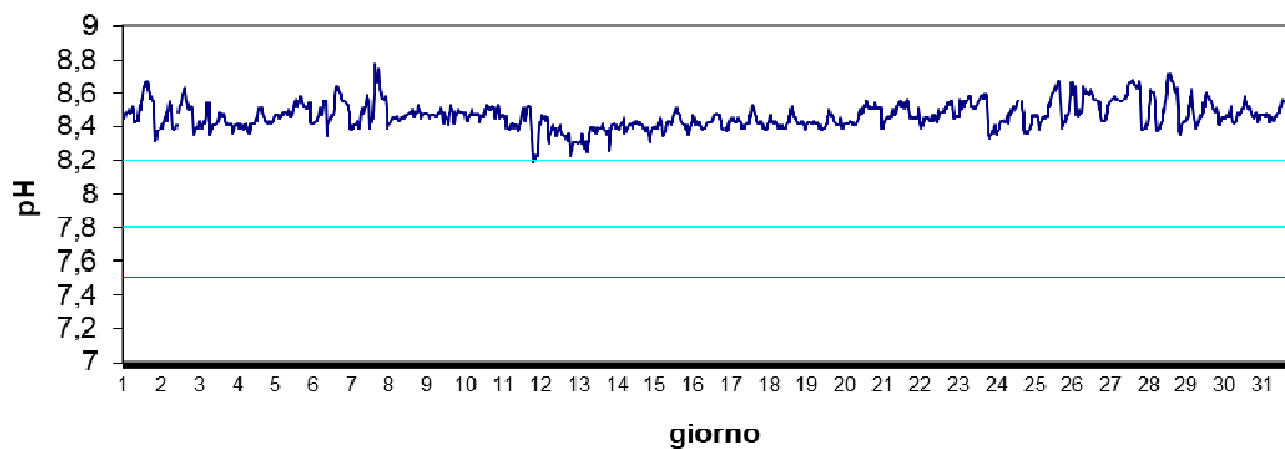
Stazione Basson Dicembre 2024 - pH
