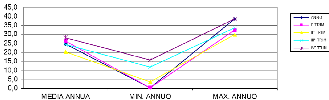
LAGUNA SCARDOVARI S. GIULIA - SALINITA'
