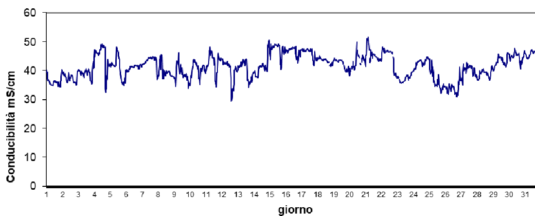
Stazione Barbamarco Dicembre 2024 - Conducibilità mS/cm
