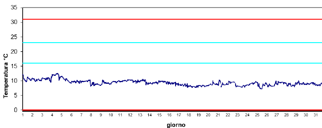
Stazione Barbamarco Dicembre 2024 - Temperatura
