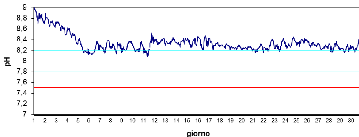
Stazione Vallona Settembre 2024 - pH
