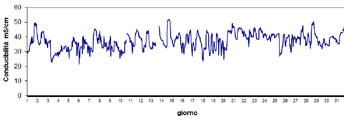
Stazione Scardovari mare Agosto 2024 - Conducibilità mS/cm
