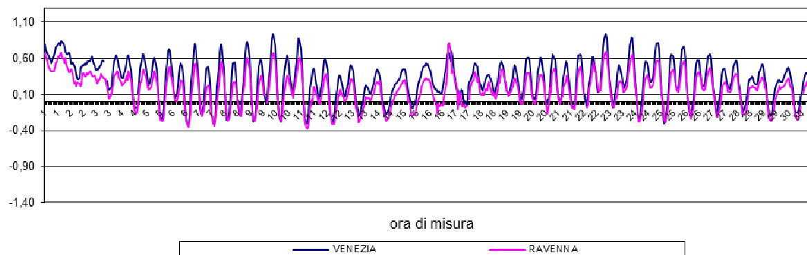
CONFRONTI CICLO di MAREA VENEZIA-RAVENNA APRILE 2024
