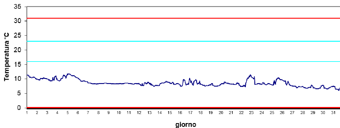
Stazione Scardovari interno Dicembre 2024 - Temperatura
