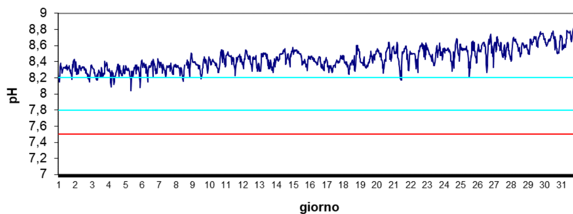
Stazione Vallona Maggio 2024 - pH
