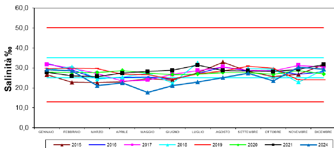
Scardovari interno - confronto Salinità MEDIA 2015 - 2016 - 2017 - 2018 - 2019 - 2020 - 2021 - 2024
