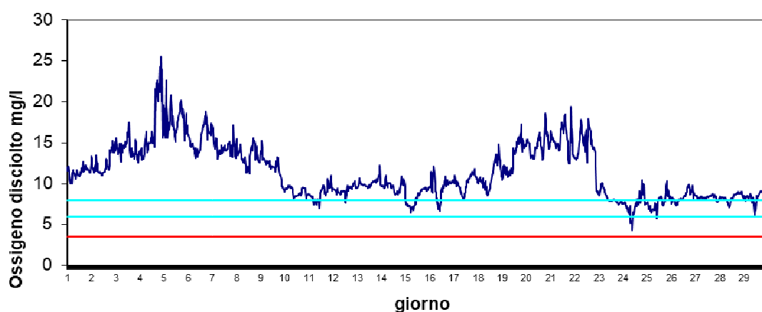
Stazione Barbamarco Febbraio 2024- Ossigeno disciolto mg/l
