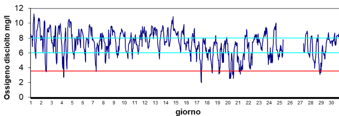
Stazione Scardovari S.Giulia Dicembre 2024 - Ossigeno disciolto mg/l
