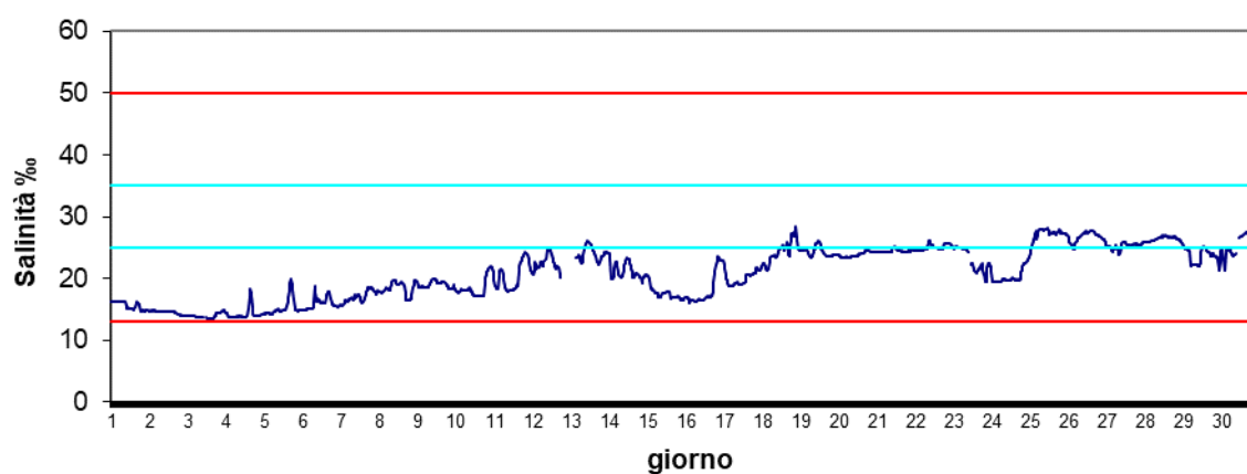
Stazione Scardovari interno Maggio 2024 - Salinità ‰
