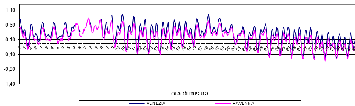
CONFRONTI CICLO di MAREA VENEZIA-RAVENNA GENNAIO 2024
