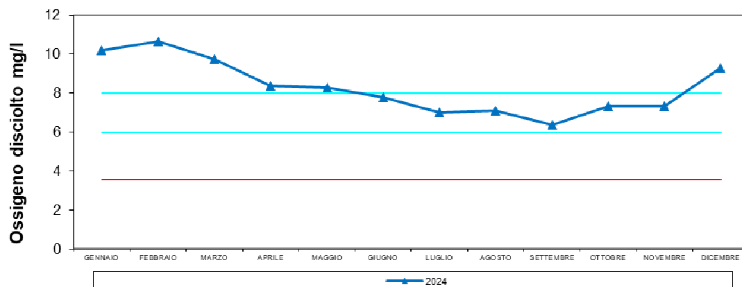
Caleri -confronto Ossigeno disciolto mg/L MINIMA 2024
