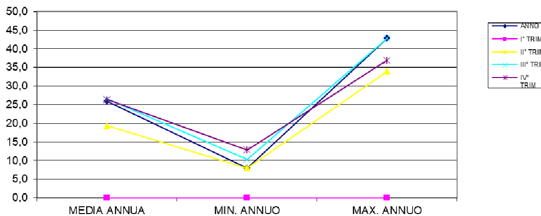
LAGUNA CANARIN - OSSIGENO DISCIOLTO
