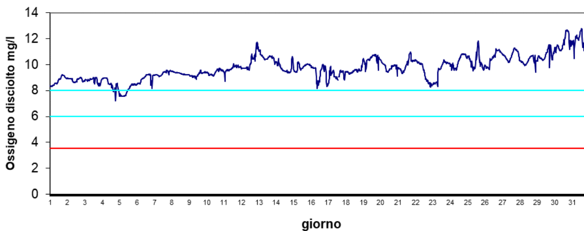
Stazione Scardovari interno Dicembre 2024 - Ossigeno disciolto mg/l
