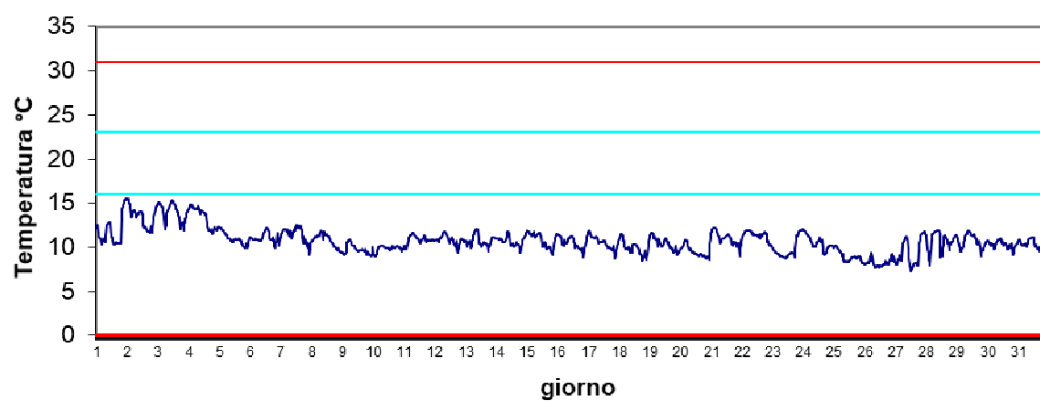
Stazione Canarin Dicembre 2024 - Temperatura
