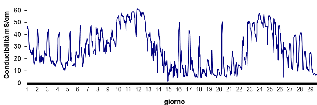
Stazione Basson Marzo 2024 - Conducibilità mS/cm
