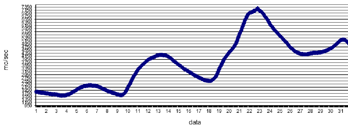
PORTATA PONTELAGOSCURO mc/sec OTTOBRE 2024
