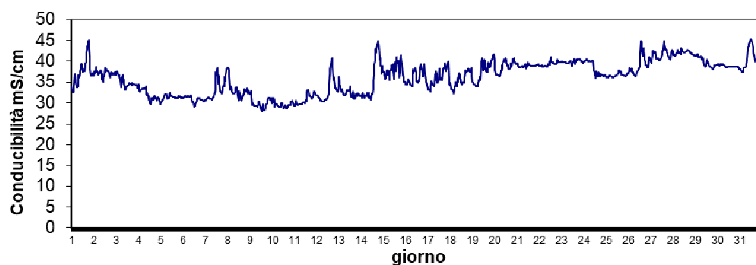
Stazione Caleri Agosto 2024 - Conducibilità mS/cm
