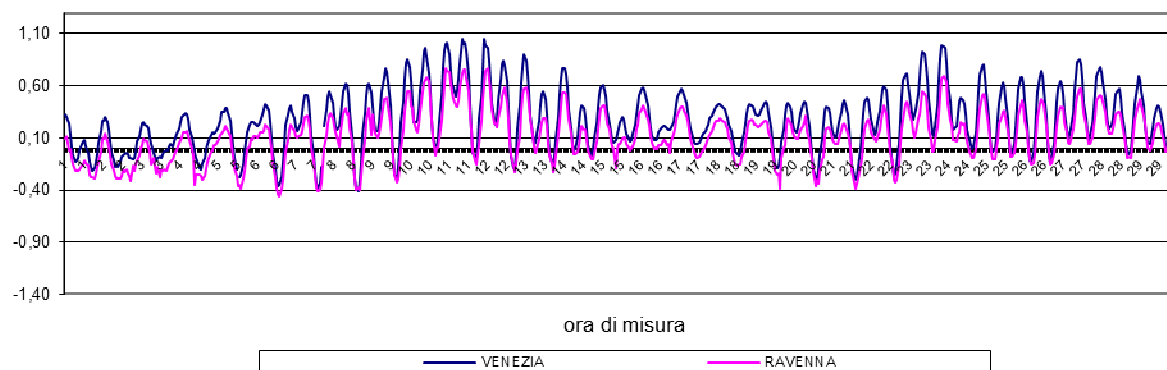
CONFRONTI CICLO di MAREA VENEZIA-RAVENNA FEBBRAIO 2024
