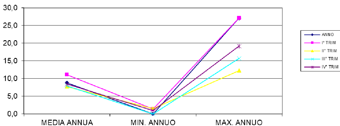
LAGUNA SCARDOVARI INTERNO - OSSIGENO DISCIOLTO
