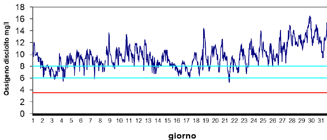
Stazione Vallona Maggio 2024 - Ossigeno disciolto mg/l
