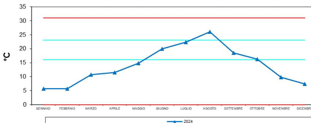
Scardovari S. Giulia - confronto Temperatura MINIMA 2024
