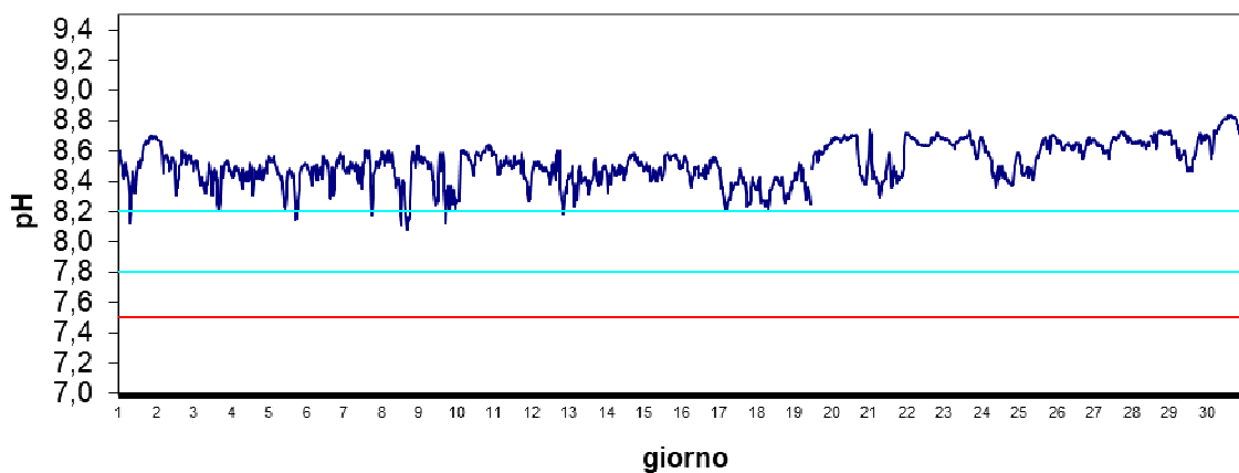
Stazione Scardovari interno Luglio 2024 - pH
