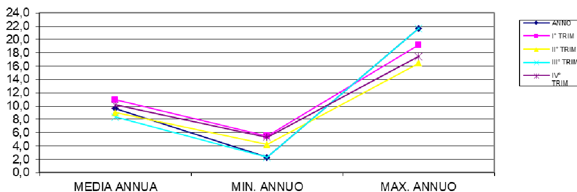
LAGUNA CALERI - OSSIGENO DISCIOLTO
