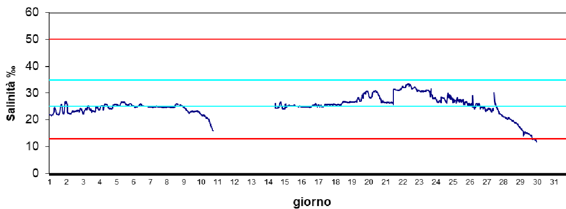
Stazione Scardovari interno Settembre 2024 - Salinità ‰
