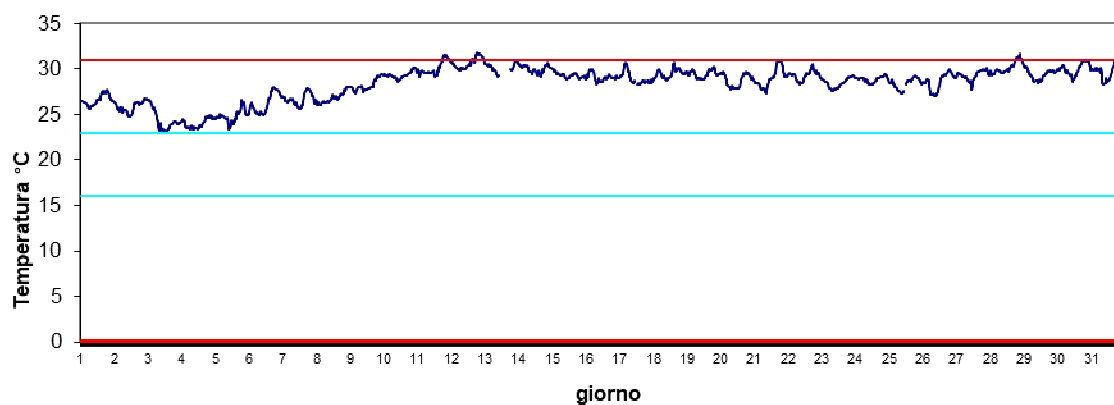
Stazione Barbamarco Luglio 2024 - Temperatura
