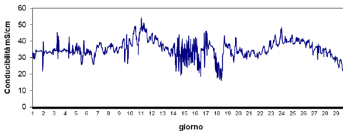
Stazione Vallona Marzo 2024 - Conducibilità mS/cm
