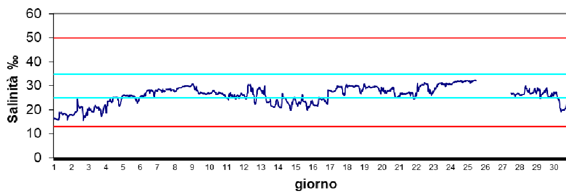
Stazione Barbamarco Dicembre 2024 - Salinità ‰
