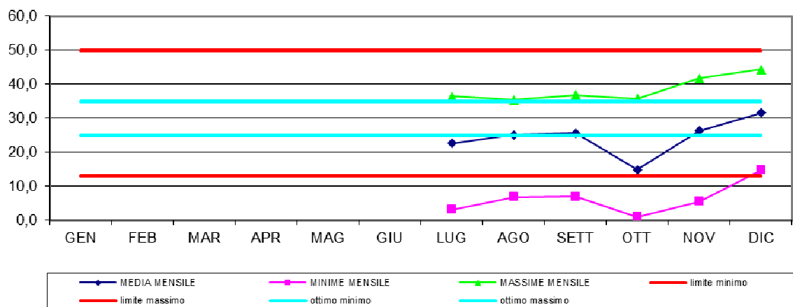
LAGUNA MARINETTA - OSSIGENO DISCIOLTO
