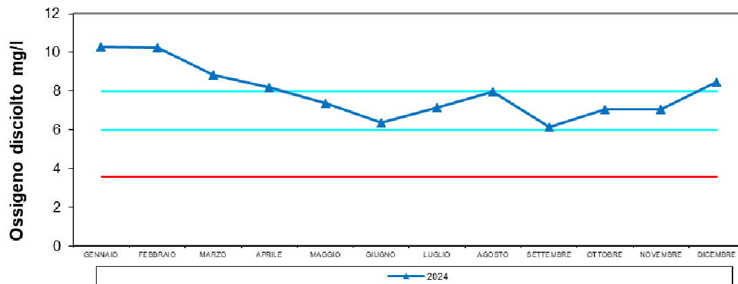
Scardovari S. Giulia - confronto Ossigeno disciolto mg/L MEDIA 2024
