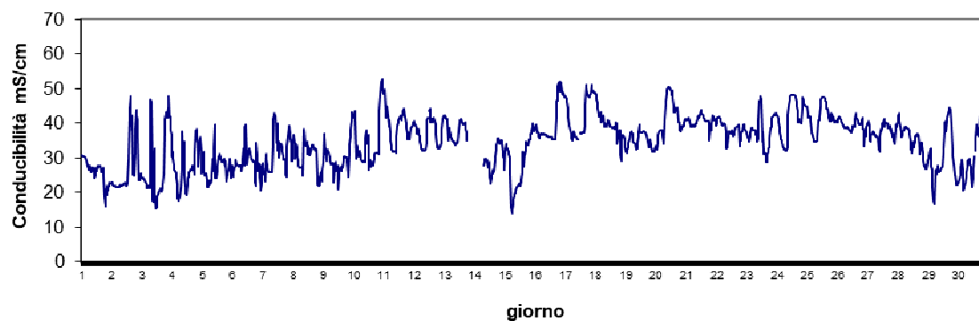
Stazione Scardovari mare Maggio 2024 - Conducibilità mS/cm
