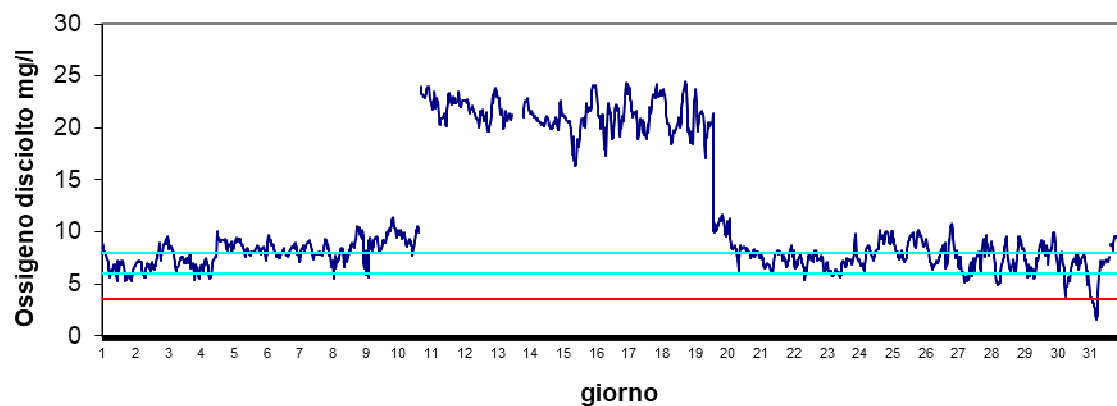
Stazione Scardovari mare Agosto 2024 - Ossigeno disciolto mg/l
