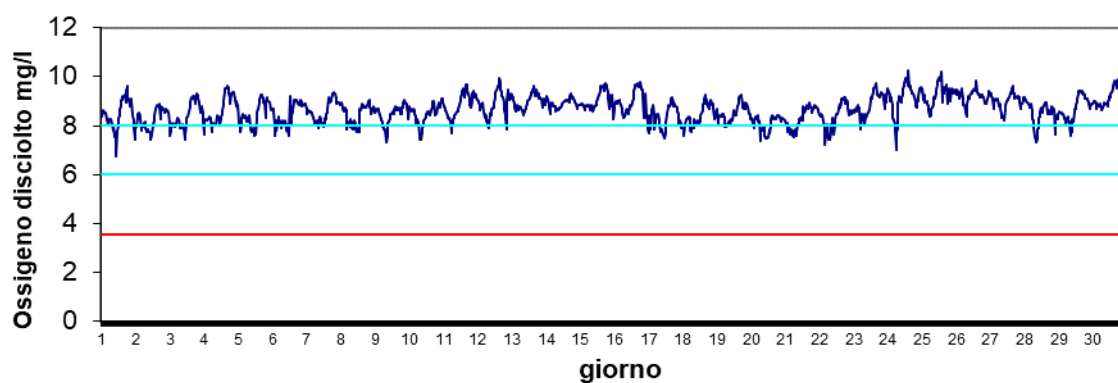
Stazione Caleri Dicembre 2024 - Ossigeno disciolto mg/l
