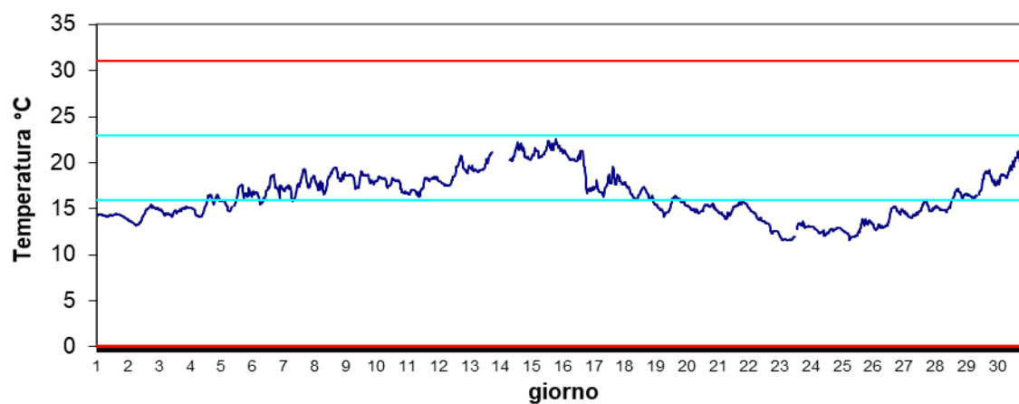
Stazione Vallona Maggio 2024 - Temperatura
