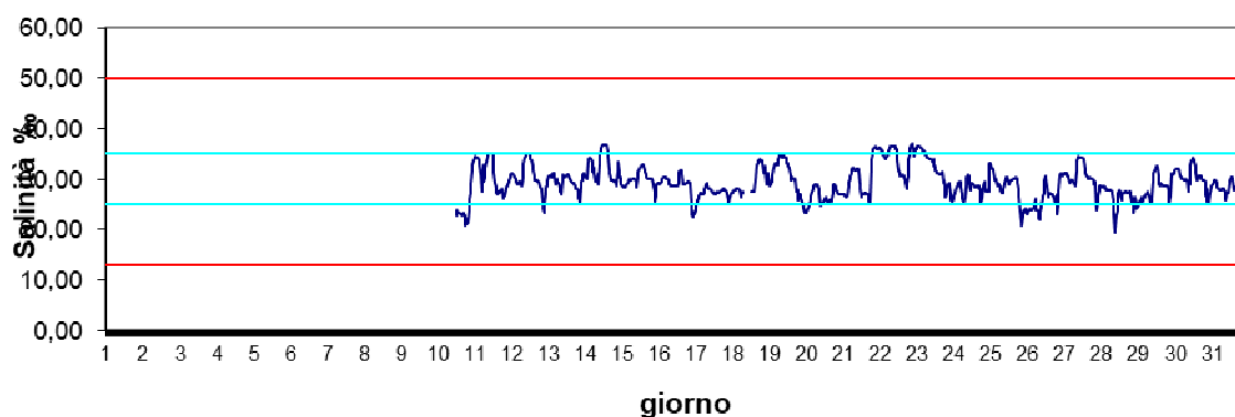
Stazione Scardovari S.Giulia Febbraio 2024 - Salinità ‰
