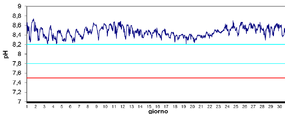
Stazione Vallona Novembre 2024 - pH
