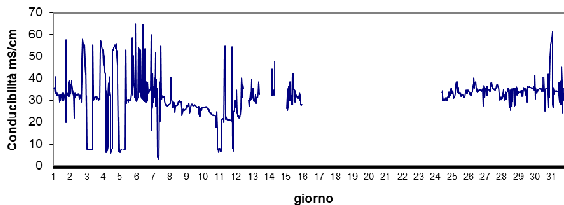
Stazione Vallona Febbraio 2024 - Conducibilità mS/cm
