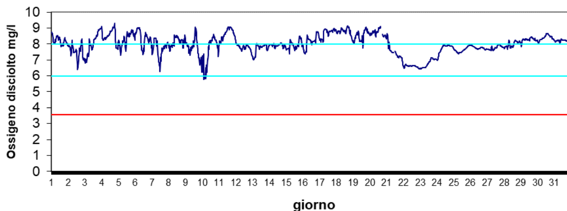
Stazione Basson Novembre 2024 - Ossigeno disciolto mg/l
