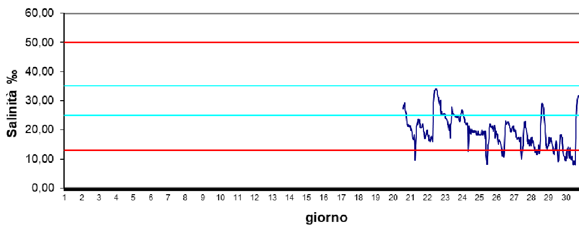
Stazione Canarin Luglio 2024 - Salinità ‰
