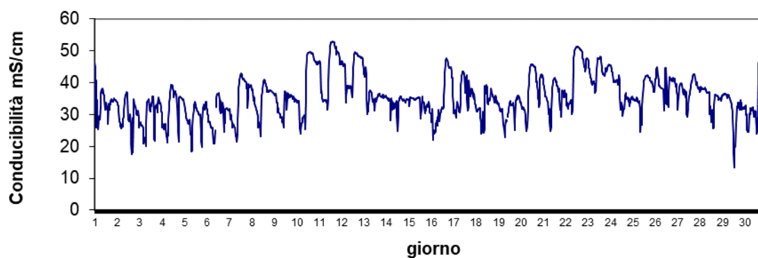
Stazione Scardovari S.Giulia Luglio 2024 - Conducibilità mS/cm
