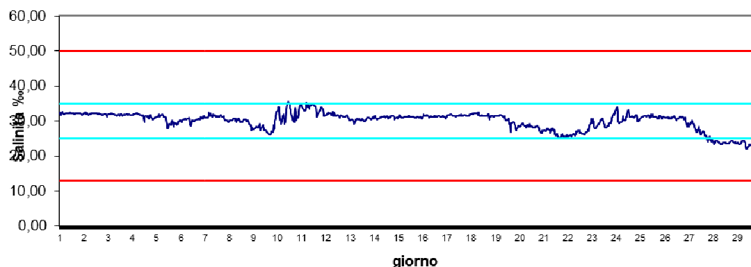
Stazione Caleri Marzo 2024 - Salinità ‰
