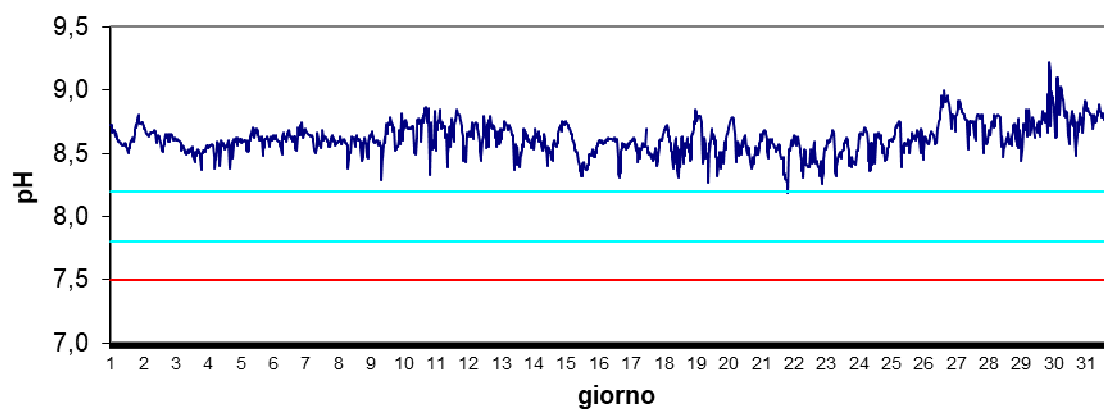
Stazione Scardovari mare Giugno 2024 - pH
