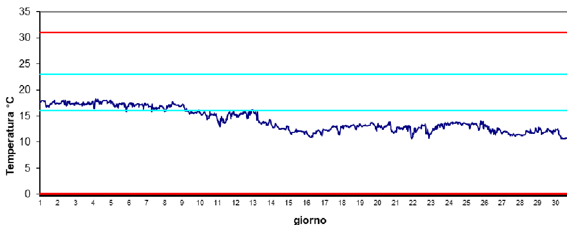
Stazione Barbamarco Novembre 2024 - Temperatura
