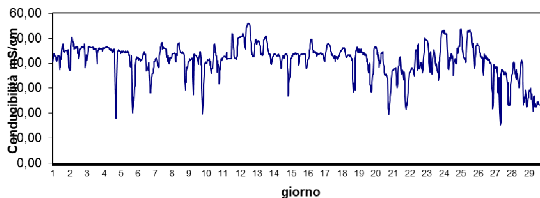
Stazione Scardovari S.Giulia Marzo 2024 - Conducibilità mS/cm
