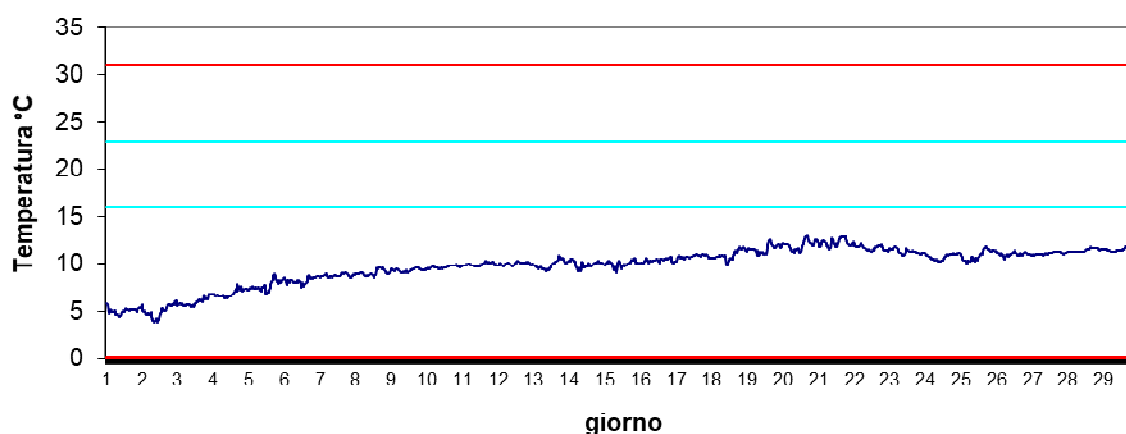
Stazione Vallona Marzo 2024 - Temperatura
