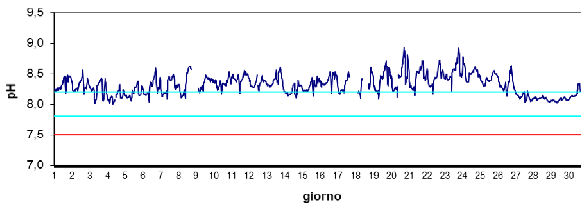
Stazione Basson Giugno 2024 - pH
