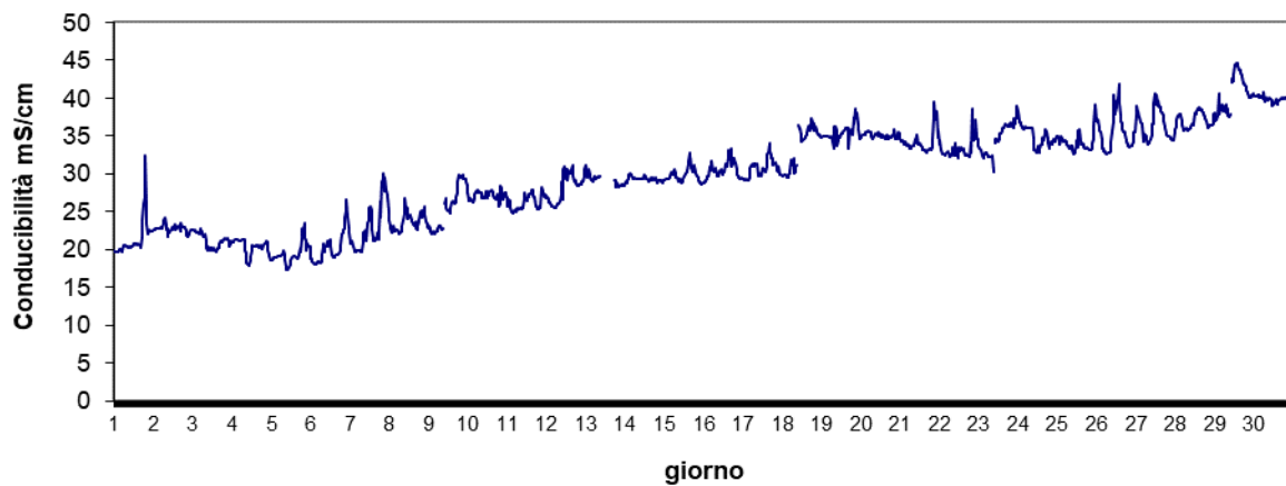
Stazione Vallona Agosto 2024 - Conducibilità mS/cm
