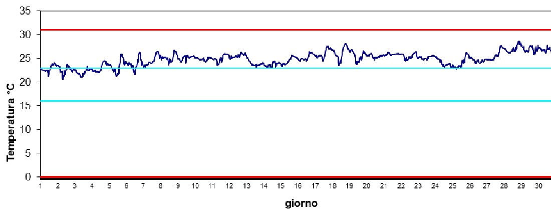
Stazione Barbamarco Giugno 2024 - Temperatura
