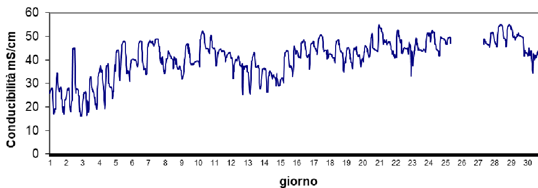
Stazione Scardovari S.Giulia Dicembre 2024 - Conducibilità mS/cm
