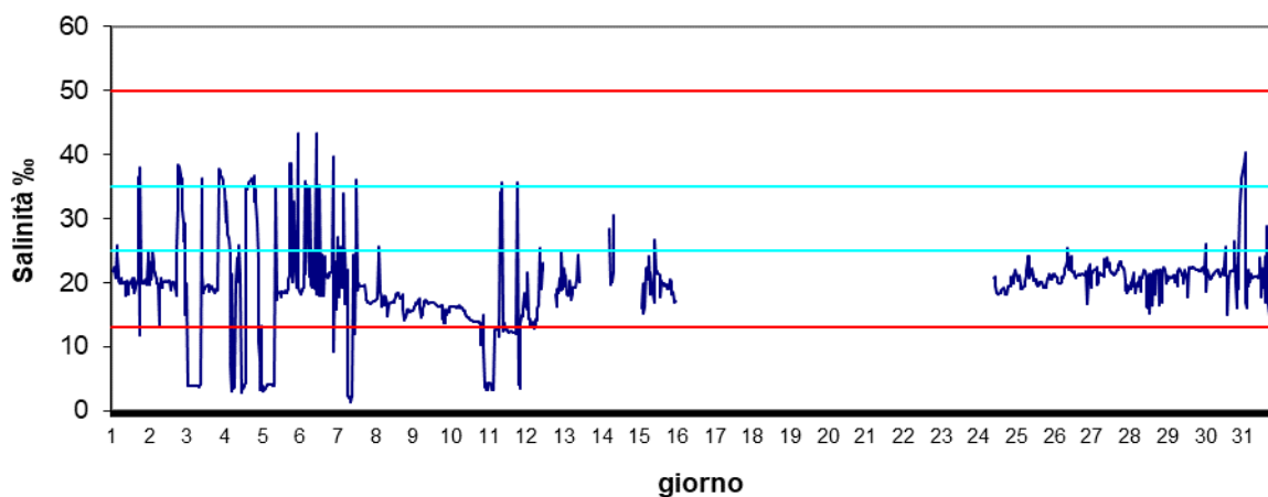
Stazione Vallona Gennaio 2024 - Salinità ‰
