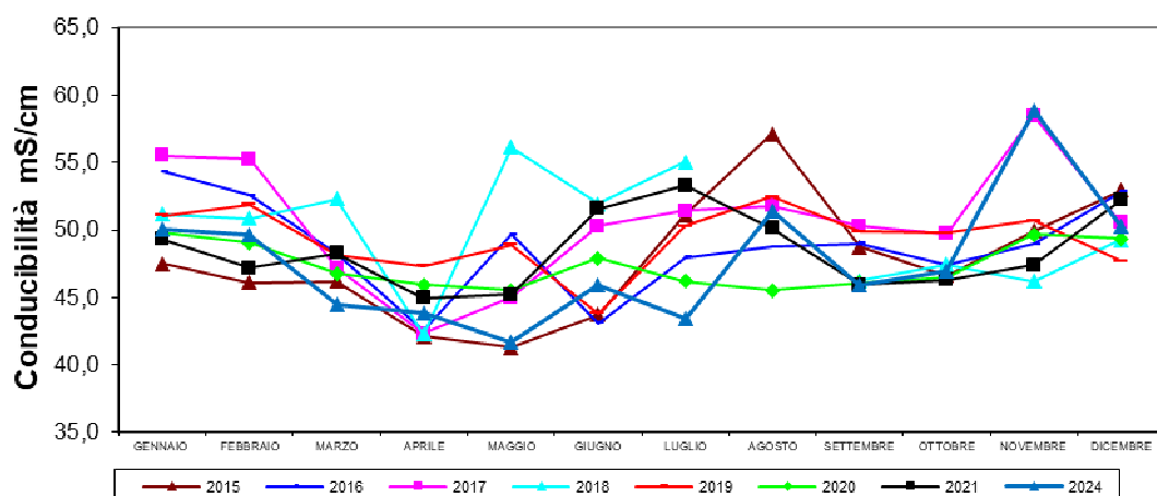
Scardovari interno - confronto Conducibilità MASSIMA 2015 - 2016 - 2017 - 2018 - 2019 - 2020 - 2021 - 2024
