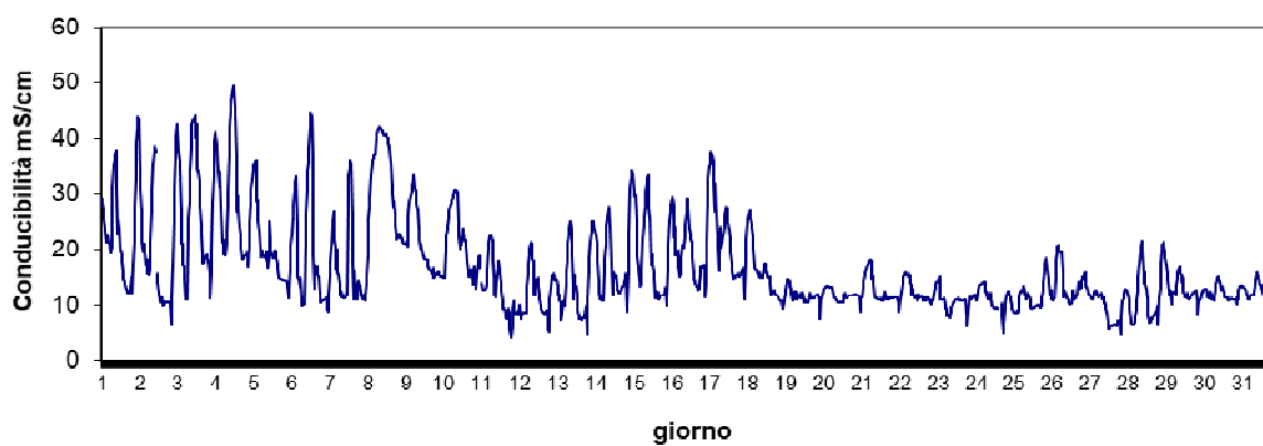
Stazione Basson Dicembre 2024 - Conducibilità mS/cm
