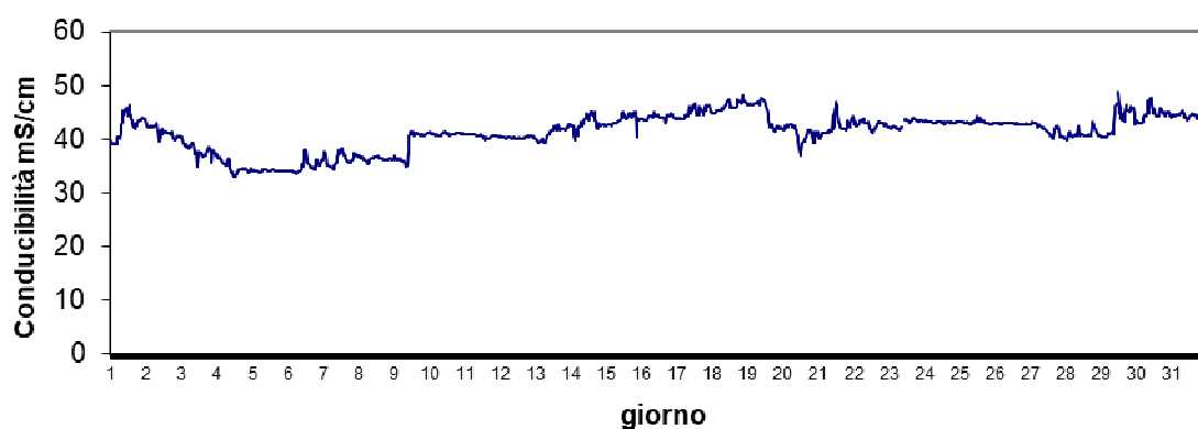
Stazione Caleri Settembre 2024 - Conducibilità mS/cm
