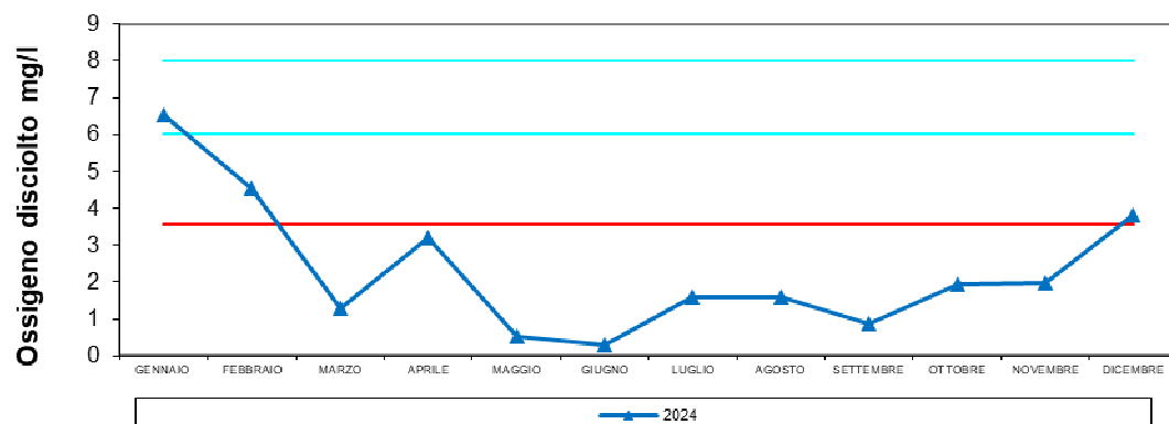
Scardovari S. Giulia - confronto Ossigeno disciolto mg/L MINIMA 2024
