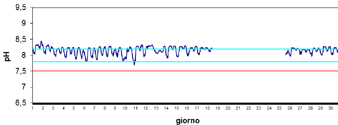
Stazione Marinetta Settembre 2024 - pH
