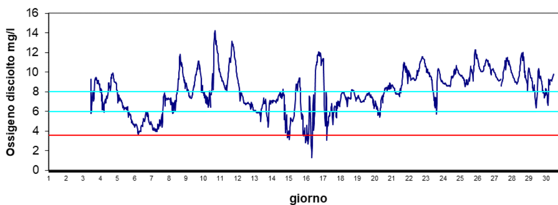
Stazione Scardovari interno Settembre 2024 - Ossigeno disciolto mg/l
