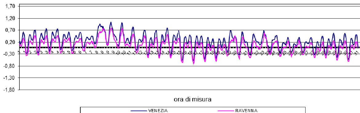
CONFRONTI CICLO di MAREA VENEZIA-RAVENNA DICEMBRE 2024
