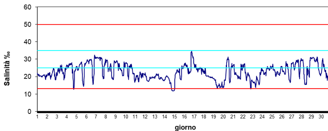
Stazione Barbamarco Aprile 2024 - Salinità ‰
