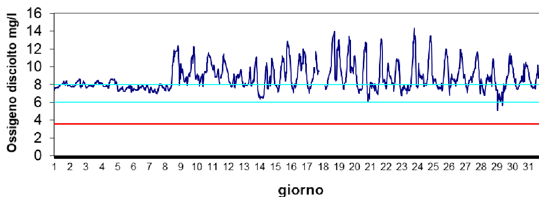
Stazione Basson Agosto 2024 - Ossigeno disciolto mg/l
