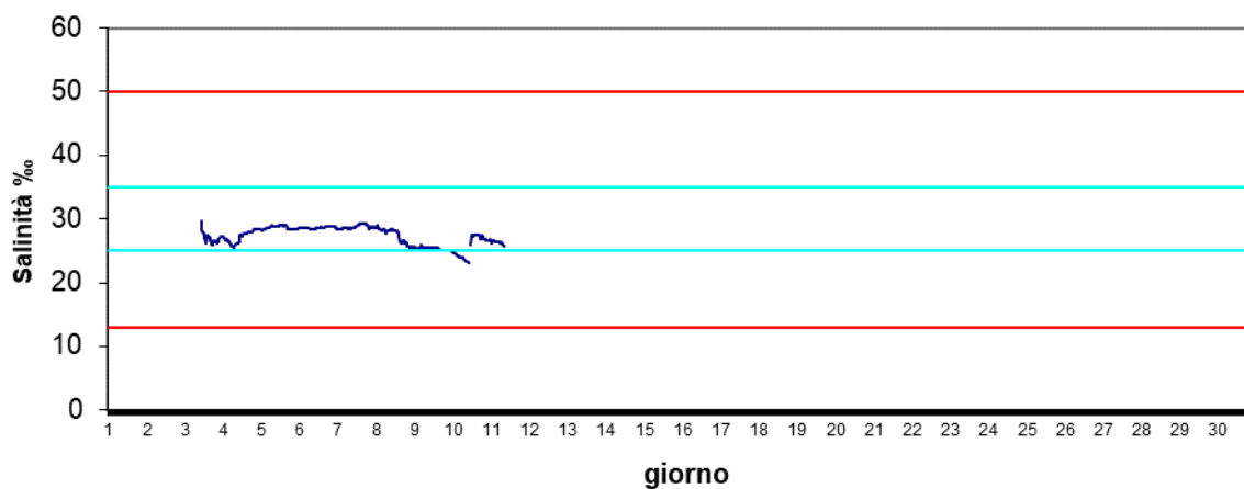
Stazione Scardovari interno Settembre 2024 - Salinità ‰
