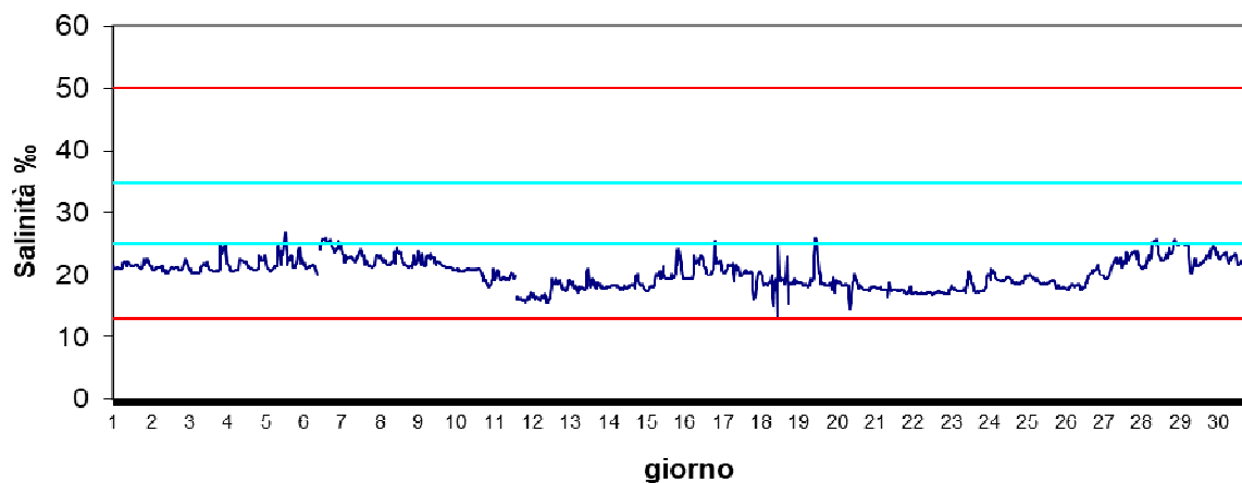
Stazione Vallona Settembre 2024 - Salinità ‰
