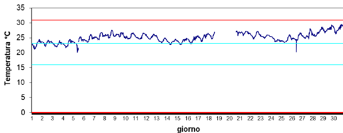
Stazione Vallona Giugno 2024 - Temperatura
