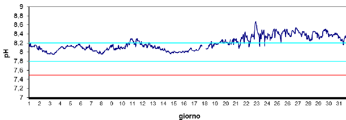
Stazione Basson Marzo 2024 - pH
