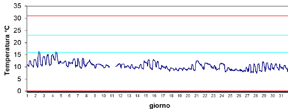
Stazione Scardovari S.Giulia Dicembre 2024 - Temperatura
