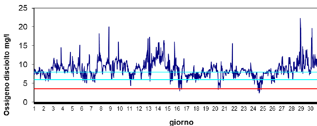
Stazione Barbamarco Aprile 2024 - Ossigeno disciolto mg/l
