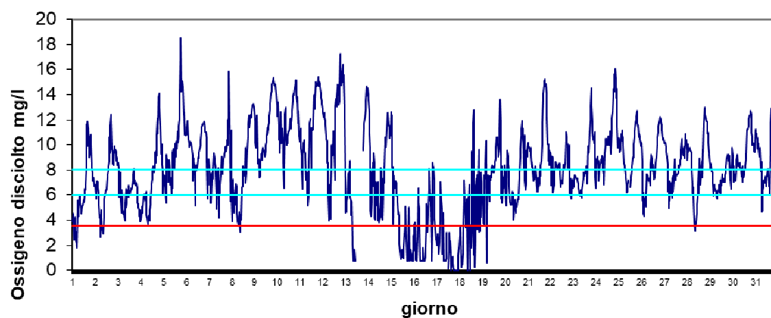
Stazione Barbamarco Luglio 2024 - Ossigeno disciolto mg/l
