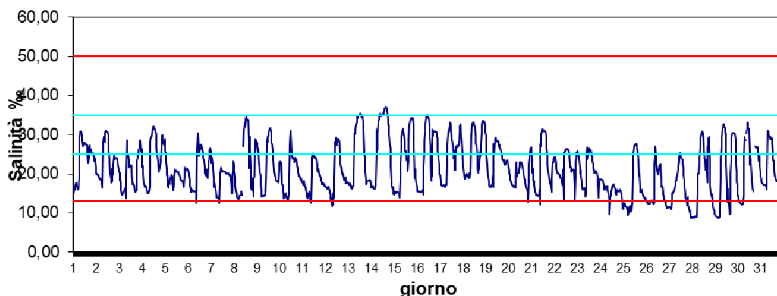
Stazione Basson Settembre 2024 - Salinità ‰
