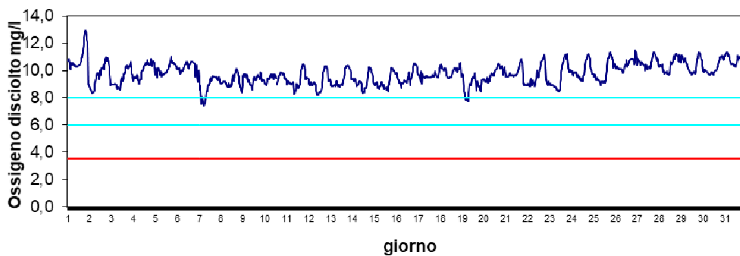
Stazione Scardovari mare Febbraio 2024 - Ossigeno disciolto mg/l
