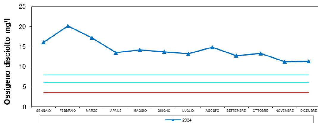
Scardovari S. Giulia - confronto Ossigeno disciolto mg/L MASSIMA 2024
