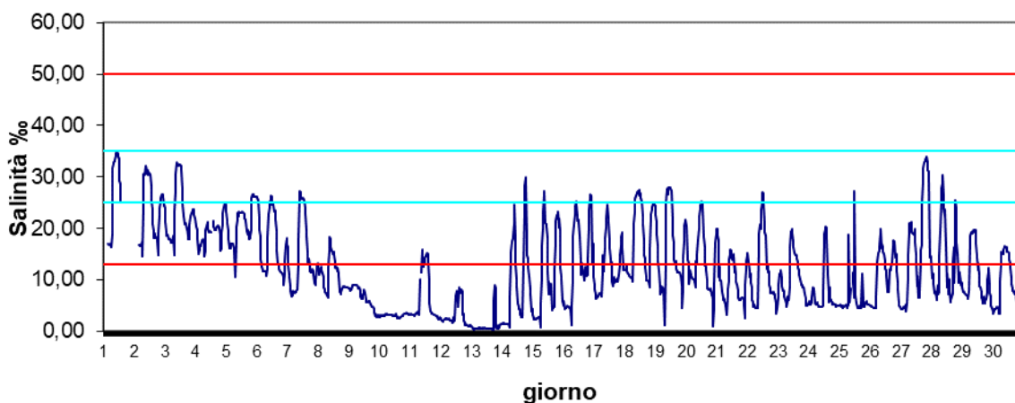
Stazione Basson Settembre 2024 - Salinità ‰
