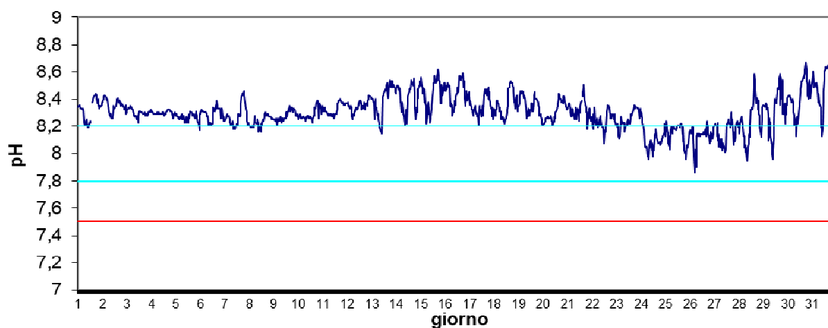
Stazione Vallona Ottobre 2024 - pH
