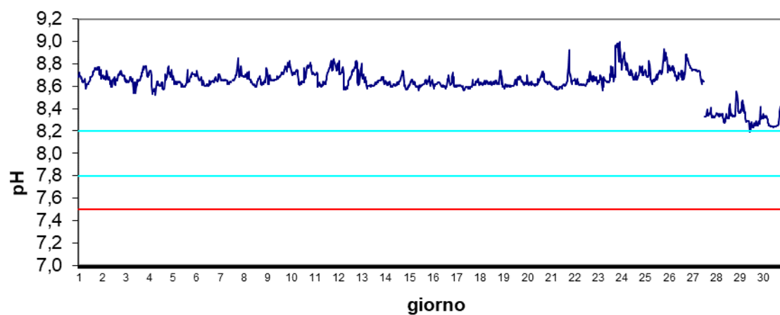
Stazione Barbamarco Novembre 2024 - pH
