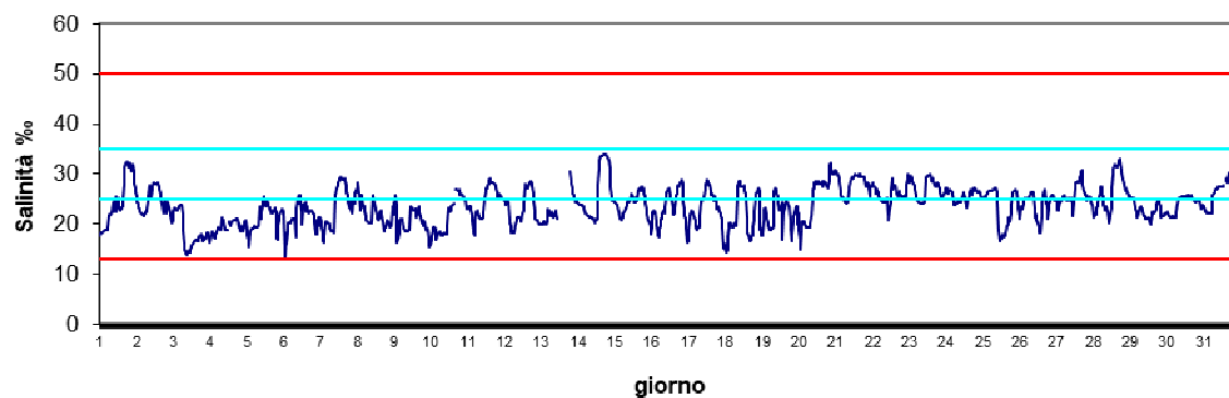
Stazione Scardovari mare Agosto 2024 - Salinità ‰
