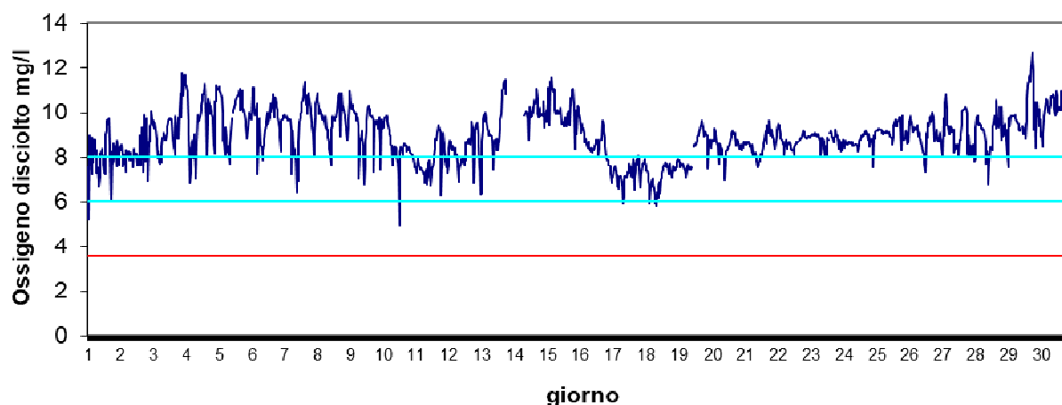
Stazione Vallona Aprile 2024 - Ossigeno disciolto mg/l
