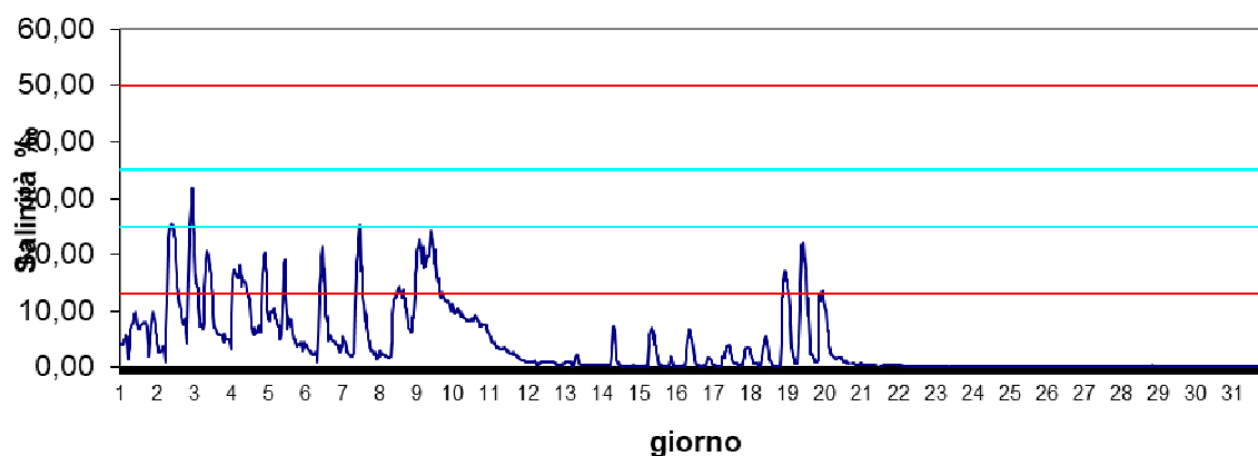
Stazione Basson Novembre 2024 - Salinità ‰
