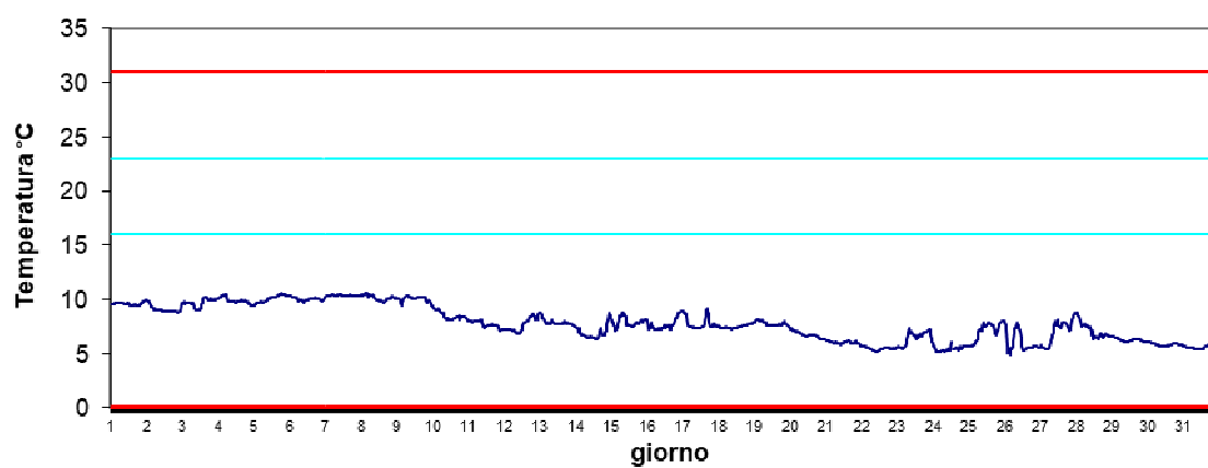
Stazione Scardovari interno Febbraio 2024 - Temperatura
