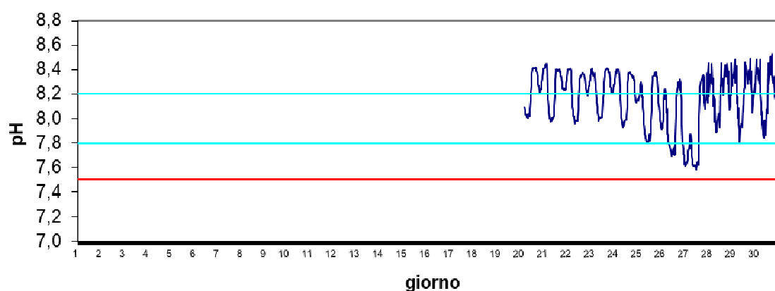
Stazione Marinetta Giugno 2024 - pH
