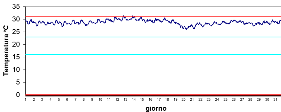
Stazione Marinetta Settembre 2024 - Temperatura
