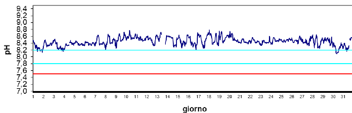
Stazione Scardovari mare Agosto 2024 - pH
