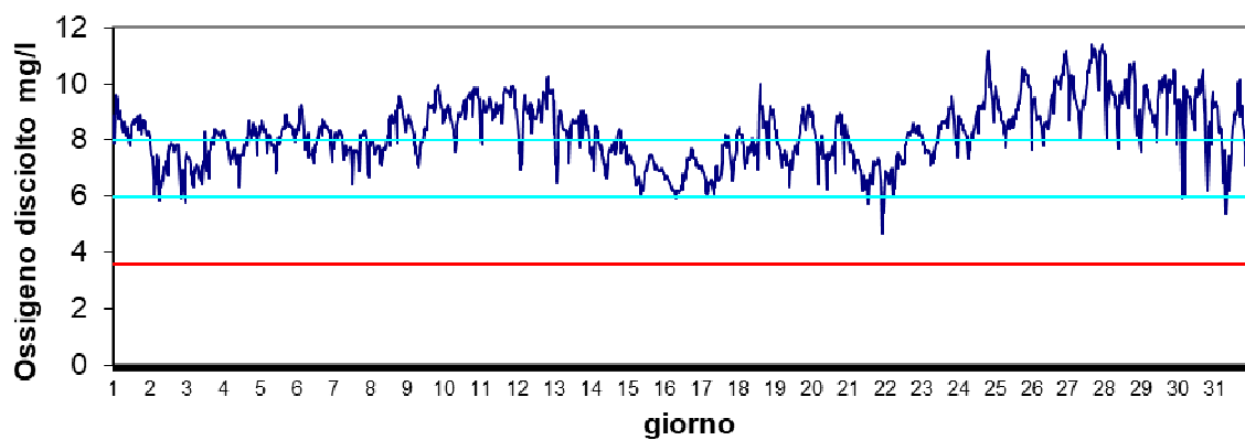
Stazione Caleri Giugno 2024 - Ossigeno disciolto mg/l
