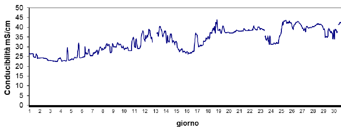
Stazione Scardovari interno Maggio 2024 - Conducibilità mS/cm
