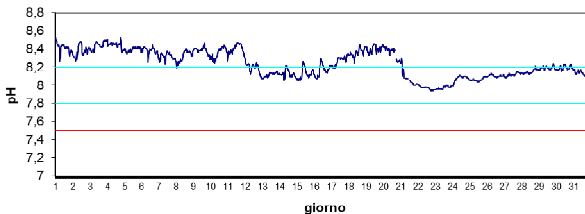
Stazione Basson Novembre 2024 - pH
