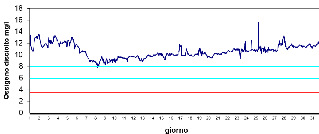
Stazione Scardovari interno Febbraio 2024 - Ossigeno disciolto mg/l
