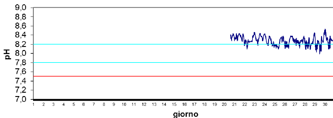
Stazione Canarin Luglio 2024 - pH
