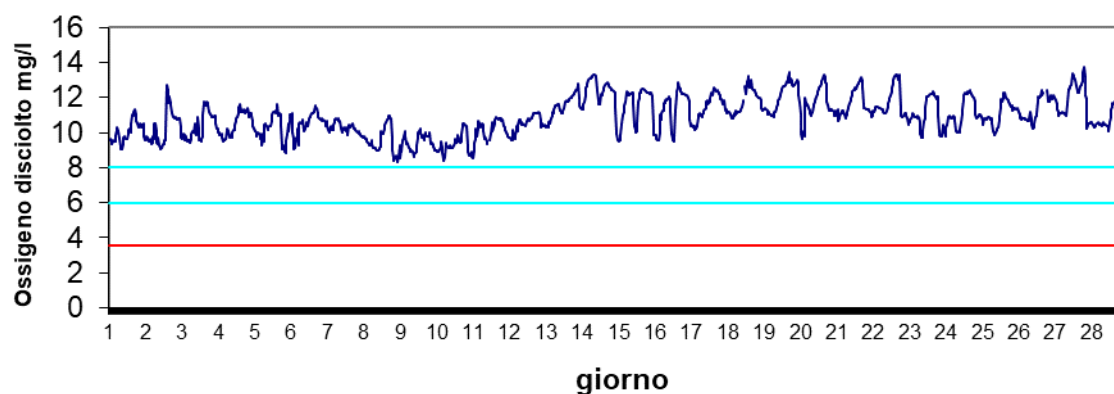
Stazione Basson Marzo 2024 - Ossigeno disciolto mg/l
