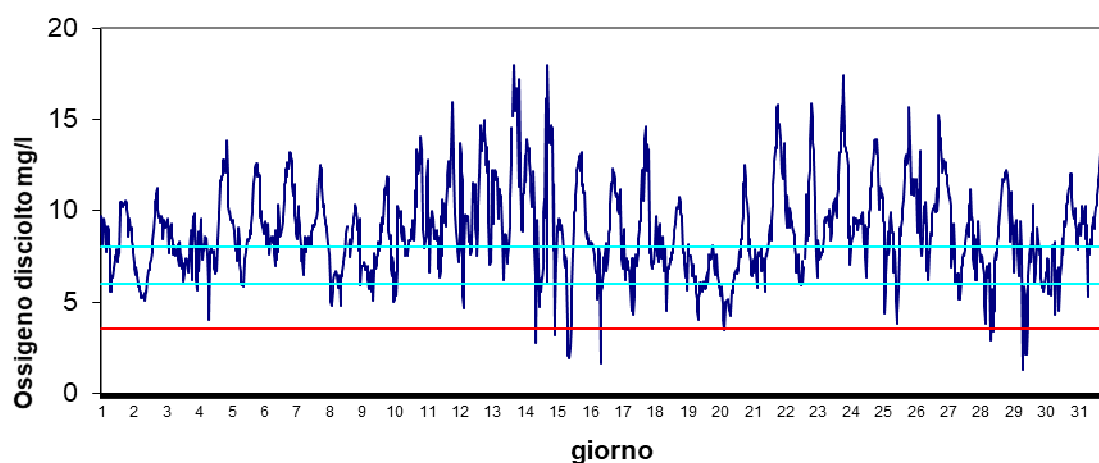
Stazione Barbamarco Agosto 2024 - Ossigeno disciolto mg/l
