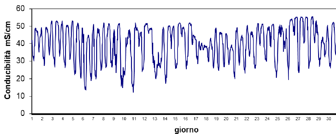
Stazione Marinetta Ottobre 2024 - Conducibilità mS/cm
