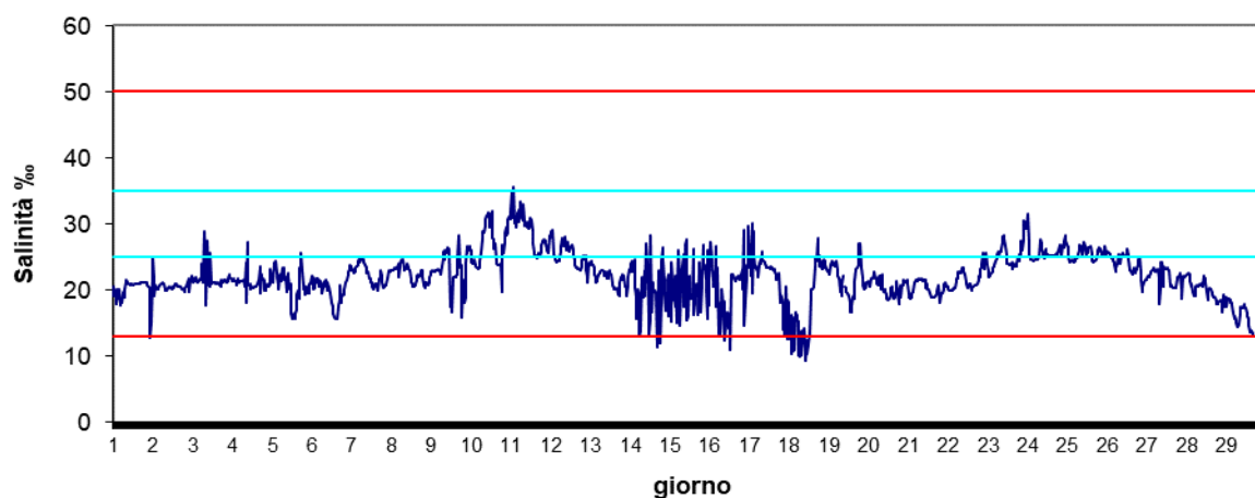
Stazione Vallona Marzo 2024 - Salinità ‰
