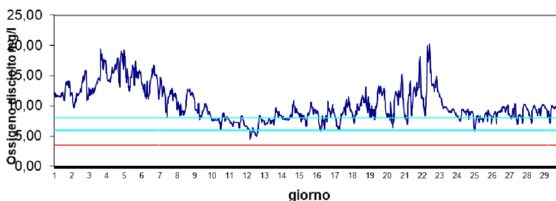
Stazione Scardovari S.Giulia Marzo 2024 - Ossigeno disciolto mg/l
