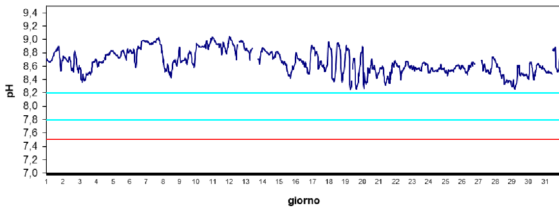
Stazione Scardovari interno Luglio 2024 - pH
