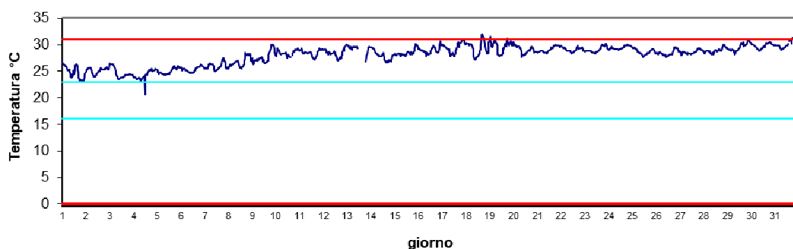
Stazione Scardovari mare Agosto 2024 - Temperatura
