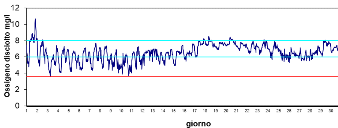
Stazione Marinetta Settembre 2024 - Ossigeno disciolto mg/l
