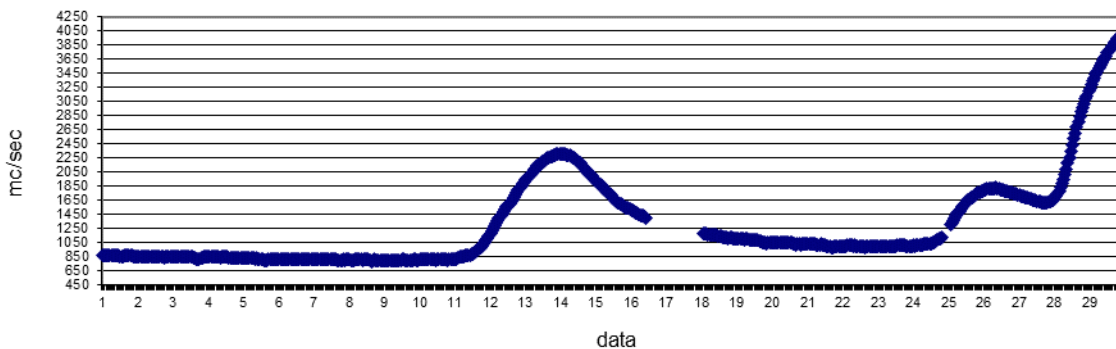
PORTATA PONTELAGOSCURO mc/sec FEBBRAIO 2024
