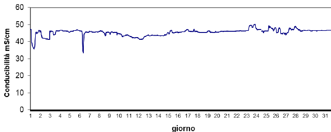
Stazione Scardovari interno Febbraio 2024 - Conducibilità mS/cm
