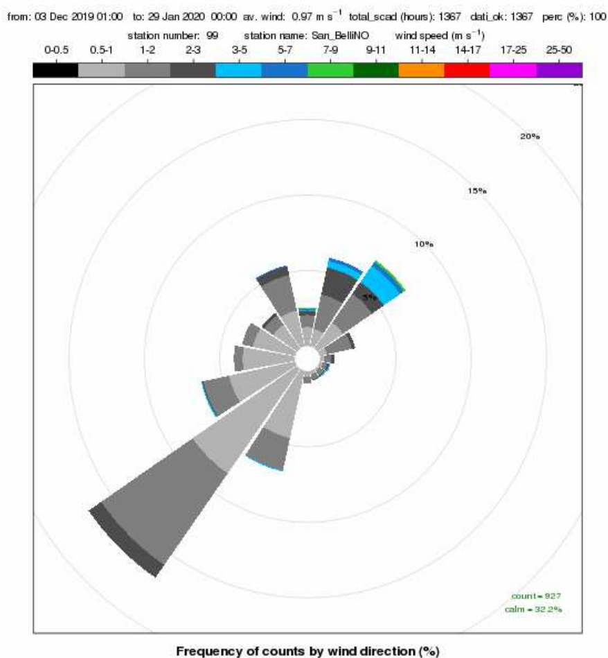
Figura 4: rosa dei venti registrati presso la stazione meteorologica di San Bellino nel periodo 3 dicembre 2019 – 28 gennaio 2020
