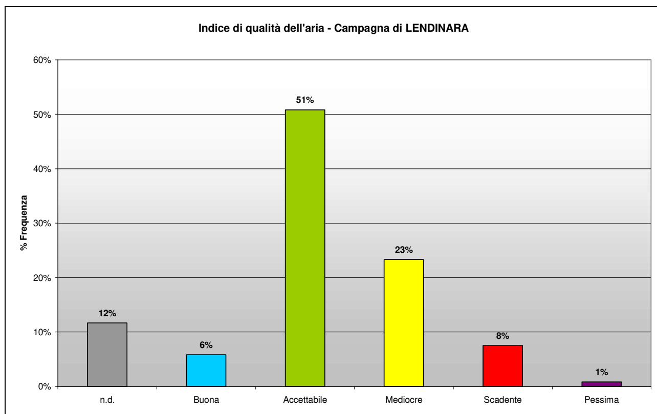
Figura 7. Calcolo dell'indice sintetico di qualità dell'aria per la campagna di Lendinara
