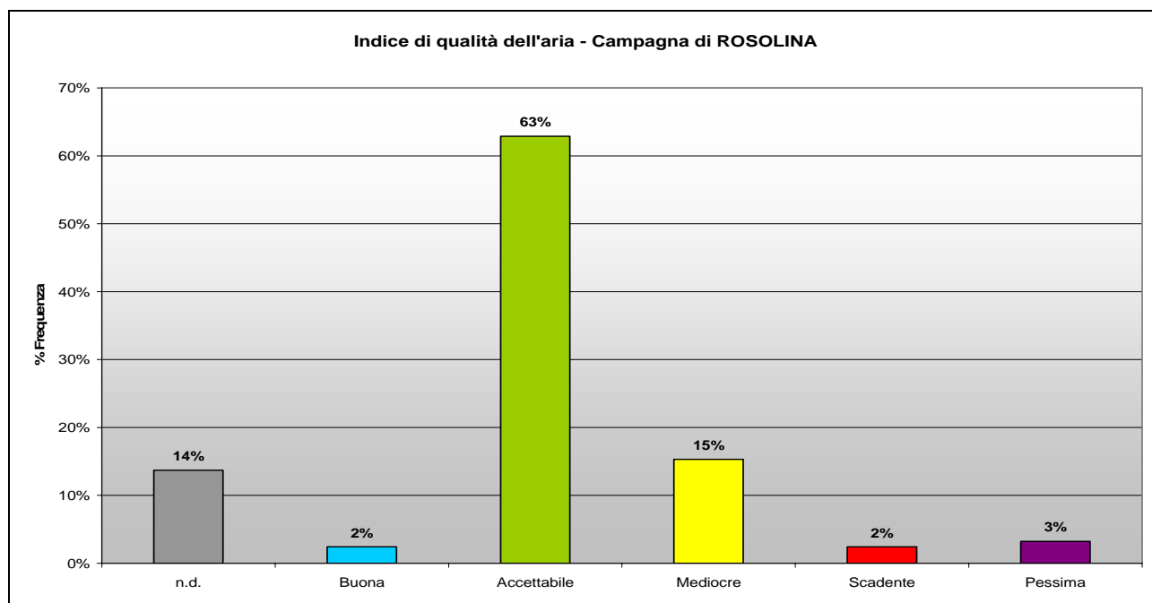
Figura 7. Calcolo dell'indice sintetico di qualità dell'aria per la campagna di Rosolina
