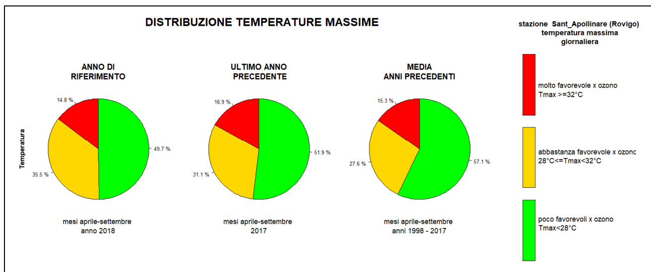
Figura 7: confronto della distribuzione delle temperature massime, rilevate presso la stazione di Sant'Apollinare, nelle tre classi di dispersione, relativamente ai mesi più critici per l'inquinamento da ozono (aprile, maggio, giugno, luglio, agosto, settembre), dell'anno 2018 con quella dell'ultimo anno precedente (2017) e con la media degli anni precedenti (anni 1998-2017).
