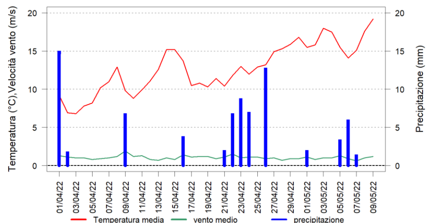
Andamento giornaliero dei parametri meteorologici a Castelfranco Veneto Periodo: 01/04/2022 - 09/05/2022
