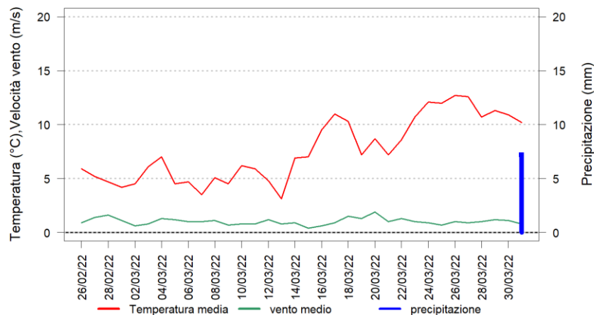
Andamento giornaliero dei parametri meteorologici a Castelfranco Veneto Periodo: 26/02/2022 - 31/03/2022
