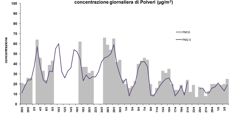
concentrazione giornaliera di Polveri (µg/m 3 )
