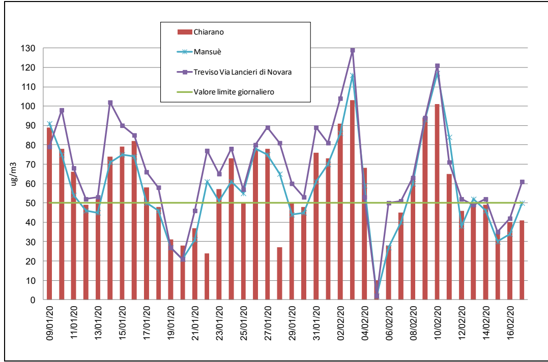
Grafico 1 – Concentrazione Giornaliera di PM10 ( \mu\text{g}/\text{m}^3 ). Campagna invernale
