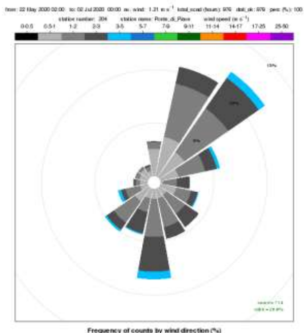
Figura 6: rosa dei venti registrati presso la stazione meteorologica di Ponte di Piave nel periodo 22 maggio – 1 luglio 2020
