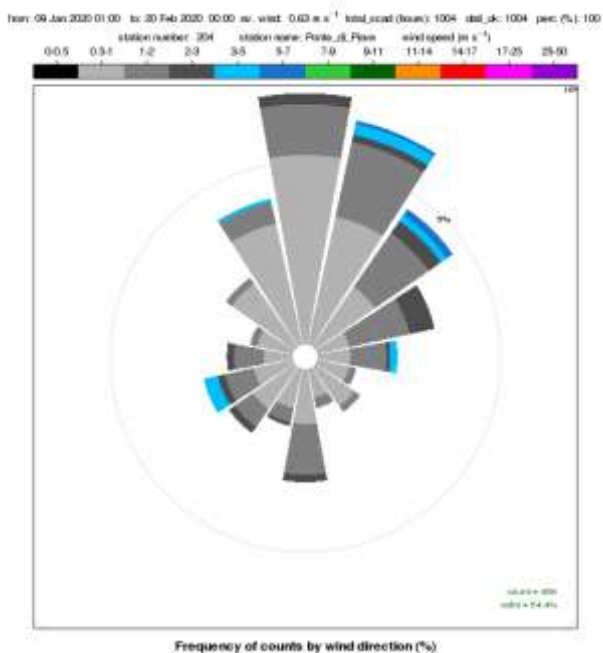
Figura 4: rosa dei venti registrati presso la stazione meteorologica di Ponte di Piave nel periodo 9 gennaio – 19 febbraio 2020
