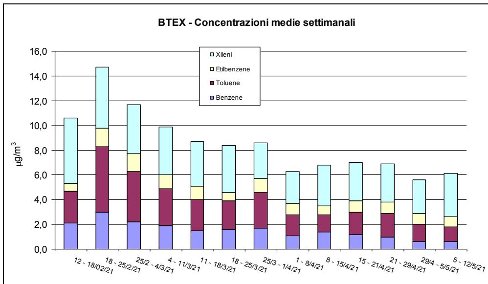
Grafico 2 - Valori settimanali di Benzene, Toluene, Etilbenzene e Xileni rilevati a Cimadolmo
