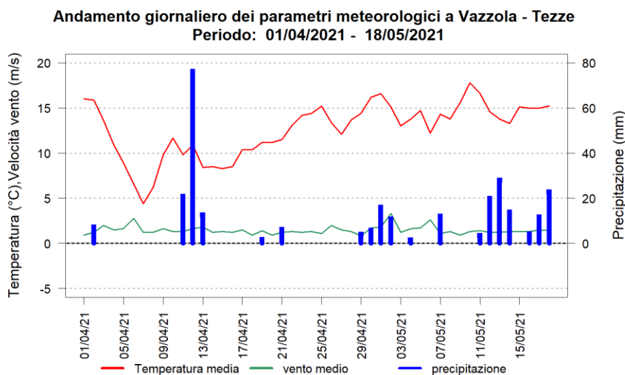
Figura 4. andamento delle precipitazioni, intensità del vento e temperatura media giornaliera rilevati presso la stazione di Vazzola durante la campagna estiva
