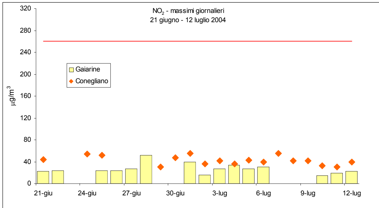
Figura 4 –Valori massimi di biossido di azoto NO 2 rilevati presso la stazione fissa di Conegliano e il Laboratorio Mobile posizionato a Gaiarine
