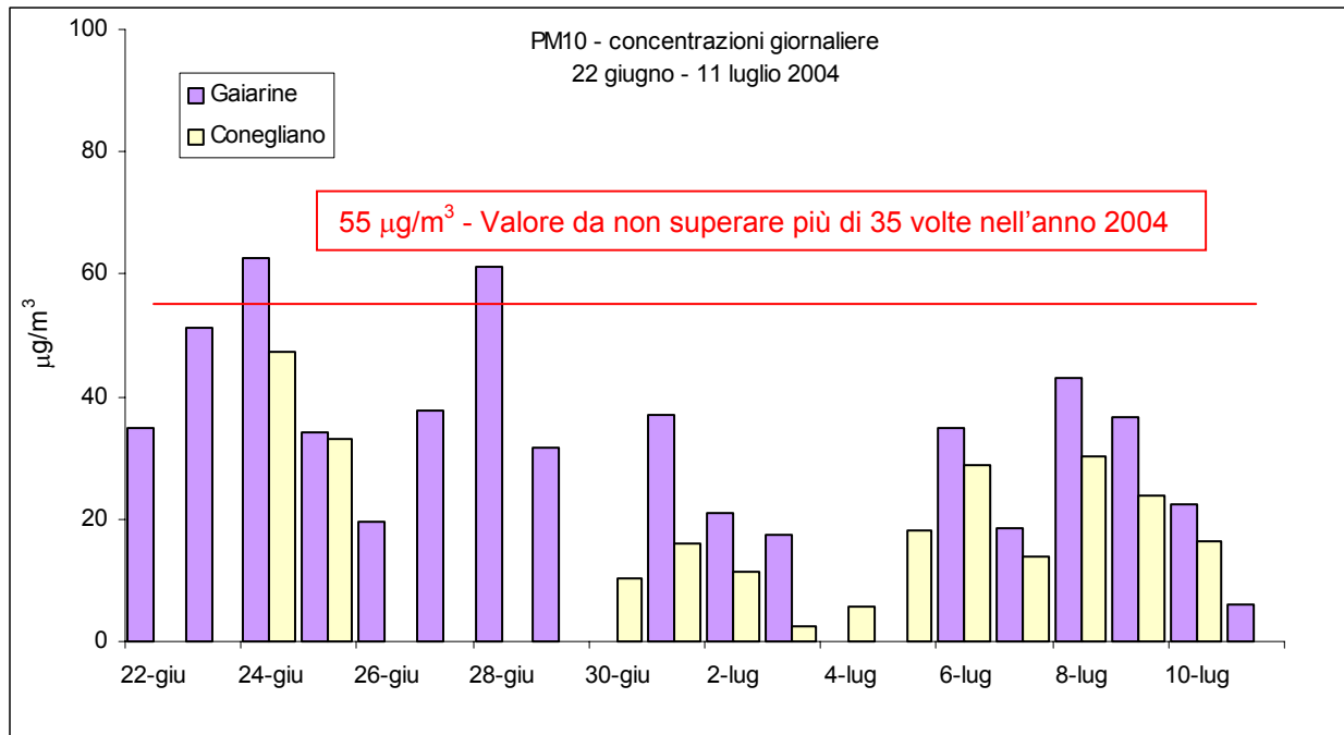
Figura 6 –Valori massimi di polveri inalabili PM10 rilevati presso la stazione fissa di Conegliano e il Laboratorio Mobile posizionato a Gaiarine
