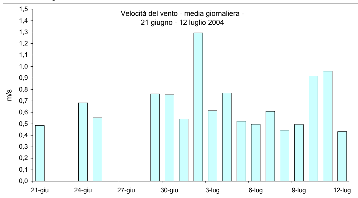
Figura 8 – Valori medi giornalieri della velocità del vento rilevati presso la stazione di Conegliano.
