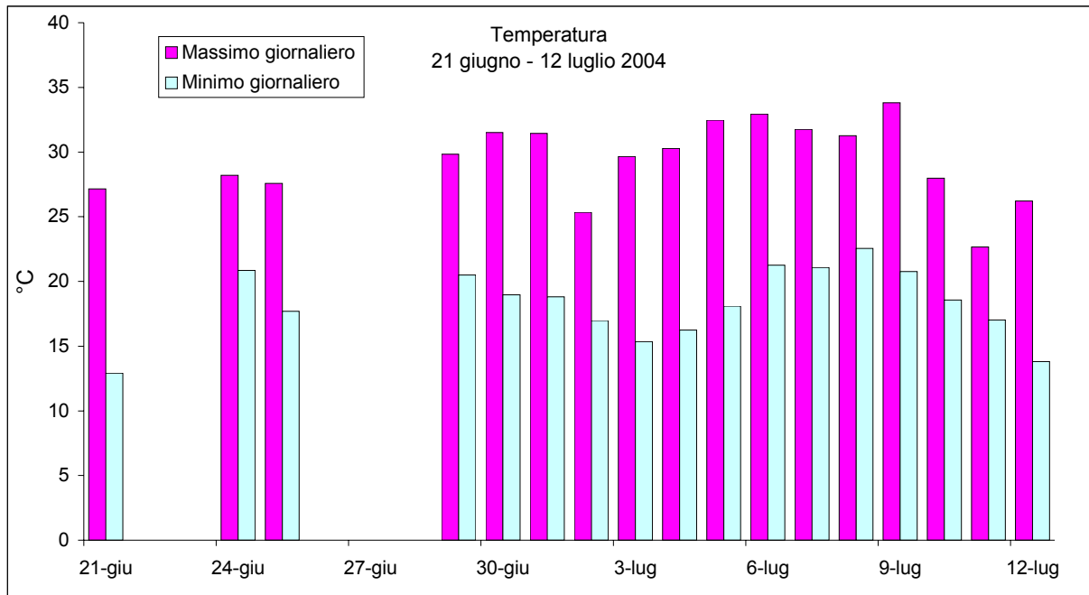
Figura 9 – Valori minimi e massimi di Temperatura rilevati presso la stazione di Conegliano.
