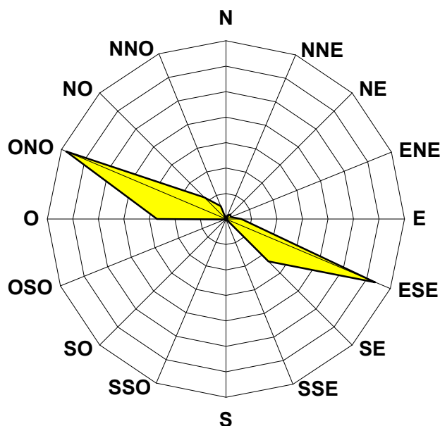
Figura 7 – Direzione del vento- numero di eventi osservati durante la campagna di rilevamento presso la stazione di Conegliano.
