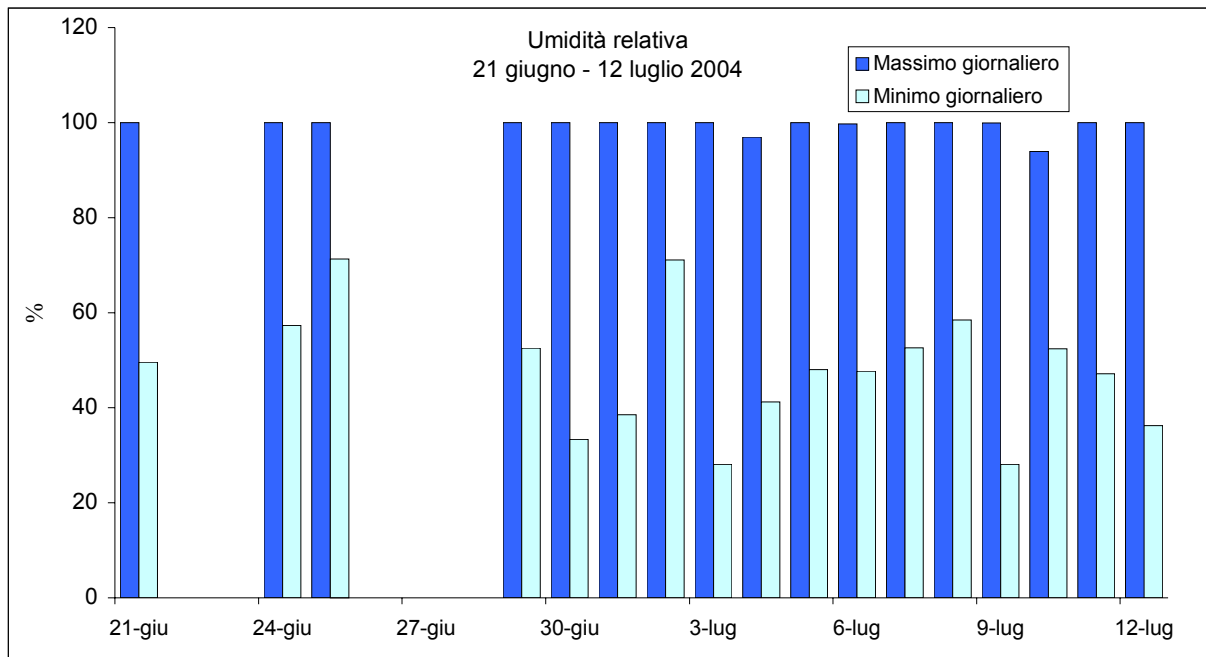
Figura 10 – Valori medi giornalieri di umidità % relativa rilevata presso la stazione di Conegliano.
