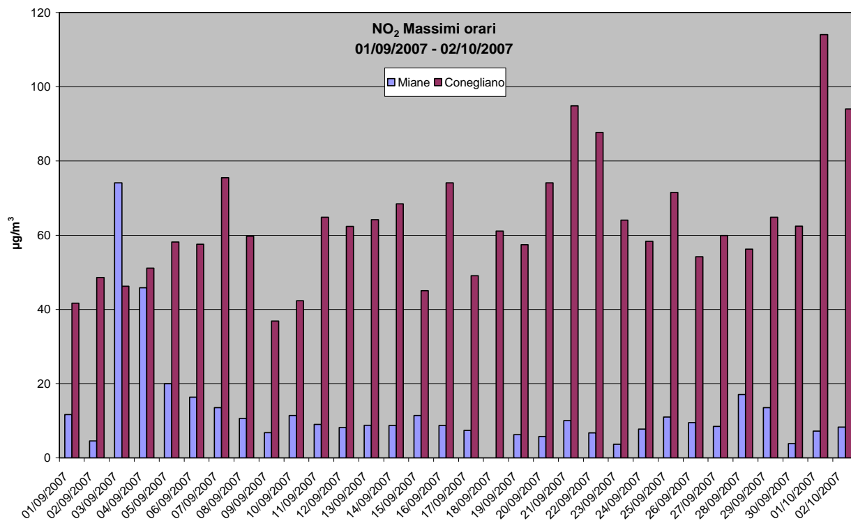
Grafico 2: Valori massimi orari di NO 2 rilevati presso la stazione fissa di Conegliano e la stazione rilocabile posizionata a Miane – campagna estiva
