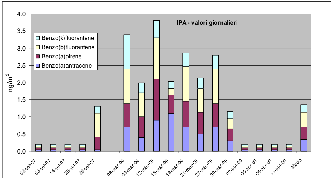
Grafico 12 Valori giornalieri di IPA (Benzo(a)pirene, Benzo(b)fluorantene, Benzo(k)fluorantene, Benzo(a)antracene) rilevati a Miane
