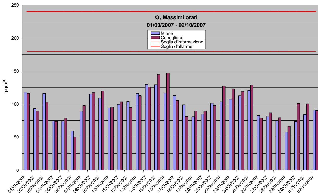
Grafico 3: Valori massimi orari di O 3 rilevati presso la stazione fissa di Conegliano e la stazione rilocabile posizionata a Miane – campagna estiva
