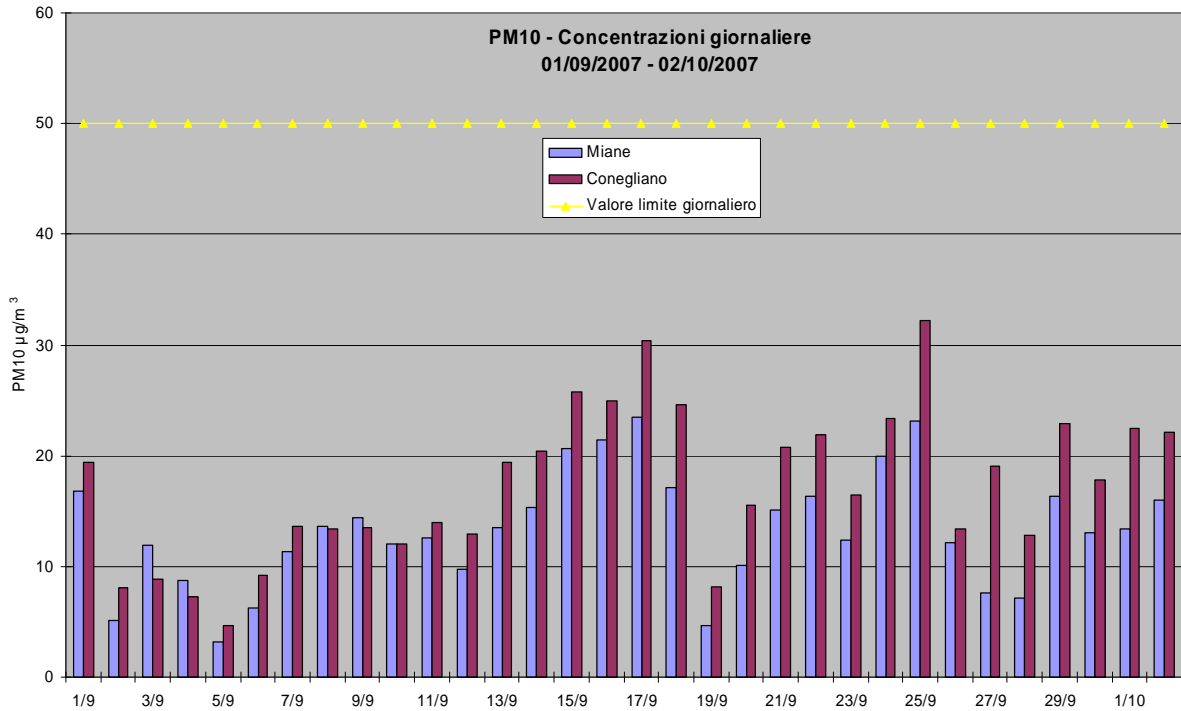
Grafico 5: Valori medi giornalieri di PM10 rilevati presso la stazione fissa di Conegliano e la stazione rilocabile posizionata a Miane – campagna estiva
