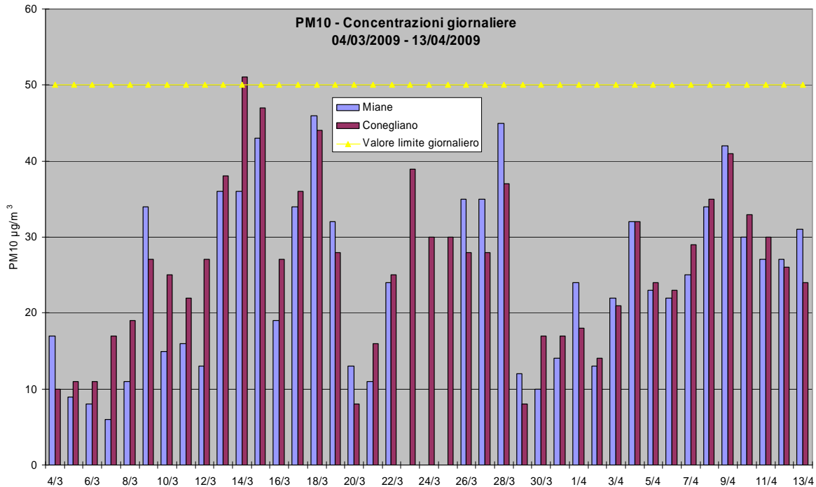
Grafico 6: Valori medi giornalieri di PM10 rilevati presso la stazione fissa di Conegliano ed il campionatore portatile posizionato a Miane – campagna invernale
