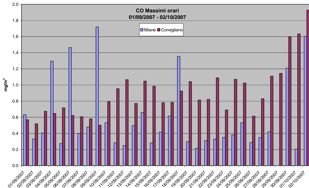
Grafico 1: Valori massimi orari di CO rilevati presso la stazione fissa di Conegliano e la stazione rilocabile posizionata a Miane – campagna estiva
