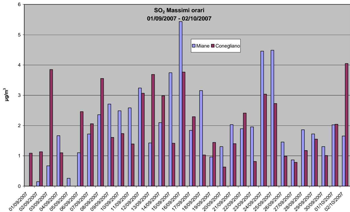
Grafico 4: Valori massimi orari di SO 2 rilevati presso la stazione fissa di Conegliano e la stazione rilocabile posizionata a Miane – campagna estiva
