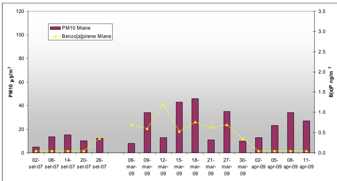
Grafico 13: Andamento del B(a)P e del PM10 rilevati presso la stazione rilocabile.
