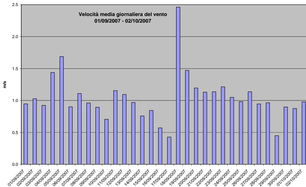
Grafico 8 Valori medi giornalieri di velocità del vento osservati presso la stazione rilocabile posizionata a Miane – campagna estiva.
