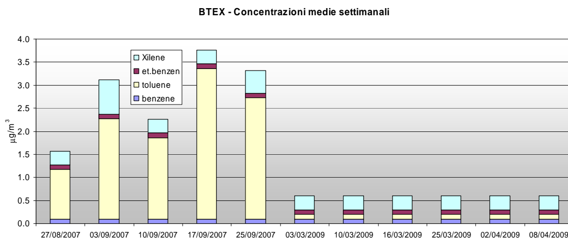
Grafico 7 Valori settimanali di BTEX (Benzene, Toluene, Etilbenzene, Xilene) rilevati a Miane
