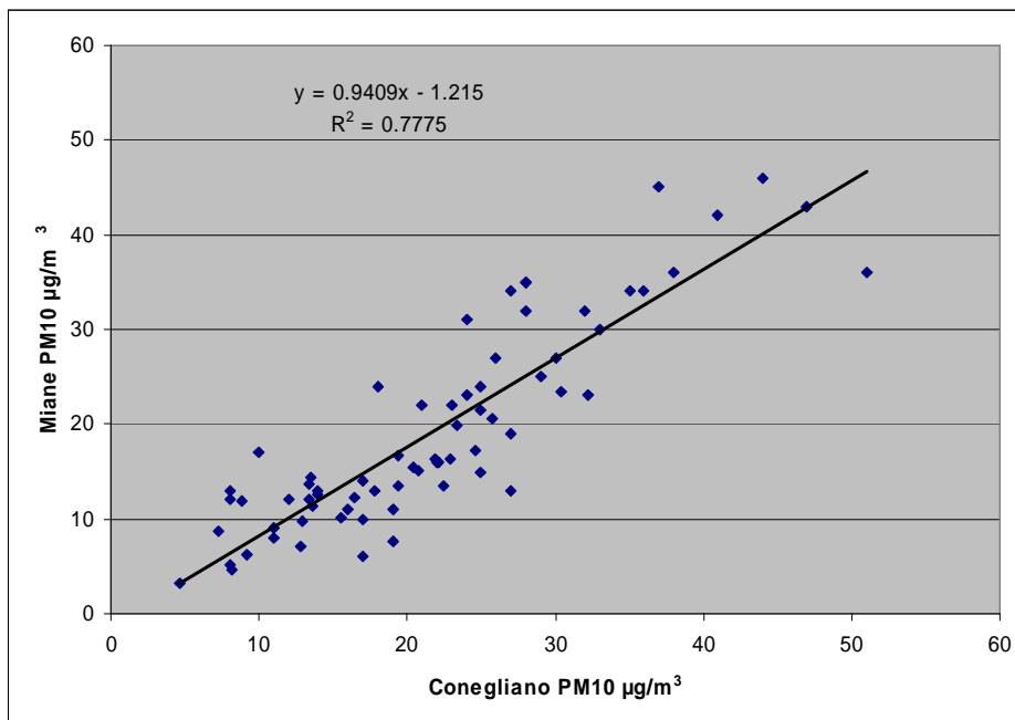
Grafico 14 PM10 - rapporto tra la stazione rilocabile e quella di Conegliano
