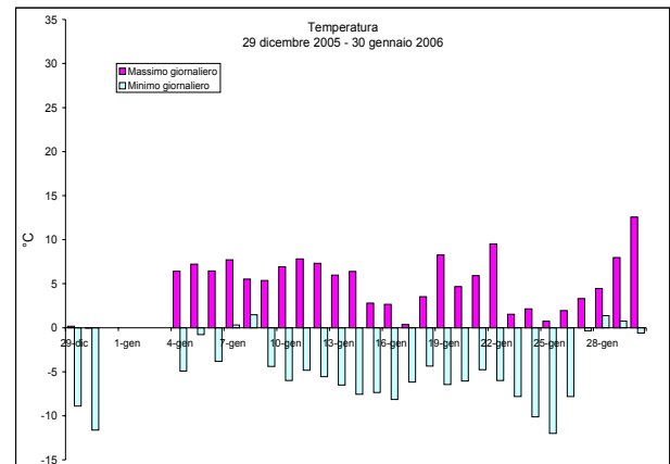
Figura 6b – Valori minimi e massimi di Temperatura osservati presso la stazione rilocabile posizionata a Moriago della Battaglia – campagna invernale.
