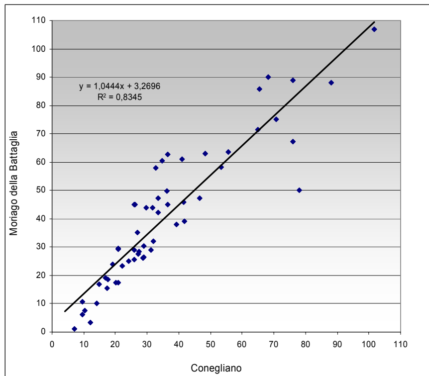
Figura 8 – correlazione tra i valori di PM10 rilevati a Moriago della Battaglia e nel Comune di Conegliano
