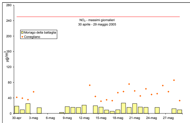
Figura 2a –Valori massimi di NO 2 rilevati presso la stazione fissa di Conegliano e la stazione rilocabile posizionata a Moriago della Battaglia – campagna estiva
