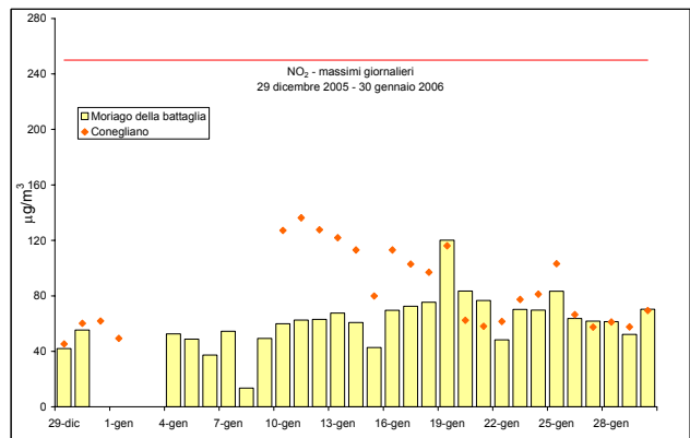
Figura 2b – Valori massimi di NO 2 rilevati presso la stazione fissa di Conegliano e la stazione rilocabile posizionata a Moriago della Battaglia – campagna invernale
