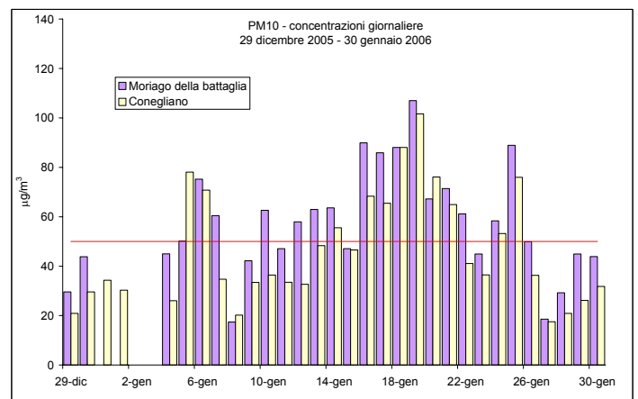
Figura 5b – Valori medi giornalieri di PM10 rilevati presso la stazione fissa di Conegliano e la stazione rilocabile posizionata a Moriago della Battaglia – campagna invernale
