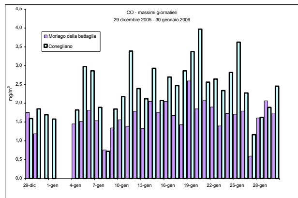
Figura 1b – Valori massimi di CO rilevati presso la stazione fissa di Conegliano e la stazione rilocabile posizionata a Moriago della Battaglia – campagna invernale
