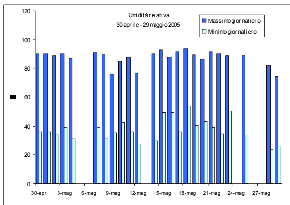
Figura 7a – Valori minimi e massimi giornalieri di Umidità % relativa osservati presso la stazione rilocabile posizionata a Moriago della Battaglia – campagna estiva.
