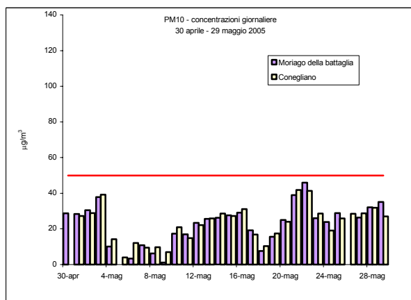
Figura 5a – Valori medi giornalieri di PM10 rilevati presso la stazione fissa di Conegliano e la stazione rilocabile posizionata a Moriago della Battaglia – campagna estiva
