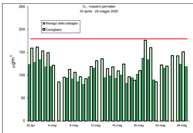
Figura 3a –Valori massimi di O 3 rilevati presso la stazione fissa di Conegliano e la stazione rilocabile posizionata a Moriago della Battaglia – campagna estiva
