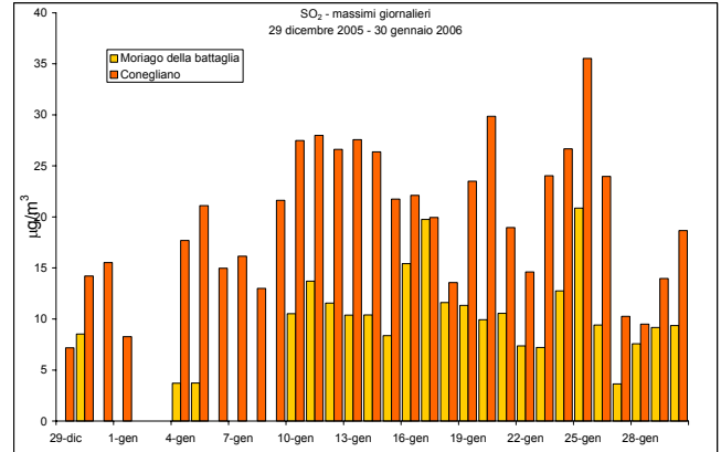
Figura 4b –Valori massimi di SO 2 rilevati presso la stazione fissa di Conegliano e la stazione rilocabile posizionata a Moriago della Battaglia – campagna invernale
