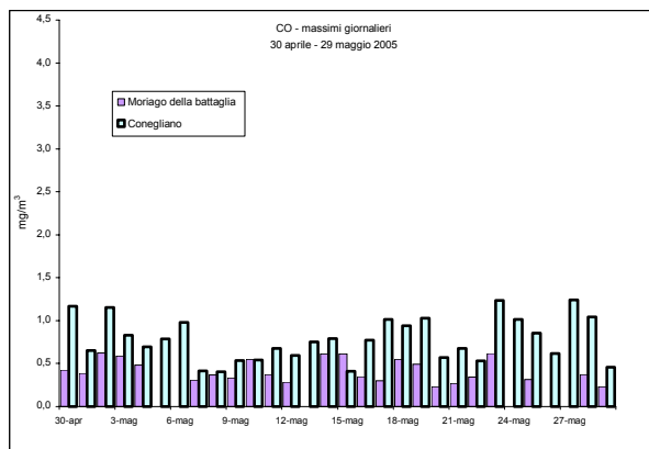
Figura 1a –Valori massimi di CO rilevati presso la stazione fissa di Conegliano e la stazione rilocabile posizionata a Moriago della Battaglia – campagna estiva
