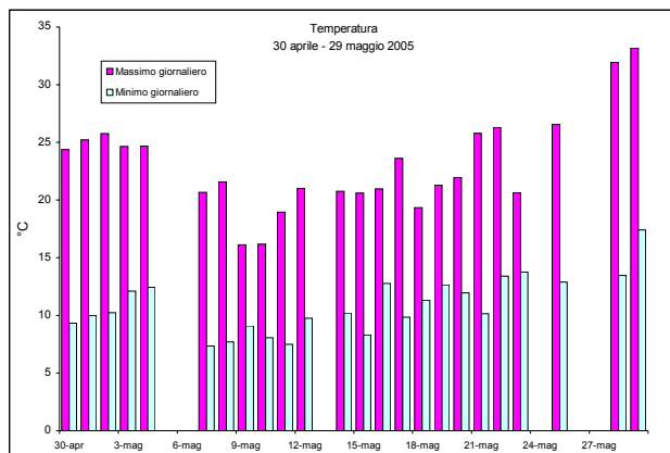
Figura 6a – Valori minimi e massimi di Temperatura osservati presso la stazione rilocabile posizionata a Moriago della Battaglia – campagna estiva.
