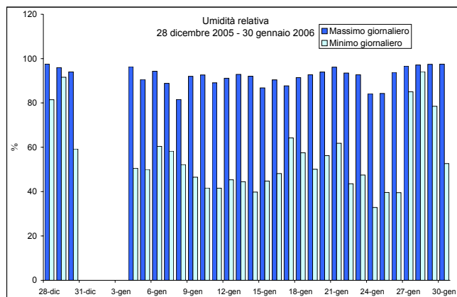
Figura 7b – Valori minimi e massimi giornalieri di Umidità % relativa osservati presso la stazione rilocabile posizionata a Moriago della Battaglia – campagna invernale.
