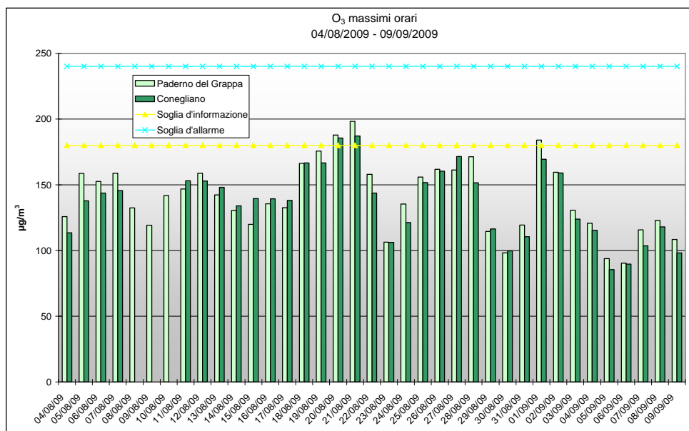
Grafico 5: Valori massimi orari di O 3 rilevati presso la stazione fissa di Conegliano e la stazione rilocabile posizionata a Paderno del Grappa – campagna estiva
