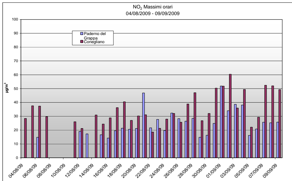
Grafico 3: Valori massimi orari di \text{NO}_2 rilevati presso la stazione fissa di Conegliano e la stazione rilocabile posizionata a Paderno del Grappa – campagna estiva
