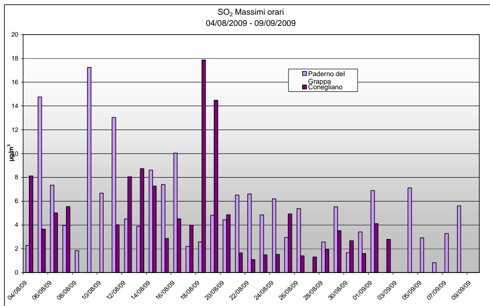
Grafico 7: Valori massimi orari di SO 2 rilevati presso la stazione fissa di Conegliano e la stazione rilocabile posiziona a Paderno del Grappa – campagna estiva
