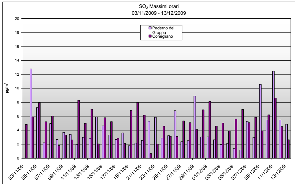
Grafico 8: Valori massimi orari di SO 2 rilevati presso la stazione fissa di Conegliano e la stazione rilocabile posizionata a Paderno del Grappa – campagna invernale
