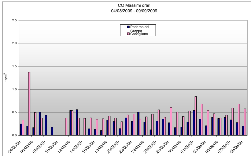
Grafico 1: Valori massimi orari di CO rilevati presso la stazione fissa di Conegliano e la stazione rilocabile posizionata a Paderno del Grappa – campagna estiva
