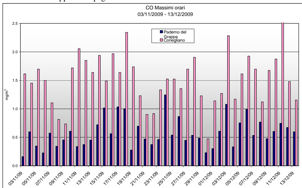
Grafico 2: Valori massimi orari di CO rilevati presso la stazione fissa di Conegliano e la stazione rilocabile posizionata a Paderno del Grappa – campagna invernale
