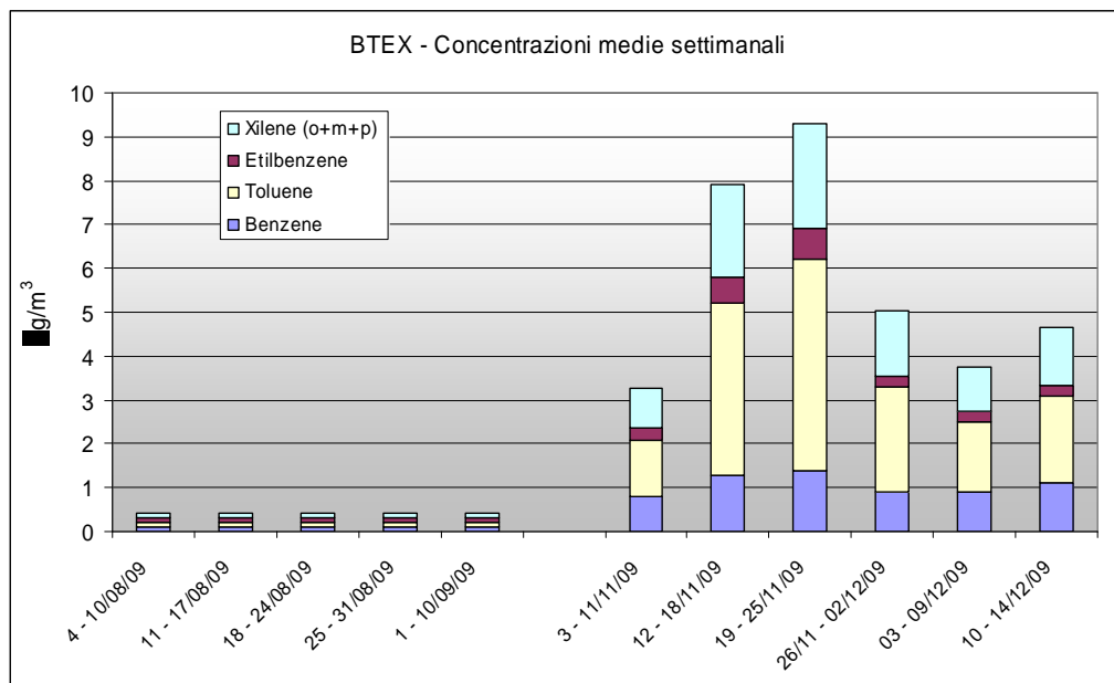
Grafico 11: Valori settimanali di BTEX (Benzene, Toluene, Etilbenzene, Xilene) rilevati a Paderno del Grappa
