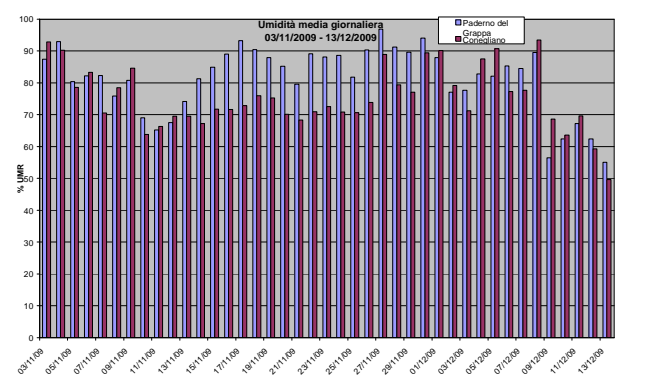
Grafico 19: Valori medi giornalieri di umidità osservati presso la stazione fissa di Conegliano e la stazione rilocabile posizionata a Paderno del Grappa – campagna invernale
