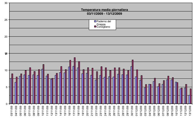
Grafico 17: Valori medi giornalieri di temperatura osservati presso la stazione fissa di Conegliano e la stazione rilocabile posizionata a Paderno del Grappa – campagna invernale
