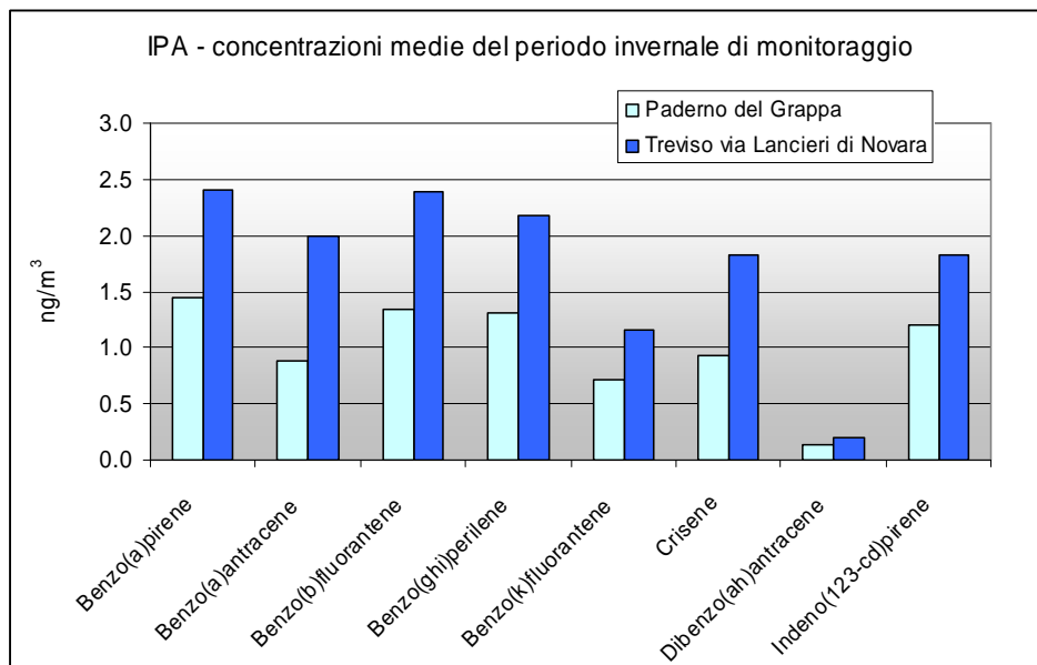
Grafico 21: Confronto tra i valori di IPA determinati su campioni di PM10 prelevati nel sito di monitoraggio e presso la stazione fissa di Treviso durante la campagna invernale
