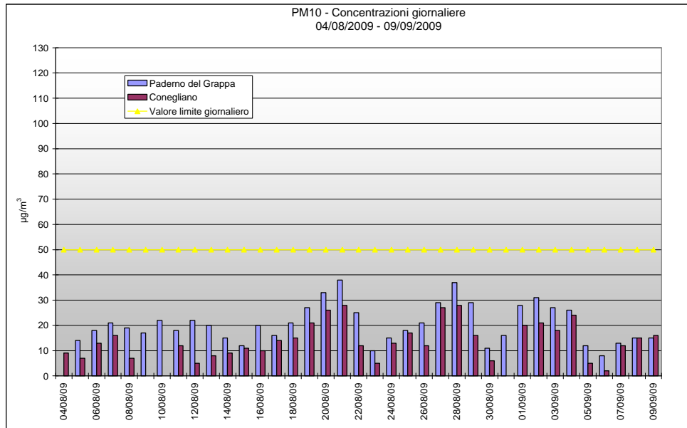
Grafico 9: Valori medi giornalieri di PM10 rilevati presso la stazione fissa di Conegliano e la stazione rilocabile posizionata a Paderno del Grappa – campagna estiva
