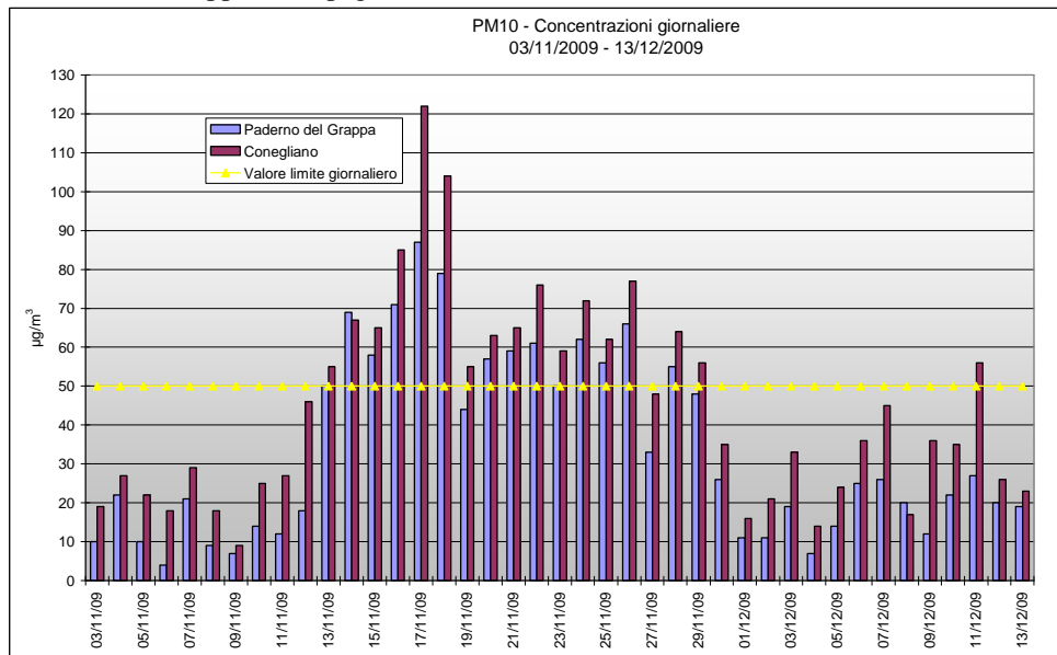
Grafico 10: Valori medi giornalieri di PM10 rilevati presso la stazione fissa di Conegliano e la stazione rilocabile posizionata a Paderno del Grappa – campagna invernale
