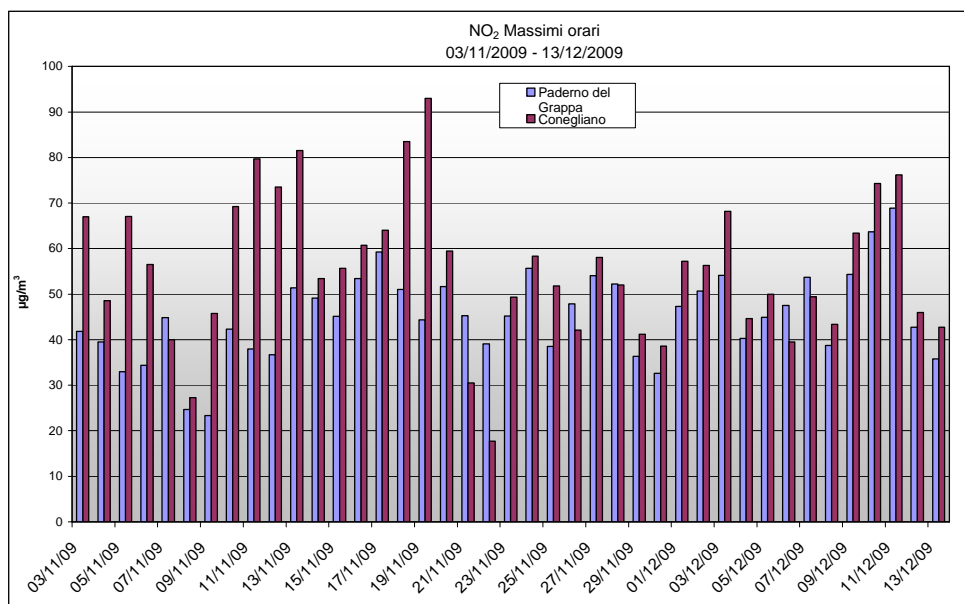
Grafico 4: Valori massimi orari di NO 2 rilevati presso la stazione fissa di Conegliano e la stazione rilocabile posizionata a Paderno del Grappa – campagna invernale
