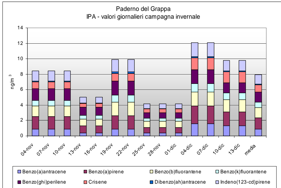
Grafico 20: Valori di IPA rilevati su campioni giornalieri di PM10 prelevati a Paderno del Grappa nel sito di monitoraggio
