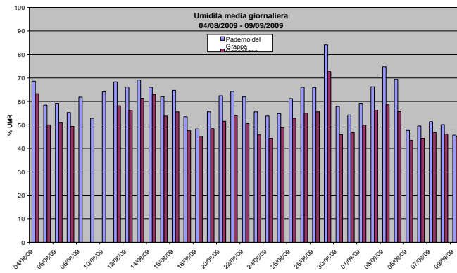
Grafico 18: Valori medi giornalieri di umidità osservati presso la stazione fissa di Conegliano e la stazione rilocabile posizionata a Paderno del Grappa – campagna estiva
