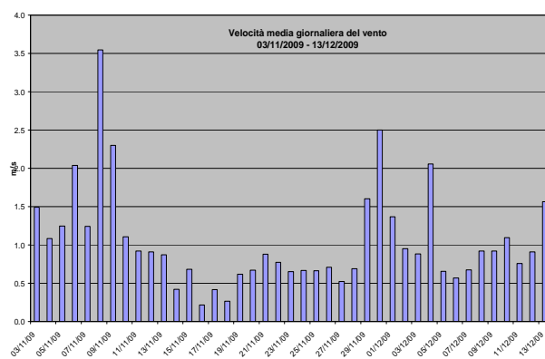
Grafico 13: Valori medi giornalieri di velocità del vento osservati presso la stazione rilocabile posizionata a Paderno del Grappa – campagna invernale
