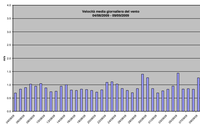
Grafico 12: Valori medi giornalieri di velocità del vento osservati presso la stazione rilocabile posizionata a Paderno del Grappa – campagna estiva
