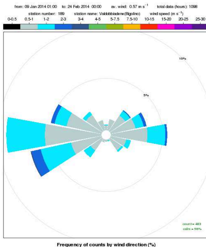
Figura 6. rose dei venti a scansione oraria registrati presso la stazione meteorologica di Valdobbadiene - Bigolino nel periodo 9 gennaio – 23 febbraio 2014.
