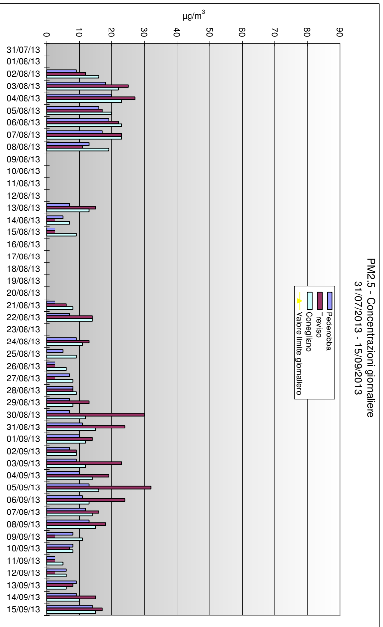
Grafico 8 – Concentrazione Giornaliera di PM 2.5 ( \mu\text{g}/\text{m}^3 ). Semestre “estivo”
