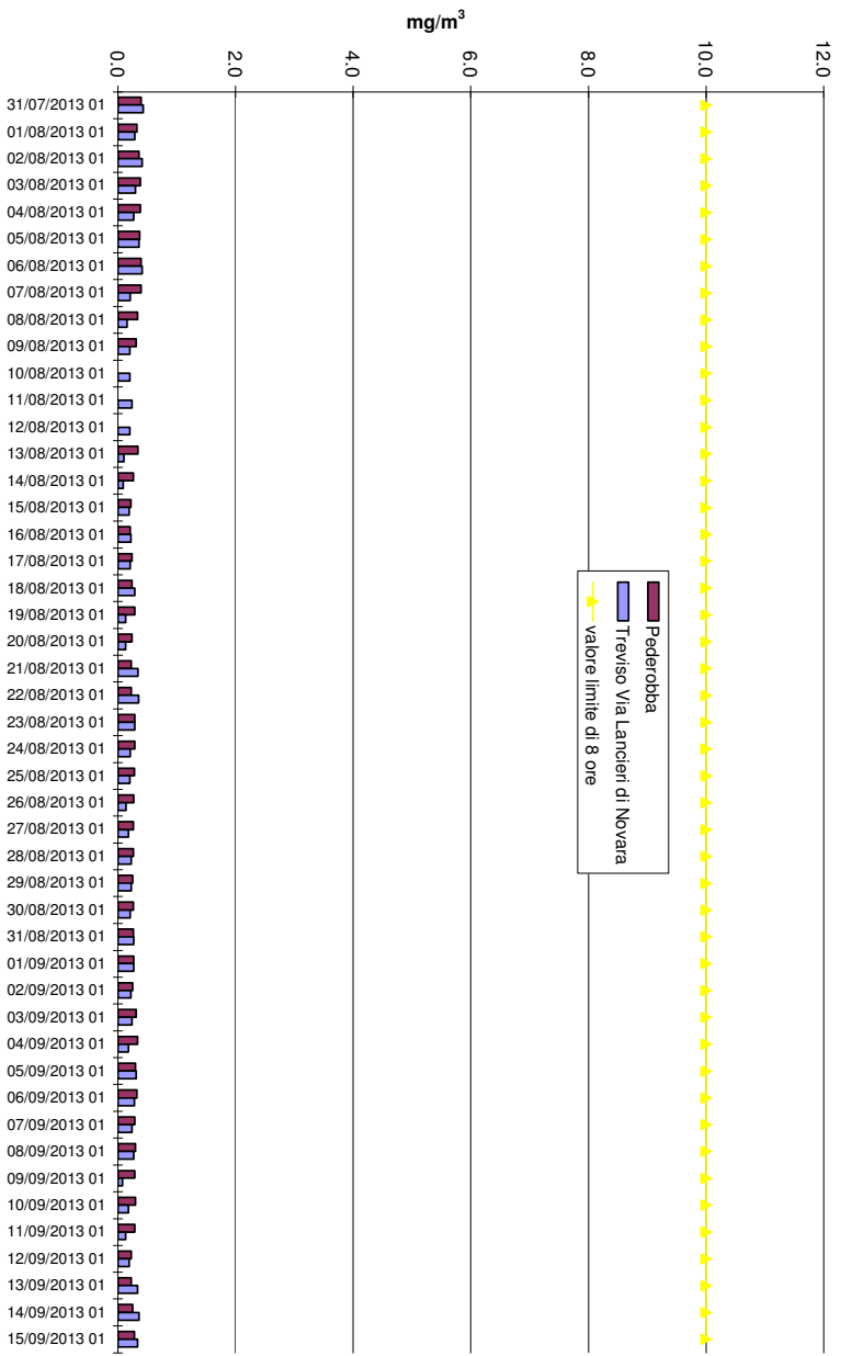
Grafico 1 – Concentrazione Massima Giornaliera della Media Mobile di 8 ore di CO (mg/m 3 ). Semestre “estivo”
