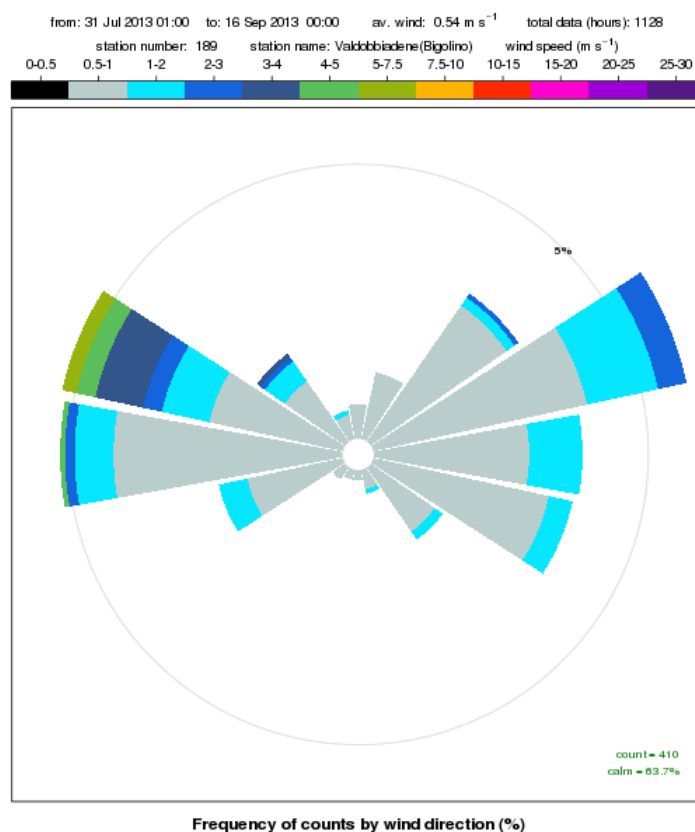
Figura 4. rose dei venti a scansione oraria registrati presso la stazione meteorologica di Valdobbadiene - Bigolino nel periodo 31 luglio – 15 settembre 2013.
