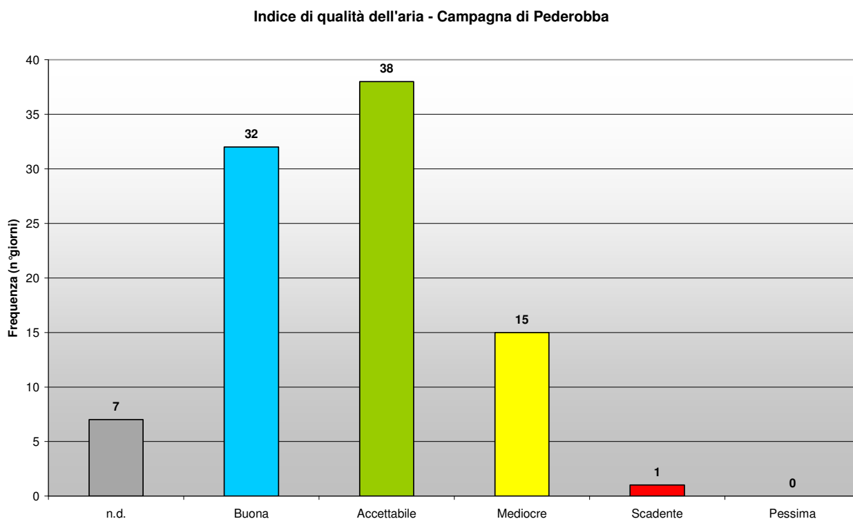
Figura 7. Calcolo dell'indice sintetico di qualità dell'aria per la campagna di Pederobba
