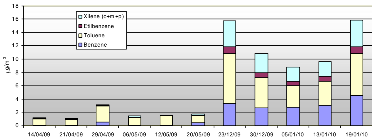
Grafico 11: Valori settimanali di BTEX (Benzene, Toluene, Etilbenzene, Xilene) rilevati a Povegliano
