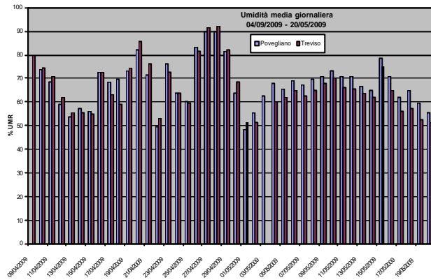
Grafico 18: Valori medi giornalieri di umidità osservati presso la stazione fissa di Treviso e la stazione rilocabile posizionata a Povegliano – campagna estiva
