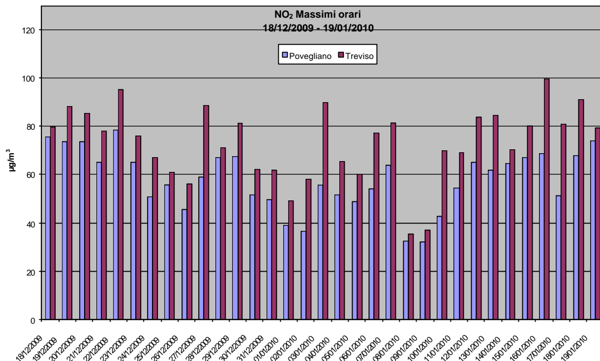
Grafico 4: Valori massimi orari di NO 2 rilevati presso la stazione fissa di Treviso e la stazione rilocabile posizionata a Povegliano – campagna invernale
