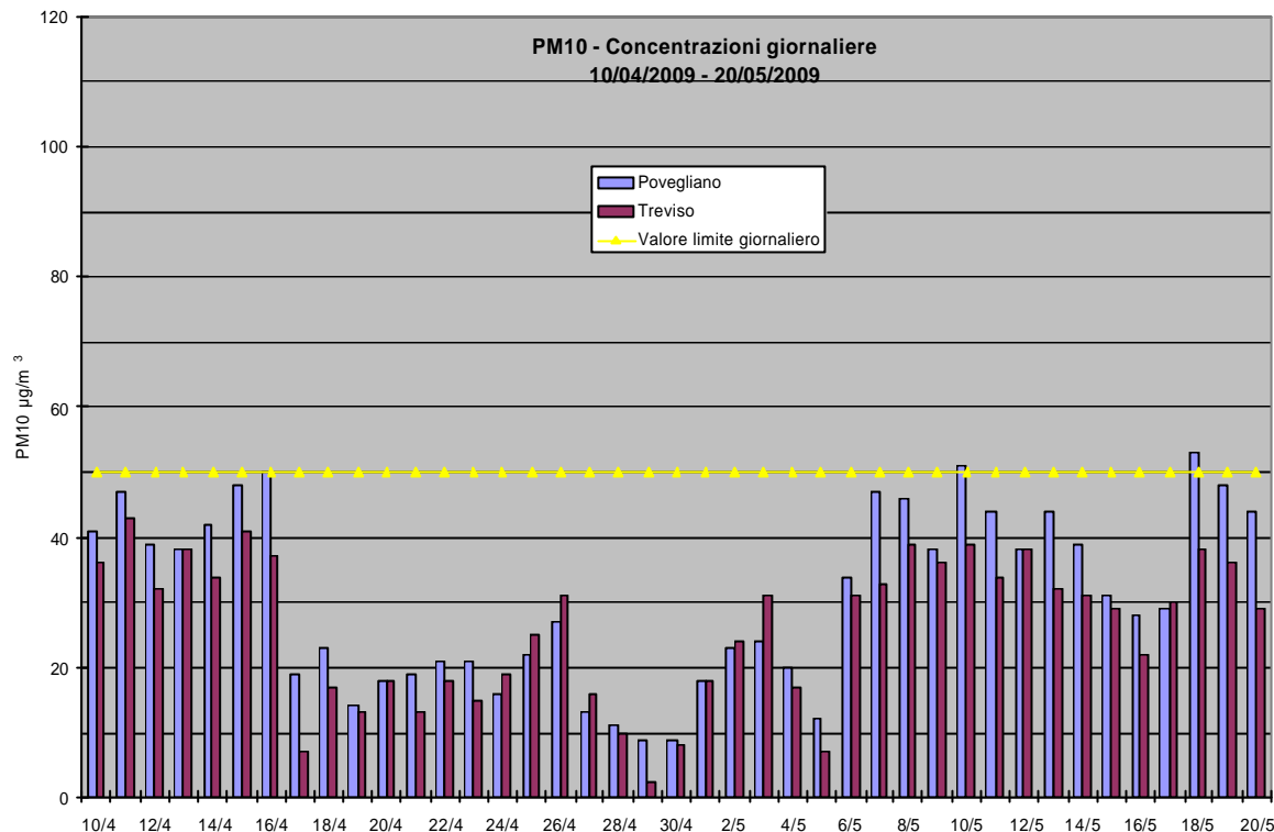
Grafico 9: Valori medi giornalieri di PM10 rilevati presso la stazione fissa di Treviso e la stazione rilocabile posizionata a Povegliano – campagna estiva
