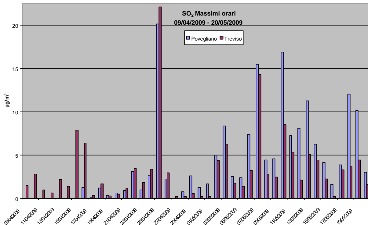
Grafico 7: Valori massimi orari di SO 2 rilevati presso la stazione fissa di Treviso e la stazione rilocabile posizionata a Povegliano – campagna estiva
