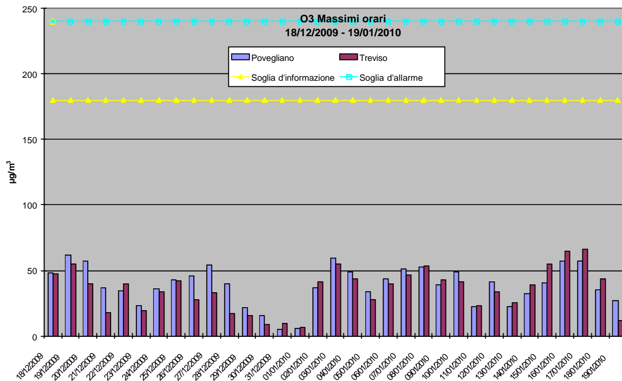
Grafico 6: Valori massimi orari di O 3 rilevati presso la stazione fissa di Treviso e la stazione rilocabile posizionata a Povegliano – campagna invernale
