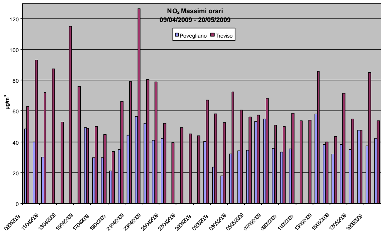
Grafico 3: Valori massimi orari di NO 2 rilevati presso la stazione fissa di Treviso e la stazione rilocabile posizionata a Povegliano – campagna estiva
