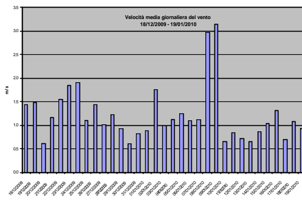
Grafico 13: Valori medi giornalieri di velocità del vento osservati presso la stazione rilocabile posizionata a Povegliano – campagna invernale
