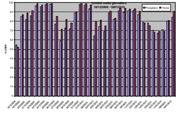
Grafico 19: Valori medi giornalieri di umidità osservati presso la stazione fissa di Treviso e la stazione rilocabile posizionata a Povegliano – campagna invernale
