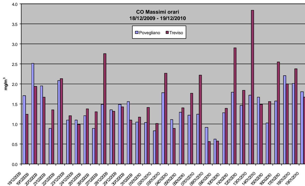
Grafico 2: Valori massimi orari di CO rilevati presso la stazione fissa di Treviso e la stazione rilocabile posizionata a Povegliano – campagna invernale.
