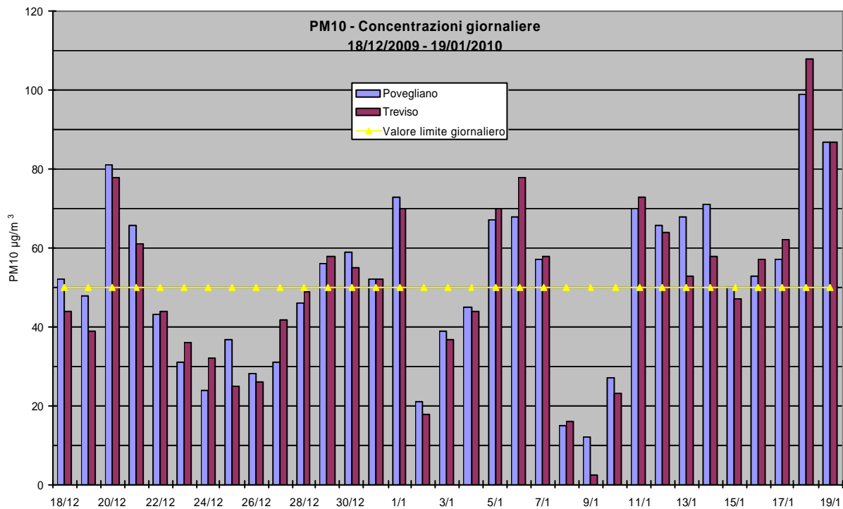
Grafico 10: Valori medi giornalieri di PM10 rilevati presso la stazione fissa di Treviso e la stazione rilocabile posizionata a Povegliano – campagna invernale
