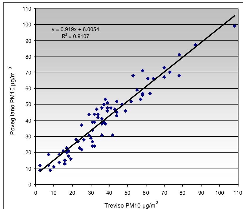
Grafico22: PM10 - rapporto tra la stazione rilocabile e quella di Treviso
