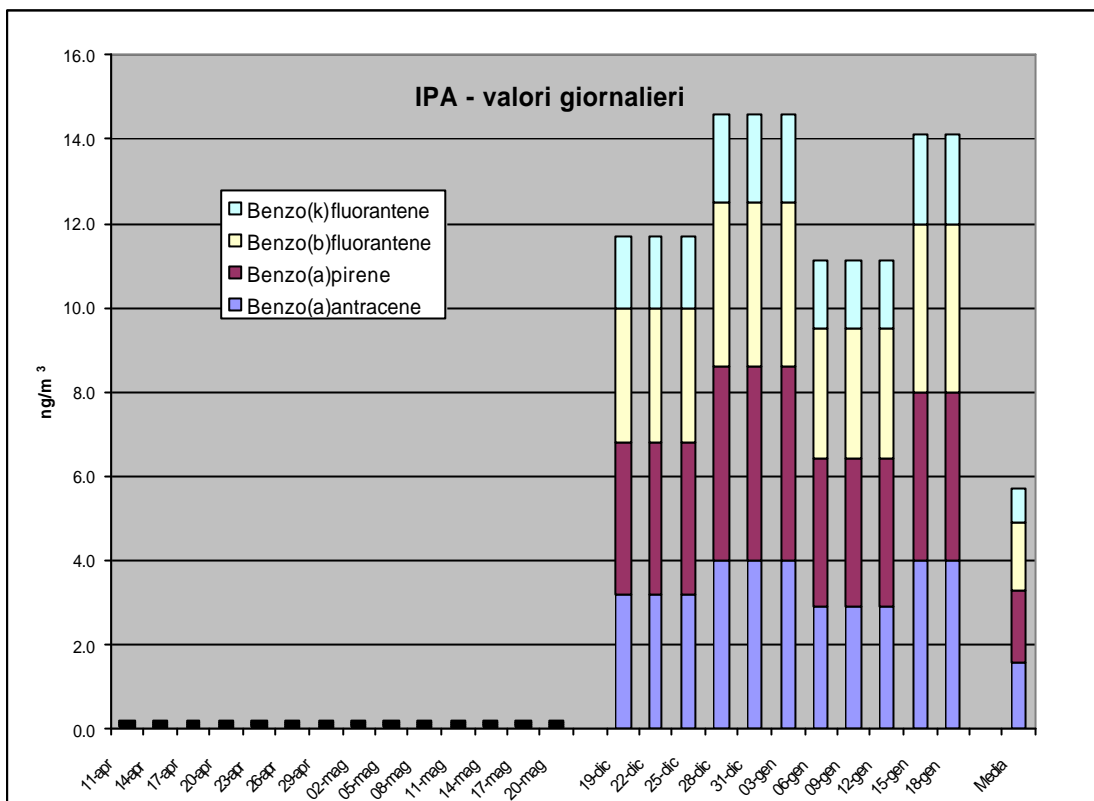
Grafico 20: Valori giornalieri di IPA (Benzo(a)pirene, Benzo(b)fluorantene, Benzo(k)fluorantene, Benzo(a)antracene) rilevati a Povegliano
