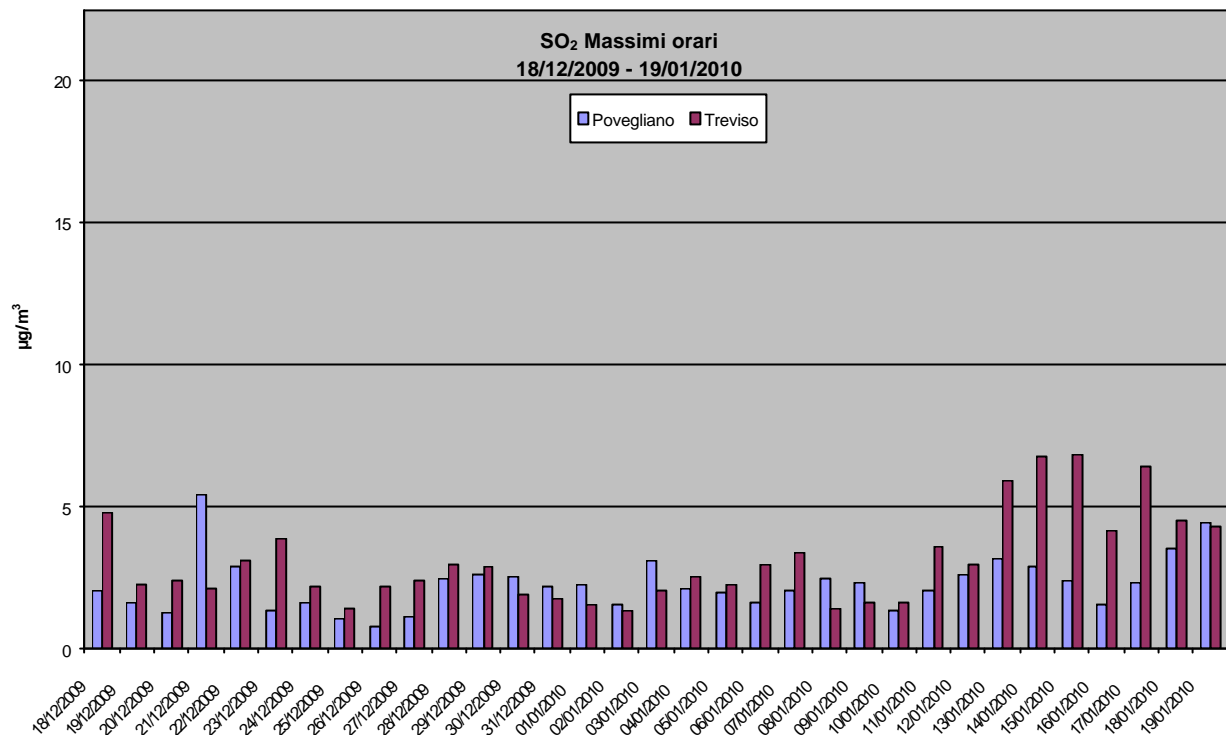
Grafico 8: Valori massimi orari di SO 2 rilevati presso la stazione fissa di Treviso e la stazione rilocabile posizionata a Povegliano – campagna invernale
