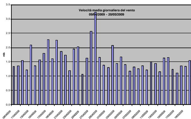
Grafico 12: Valori medi giornalieri di velocità del vento osservati presso la stazione rilocabile posizionata a Povegliano – campagna estiva
