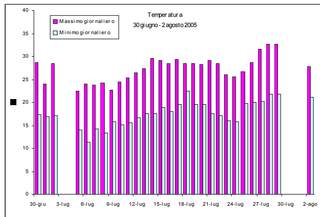
Figura 8b – Valori minimi e massimi giornalieri di Temperatura osservati presso la stazione rilocabile posizionata a Refrontolo – campagna estiva
