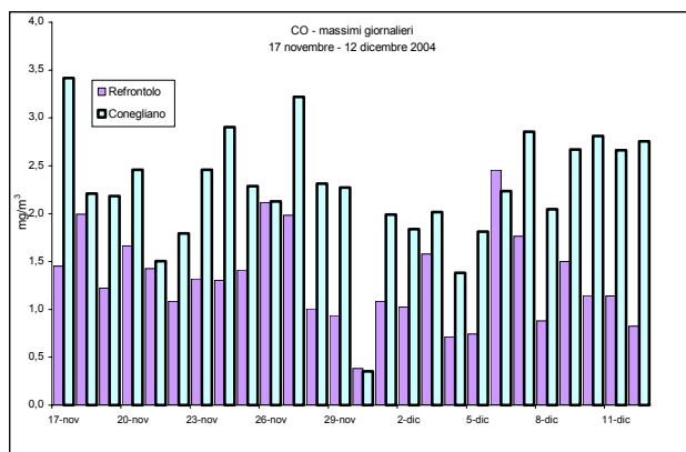
Figura 1a –Valori massimi di CO rilevati presso la stazione fissa di Conegliano e la stazione rilocabile posizionata a Refrontolo – campagna invernale
