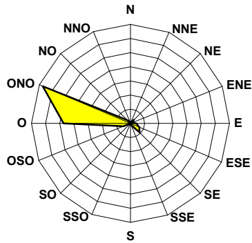
Figura 6a – Direzione del vento – numero di eventi osservati presso la stazione fissa di Conegliano – campagna invernale
