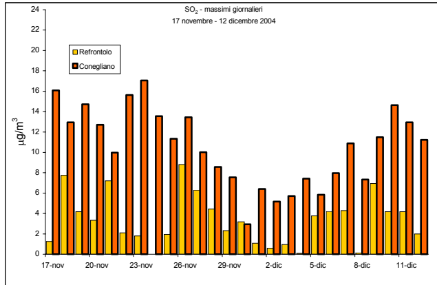
Figura 4a –Valori massimi di SO 2 rilevati presso la stazione fissa di Conegliano e la stazione rilocabile posizionata a Refrontolo – campagna invernale
