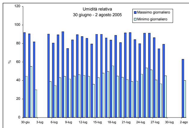
Figura 9b – Valori minimi e massimi giornalieri di Umidità % relativa osservati presso la stazione rilocabile posizionata a Refrontolo – campagna estiva
