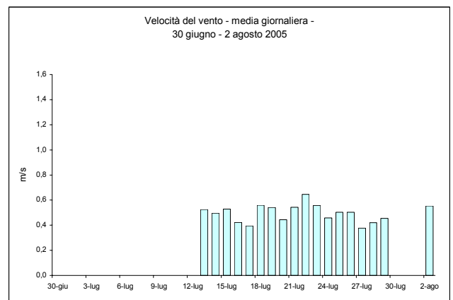
Figura 7b – Valori medi giornalieri di Velocità del vento osservati presso la stazione rilocabile posizionata a Refrontolo – campagna estiva
