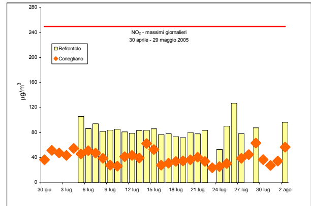
Figura 2b –Valori massimi di NO 2 rilevati presso la stazione fissa di Conegliano e la stazione rilocabile posizionata a Refrontolo – campagna estiva
