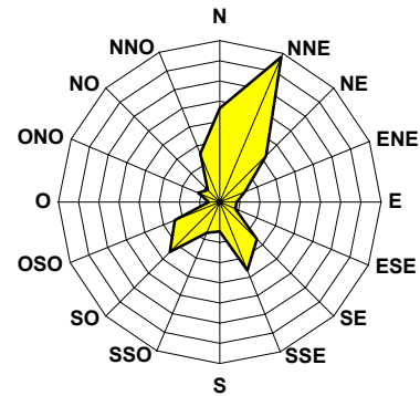
Figura 6b – Direzione del vento – numero di eventi osservati presso la stazione rilocabile posizionata a Refrontolo – campagna estiva
