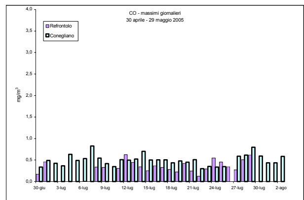
Figura 1b –Valori massimi di CO rilevati presso la stazione fissa di Conegliano e la stazione rilocabile posizionata a Refrontolo – campagna estiva
