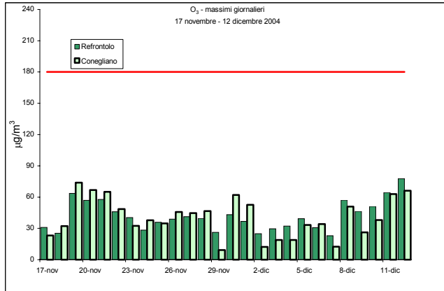
Figura 3a –Valori massimi di O 3 rilevati presso la stazione fissa di Conegliano e la stazione rilocabile posizionata a Refrontolo – campagna invernale
