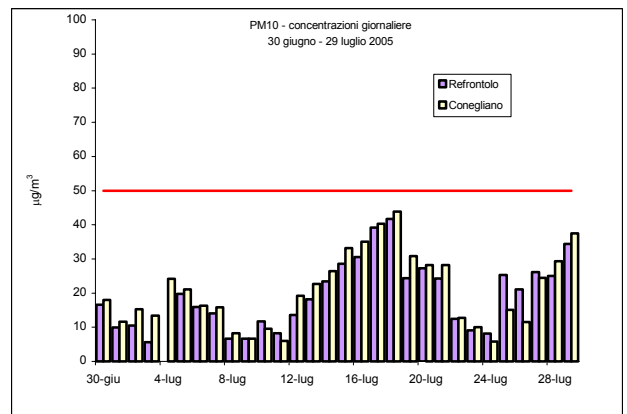
Figura 5b –Valori medi giornalieri di PM10 rilevati presso la stazione fissa di Conegliano e la stazione rilocabile posizionata a Refrontolo – campagna estiva
