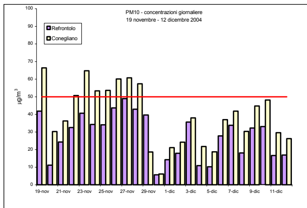
Figura 5a –Valori medi giornalieri di PM10 rilevati presso la stazione fissa di Conegliano e la stazione rilocabile posizionata a Refrontolo – campagna invernale
