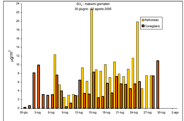
Figura 4b –Valori massimi di SO 2 rilevati presso la stazione fissa di Conegliano e la stazione rilocabile posizionata a Refrontolo – campagna estiva
