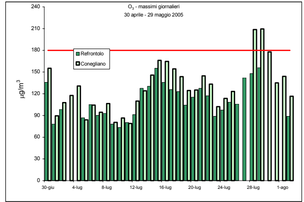
Figura 3b –Valori massimi di O 3 rilevati presso la stazione fissa di Conegliano e la stazione rilocabile posizionata a Refrontolo – campagna estiva
