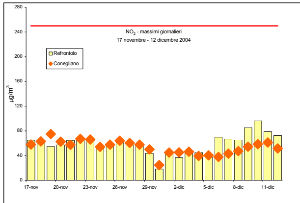
Figura 2a –Valori massimi di NO 2 rilevati presso la stazione fissa di Conegliano e la stazione rilocabile posizionata a Refrontolo – campagna invernale
