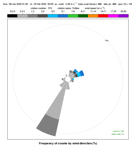
Figura 4: rosa dei venti a scansione oraria registrati presso la stazione meteorologica di Follina nel periodo 8 gennaio – 17 febbraio 2020
