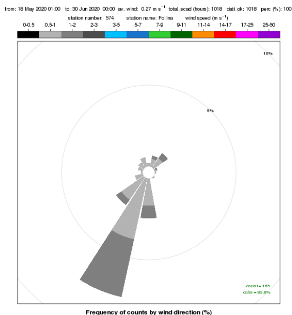
Figura 6: rosa dei venti a scansione oraria registrati presso la stazione meteorologica di Follina nel periodo 18 maggio – 29 giugno 2020
