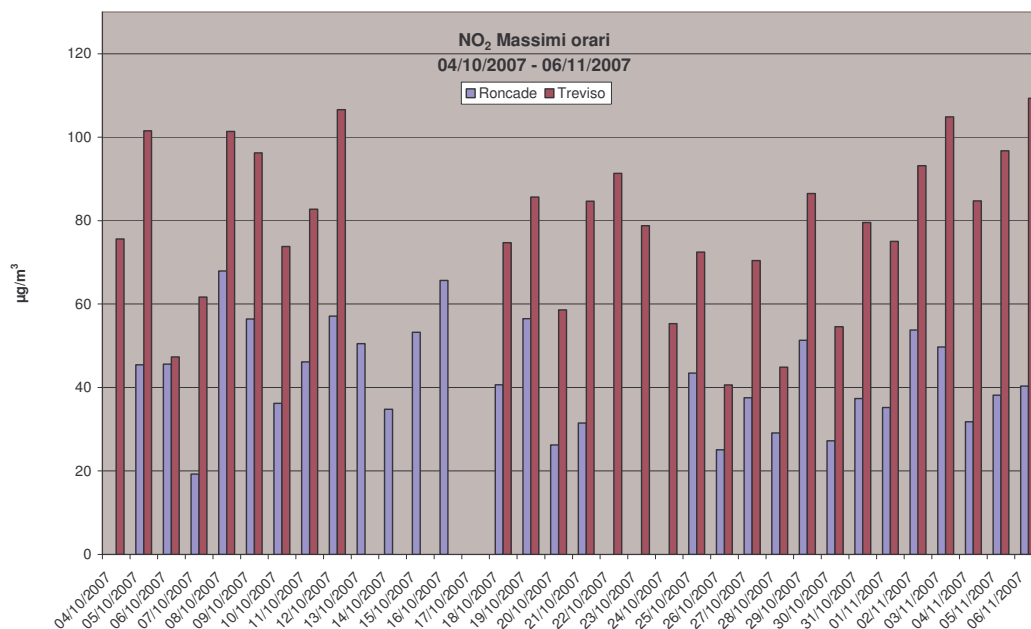
Grafico 4: Valori massimi orari di NO 2 rilevati presso la stazione fissa di Treviso e la stazione rilocabile posizionata a Roncade – campagna invernale.
