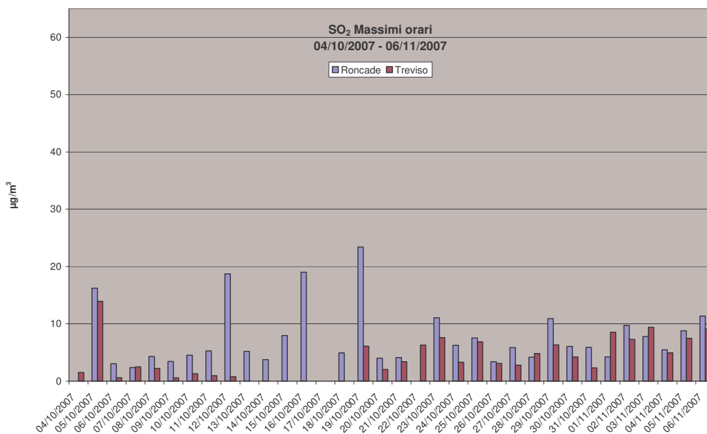
Grafico 8: Valori massimi orari di SO 2 rilevati presso la stazione fissa di Treviso e la stazione rilocabile posizionata a Roncade – campagna invernale.
