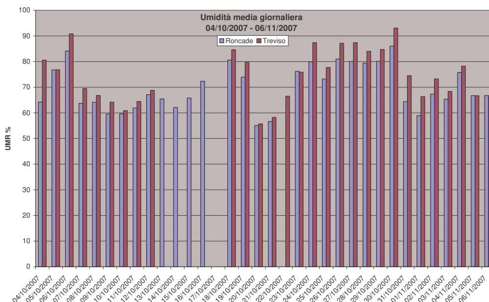
Grafico 18: Valori medi giornalieri di umidità osservati presso la stazione fissa di Treviso e la stazione rilocabile posizionata a Roncade – campagna invernale.
