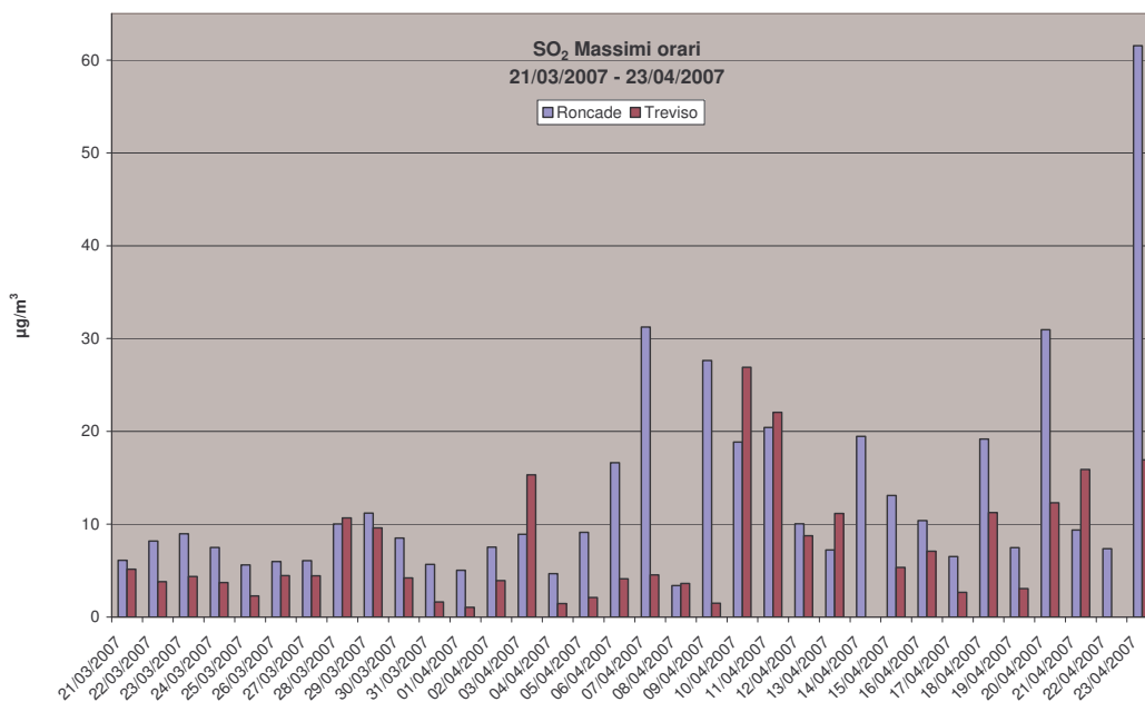
Grafico 7: Valori massimi orari di SO 2 rilevati presso la stazione fissa di Treviso e la stazione rilocabile posizionata a Roncade – campagna estiva.
