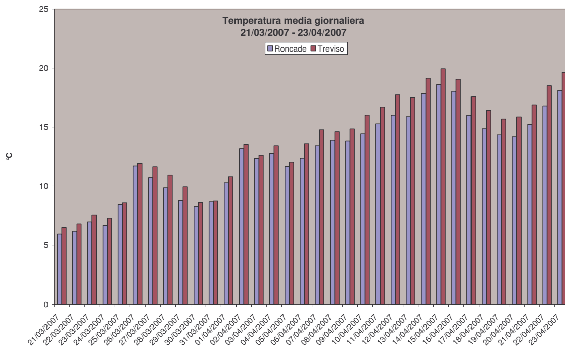
Grafico 15: Valori medi giornalieri di temperatura osservati presso la stazione fissa di Treviso e la stazione rilocabile posizionata a Roncade – campagna estiva.
