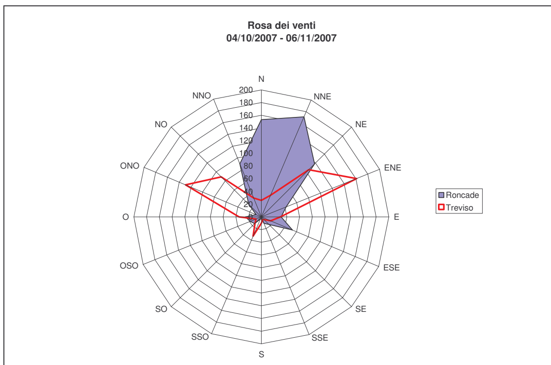
Grafico 14: Rosa dei venti presso la stazione fissa di Treviso e la stazione rilocabile posizionata a Roncade – campagna invernale.
