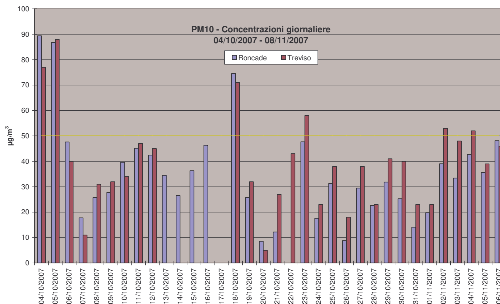
Grafico 10: Valori medi giornalieri di PM 10 rilevati presso la stazione fissa di Treviso e la stazione rilocabile posizionata a Roncade – campagna invernale.
