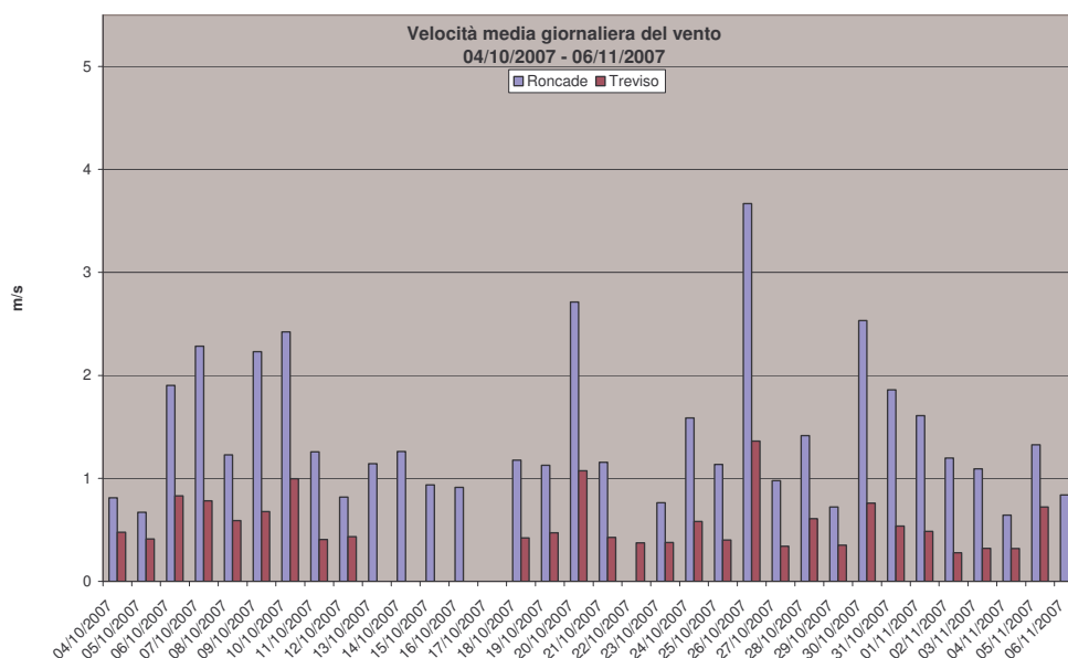
Grafico 12: Valori medi giornalieri di velocità del vento osservati presso la stazione fissa di Treviso e la stazione rilocabile posizionata a Roncade – campagna invernale.
