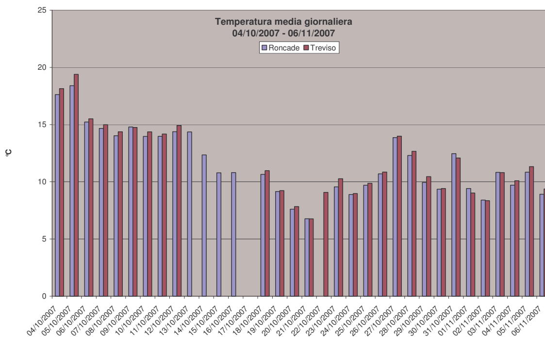
Grafico 16: Valori medi giornalieri di temperatura osservati presso la stazione fissa di Treviso e la stazione rilocabile posizionata a Roncade – campagna invernale.
