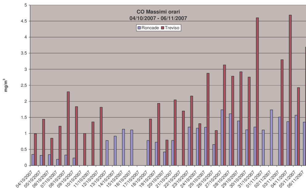
Grafico 2: Valori massimi orari di CO rilevati presso la stazione fissa di Treviso e la stazione rilocabile posizionata a Roncade – campagna invernale.
