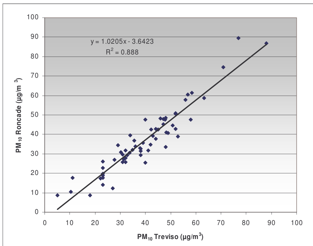
Grafico 20: Correlazione tra le concentrazioni di PM_{10} rilevate presso la stazione di Treviso e a Roncade.
