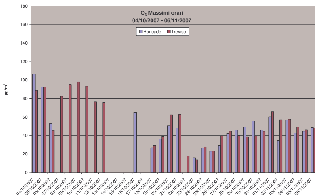
Grafico 6: Valori massimi orari di O 3 rilevati presso la stazione fissa di Treviso e la stazione rilocabile posizionata a Roncade – campagna invernale.
