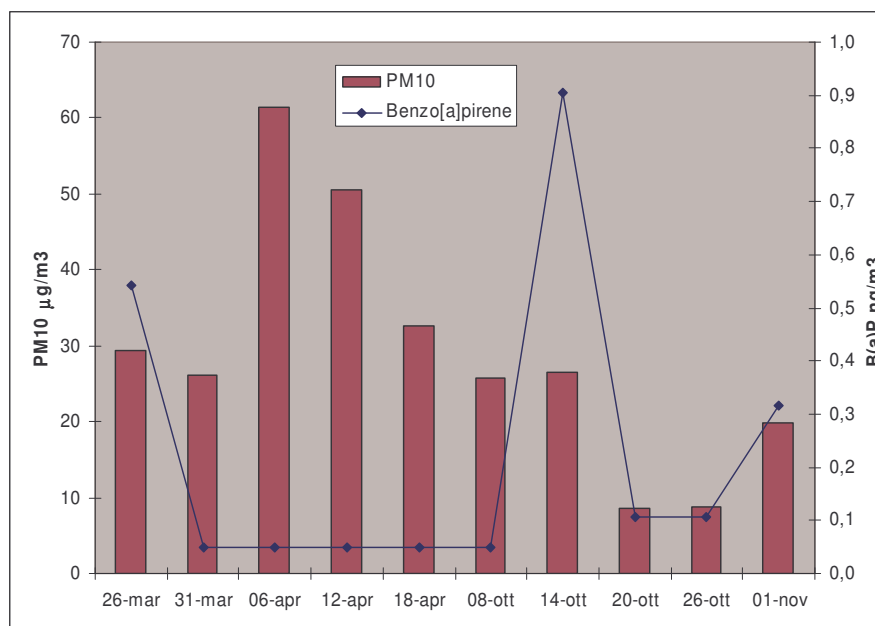
Grafico 19: Andamento del B(a)P e del PM 10 rilevati presso la stazione rilocabile.
