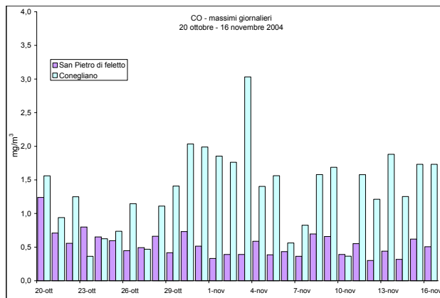
Figura 1a –Valori massimi di CO rilevati presso la stazione fissa di Conegliano e la stazione rilocabile posizionata a San Pietro di Feletto – campagna invernale
