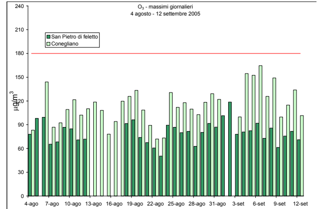
Figura 3b –Valori massimi di O 3 rilevati presso la stazione fissa di Conegliano e la stazione rilocabile posizionata a San Pietro di Feletto – campagna estiva
