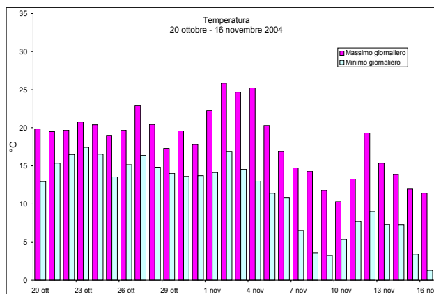
Figura 8a – Valori minimi e massimi giornalieri di Temperatura osservati presso la stazione fissa di Conegliano – campagna invernale
