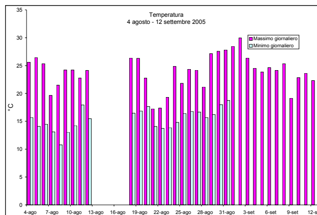
Figura 8b – Valori minimi e massimi giornalieri di Temperatura osservati presso la stazione rilocabile posizionata a San Pietro di Feletto – campagna estiva
