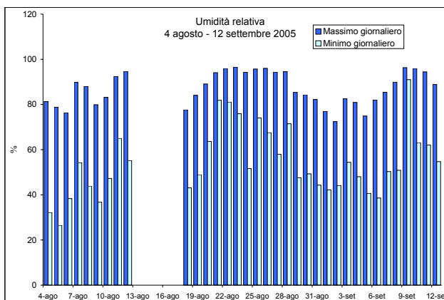
Figura 9b – Valori minimi e massimi giornalieri di Umidità % relativa osservati presso la stazione rilocabile posizionata a San Pietro di Feletto – campagna estiva
