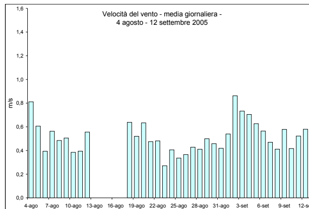
Figura 7b – Valori medi giornalieri di Velocità del vento osservati presso la stazione rilocabile posizionata a San Pietro di Feletto – campagna estiva
