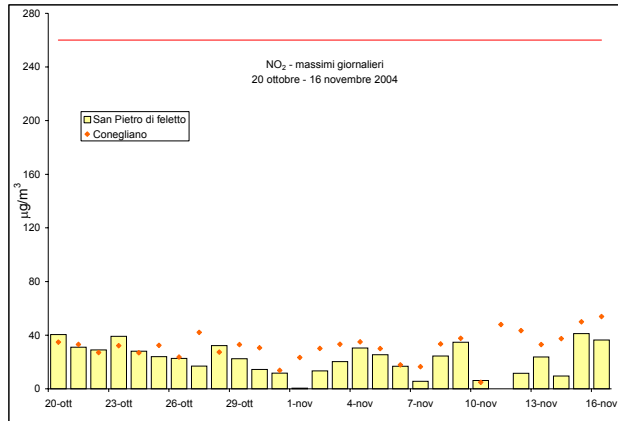
Figura 2a –Valori massimi di NO 2 rilevati presso la stazione fissa di Conegliano e la stazione rilocabile posizionata a San Pietro di Feletto – campagna invernale
