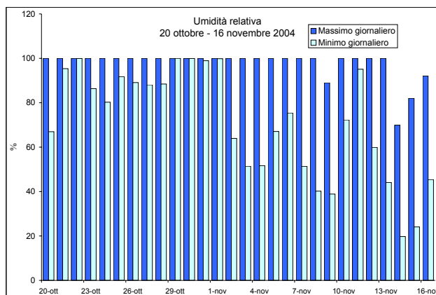
Figura 9a – Valori minimi e massimi giornalieri di Umidità % relativa osservati presso la stazione fissa di Conegliano – campagna invernale
