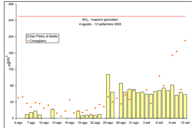
Figura 2b –Valori massimi di NO 2 rilevati presso la stazione fissa di Conegliano e la stazione rilocabile posizionata a San Pietro di Feletto – campagna estiva
