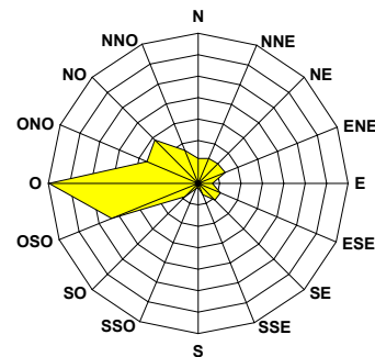
Figura 6b – Direzione del vento – numero di eventi osservati presso la stazione rilocabile posizionata a San Pietro di Feletto – campagna estiva
