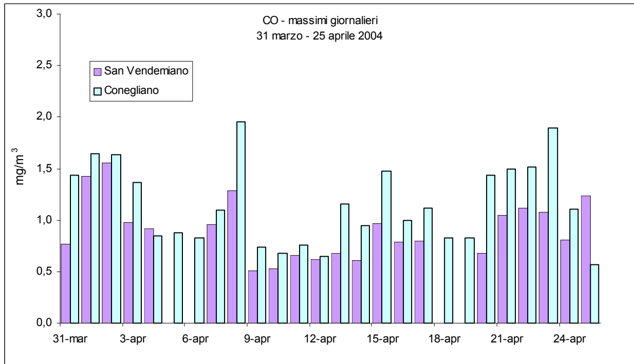
Figura 3 –Valori massimi di monossido di carbonio CO rilevati presso la stazione fissa di Conegliano e il Laboratorio Mobile posizionato a San Vendemiano
