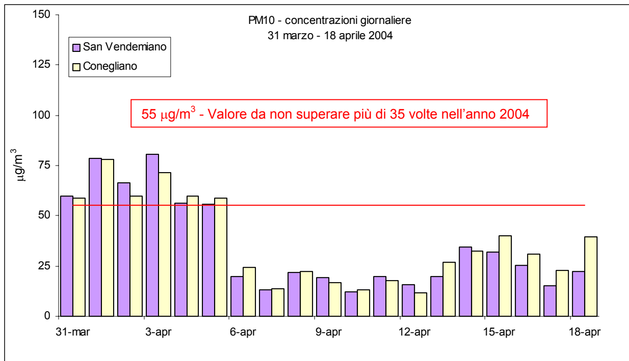
Figura 6 –Valori massimi di polveri inalabili PM10 rilevati presso la stazione fissa di Conegliano e il Laboratorio Mobile posizionato a San Vendemiano
