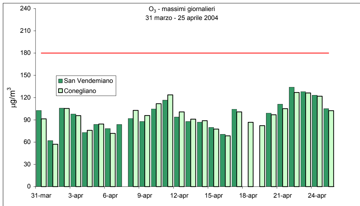
Figura 5 –Valori massimi di ozono O 3 rilevati presso la stazione fissa di Conegliano e il Laboratorio Mobile posizionato a San Vendemiano
