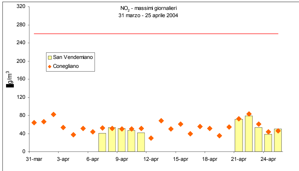
Figura 4 –Valori massimi di biossido di azoto NO 2 rilevati presso la stazione fissa di Conegliano e il Laboratorio Mobile posizionato a San Vendemiano
