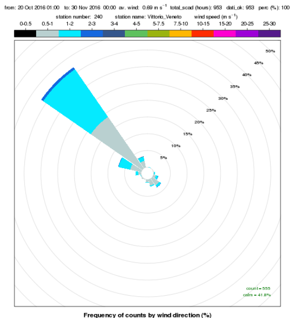
Figura 6. rosa dei venti a scansione oraria registrati presso la stazione meteorologica di Vittorio Veneto nel periodo 20 ottobre - 29 novembre 2016
