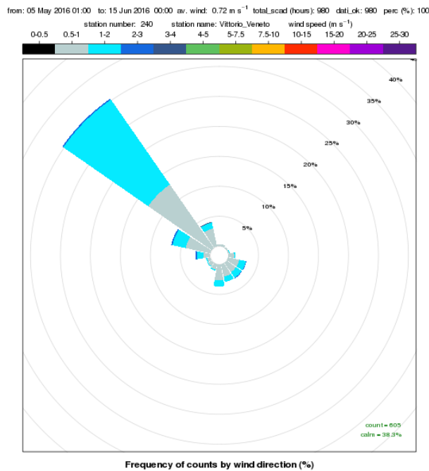
Figura 4. rosa dei venti a scansione oraria registrati presso la stazione meteorologica di Vittorio Veneto nel periodo 5maggio - 14 giugno 2016
