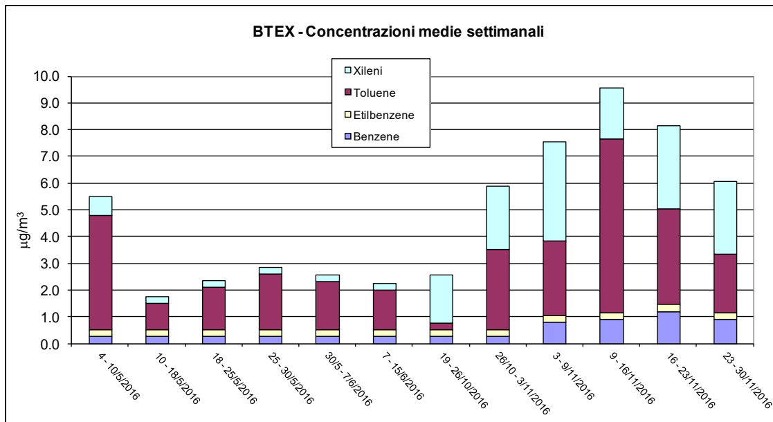
Grafico 2 - Valori settimanali di BTEX (benzene, toluene, etilbenzene e xilene) rilevati a Sarmede.
