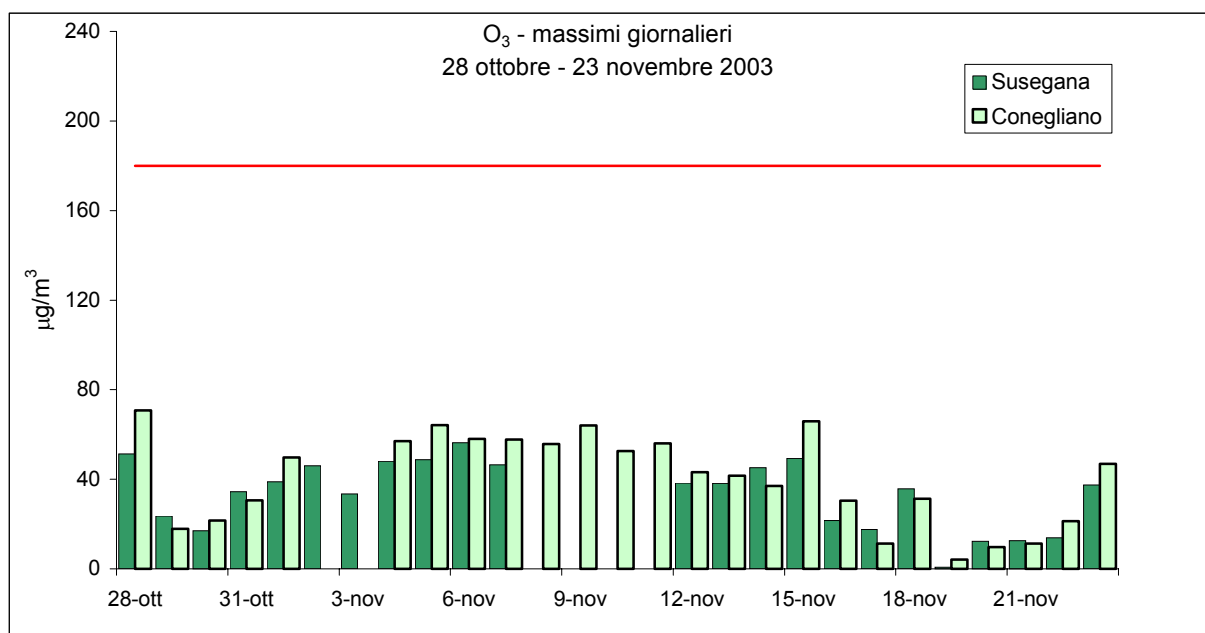
Figura 6 –Valori massimi di ozono O 3 rilevati presso la stazione fissa di Conegliano e il Laboratorio Mobile posizionato a Susegana
