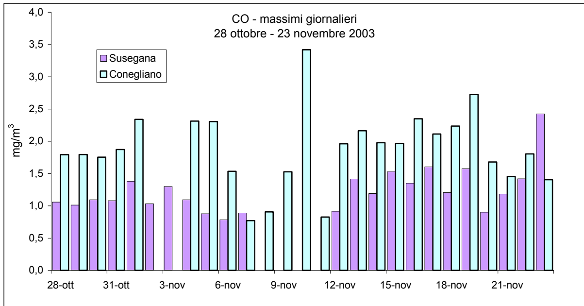
Figura 4 –Valori massimi di monossido di carbonio CO rilevati presso la stazione fissa di Conegliano e il Laboratorio Mobile posizionato a Susegana
