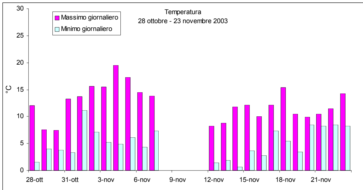
Figura 11 – Valori minimi e massimi di Temperatura rilevati presso il Laboratorio Mobile posizionato a Susegana.
