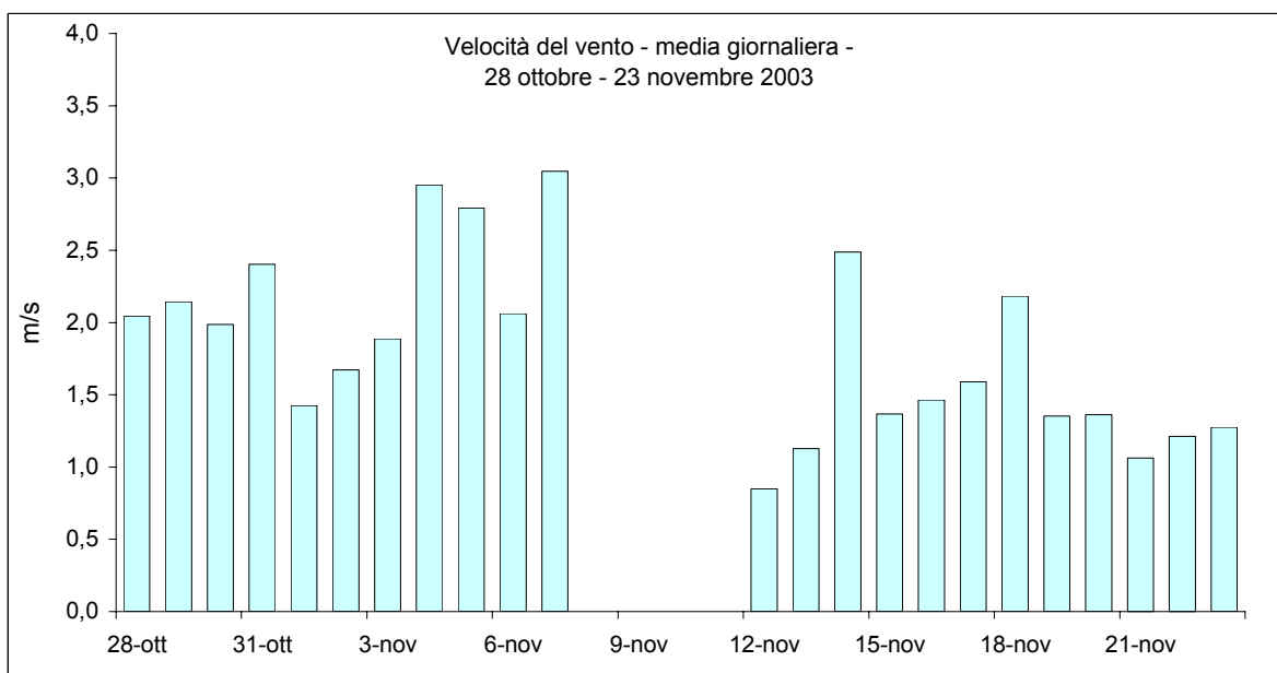
Figura 9 – Valori medi giornalieri della velocità del vento rilevati presso il Laboratorio Mobile posizionato a Susegana.
