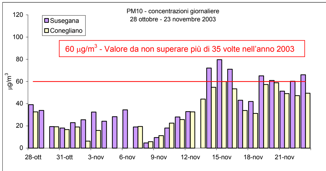
Figura 7 –Valori massimi di polveri inalabili PM10 rilevati presso la stazione fissa di Conegliano e il Laboratorio Mobile posizionato a Susegana
