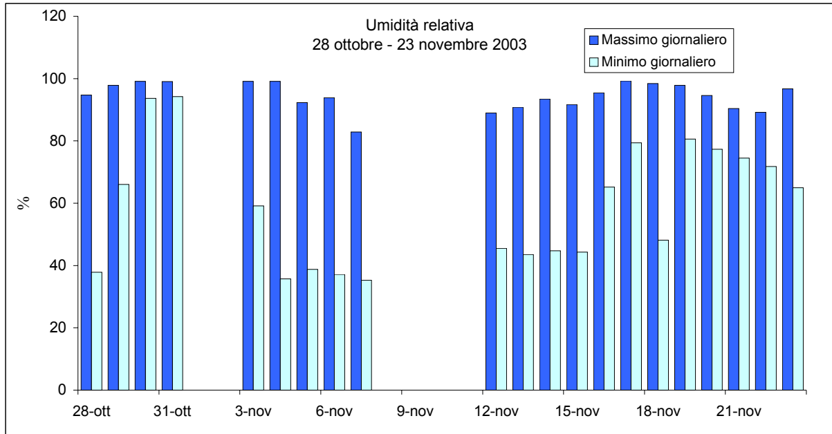
Figura 12 – Valori medi giornalieri di umidità % relativa rilevata presso il Laboratorio Mobile posizionato a Susegana.
