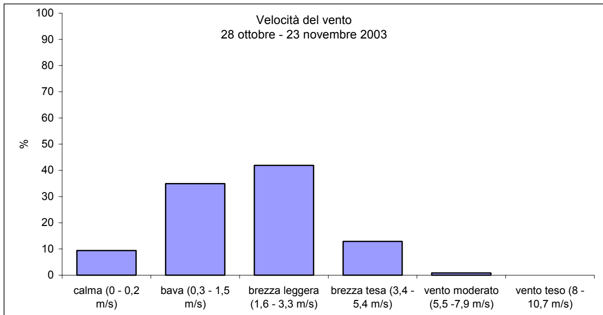
Figura 10 – Distribuzione di frequenza % delle classi di velocità del vento misurate presso il Laboratorio Mobile posizionato nel comune di Susegana.
