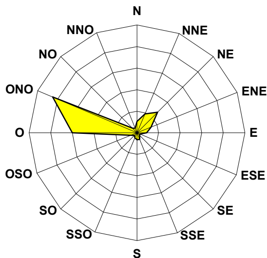
Figura 8 – Direzione del vento- numero di eventi osservati durante la campagna di rilevamento con Laboratorio Mobile posizionato a Susegana.
