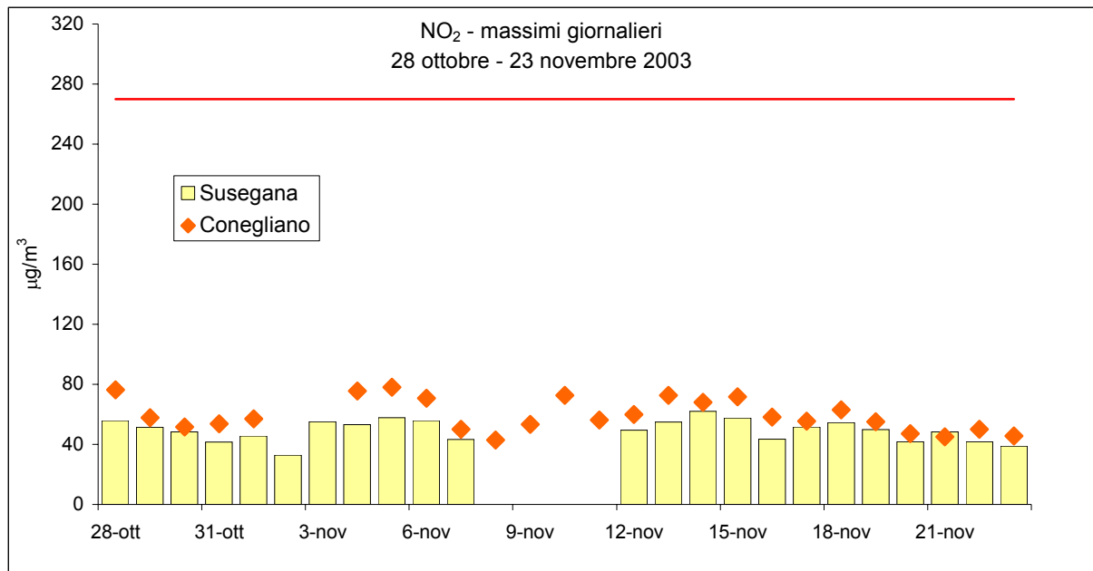
Figura 5 –Valori massimi di biossido di azoto NO 2 rilevati presso la stazione fissa di Conegliano e il Laboratorio Mobile posizionato a Susegana
