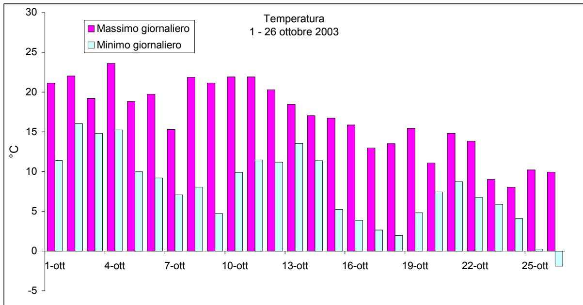
Figura 11 – Valori minimi e massimi di Temperatura rilevati presso il Laboratorio Mobile posizionato a Vazzola.
