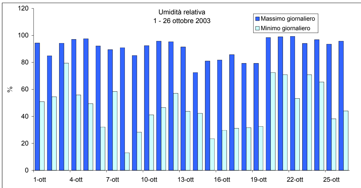
Figura 12 – Valori medi giornalieri di umidità % relativa rilevata presso il Laboratorio Mobile posizionato a Vazzola.
