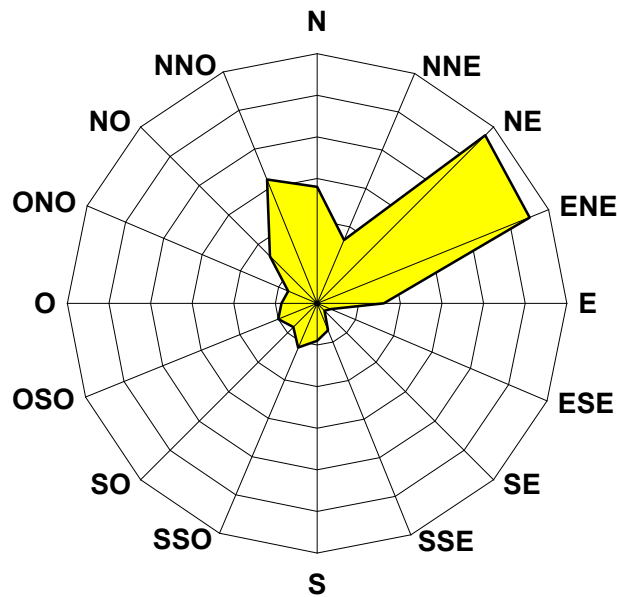
Figura 8 – Direzione del vento- numero di eventi osservati durante la campagna di rilevamento con Laboratorio Mobile posizionato a Vazzola.
