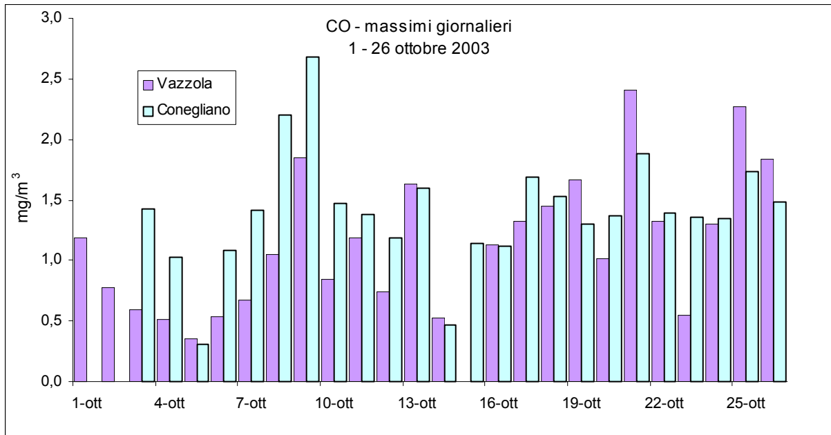
Figura 4 –Valori massimi di monossido di carbonio CO rilevati presso la stazione fissa di Conegliano e il Laboratorio Mobile posizionato a Vazzola
