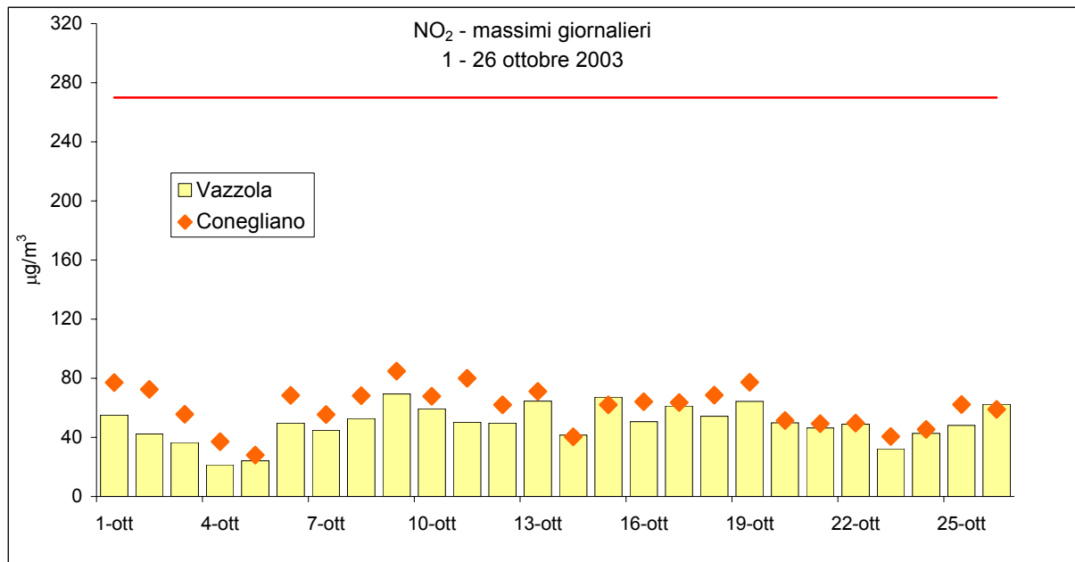
Figura 5 –Valori massimi di biossido di azoto NO 2 rilevati presso la stazione fissa di Conegliano e il Laboratorio Mobile posizionato a Vazzola
