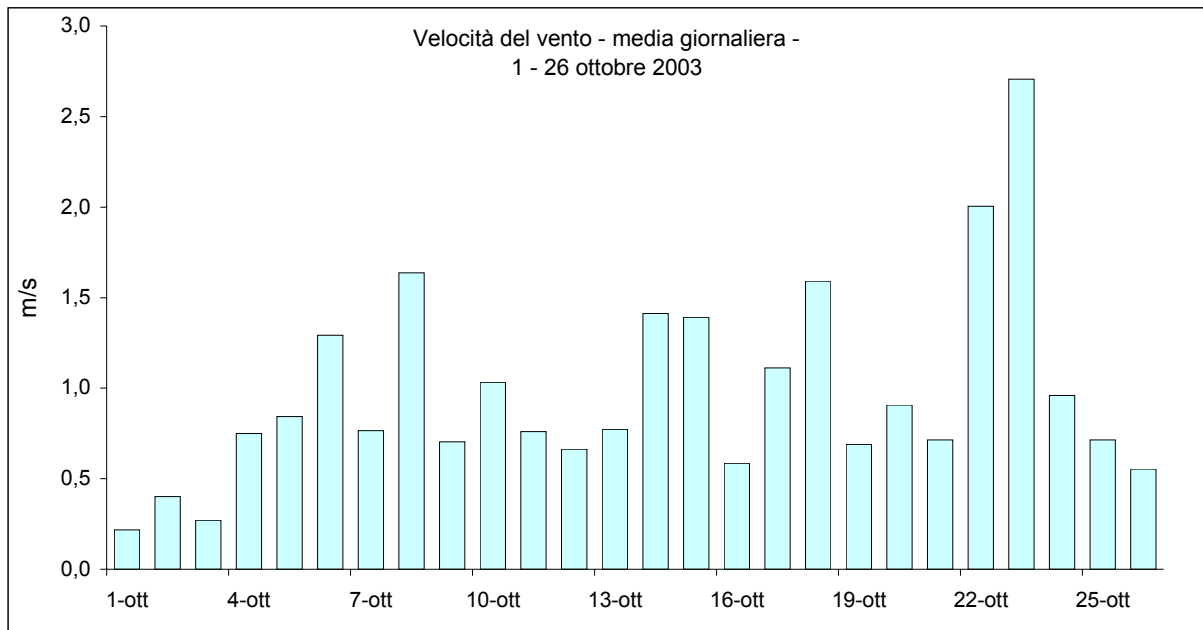
Figura 9 – Valori medi giornalieri della velocità del vento rilevati presso il Laboratorio Mobile posizionato a Vazzola.
