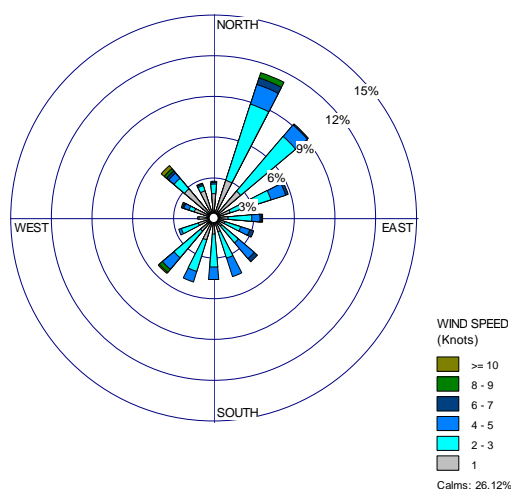
Figura 4. rosa dei venti a scansione oraria registrati presso la stazione meteorologica di Castelfranco Veneto nel periodo 8 aprile – 18 maggio 2014
