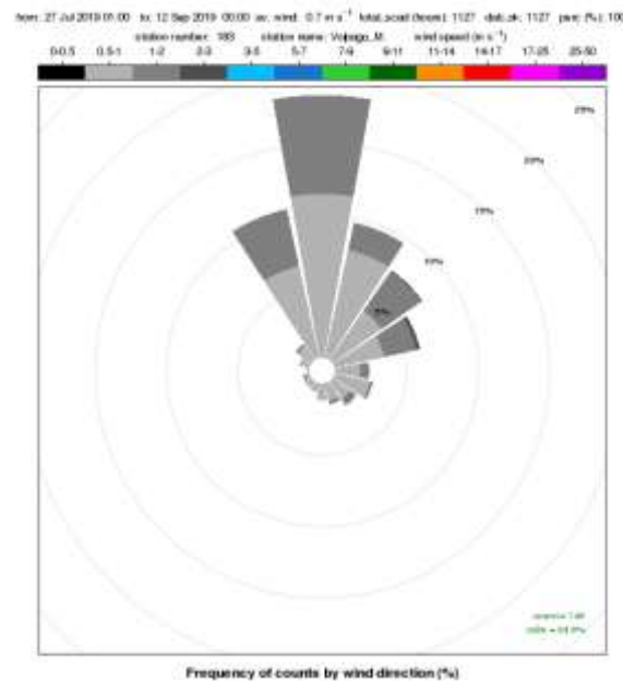
Figura 6. rosa dei venti a scansione oraria registrati presso la stazione meteorologica di Volpago del Montello nel periodo 27 luglio – 11 settembre 2019
