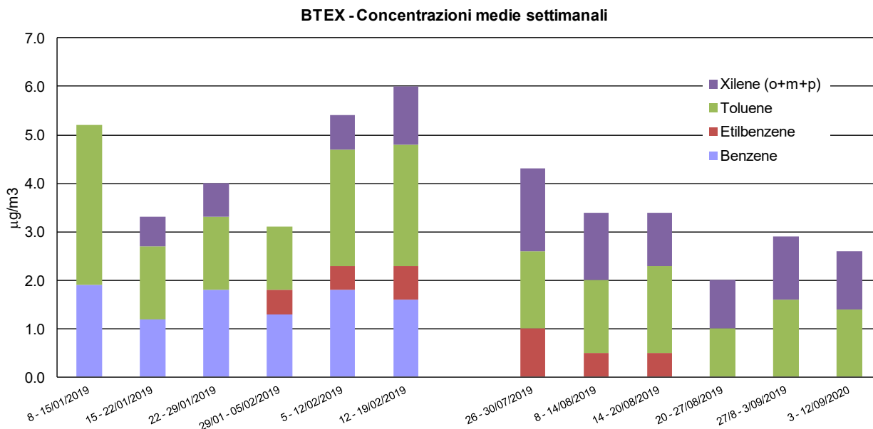
Grafico 8 Concentrazioni Medie Settimanali di BTEX rilevate a Volpago del Montello.
