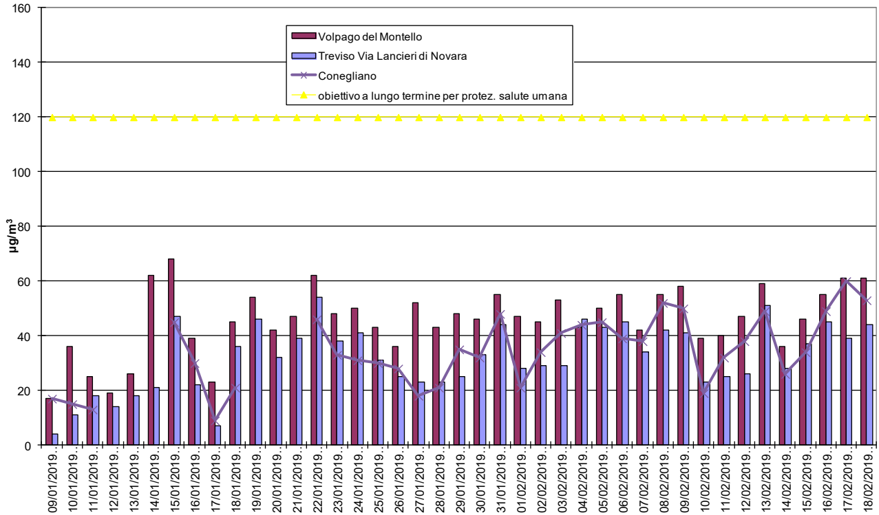
Grafico 5 – Concentrazione Massima Giornaliera della Media Mobile di 8 ore di O 3 (µg/m 3 ). Semestre “invernale”
