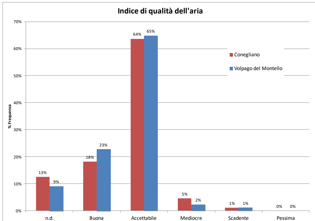
Figura 7. Indice sintetico di qualità dell'aria per la campagna di Volpago del Montello confrontato con quello calcolato per la stazione fissa di Treviso – via Lancieri di Novara
