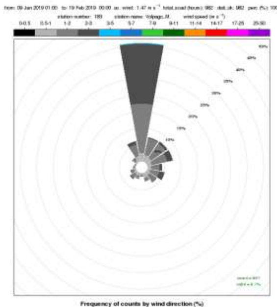
Figura 4. rosa dei venti a scansione oraria registrati presso la stazione meteorologica di Volpago del Montello nel periodo 9 gennaio – 18 febbraio 2019.
