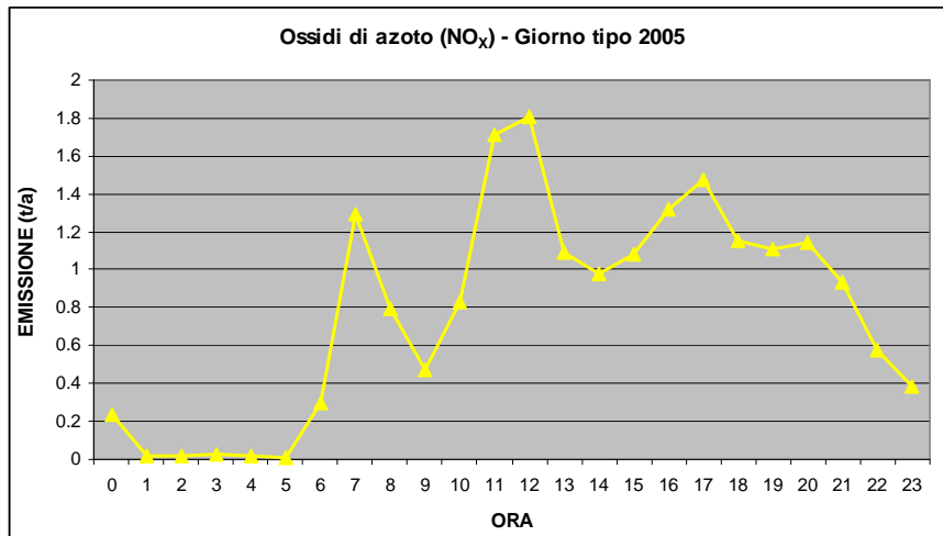
Grafico 1: Giorno tipo 2005 dell'emissione di ossidi di azoto
