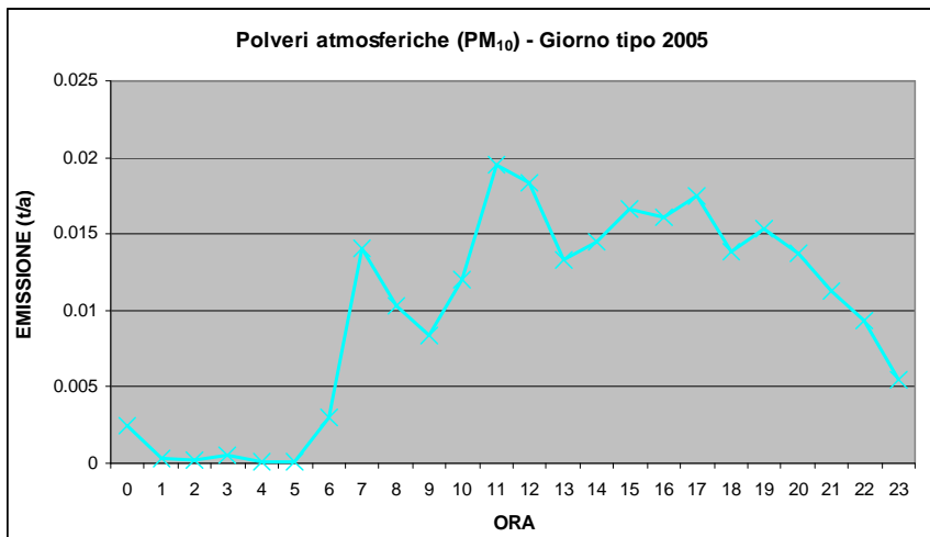
Grafico 4: Giorno tipo 2005 dell'emissione di PM10
