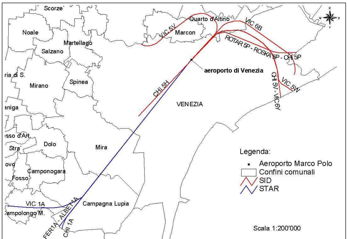
Figura 2: Rotte standard AIP Italia
