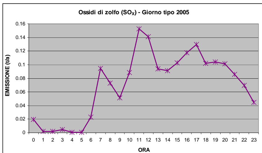
Grafico 3: Giorno tipo 2005 dell'emissione di ossidi di zolfo
