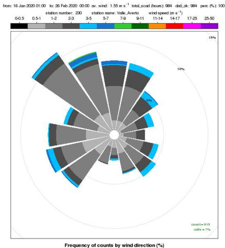
Figura 4. Rosa dei venti registrati presso la stazione meteorologica di Campagna Lupia – Valle Averto nel periodo 16 gennaio – 25 febbraio 2020
