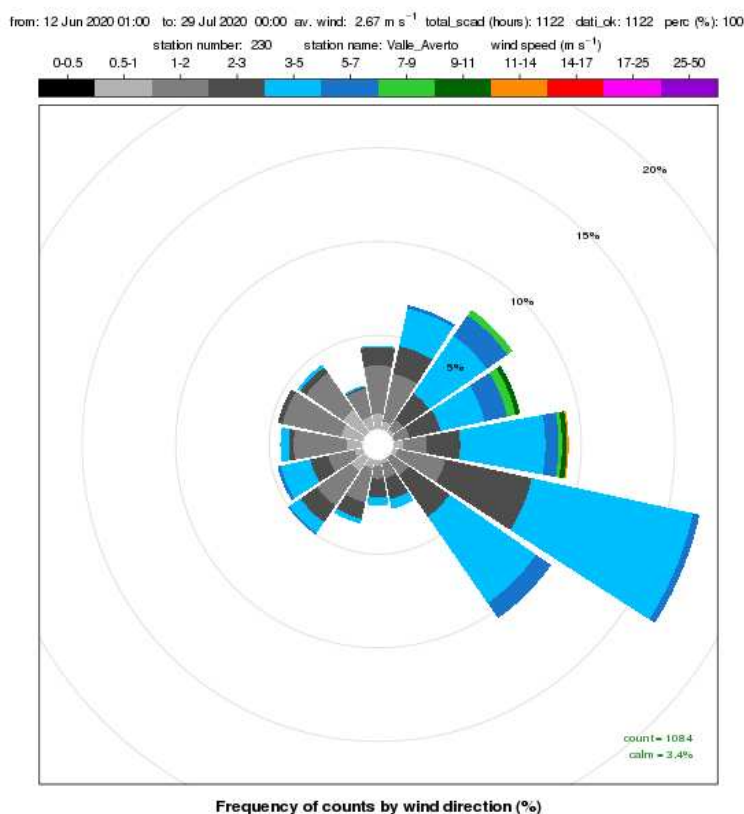
Figura 6. Rosa dei venti registrati presso la stazione meteorologica di Campagna Lupia – Valle Averto nel periodo 12 giugno – 28 luglio 2020
