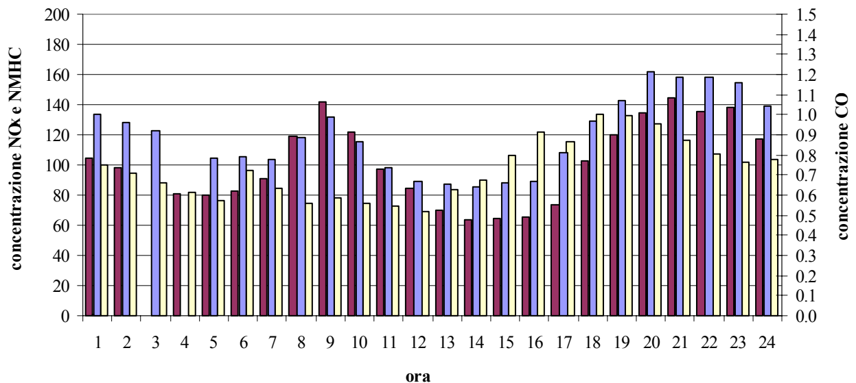
Grafico 8 – Giorno tipo di NMHC, NO x e CO.
