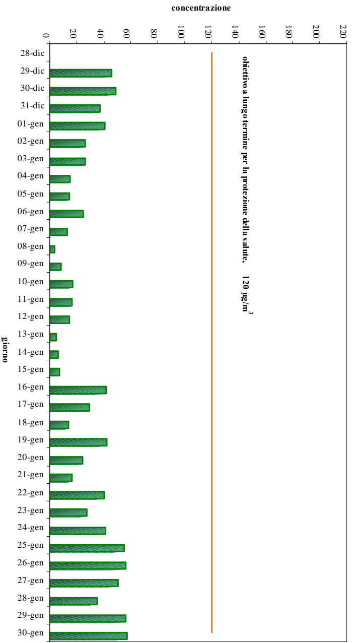
Grafico 6 – Concentrazione Massima Giornaliera della Media Mobile di 8 ore di O 3 (µg/m 3 ).
