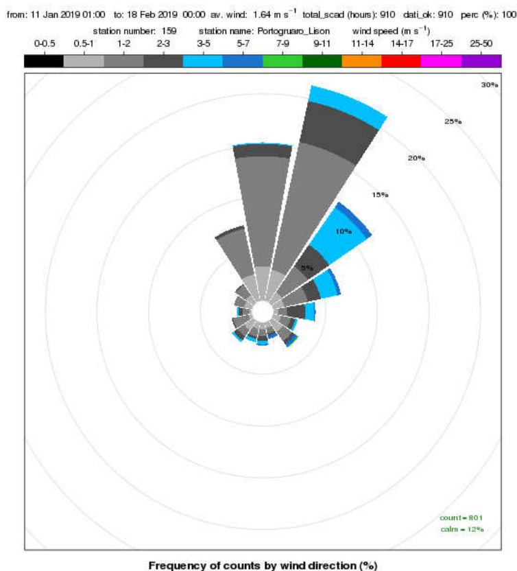
Figura 4. Rosa dei venti registrati presso la stazione meteorologica di Portogruaro Lison nel periodo 11 gennaio – 17 febbraio 2019
