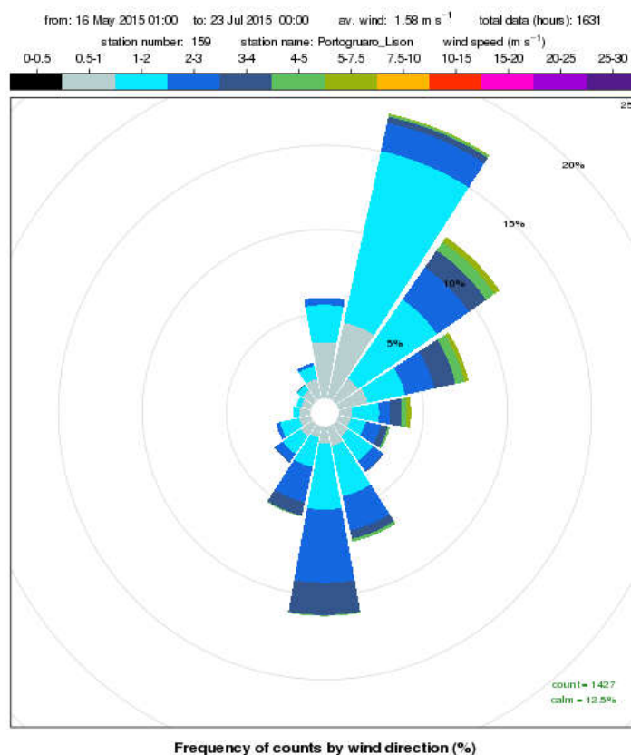
Figura 4: rosa dei venti registrati presso la stazione meteorologica di Portogruaro Lison nel periodo 16 maggio - 22 luglio 2015
