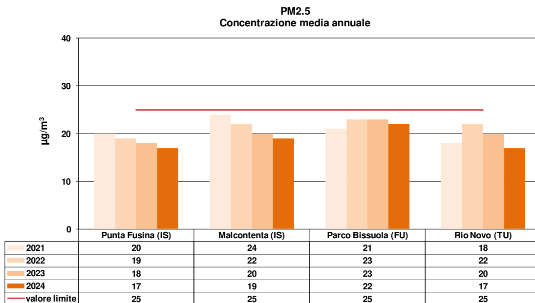
Grafico 20 – Concentrazioni medie annue di PM2.5 (µg/m 3 ). Confronto tra Punta Fusina e le altre stazioni fisse presenti in Comune di Venezia. Anni dal 2021 al 2024
