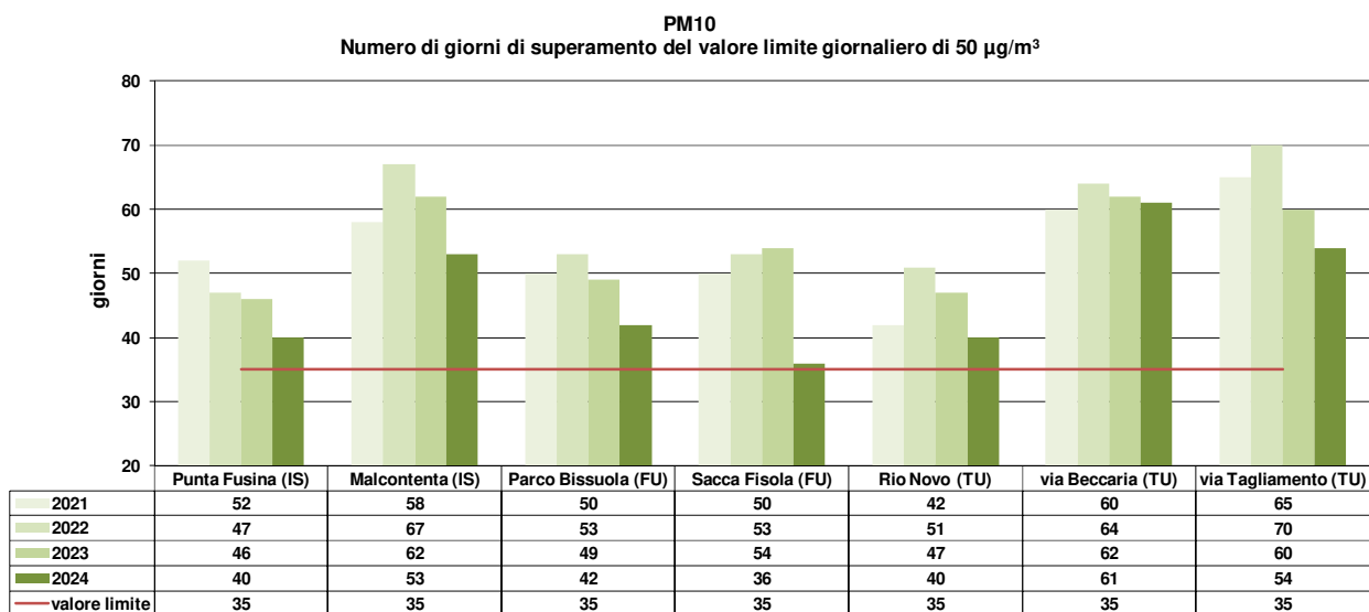
Grafico 19 – Giorni di superamento del valore limite giornaliero per la protezione della salute umana del PM10. Confronto tra Punta Fusina e le altre stazioni fisse presenti in Comune di Venezia. Anni dal 2021 al 2024
