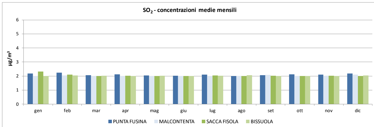
Grafico 5 – Medie mensili della concentrazione di SO_2 ( \mu g/m^3 ). Confronto tra Punta Fusina e le altre stazioni fisse presenti in Comune di Venezia
