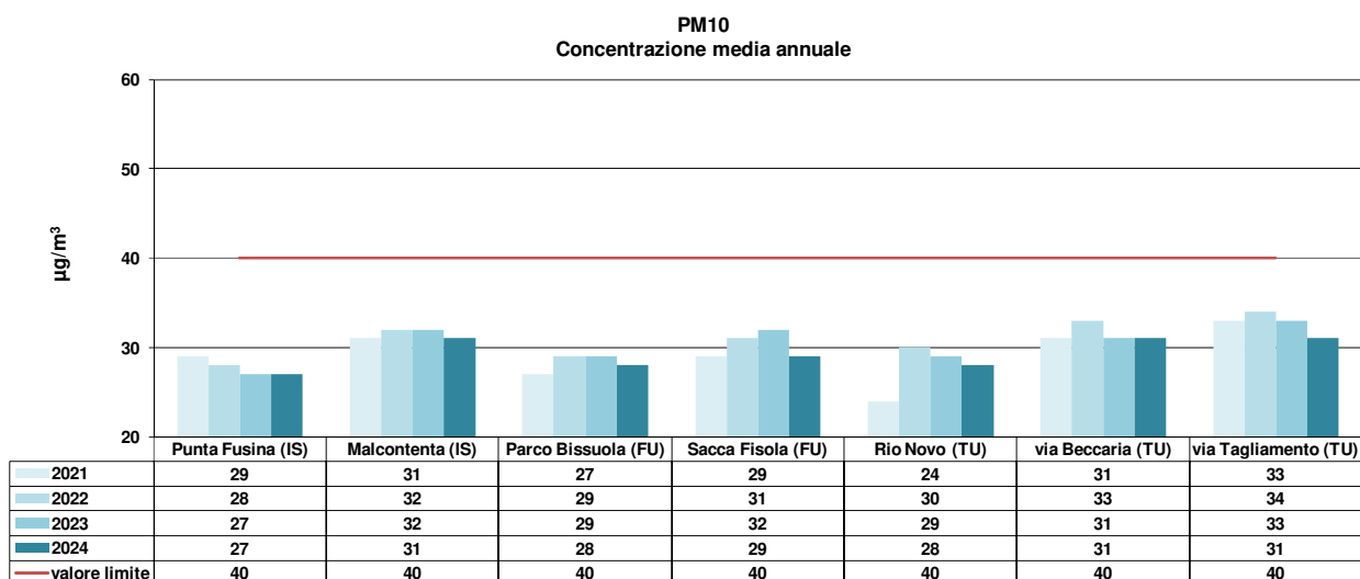
Grafico 18 – Concentrazioni medie annue di PM10 ( \mu\text{g}/\text{m}^3 ). Confronto tra Punta Fusina e le altre stazioni fisse presenti in Comune di Venezia. Anni dal 2021 al 2024
