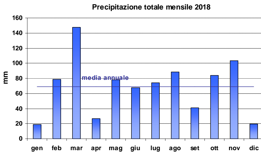
Grafico 9: Precipitazione totale mensile anno 2018.
