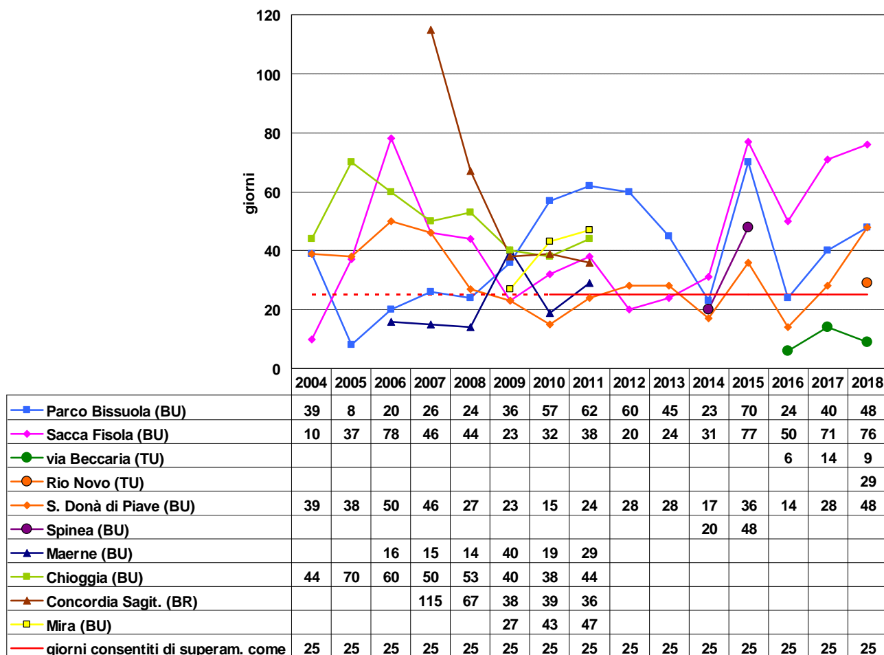
O3: numero di giorni di superamento del valore obiettivo per la protezione della salute umana (Dlgs 155/10)
