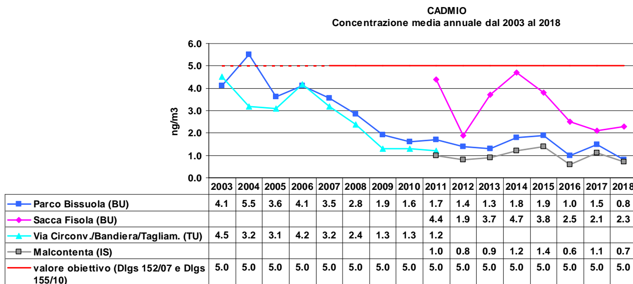
Grafico 53: Confronto tra le concentrazioni medie annuali di cadmio in riferimento al valore obiettivo di 5.0 ng/m 3 in vigore dal 2007. Dal 2003 al 2006 il valore limite annuale è indicato con la linea tratteggiata poiché, sebbene trattato dalla Direttiva Europea 2004/107/CE, è entrato in vigore solo dal 2007 (Dlgs 152/07).
