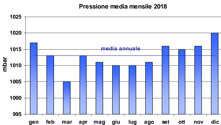
Grafico 8: Pressione media mensile anno 2018.
