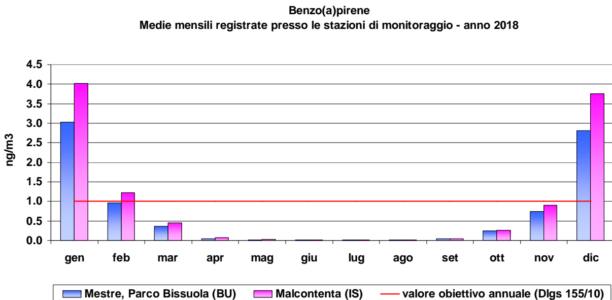
Grafico 34: Medie mensili di benzo(a)pirene registrate presso le stazioni di monitoraggio nel 2018.
