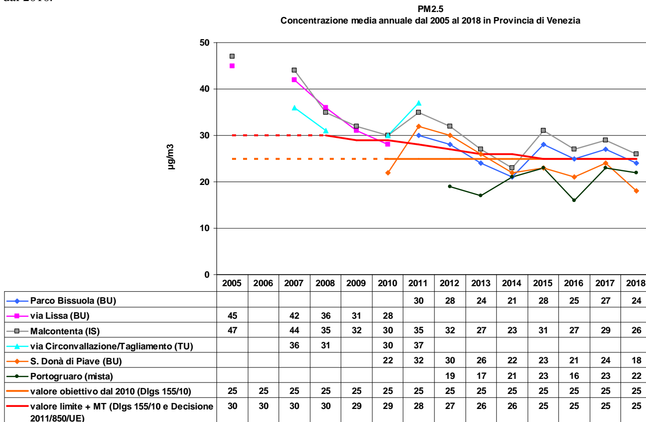
Grafico 49: Confronto tra le concentrazioni medie annuali di PM 2.5 in riferimento al valore limite annuale di 25 µg/m 3 valido dal 2015, aumentato del margine di tolleranza dal 2008 al 2014, ed il valore obiettivo sempre di 25 µg/m 3 valido dal 2010.
