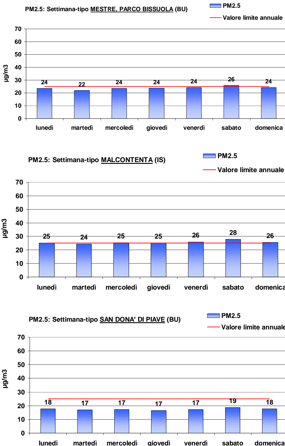
Grafico 31: Settimana tipo della concentrazione di polveri inalabili PM 2.5 misurata nelle tre stazioni di monitoraggio.
