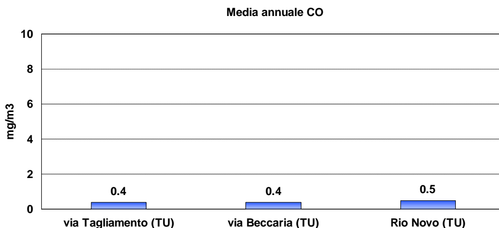
Grafico 16: Media annuale CO, anno 2018.
