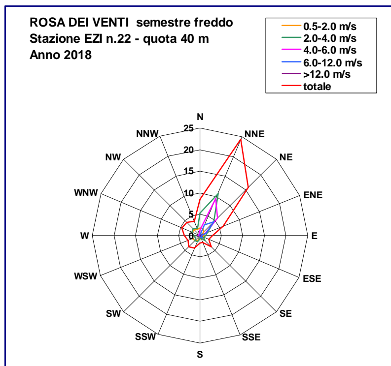
Grafico 14: Rosa dei venti semestre freddo 2018.
