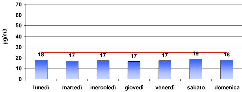
PM2.5: Settimana-tipo PORTOGRUARO (mista)
