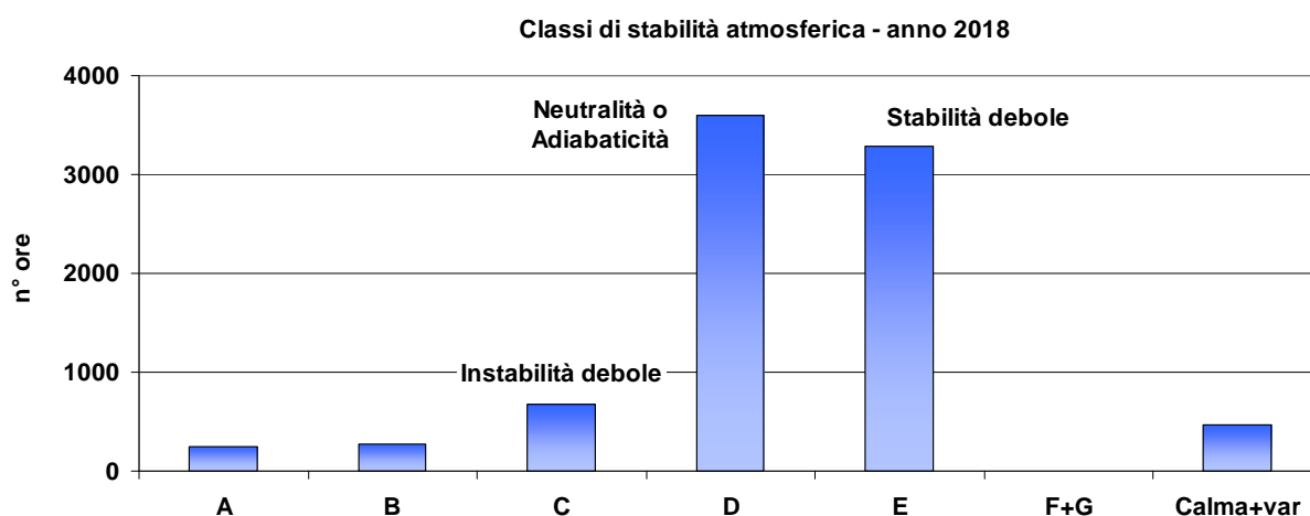
Grafico 10: Classi di stabilità atmosferica - anno 2018.
