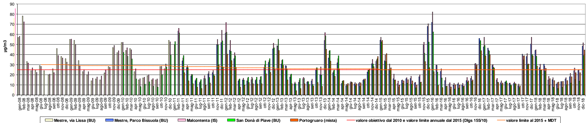
Polveri fini - PM 2,5 Medie mensili registrate presso le stazioni storiche di monitoraggio
