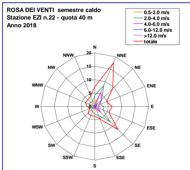
Grafico 13: Rosa dei venti semestre caldo 2018.
