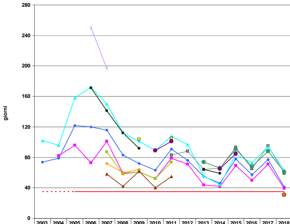
PM10 Numero di giorni di superamento del valore limite giornaliero di 50 µg/m 3 dal 2003 al 2018 in Provincia di Venezia
