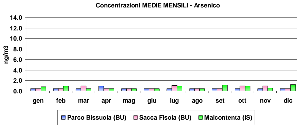
Grafico 36: Confronto delle concentrazioni medie mensili 2018 di arsenico, cadmio, nichel e piombo nelle tre stazioni di monitoraggio della Rete provinciale ARPAV.
