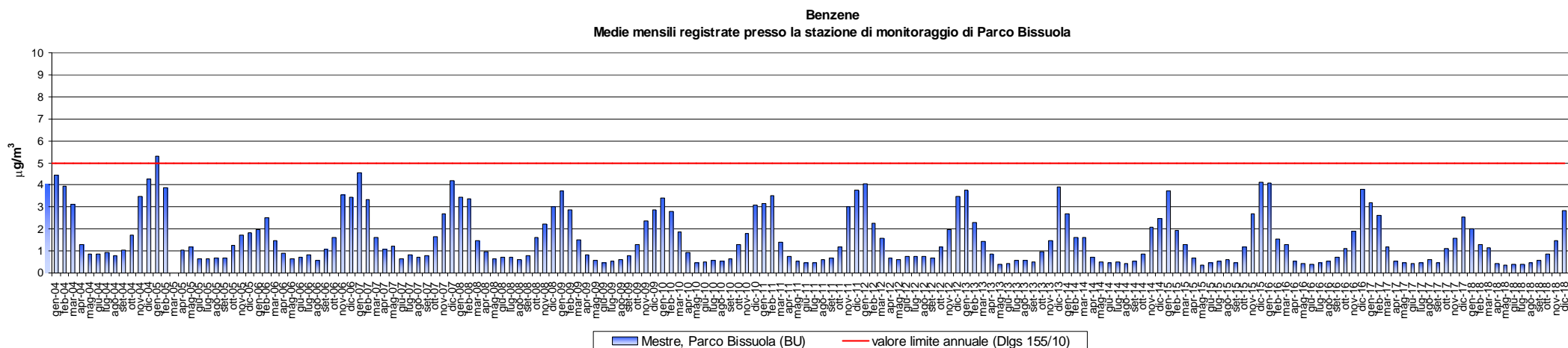
Grafico 42: Medie mensili di benzene registrate presso la stazione storica di monitoraggio di Mestre - Parco Bissuola da gennaio 2004 a dicembre 2018.
