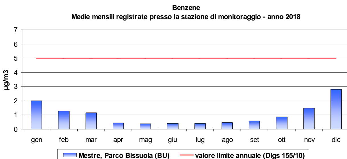
Grafico 32: Medie mensili di benzene registrate nel 2018 presso la stazione della Rete di Monitoraggio di Mestre ó Parco Bissuola.
