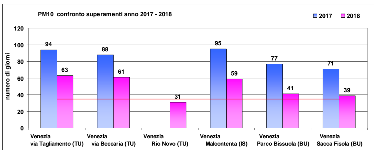
Grafico 26: Numero di superamenti del valore limite di 24 ore per il PM 10 per la protezione della salute umana a confronto con l'anno precedente. Si ricorda che la stazione di Rio Novo è attiva dal 1 settembre 2017.
