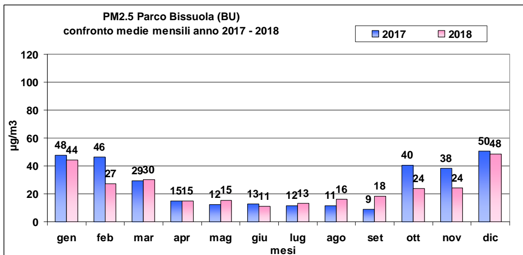
Grafico 29: Confronto delle medie mensili registrate durante l'anno 2017 e 2018 presso le stazioni di monitoraggio di PM 2.5 in Provincia di Venezia.
