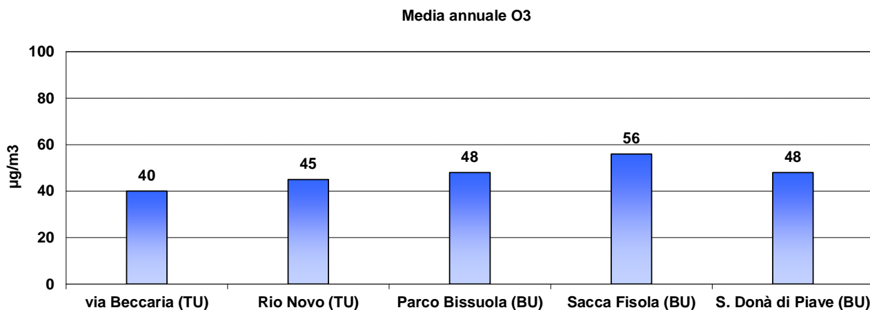
Grafico 19: Media annuale ozono, anno 2018.
