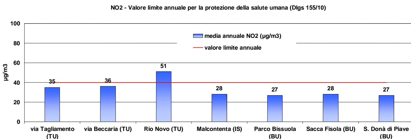
Grafico 17: Confronto della media annuale 2018 delle concentrazioni orarie di NO 2 con il valore limite annuale per la protezione della salute umana (Dlgs 155/10).
