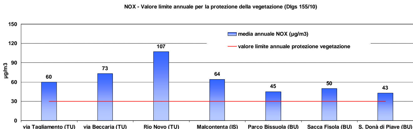
Grafico 18: Confronto della media annuale 2018 delle concentrazioni orarie di NO x con il valore limite annuale di protezione degli ecosistemi (Dlgs 155/10).
