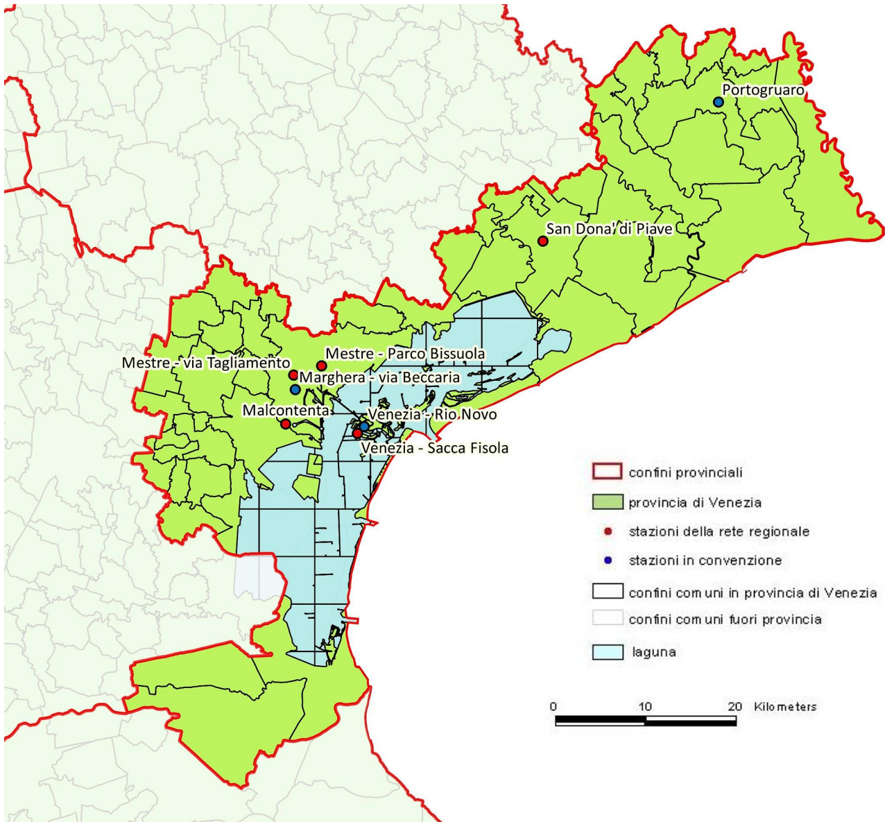
Figura 1: Localizzazione delle stazioni di misura dell'inquinamento atmosferico in Provincia di Venezia ó anno 2018.
