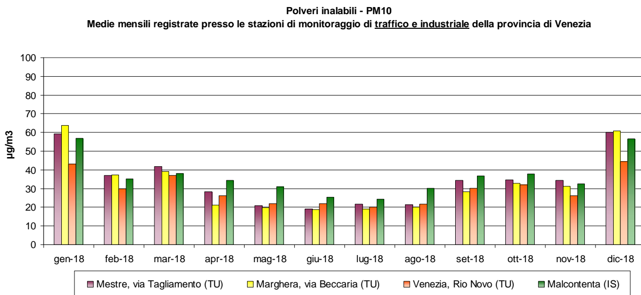
Grafico 23: Medie mensili di PM 10 registrate presso le stazioni di monitoraggio di traffico e industriale della Provincia di Venezia nel 2018.
