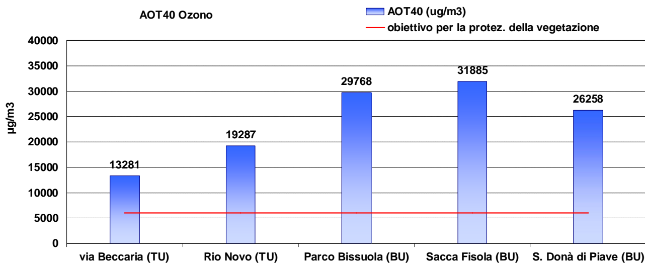
Grafico 21: AOT40 calcolato sulla base dei dati orari rilevati dal 1 maggio al 31 luglio 2018.
