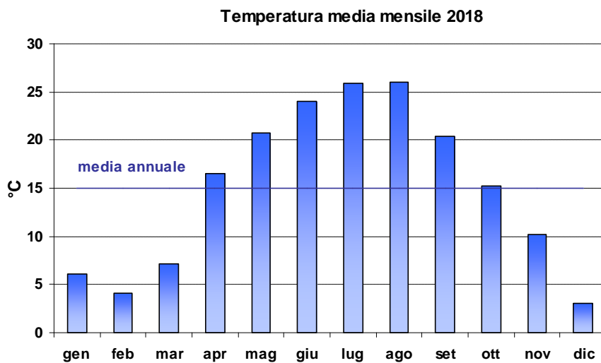
Grafico 5: Temperatura media mensile anno 2018.
