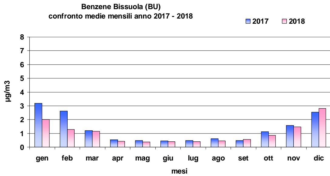
Grafico 33: Confronto delle medie mensili di benzene registrate durante gli anni 2017 e 2018 presso la stazione storica di monitoraggio di Mestre - Parco Bissuola.
