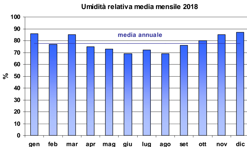
Grafico 7: Umidità relativa media mensile anno 2018.
