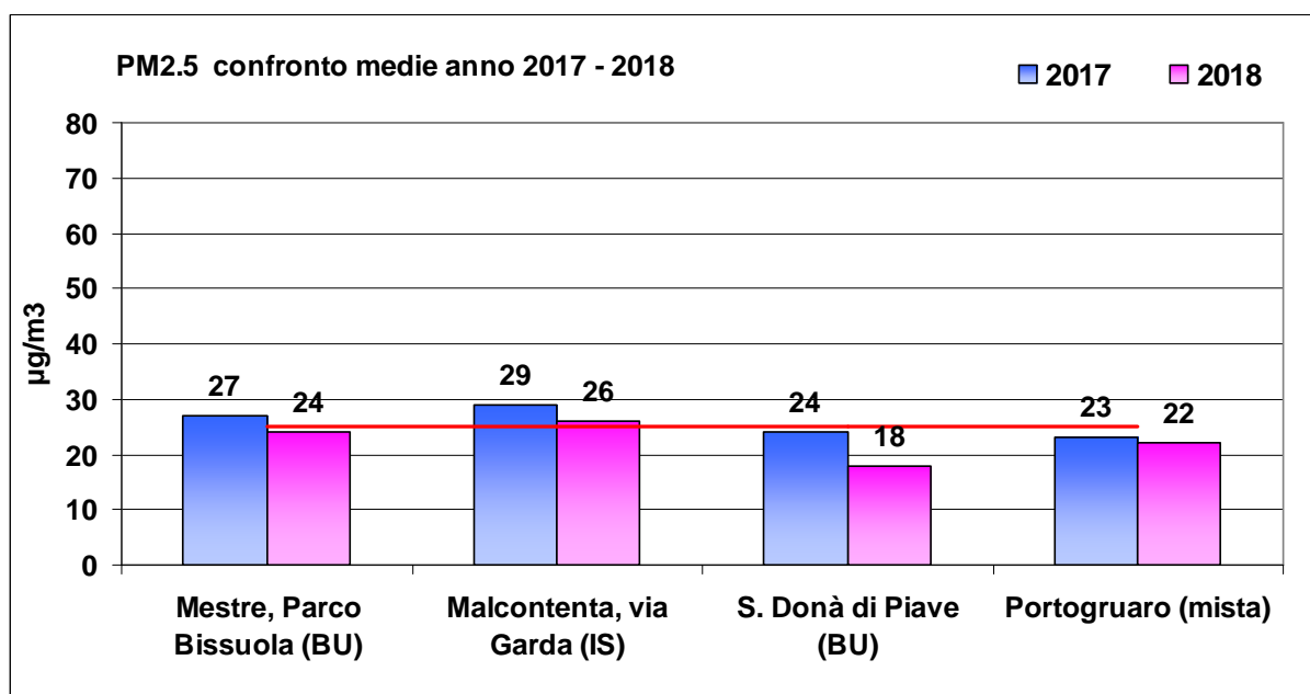
Grafico 30: Media annuale della concentrazione di PM 2.5 in Provincia di Venezia a confronto con l'anno precedente e con il valore limite (linea rossa).
