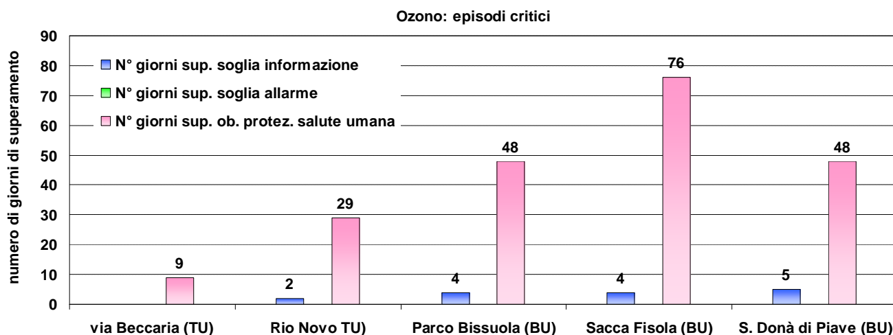
Grafico 20: Numero di giorni in cui si è verificato almeno un superamento della soglia di informazione di O 3 o della soglia di allarme o dell'obiettivo a lungo termine per la protezione della salute umana nell'anno 2018.
