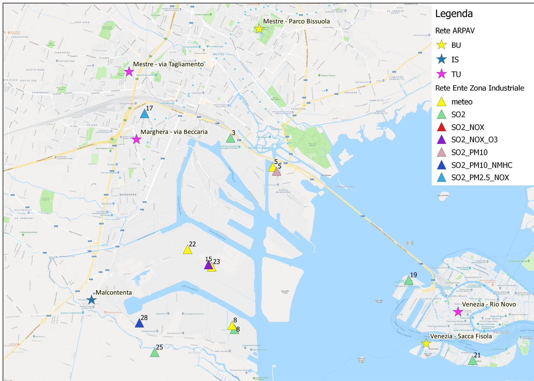
Figura 2: Localizzazione delle stazioni di misura di ARPAV e dell'Ente Zona Industriale di Porto Marghera, attive in Comune di Venezia nell'anno 2018.
