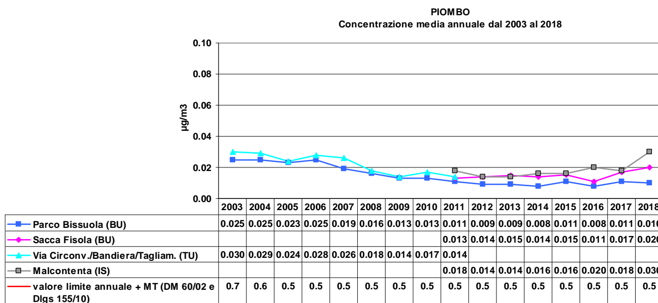
Grafico 51: Confronto tra le concentrazioni medie annuali di piombo. Il valore limite è pari a 0.5 \mu\text{g}/\text{m}^3 (aumentato del margine di tolleranza prima del 2005).
