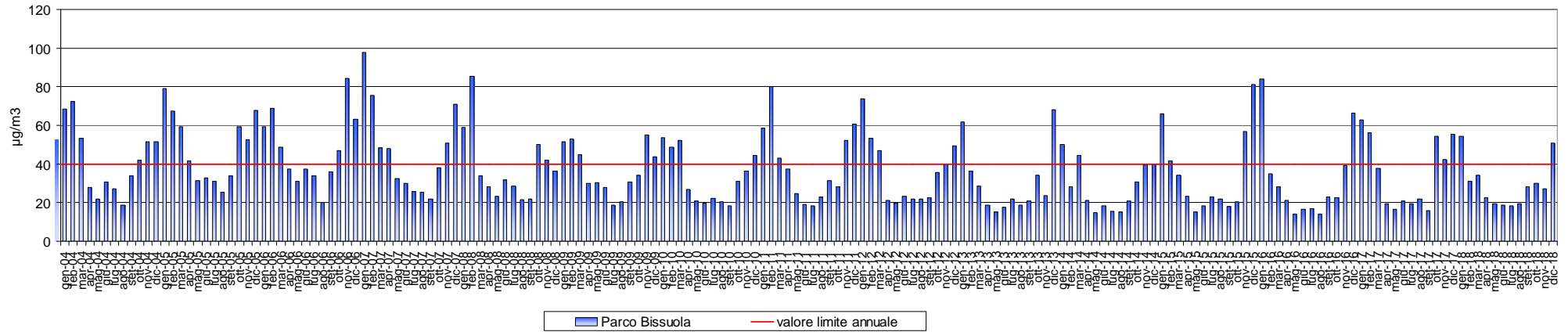
Polveri inalabili - PM10 Medie mensili registrate presso la stazione di monitoraggio di Parco Bissuola a Mestre
