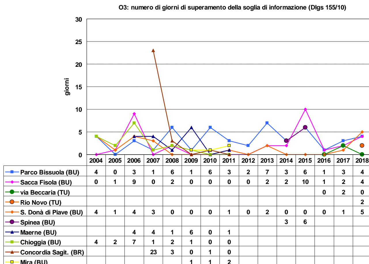
Grafico 39: Numero di giorni di superamento della soglia di informazione per l'O 3 di 180 µg/m 3 nelle stazioni di monitoraggio della Provincia di Venezia.
