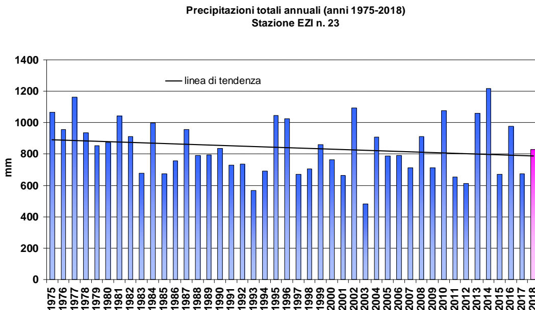
Grafico 4: Precipitazioni totali annuali
