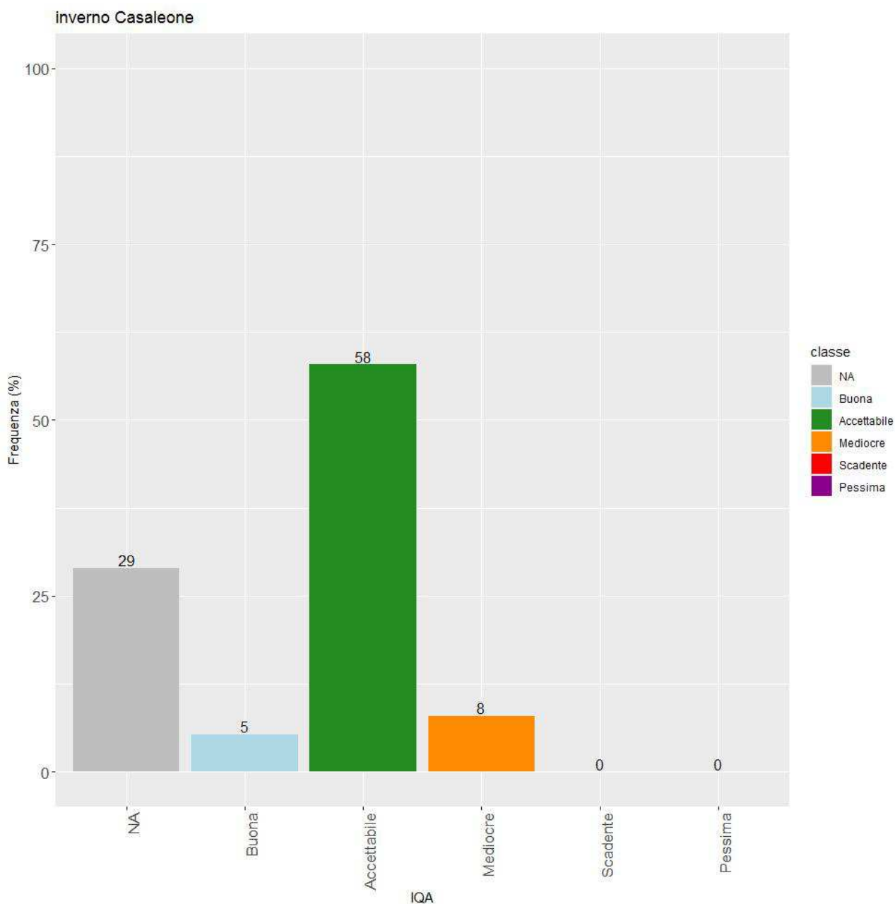
Figura 11. Indice di Qualità dell'aria a Casaleone, campagna INVERNO: frequenza delle diverse "classi" di qualità dell'aria. Elaborazione eseguita a partire da tutti i dati disponibili per Casaleone. NA (Not Available, non disponibile), è relativo alle giornate in cui non è stato possibile calcolare l'indice, a causa della mancanza di dati.
