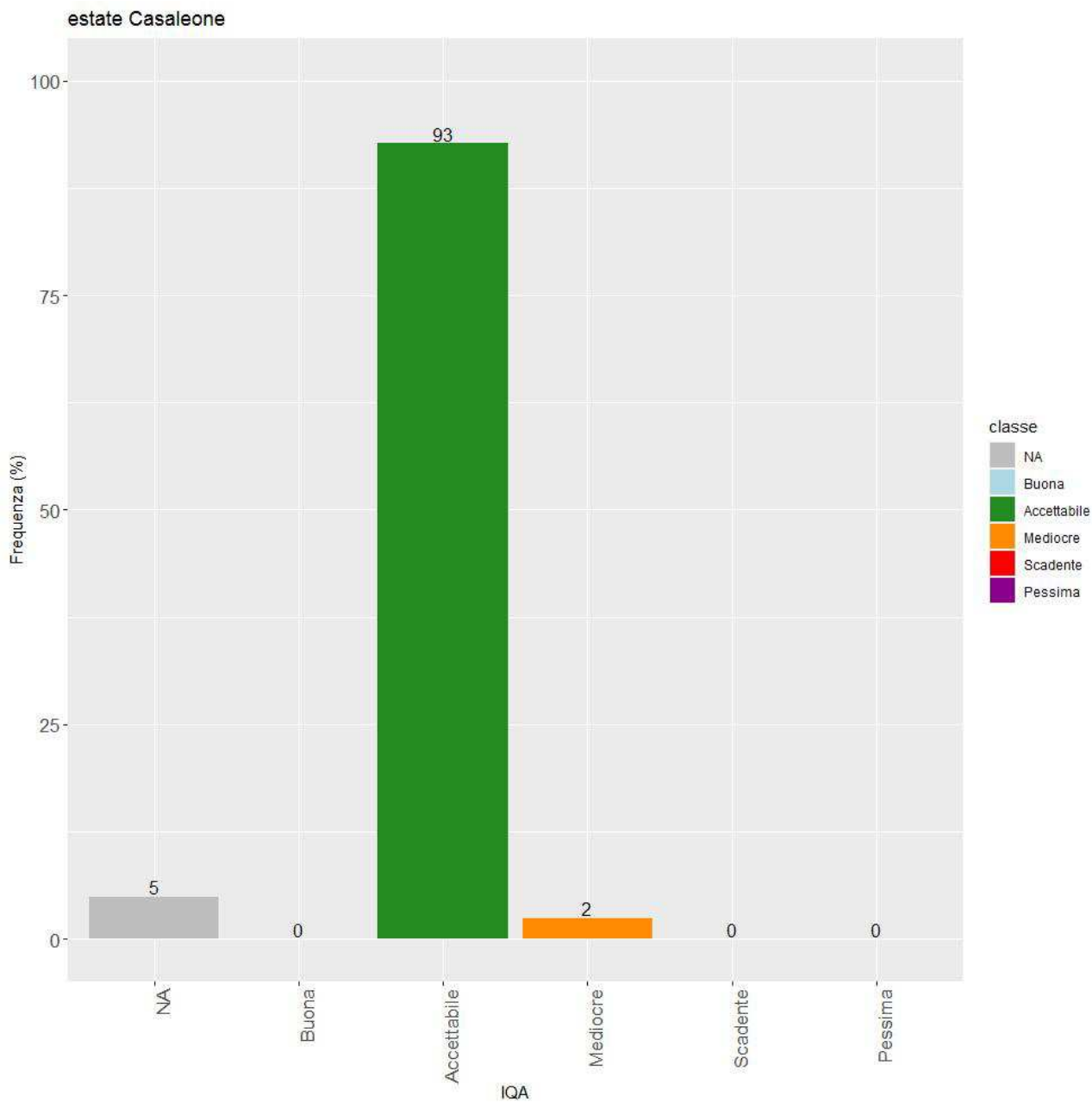
Figura 10. Indice di Qualità dell'aria a Casaleone, campagna ESTIVA: frequenza delle diverse "classi" di qualità dell'aria. Elaborazione eseguita a partire da tutti i dati disponibili per Casaleone. NA (Not Available, non disponibile), è relativo alle giornate in cui non è stato possibile calcolare l'indice, a causa della mancanza di dati.
