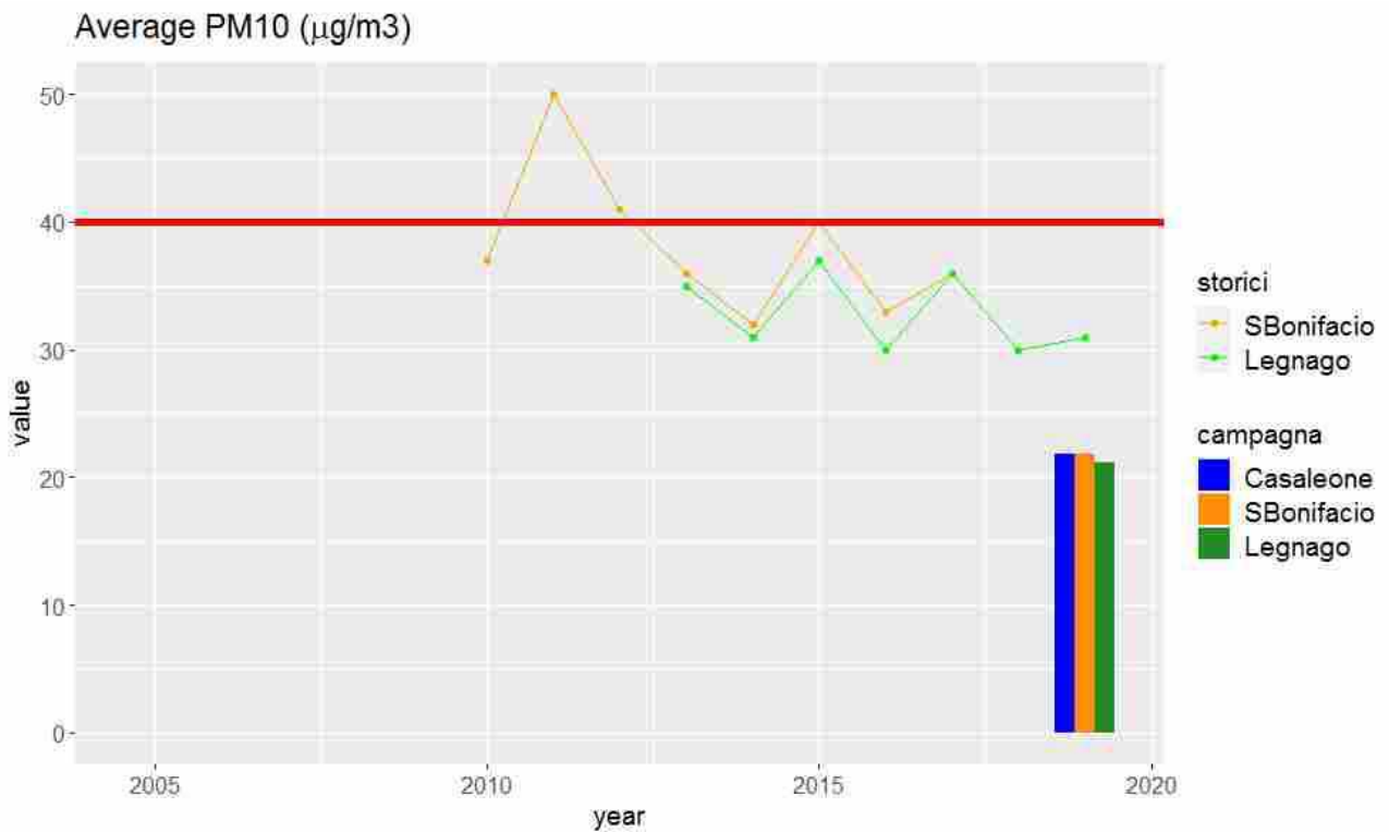
Figura 15. PM10: concentrazione media annua misurata dalle centraline fisse di San Bonifacio e Legnago, e concentrazione media durante le campagne di misura del 2019, misurata dal mezzo mobile a Casaleone, e dalle centraline di San Bonifacio e Legnago (come in figura 14). La linea orizzontale rossa corrisponde al limite annuale.
