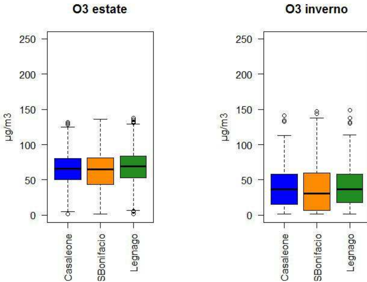
Figura 8. Box-plot della concentrazione di O 3 . Dati relativi a Casaleone e alla centralina di riferimento di Legnago. Campagna di misura estiva (pannello a sinistra) e invernale (pannello a destra).
