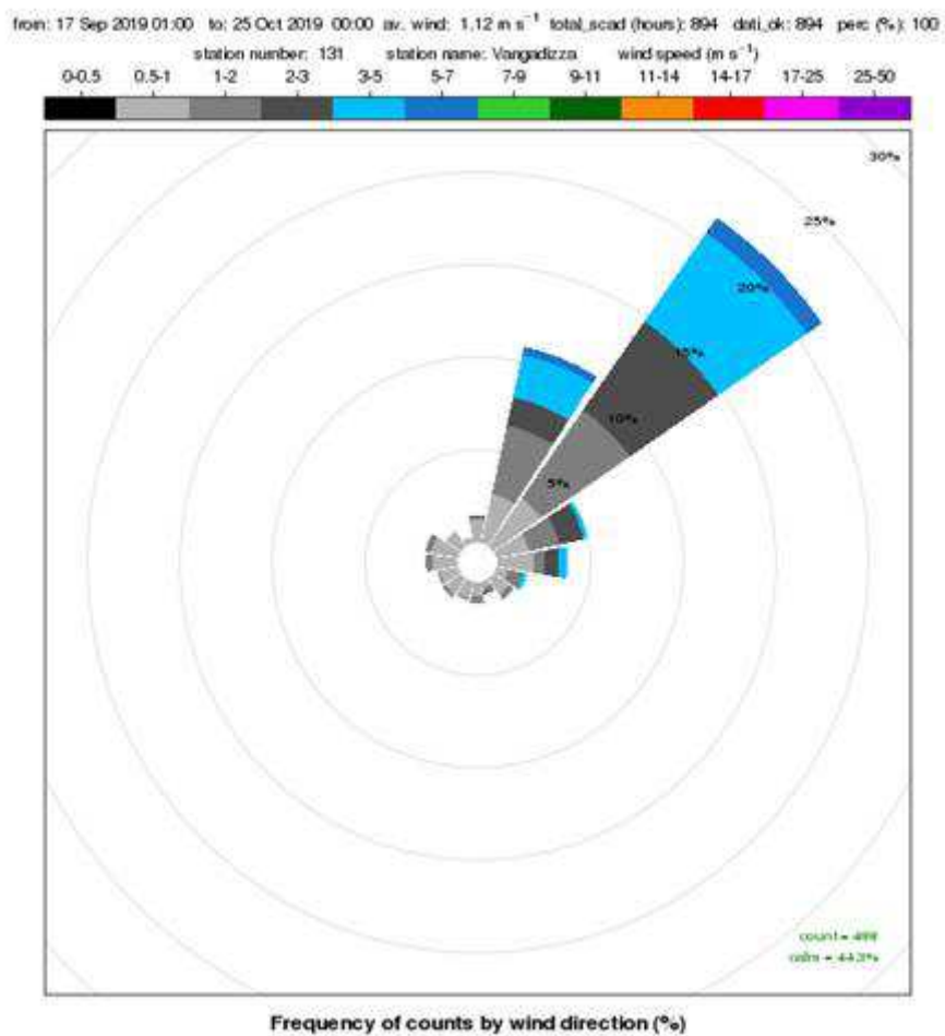
Figura 6: rosa dei venti registrati presso la stazione meteorologica di Vangadizza nel periodo 17 settembre – 24 ottobre 2019
