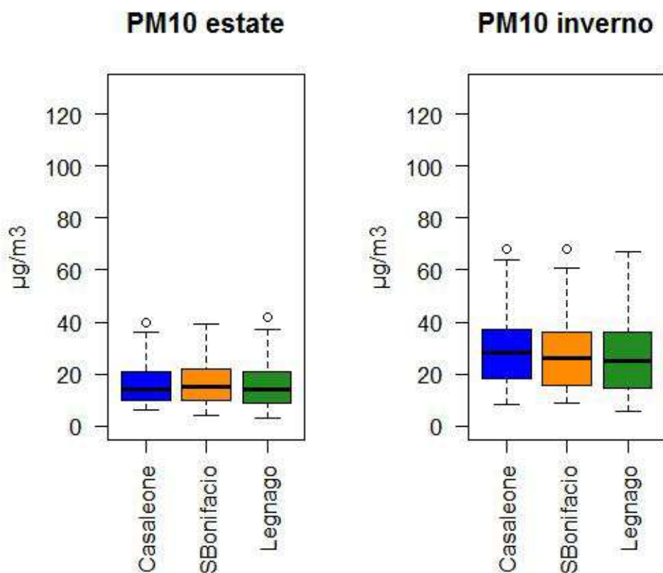
Figura 9. Box-plot della concentrazione di PM 10 . Dati relativi a Casaleone e alle centraline di riferimento di San Bonifacio e Legnago. Campagna di misura estiva (pannello a sinistra) e invernale (pannello a destra).
