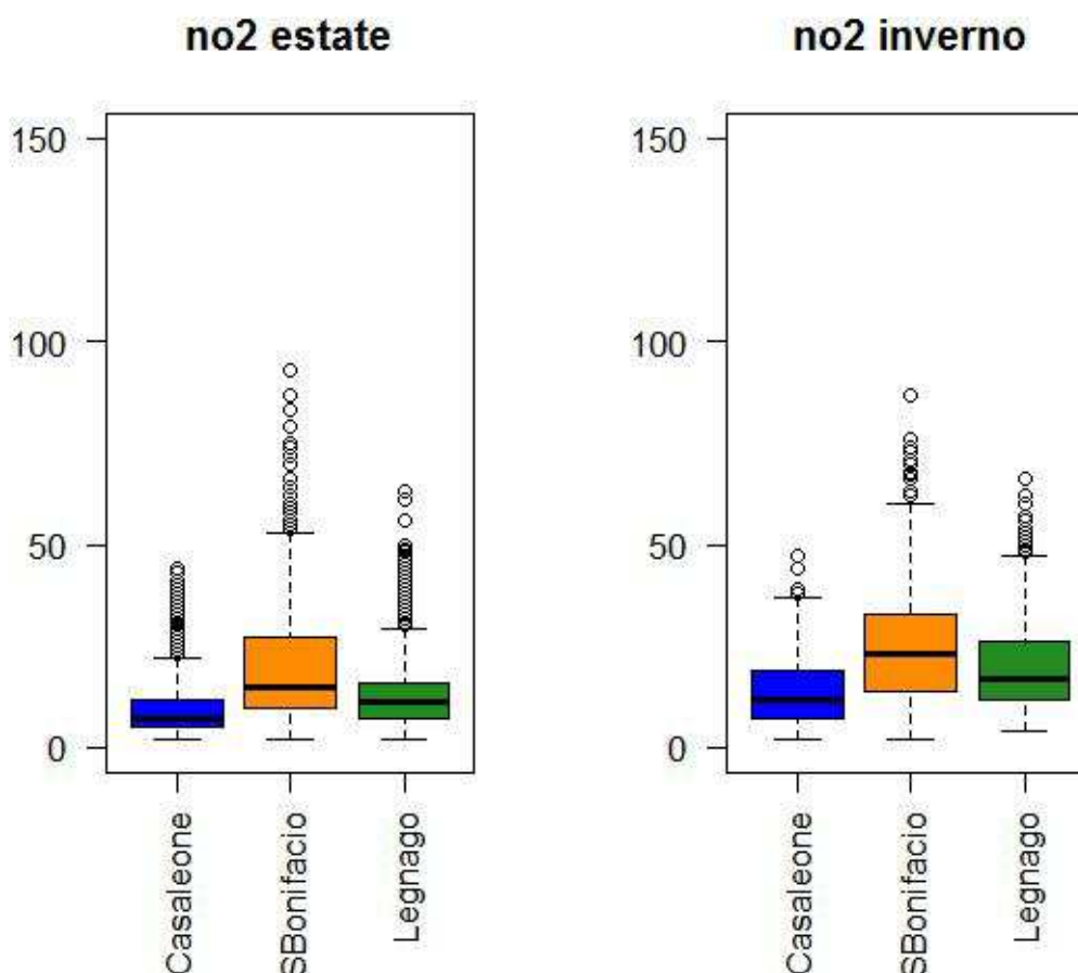
Figura 7. Box-plot della concentrazione di NO 2 . Dati relativi a Casaleone e alle due centraline di riferimento di San Bonifacio e Legnago. Campagna di misura estiva (pannello a sinistra) e invernale (pannello a destra).
