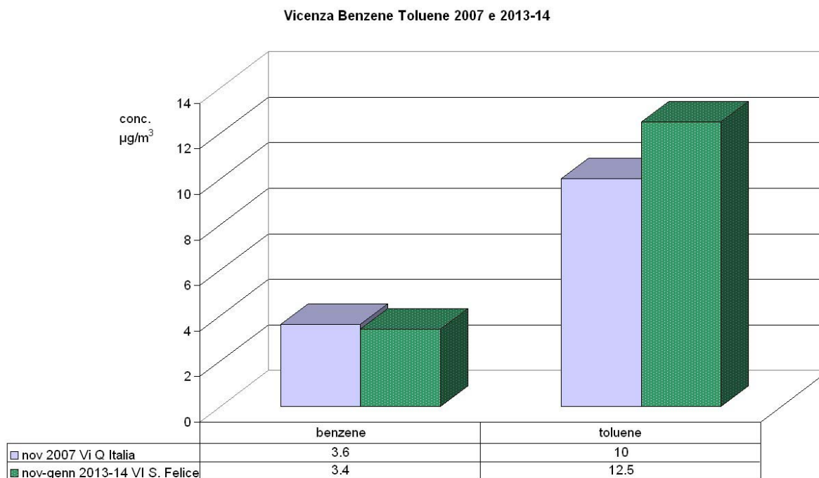
Figura 10 andamento delle concentrazioni medie di benzene e toluene a Vicenza
