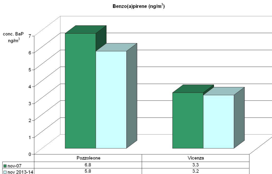
Figura 8 Benzo(a)pirene a Pozzoleone e a Vicenza quartiere Italia, stessi periodi a confronto.
