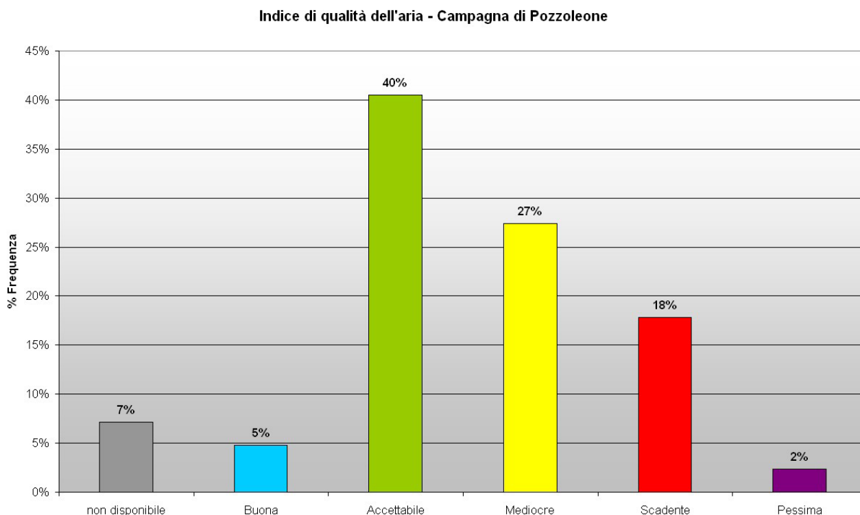
Figura 7: Calcolo dell'indice sintetico di qualità dell'aria per la campagna Pozzoleone 2013-2014
