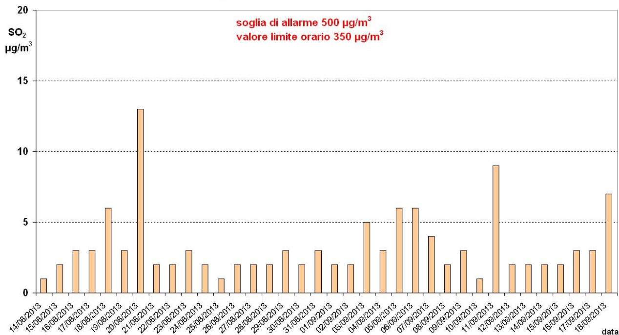
SO 2 massima giornaliera della media oraria agosto settembre 2013 Pozzoleone
