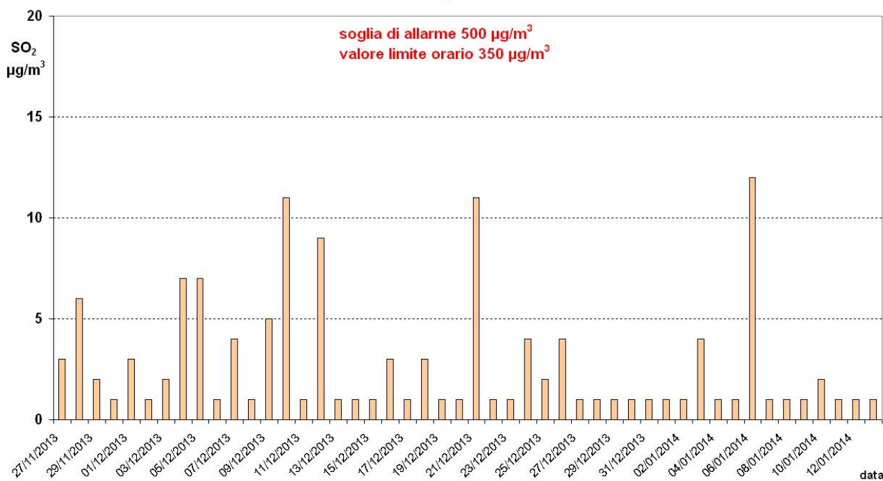
SO 2 massima giornaliera della media oraria novembre dicembre 2013 gennaio 2014 - Pozzoleone
