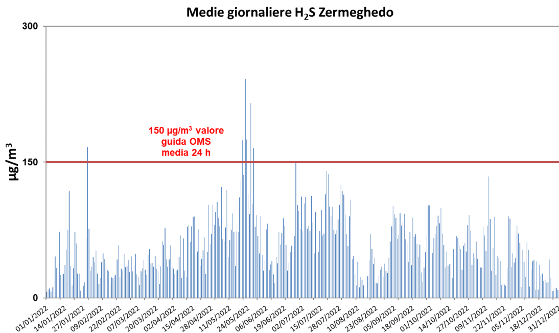
Grafico 1 Acido Solfidrico - Zermeghedo via Marconi medie giornaliere 2022
