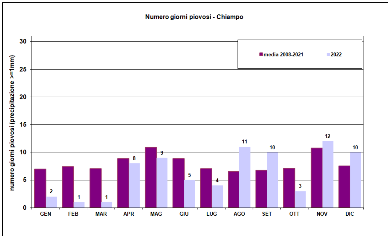
Figura 2: confronto del numero di giorni di pioggia (precipitazione giornaliera \geq 1 mm) mensili registrati nell'anno 2022 con la media di riferimento (anni 2008-2021) registrati presso la stazione di Chiampo.
