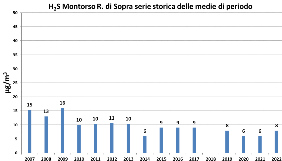
Grafico 8 H 2 S serie storiche delle medie di periodo, Montorso Vic. Via Roggia di Sopra
