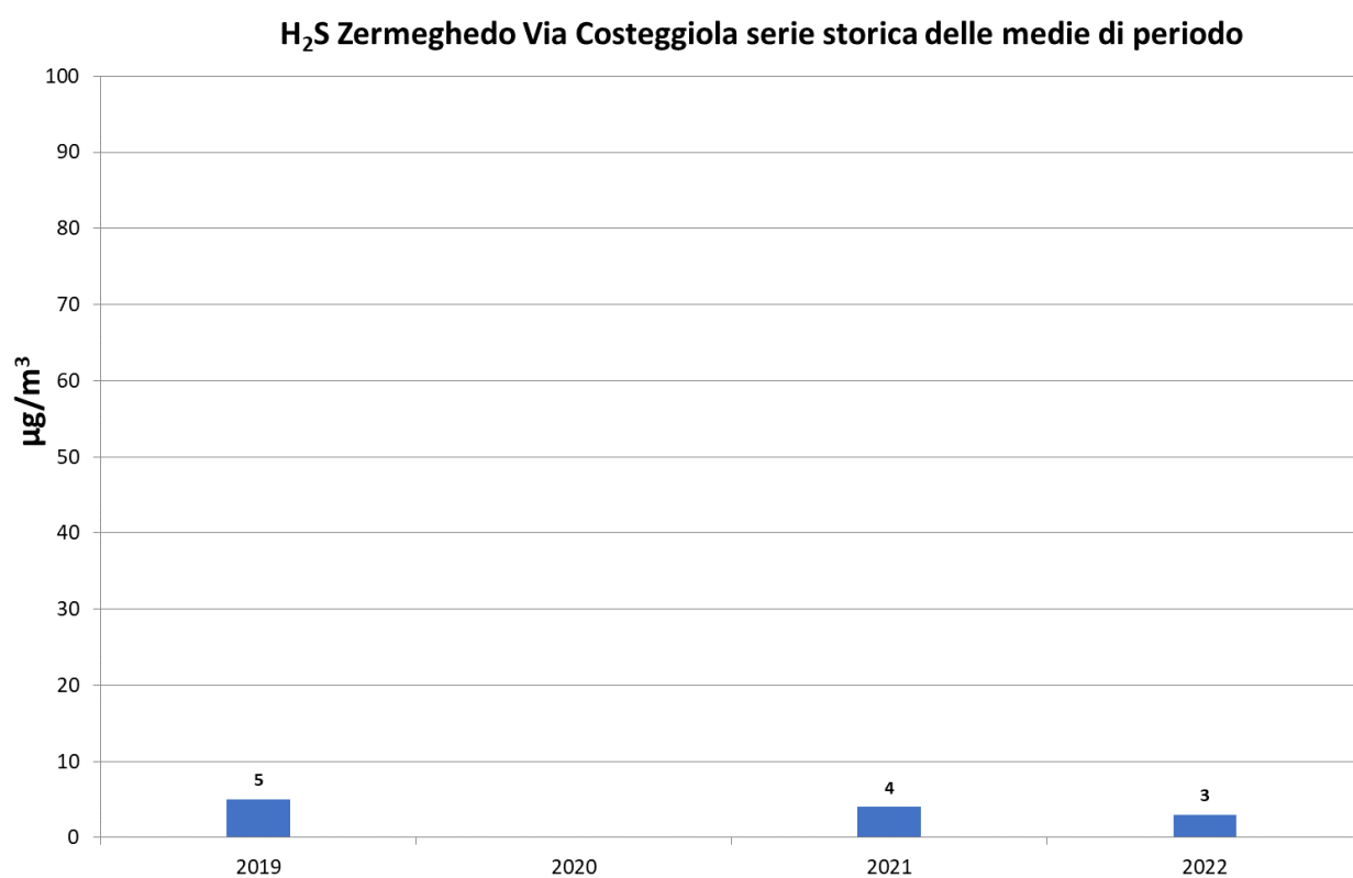
Grafico 13 H 2 S serie storiche delle medie di periodo, Zermeghedo Costeggiola
