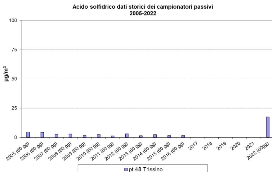
Grafico 17 medie complessive dal 2005 al 2022, Trissino punto 48
