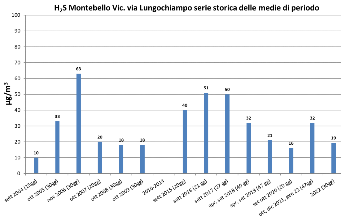
Grafico 10 H_2S serie storiche delle medie di periodo, Montebello via Lungochiampo
