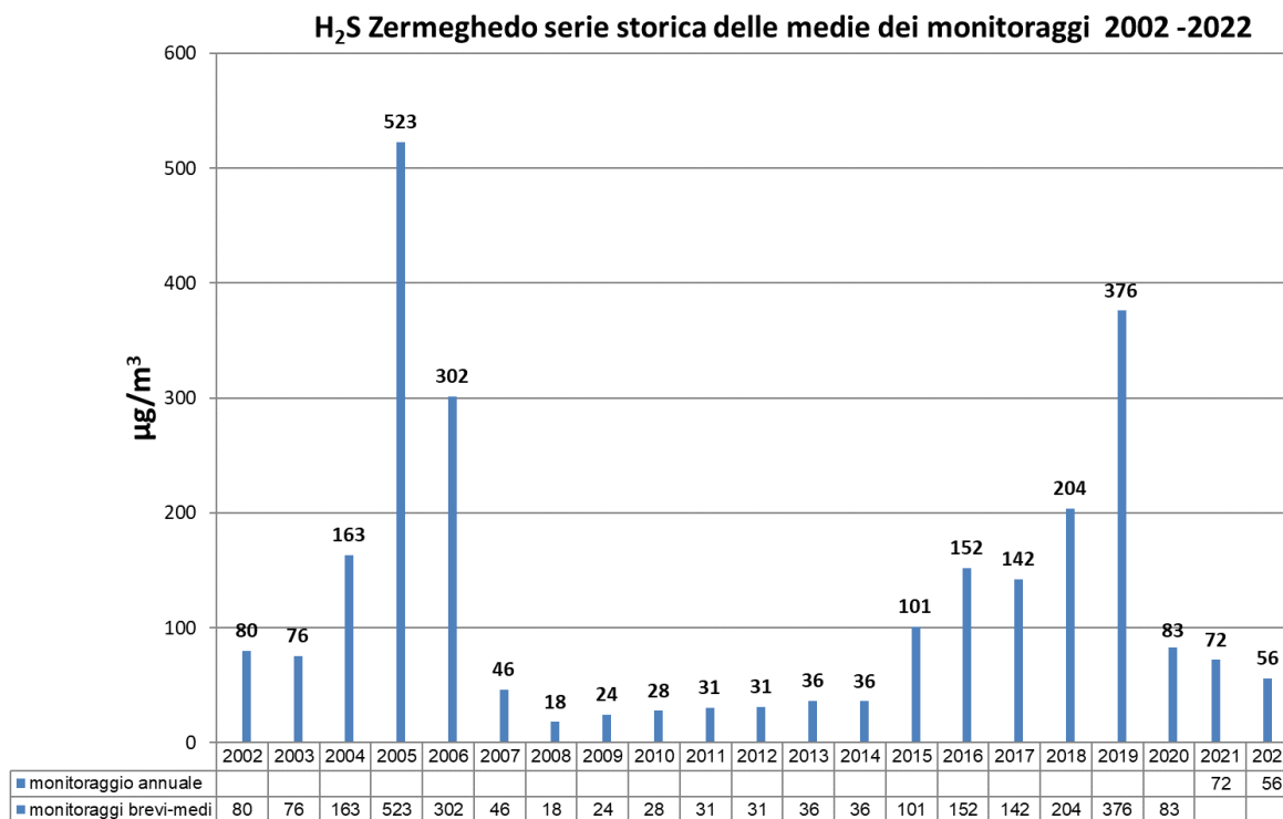
Grafico 6 H 2 S serie storiche delle medie di periodo, Zermeghedo Via Marconi
