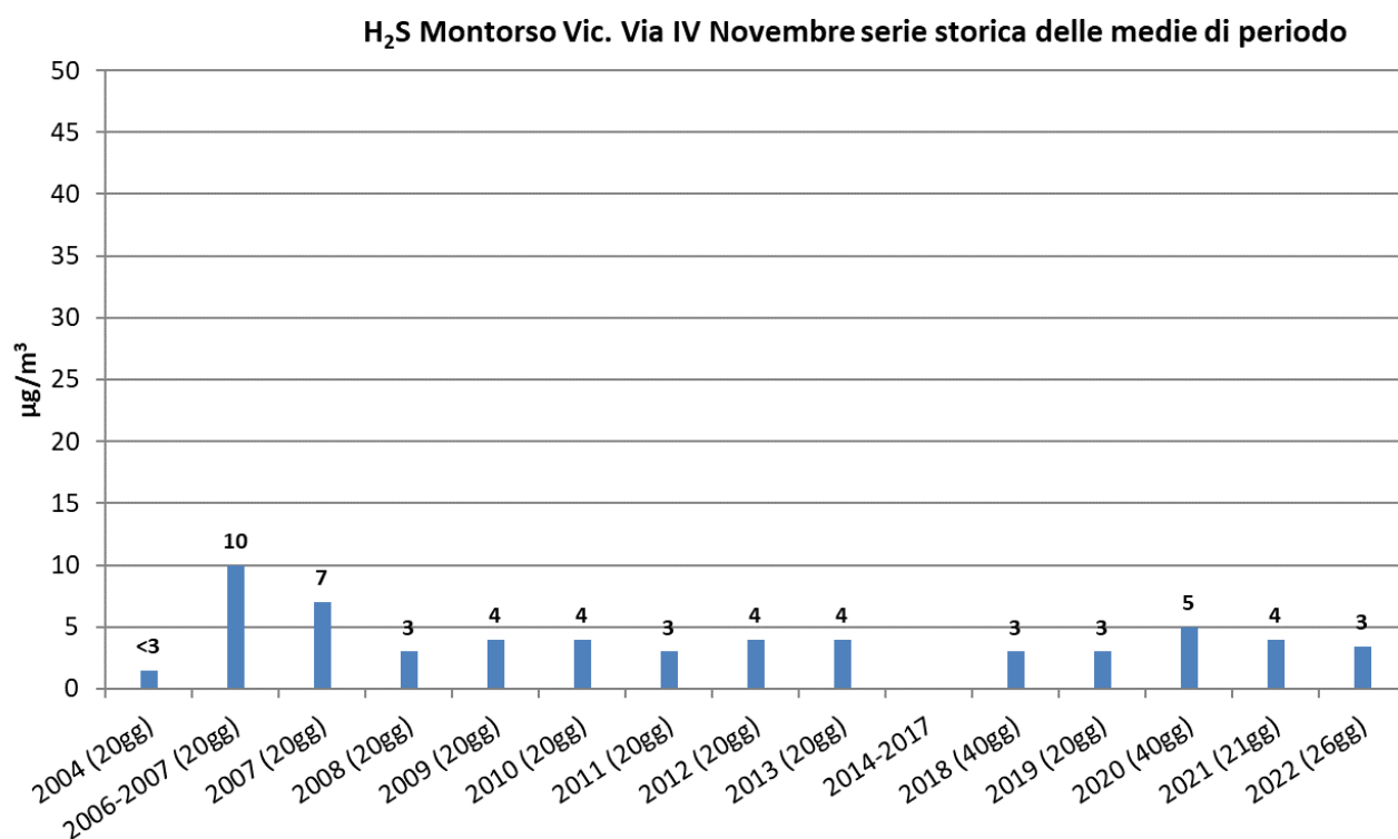
Grafico 12 H 2 S serie storiche delle medie di periodo, Montorso Vic. Via IV Novembre
