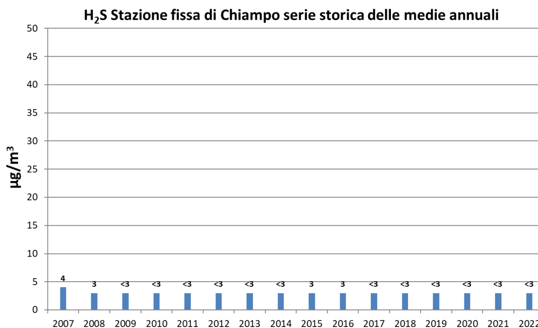
Grafico 7 H 2 S serie storiche delle medie annuali, stazione fissa di Chiampo Via dei Laghi
