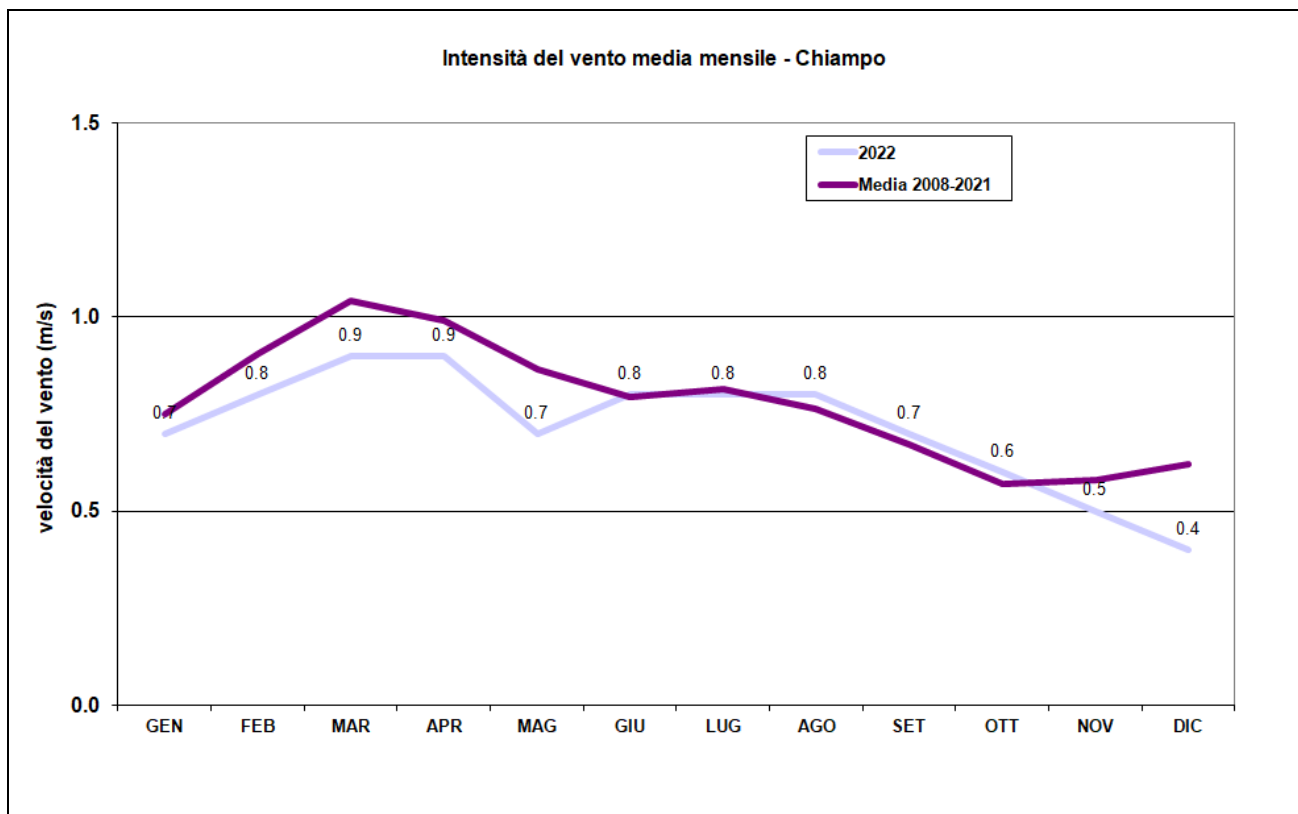
Figura 3: confronto delle intensità del vento medie mensili dell'anno 2022 con le rispettive medie (anni 2008-2021) rilevate presso la stazione di Chiampo.
