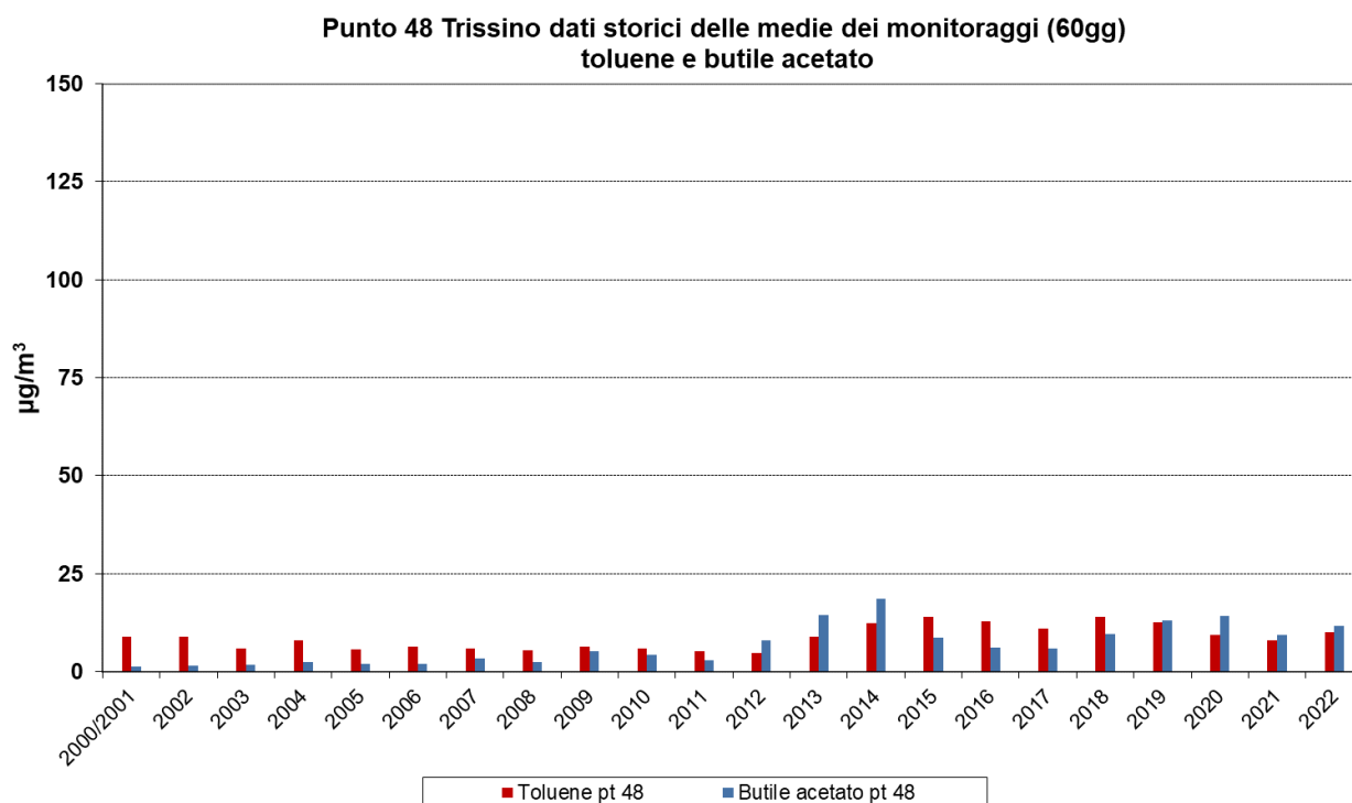
Grafico 29 andamento storico del toluene e del butile acetato (Trissino – punto 48)
