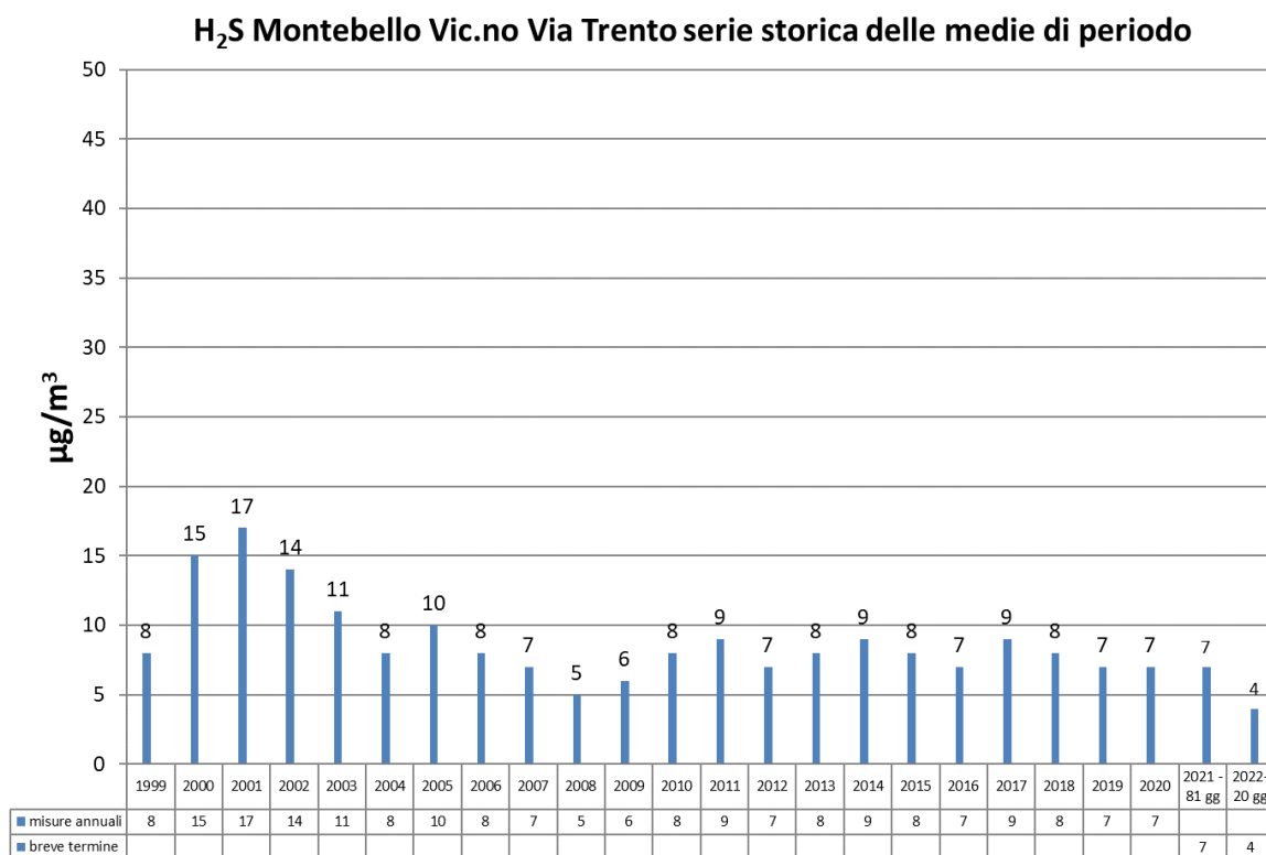
Grafico 9 H 2 S serie storiche delle medie di periodo, Montebello Vic. Via Trento
