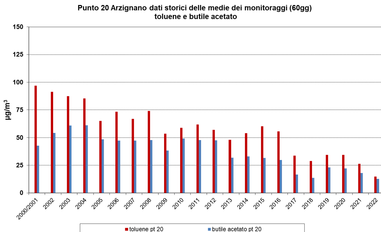
Grafico 25 andamento storico del toluene e del butile acetato (Arzignano - punto 20)
