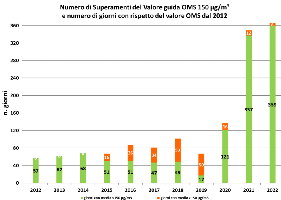
Grafico 5 \text{H}_2\text{S} serie storiche dei giorni di superamento del VG OMS, Zermeghedo
