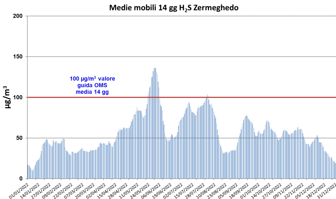
Grafico 2 Acido Solfidrico - Zermeghedo via Marconi medie mobili 14 giorni 2022
