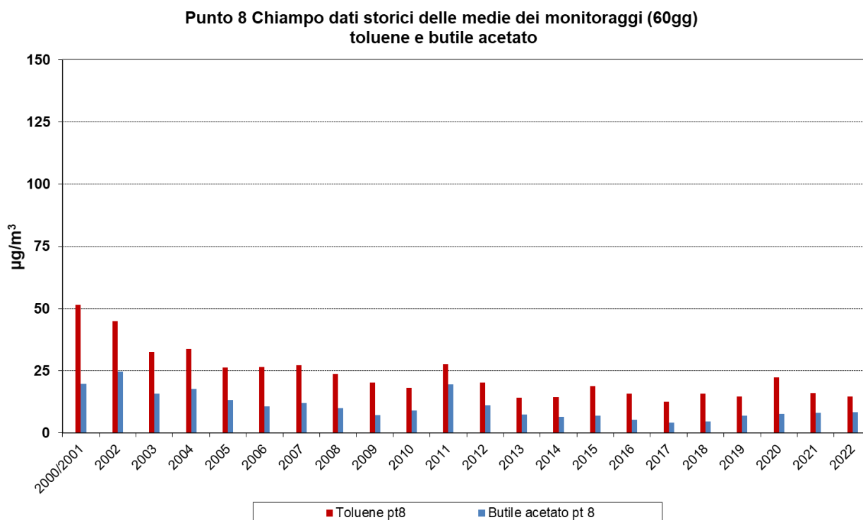
Grafico 24 andamento storico del toluene e del butile acetato (Chiampo - punto 8)
