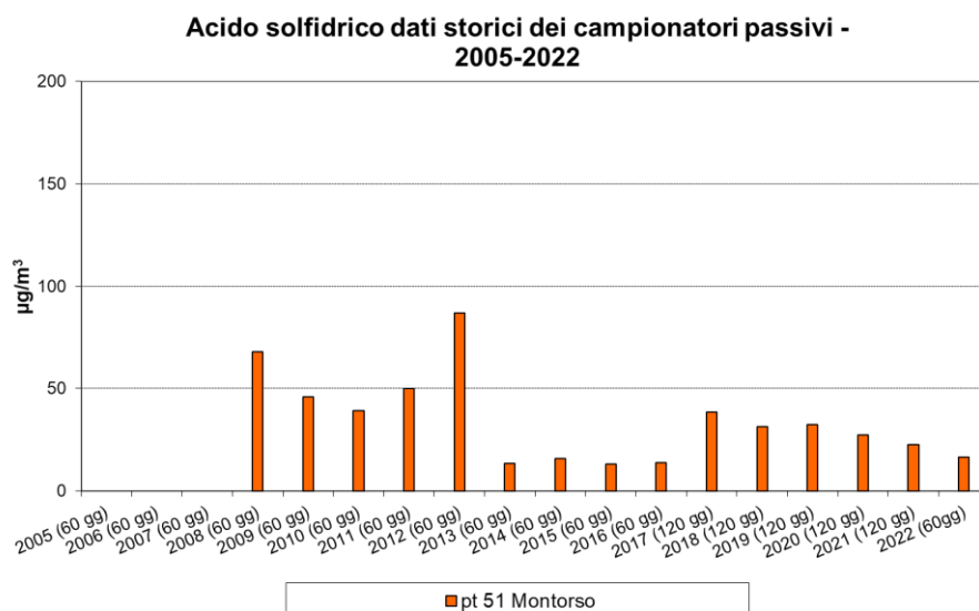
Grafico 18 medie complessive dal 2008 al 2022 Montorso Vic. pt 51
