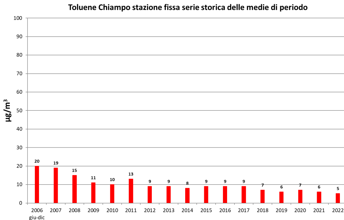
Grafico 14 Toluene, storico delle medie annuali a Chiampo
