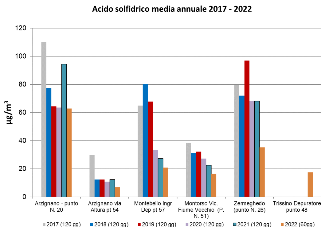
Grafico 16 medie complessive dal 2017 al 2022 per ciascun punto
