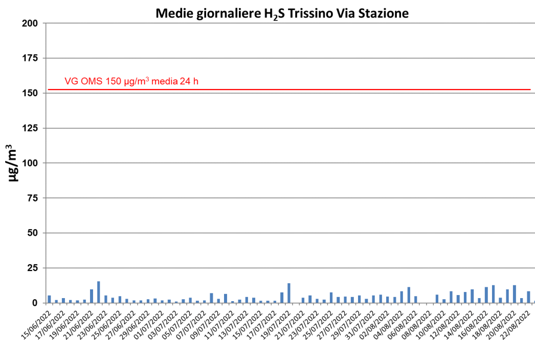
Grafico 4 Acido Solfidrico - Trissino Va Stazione medie giornaliere 2022
