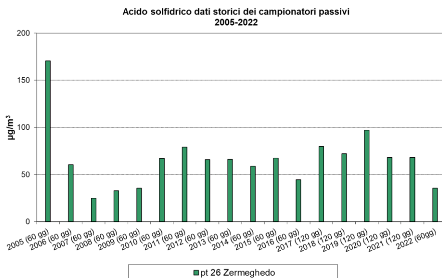
Grafico 19 medie complessive dal 2005 al 2022 Zermeghedo pt 26
