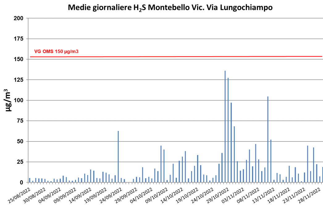
Grafico 3 Acido Solfidrico - Montebello Vic. Via Lungochiampo medie giornaliere 2022
