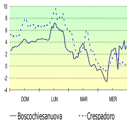
Temperatura aria 2m (°C) ultimi 4 g.
